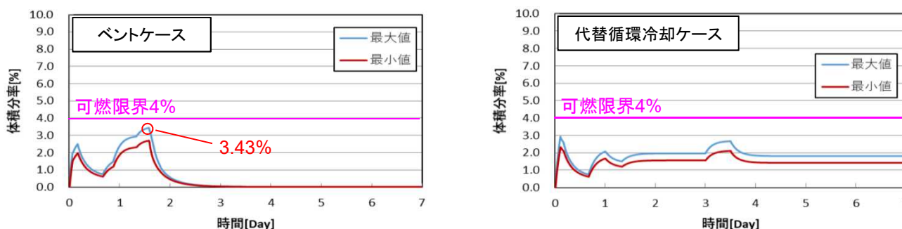
図7 【解析モデル修正後(設工認条件)】 上部D/W機器搬入用ハッチ室 水素体積分率時間推移
