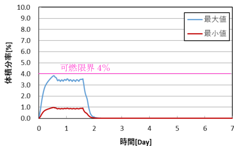
図 1.2.29 サプレッションチェンバ出入口室の水素濃度推移（局所エリア水素発生量増加格納容器ベントケース）
