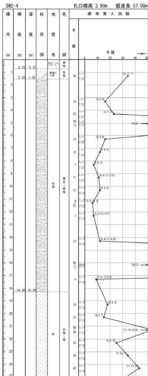
添付 1-38 図(1/3) ボーリング柱状図・コア写真 (SW2-4)
