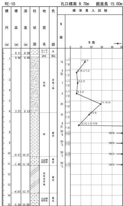
添付 1-22 図 ボーリング柱状図・コア写真 (RE-10)
