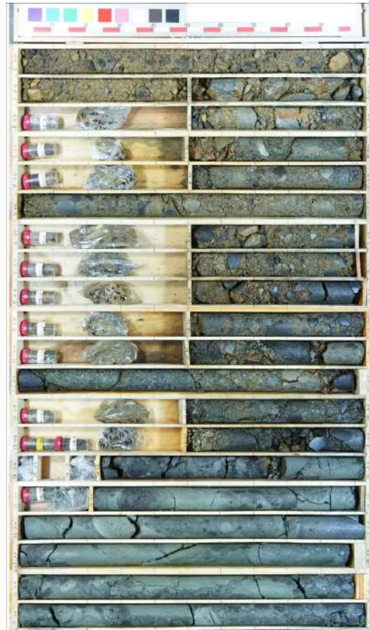
添付 1-1 図 ボーリング柱状図・コア写真 (SW2-3)
