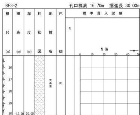
添付 1-27 図(2/2) ボーリング柱状図・コア写真 (BF3-2)
