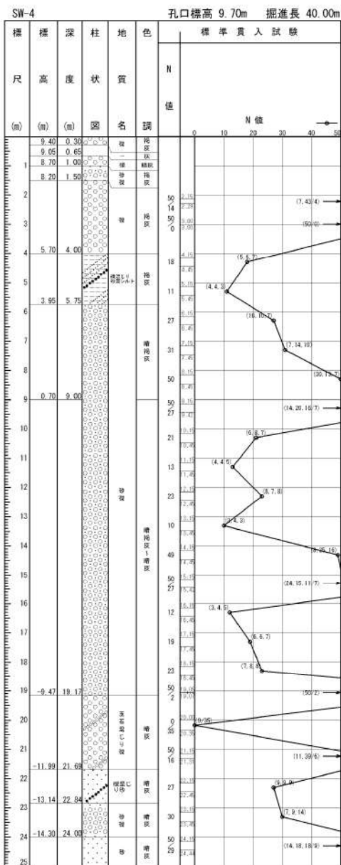
添付 1-35 図(1/2) ボーリング柱状図・コア写真 (SW-4)
