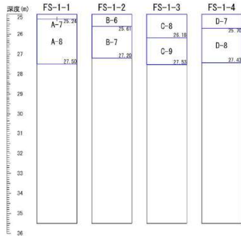
添付 1-39 図(2/10) ボーリング柱状図・コア写真 (FS-1)
