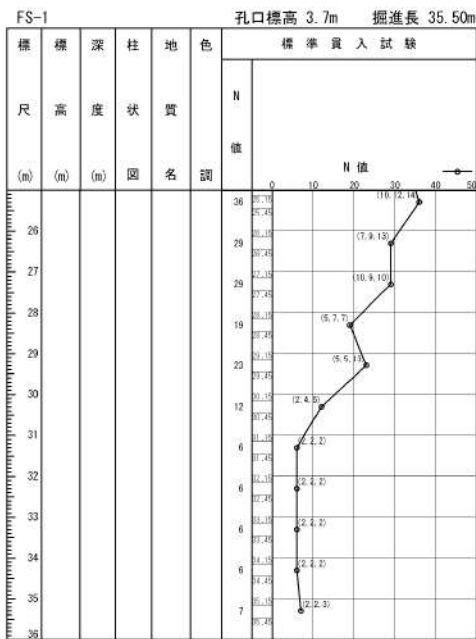
添付 1-39 図(2/10) ボーリング柱状図・コア写真 (FS-1)
