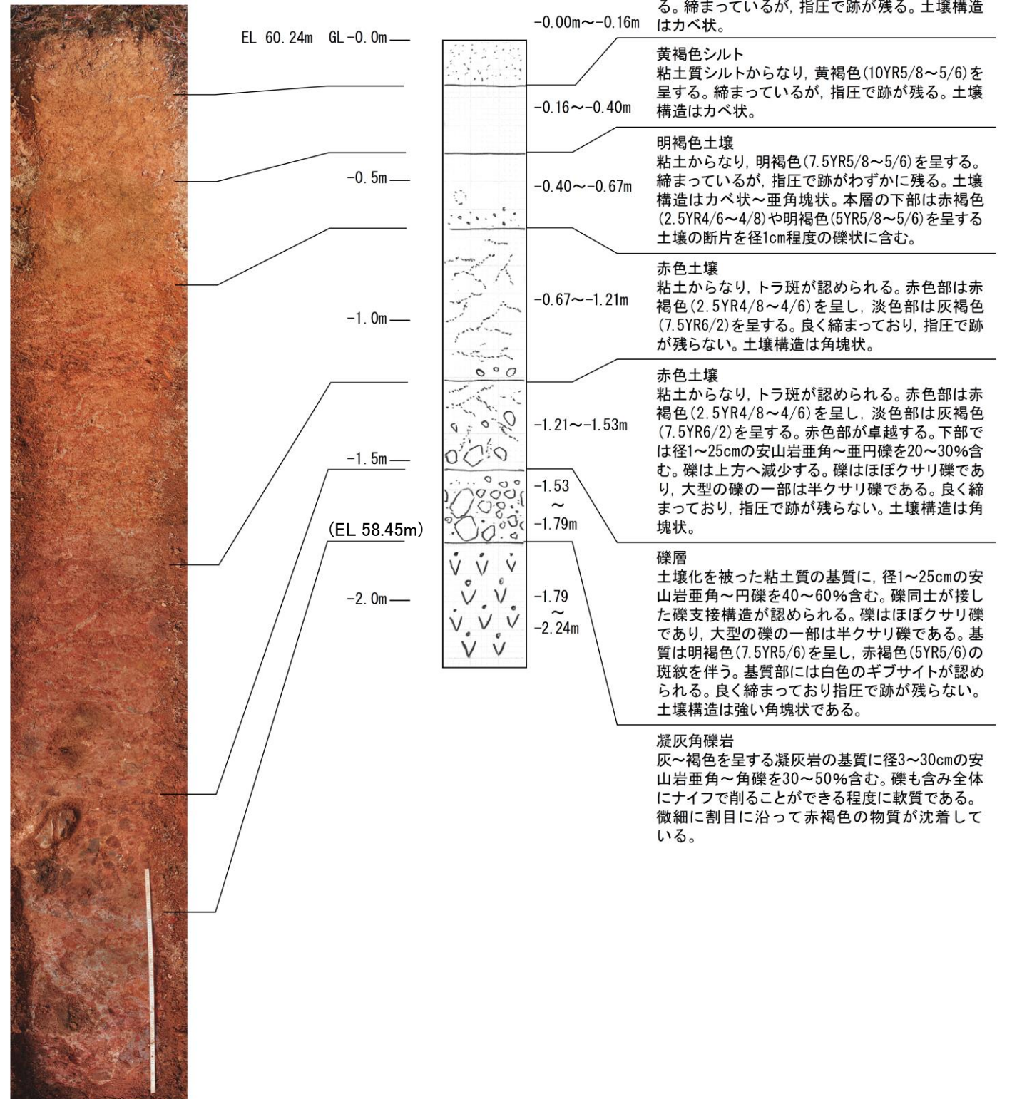
露頭写真
