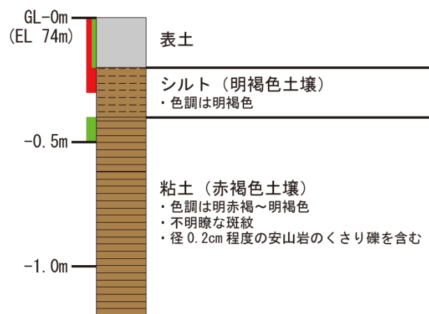
柱状図
