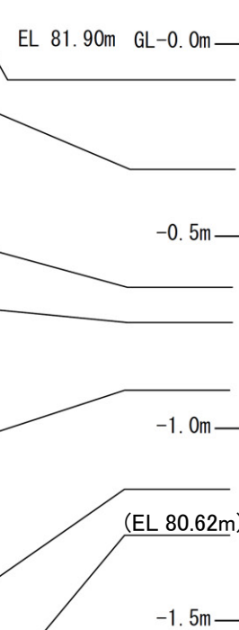
<柱状図>
