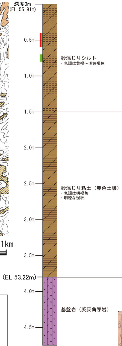
柱状図
