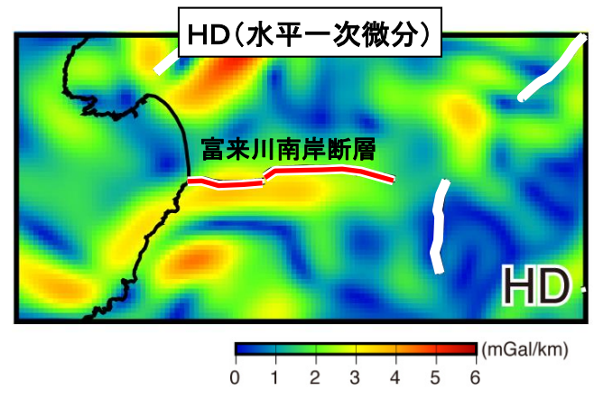
重力勾配テンソルを用いた解析結果(Hiramatsu et al.(2019)に一部加筆)
