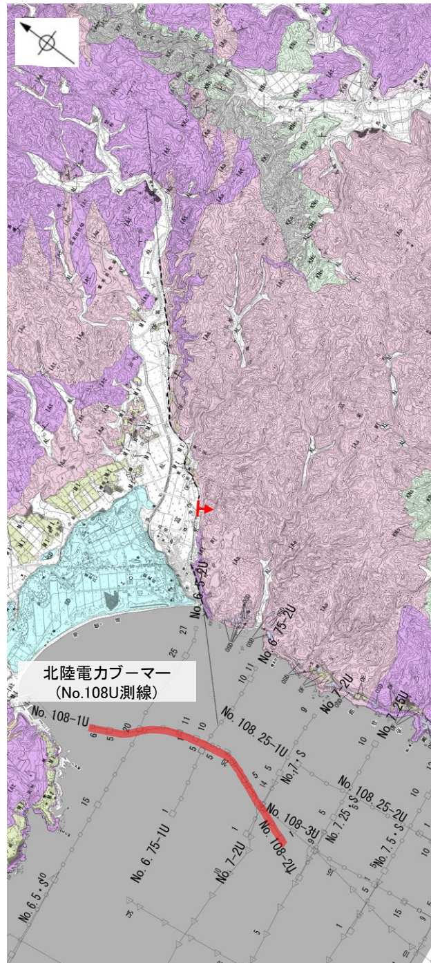
地質図
