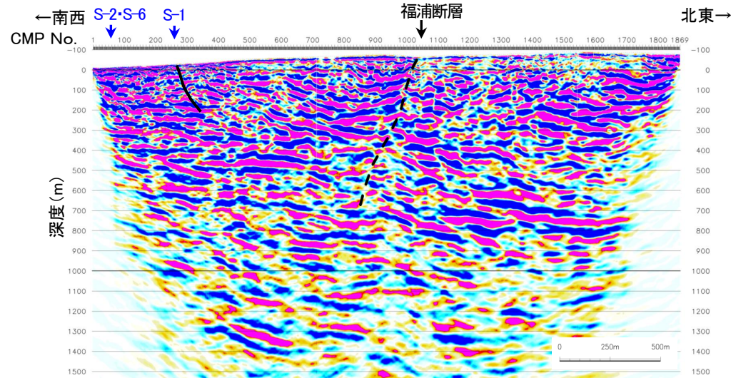
福浦断層を推定した各測線の深度断面
