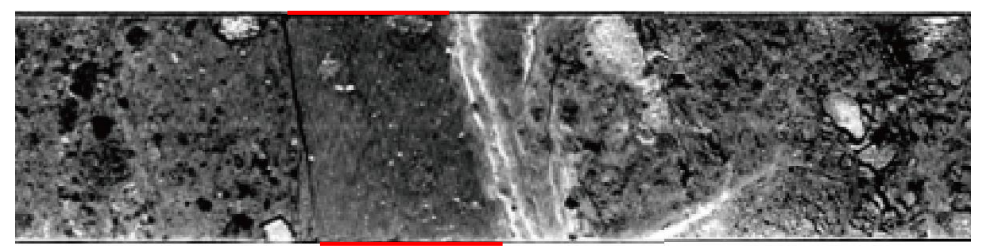
拡大図(上:コア写真, 下:CT画像)
