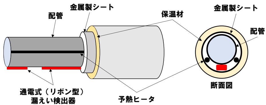
第 2. 2. 3 図 通電式(リボン型)のナトリウム漏えい検出器の設置の概念図
