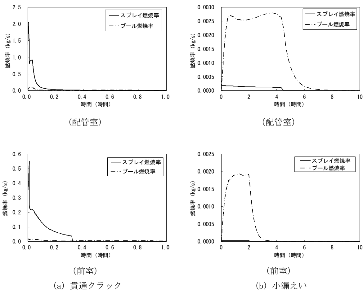
第 1 図 スプレイ及びプール燃焼率の時刻歴変化
