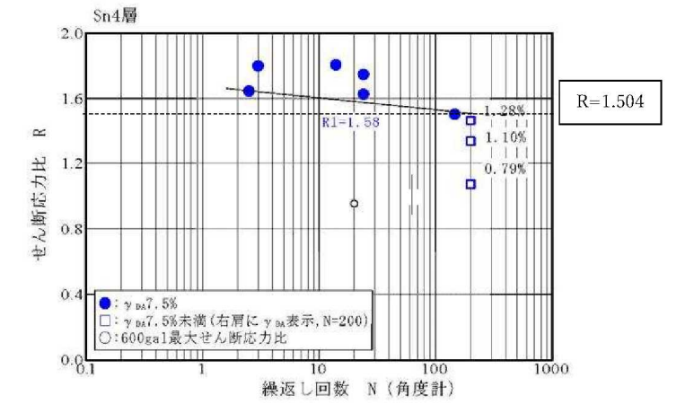
図7 中空円筒供試体による繰返しねじりせん断試験結果 (砂子又層上部軽石混じり砂岩 (Sn 4 ))
