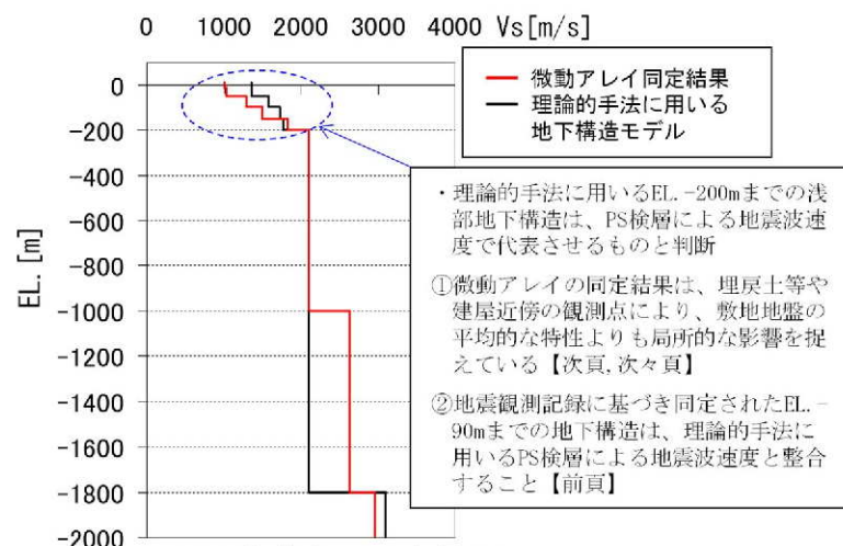
せん断波速度の同定結果
