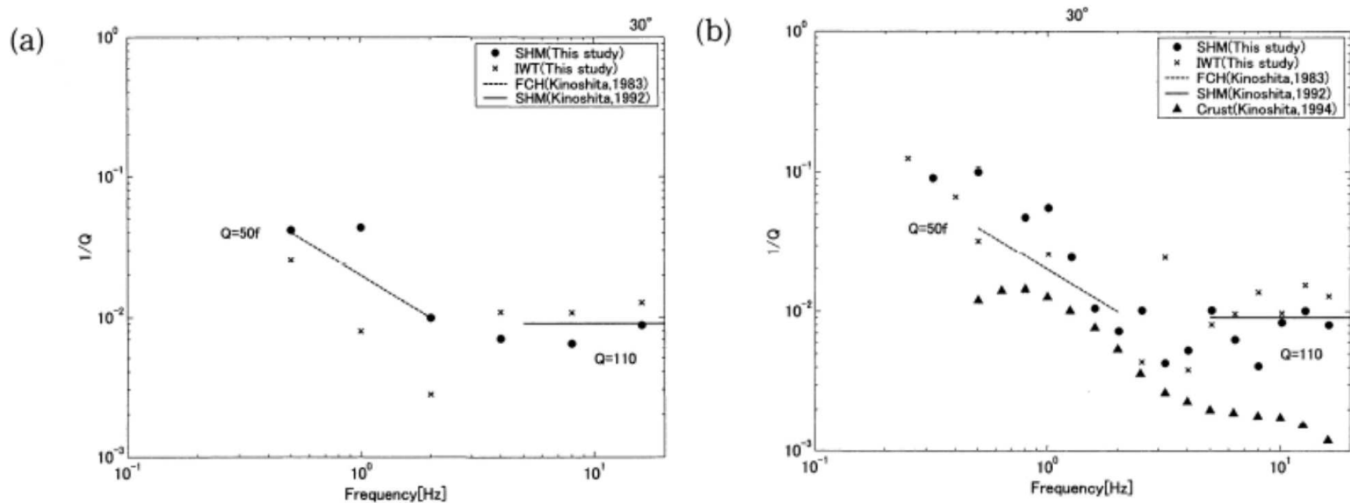
(a) フーリエ振幅スペクトルをオクターブ帯域幅で平滑化した場合
