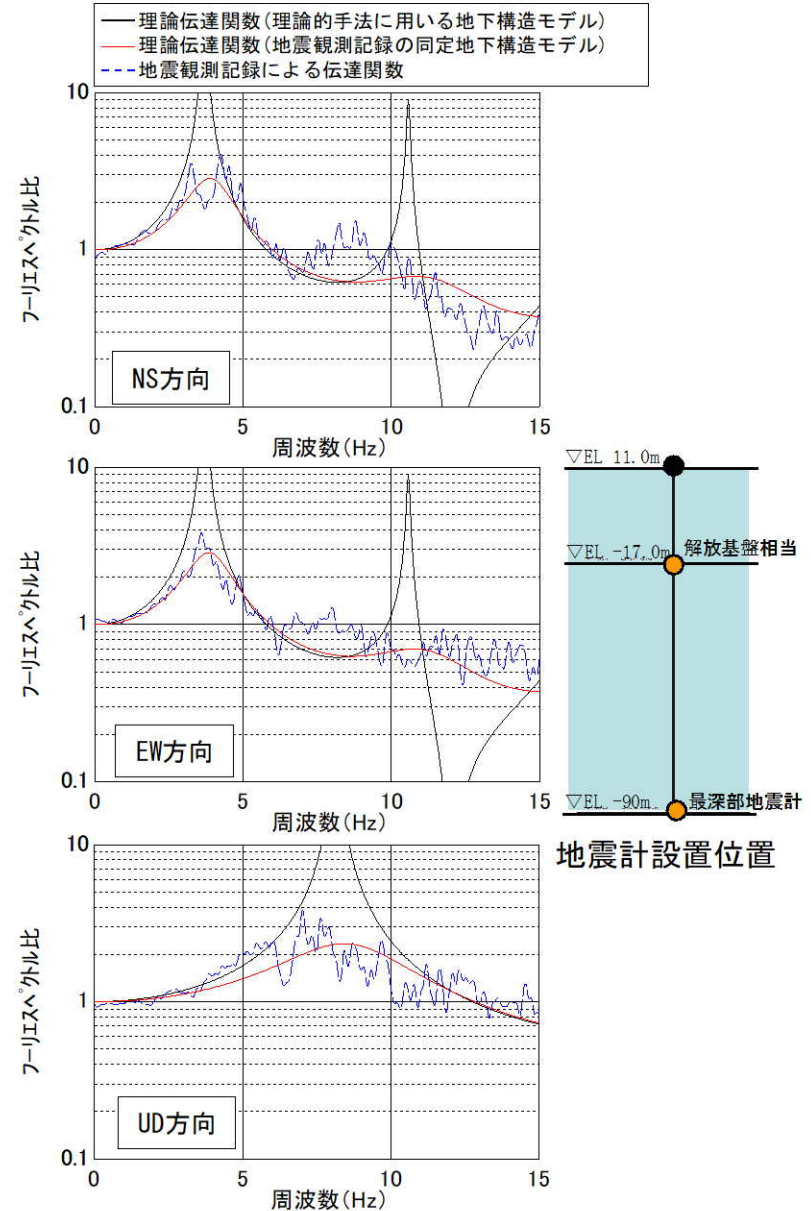
伝達関数(EL. -17m/EL. -90m)の比較
