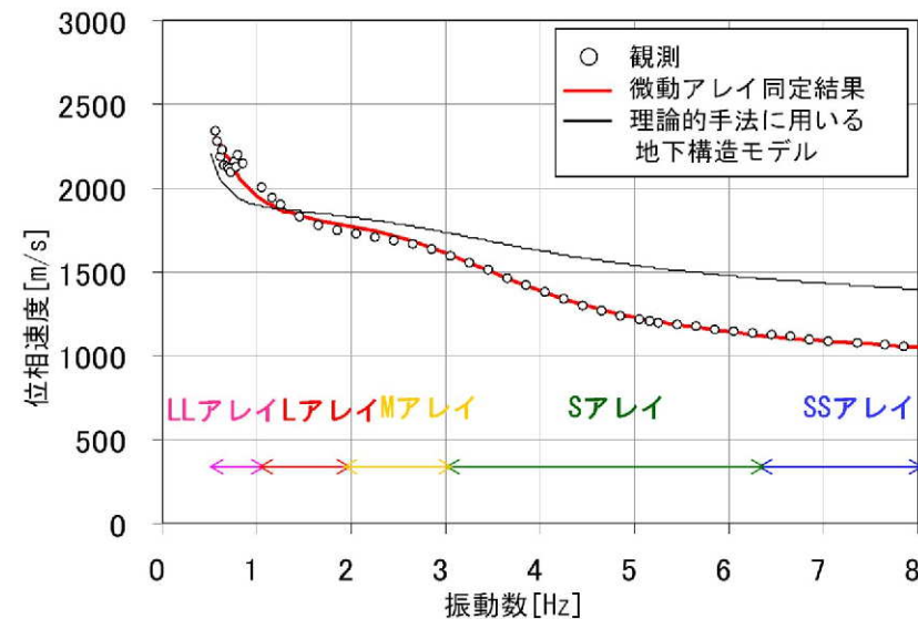
観測分散曲線と理論分散曲線
