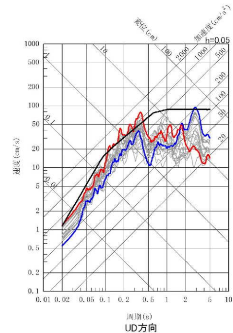
竹木場断層
