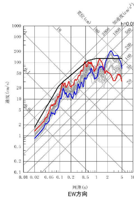
城山南断層
