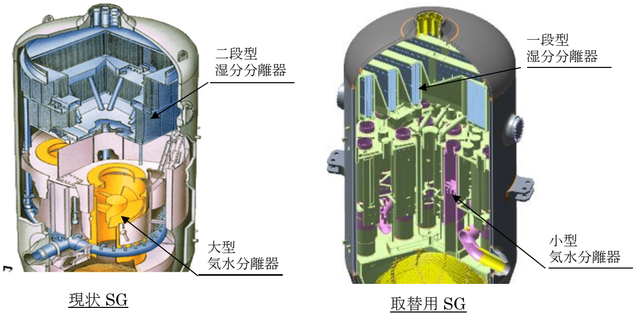
(b) 気水分離器及び湿水分離器
