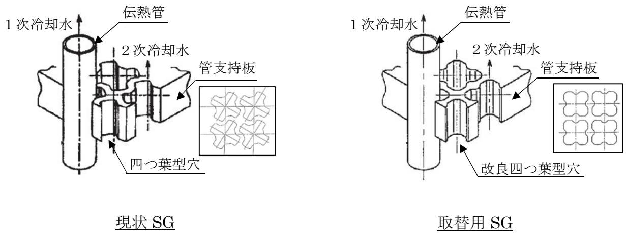
(b) 管支持板管穴形状の改良
