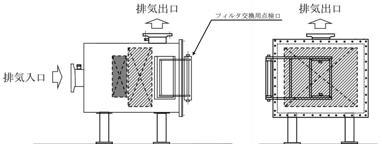
焼却・溶融設備の排気フィルタユニットの構造
