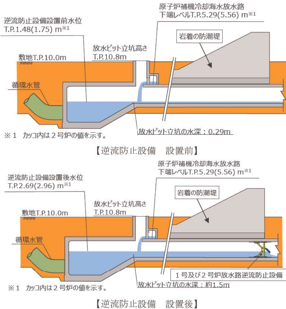
図 11 逆流防止設備設置前後の放水ピット水位
