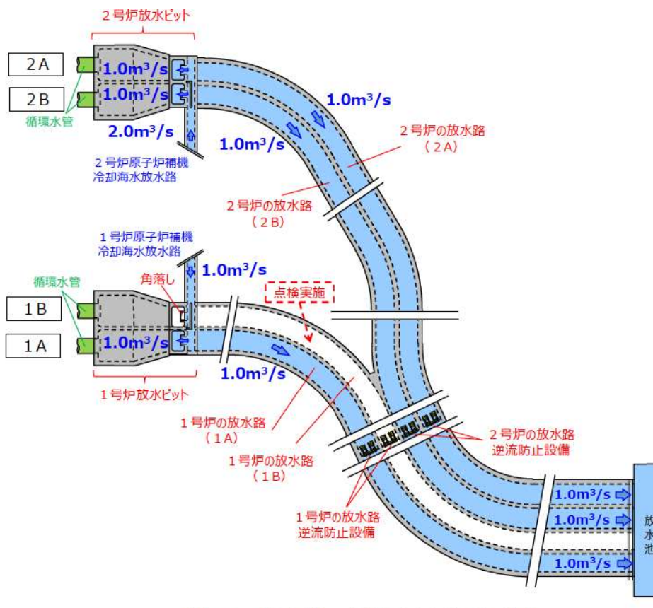
図10 放水路の流量を示す平面図 (プラント状態：外部電源喪失時，放水路の状態：片トレン通水時)
