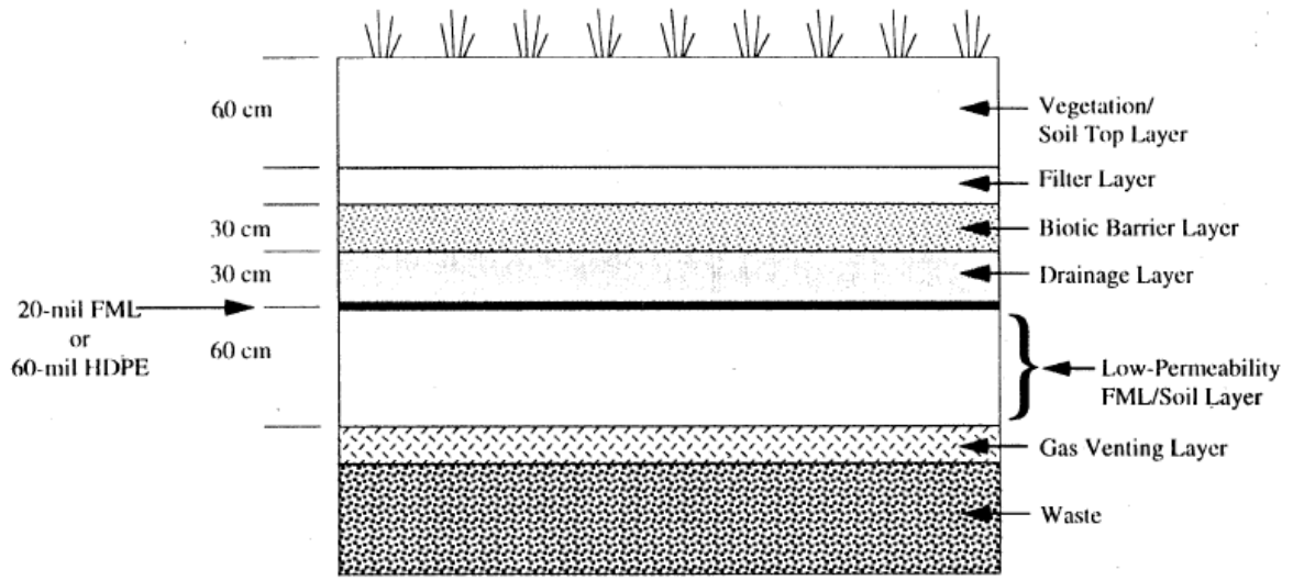
第 1 図 E P A における代替最終覆土設計の追加要素の例
