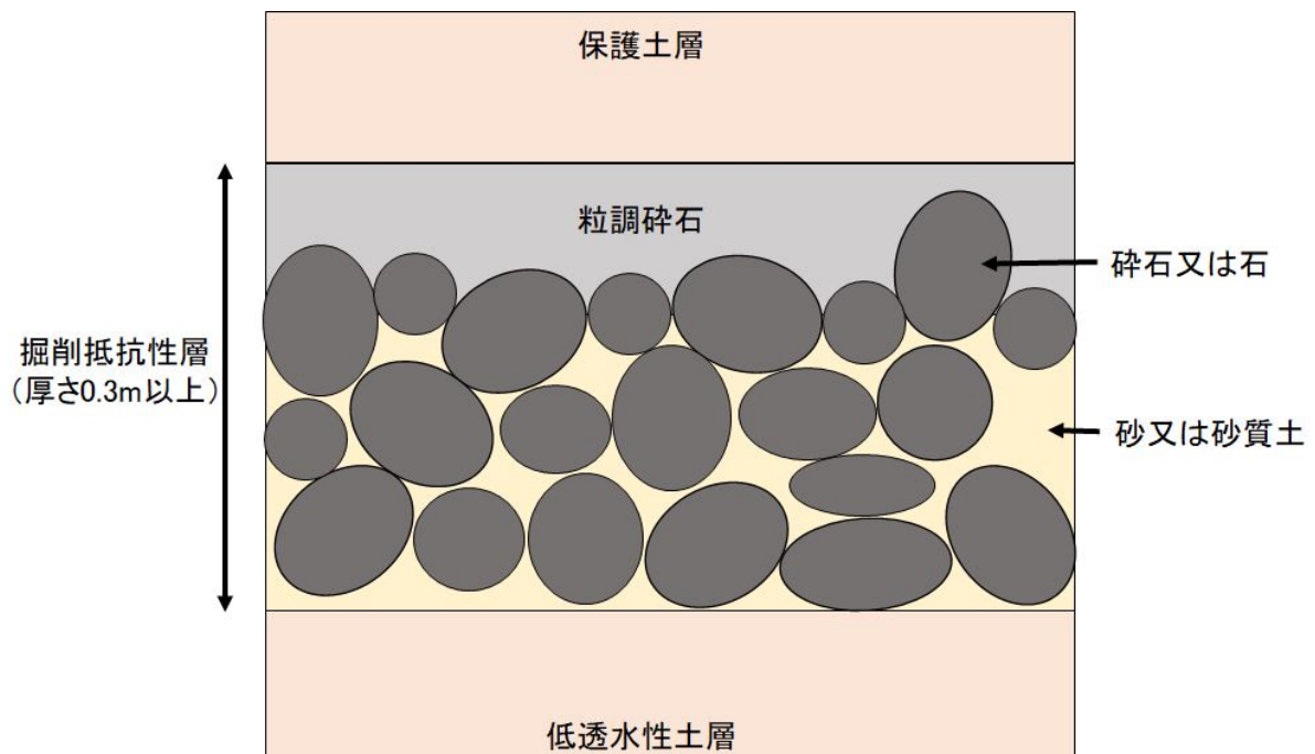
第 1 図 掘削抵抗性層の構造
