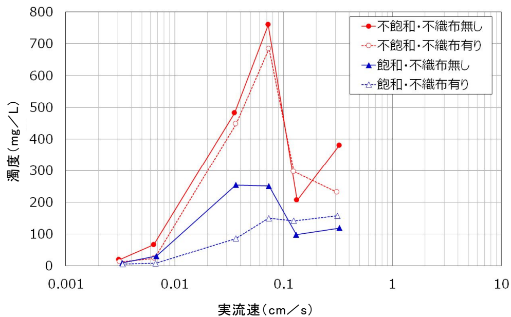
第 3 図 流出試験の結果 (濁度と実流速の関係)
