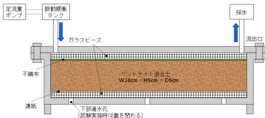
第7図 流出試験装置の概略図
