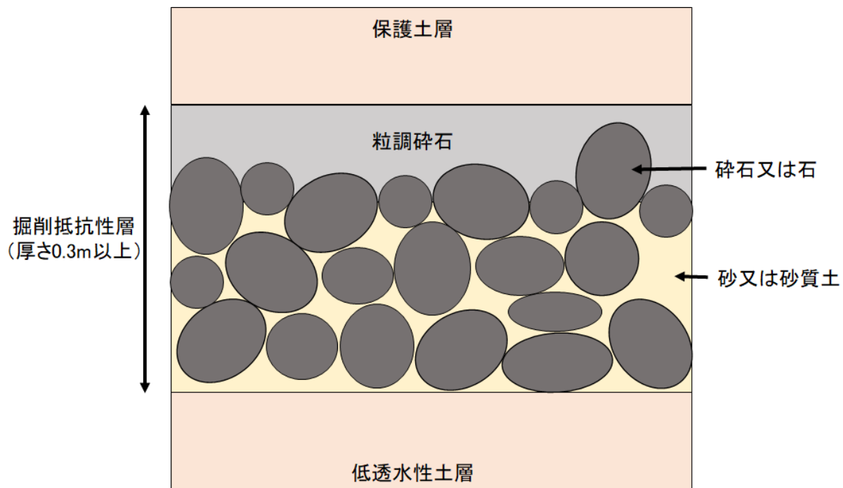
第6図 掘削抵抗性層の構造
