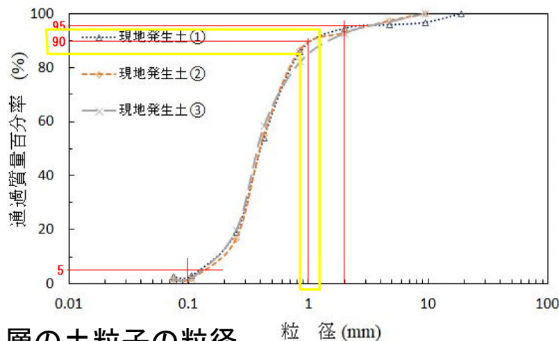
第5図 保護土層の土粒子の粒径
