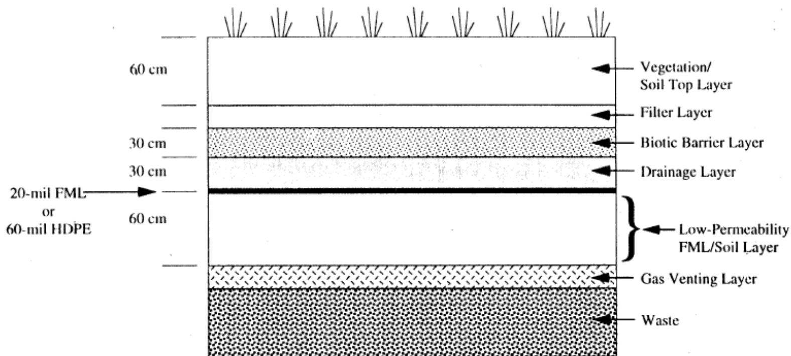
参図1 EPAにおける代替最終覆土設計の追加要素の例
