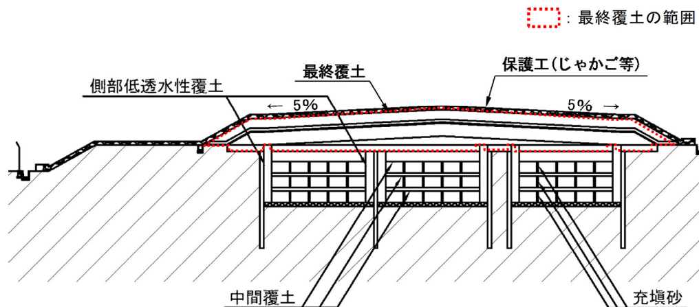
第1図 覆土の断面図(西側)
