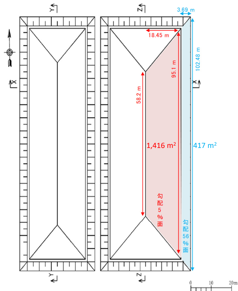
第4図 廃棄物埋設地 平面図
