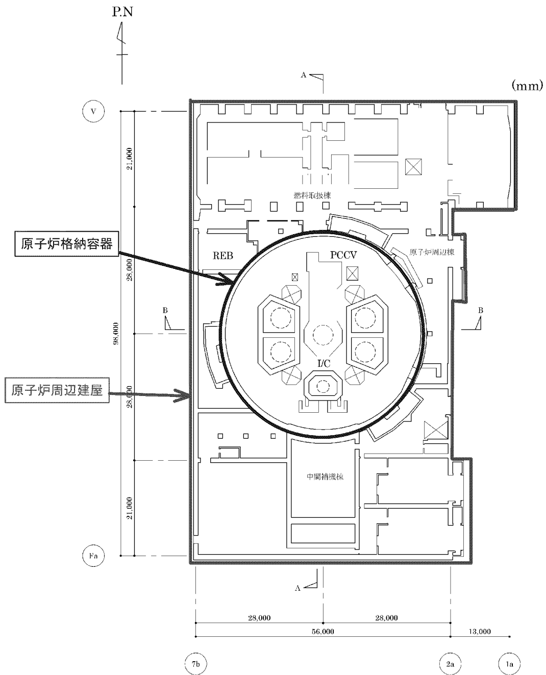
第2-2図 原子炉格納容器及び原子炉周辺建屋の概略平面図(EL.11.30m)
