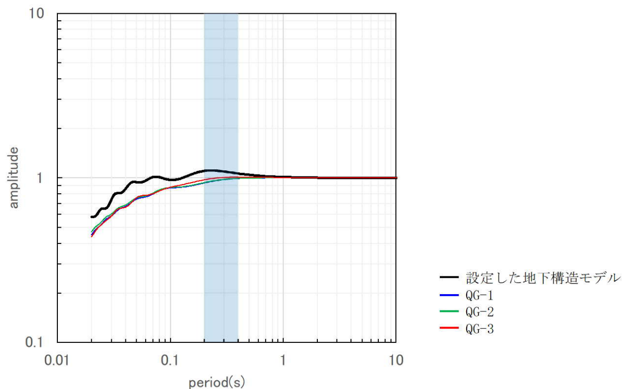
伝達関数の比較（EL. -15m/EL. -200m、上下方向）
