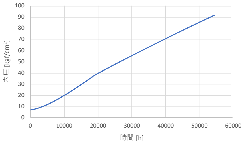
第 2.3 図 被覆管内圧の計算結果
