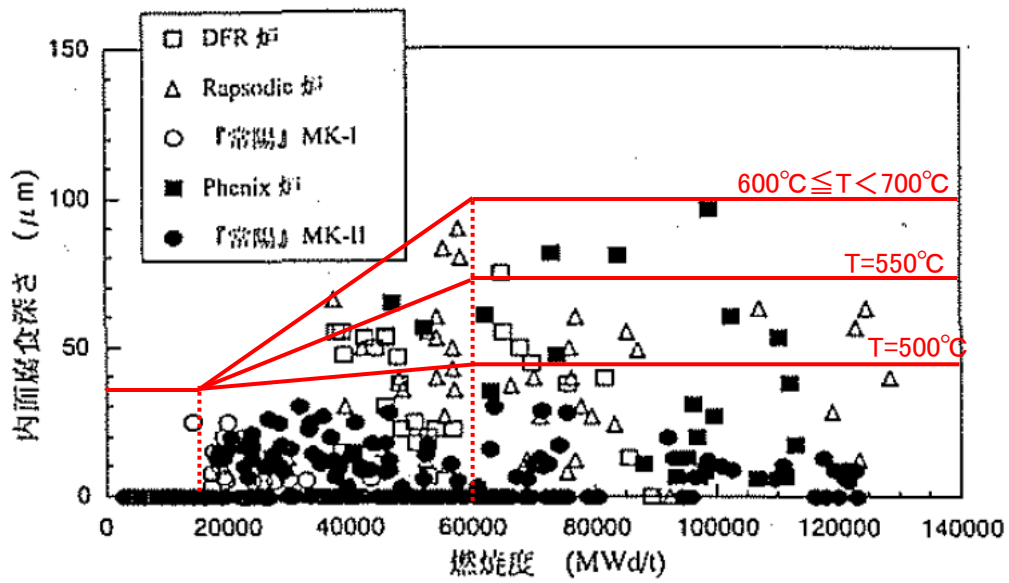
第1図 SUS316 相当ステンレス鋼の被覆管内面腐食と照射試験データの関係
