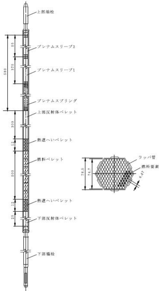
第 4.1.1 図 炉心燃料要素
