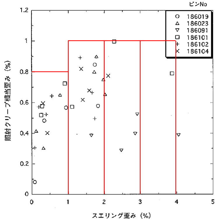
第4図 MFA-1 (SUS316 相当ステンレス鋼) におけるスエリングと照射クリープ歪の関係
