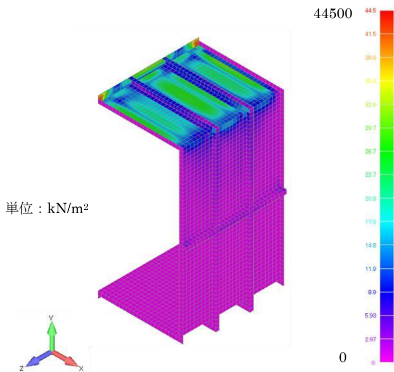
第3図 屋外ダクト水平部の \sigma ミーゼス応力コンター
