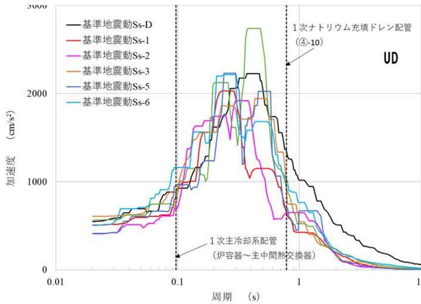
第1図 地盤物性のばらつき及び建物剛性の変動に係る影響確認 (設計成立性確認) に使用する基準地震動
