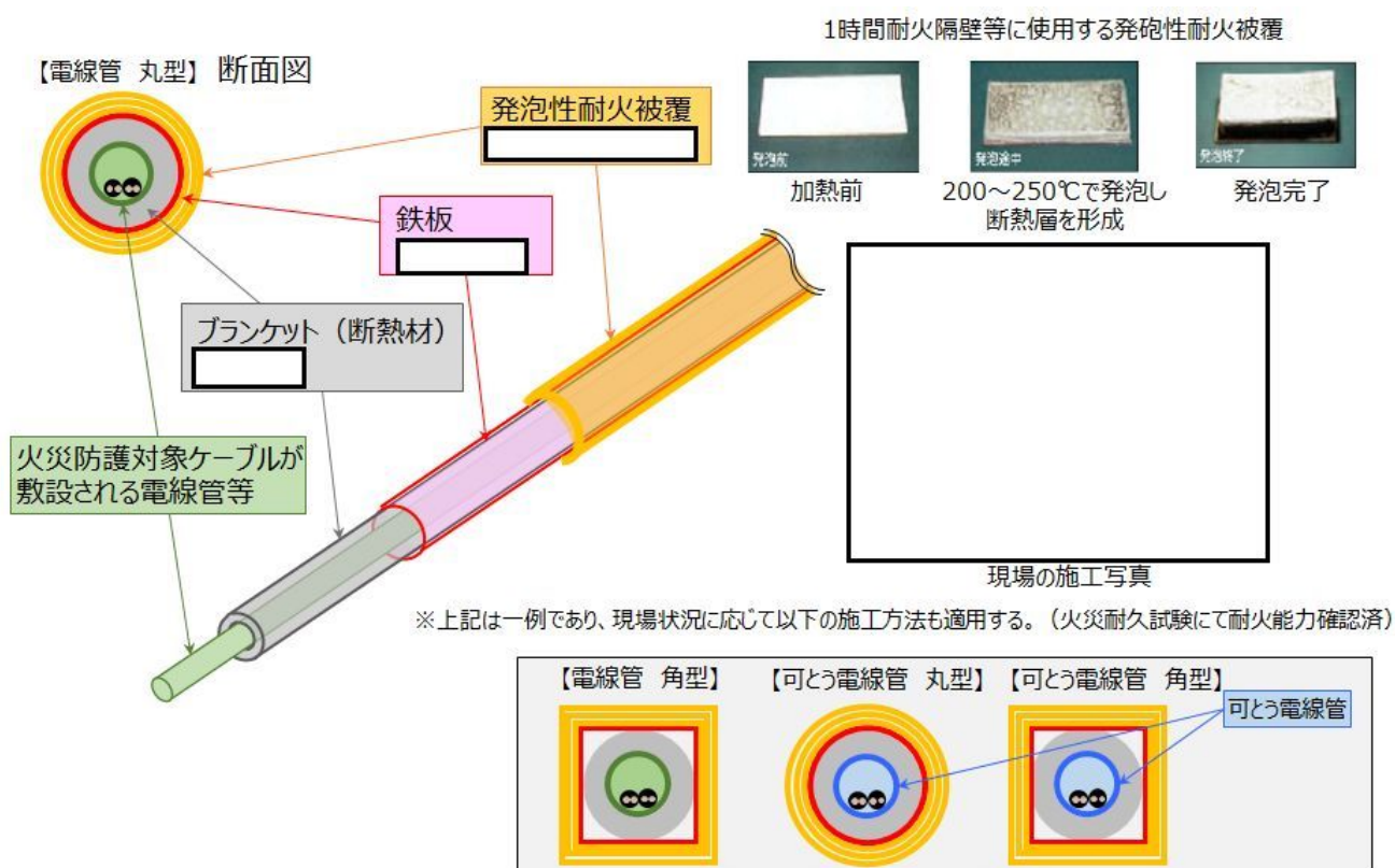
第1-1-9図 電線管ラッピングの施工方法
