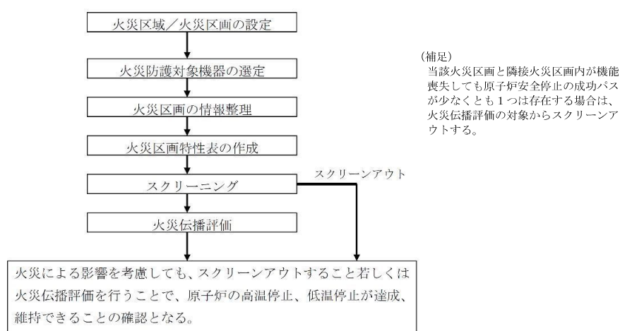
第 1-5-1 図 火災影響評価のフロー（設置許可まとめ資料より）
