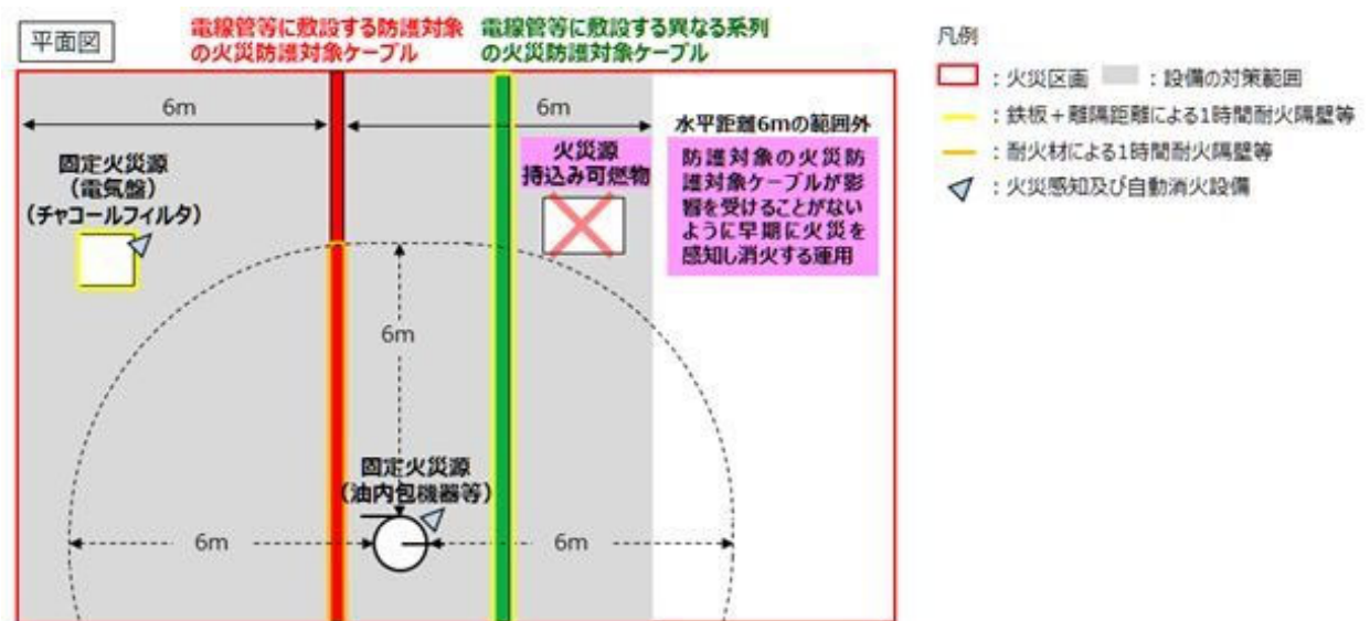
第 1-1-5 図 隔壁等の設置に係る基本設計方針の概念図
