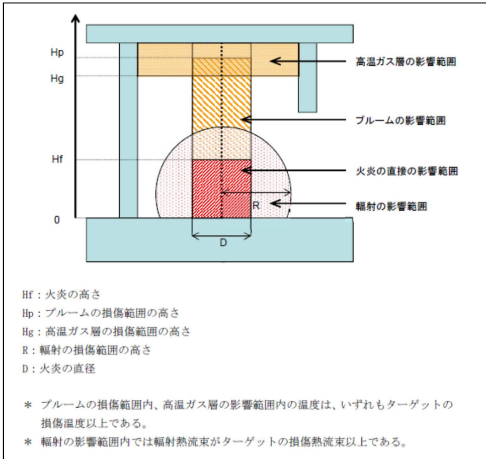
第 1-7-1 図 火災影響範囲 (ZOI) の評価モデル (FDT s 計算モデルによる影響範囲の概念図) (「原子力発電所の内部火災影響評価ガイド」より抜粋)
