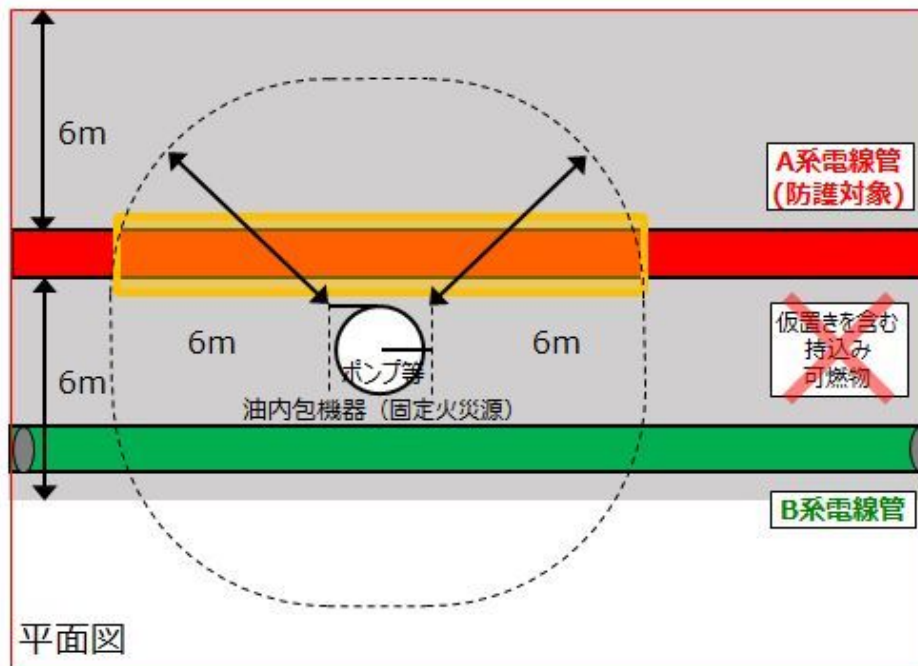
第 1-1-7 図 固定火災源が油内包機器の場合の電線管等への隔壁等の設置イメージ
