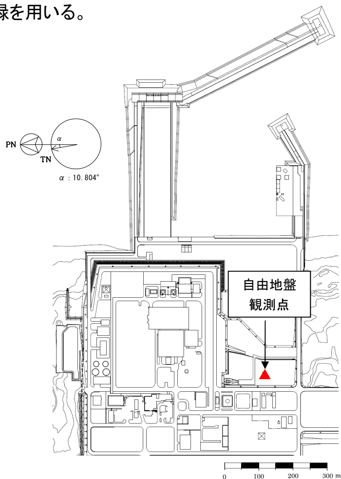
平面配置図
