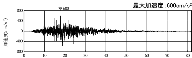
時間(秒) 加速度波形(水平)
