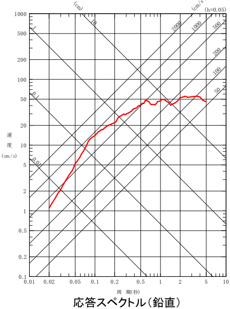
— :解放基盤表面位置に引き上げた地震動(鉛直)
