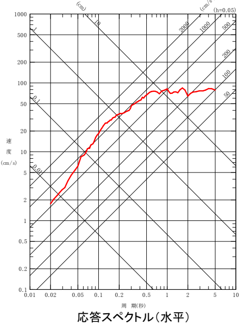
— :解放基盤表面位置に引き上げた地震動(水平)
