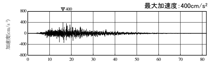
時間(秒) 加速度波形(鉛直)
