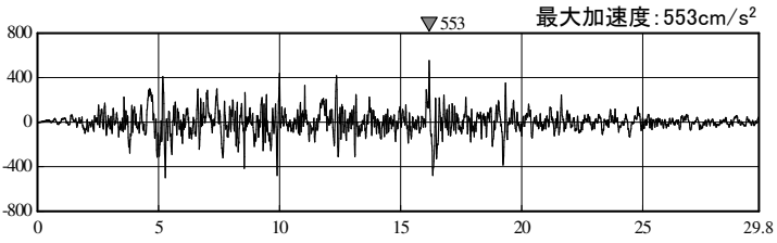
時間(秒) 加速度波形(水平) 水平方向
