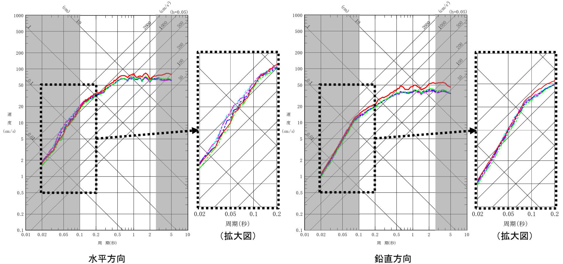
図1 各入力位置による解放基盤表面における地震動(応答スペクトル) ※4
