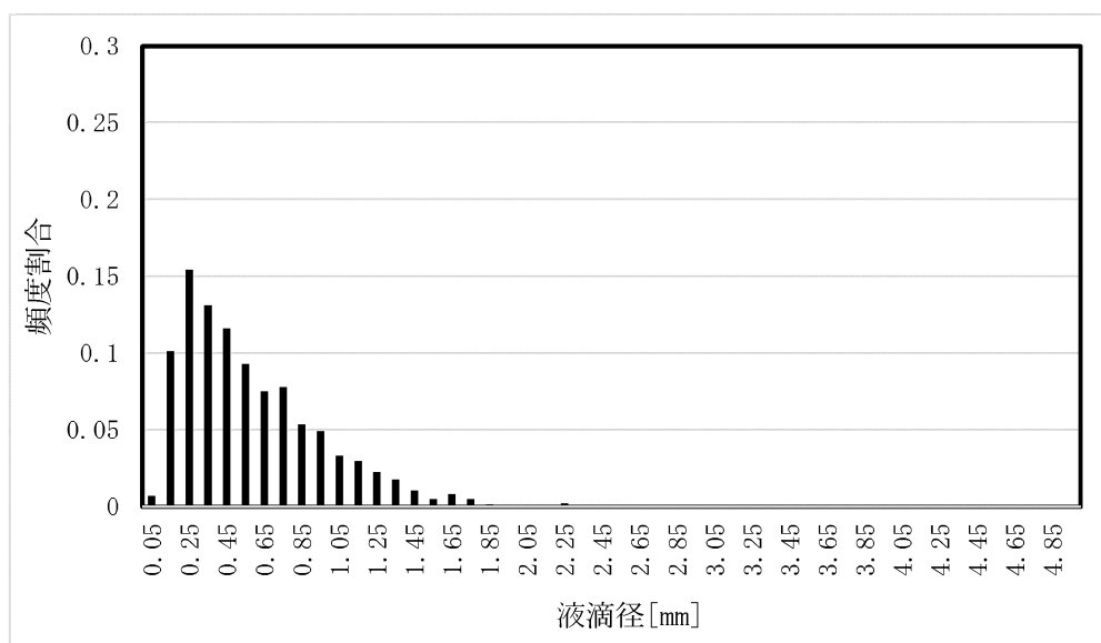
測定点①
