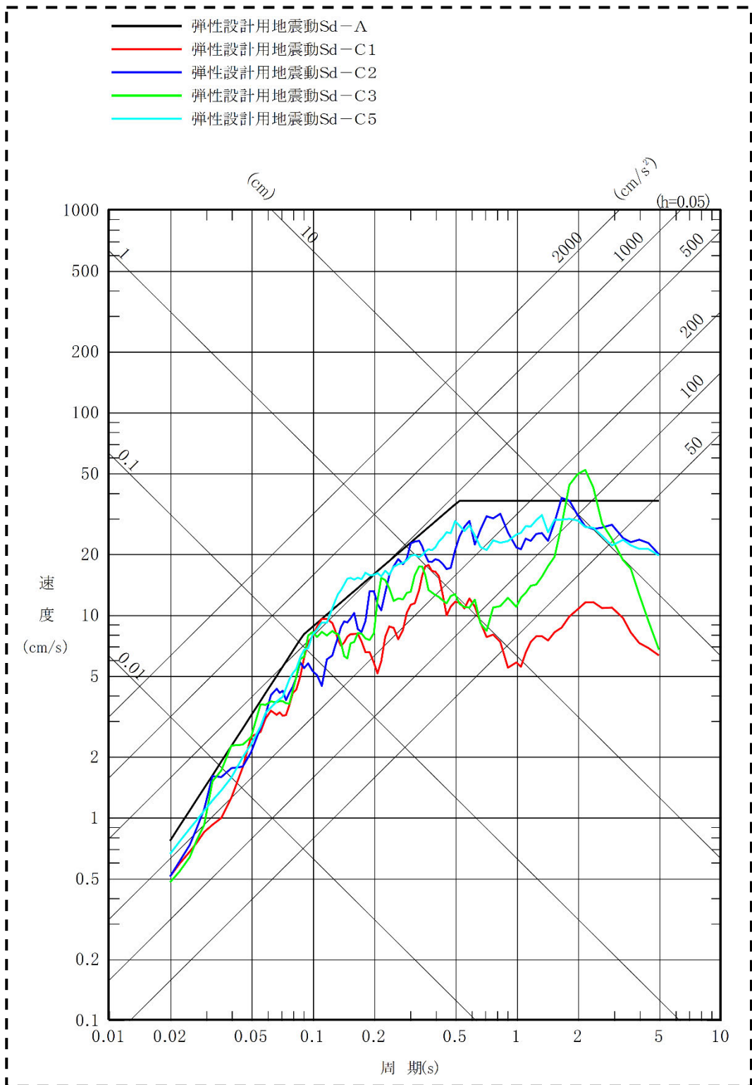
第 1.5-1 図 (5) 弾性設計用地震動の応答スペクトル (鉛直方向) 注 2
