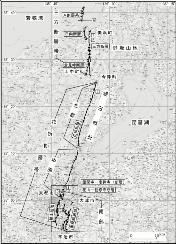
図 2 - 1 三方・花折断層帯の活断層位置と主な調査地点 1: 久々子地点 2: 気山地点 3: 途中谷地点 4: 修学院地点 5: 今出川地点 A: 文献6 B: 文献7 C: 文献4 活断層の位置は文献2及び10に基づく ●: 断層帯の北端と南端 中: 花折断層帯の北部・中部・南部の境界 図は国土地理院発行数値地図200000「岐阜」、「名古屋」、「宮津」及び「京都及大阪」を使用。 (長方形は図2-2の範囲)
