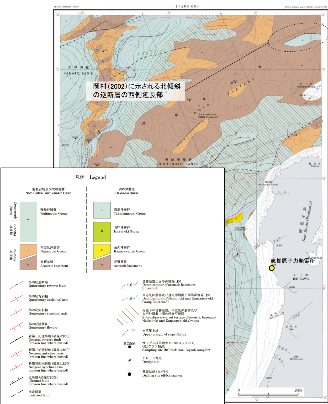
能登半島西方海底地質図 (岡村(2007)に一部加筆)
