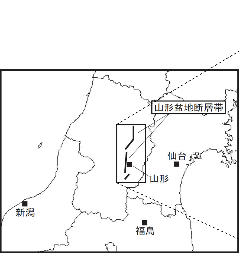
図1-1 山形盆地断層帯の概略位置図 (長方形は図2の範囲)
