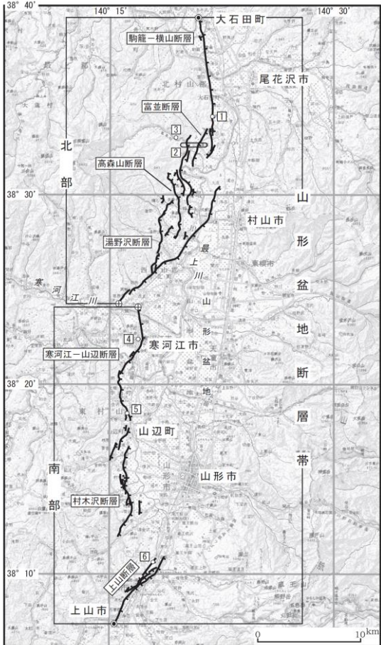
図2 山形盆地断層帯の位置と主な調査地点 1：横山地点 2：富並地点 3：山の内地点 4：高森山地点 5：大寺地点 6：上山地点 ●：断層帯の北端と南端 ○：断層帯の北端・南端の北端・南端の北端 断層の位置は文献3、6、7及び151に基づく 基図は国土院発行数値地図200000「仙台」を使用。
