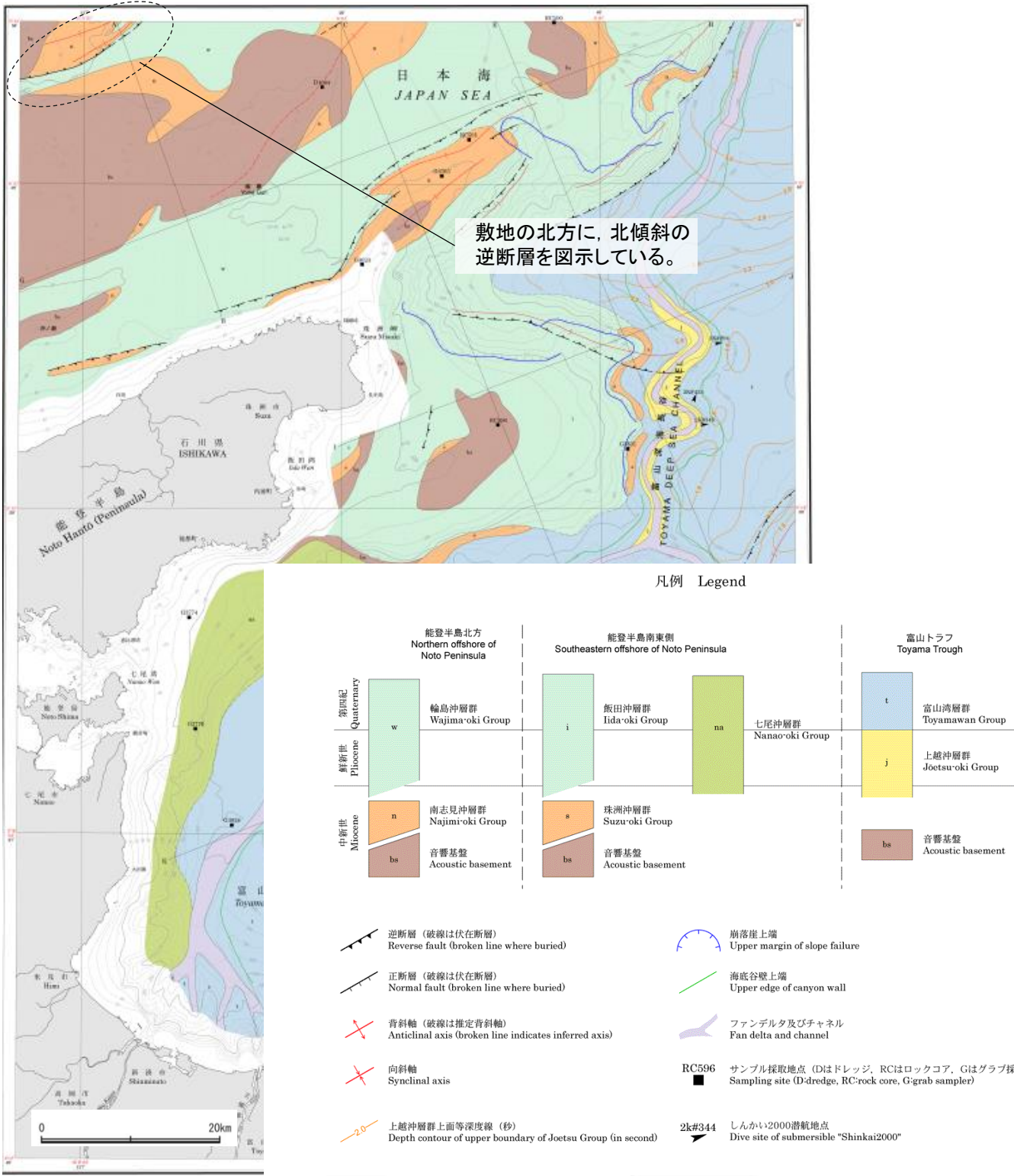
能登半島東方海底地質図 (岡村(2002)に一部加筆)
