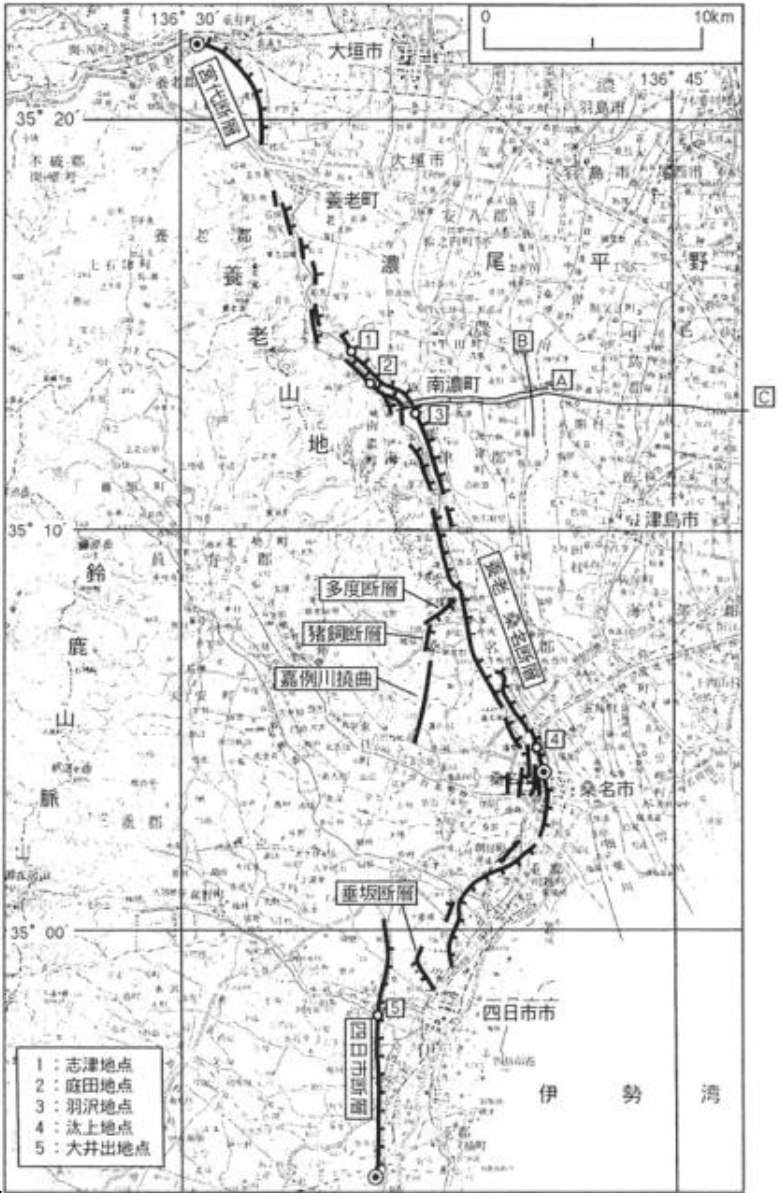
図2 養老－桑名－四日市断層帯の活断層位置と調査地点 活断層の位置は岡田・東郷編(2000)に基づく。 1－5: 主な調査地点。細線は反射法弾性波探査測線。A: 東西測線。 B: 南北測線。C: 濃尾平野中部測線。 ●: 断層帯の北端、南端及び屈曲点。 基図は国土地理院発行1:200,000地勢図「名古屋」及び「岐阜」を使用。
