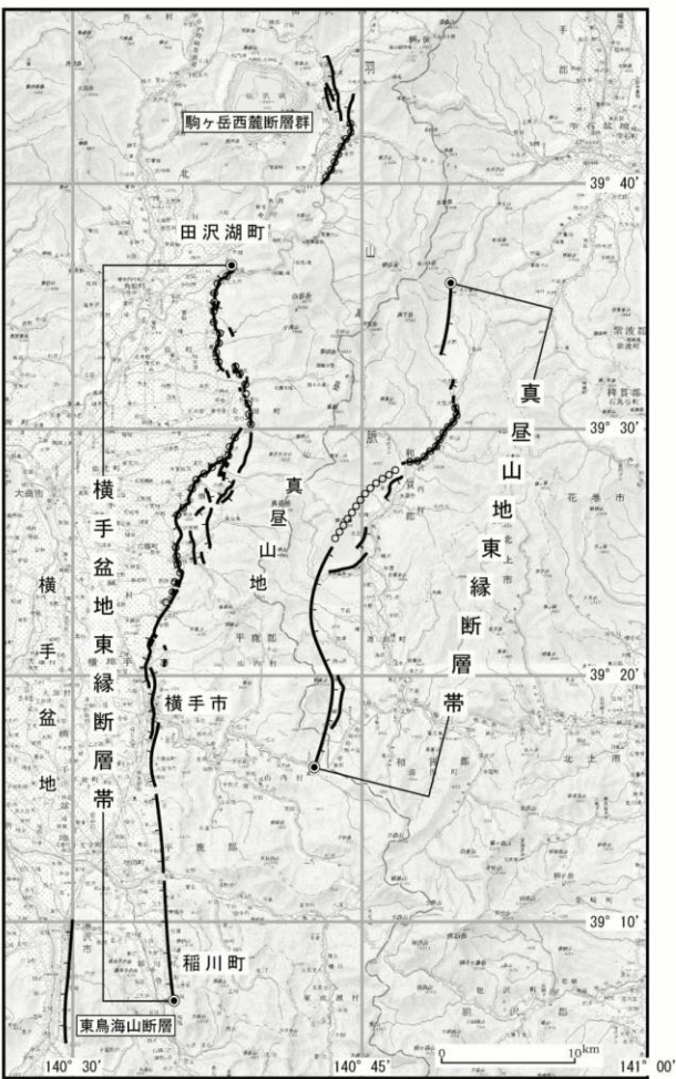
横手盆地東縁断層帯の評価において考慮した断層 (地震調査委員会, 2005a)
