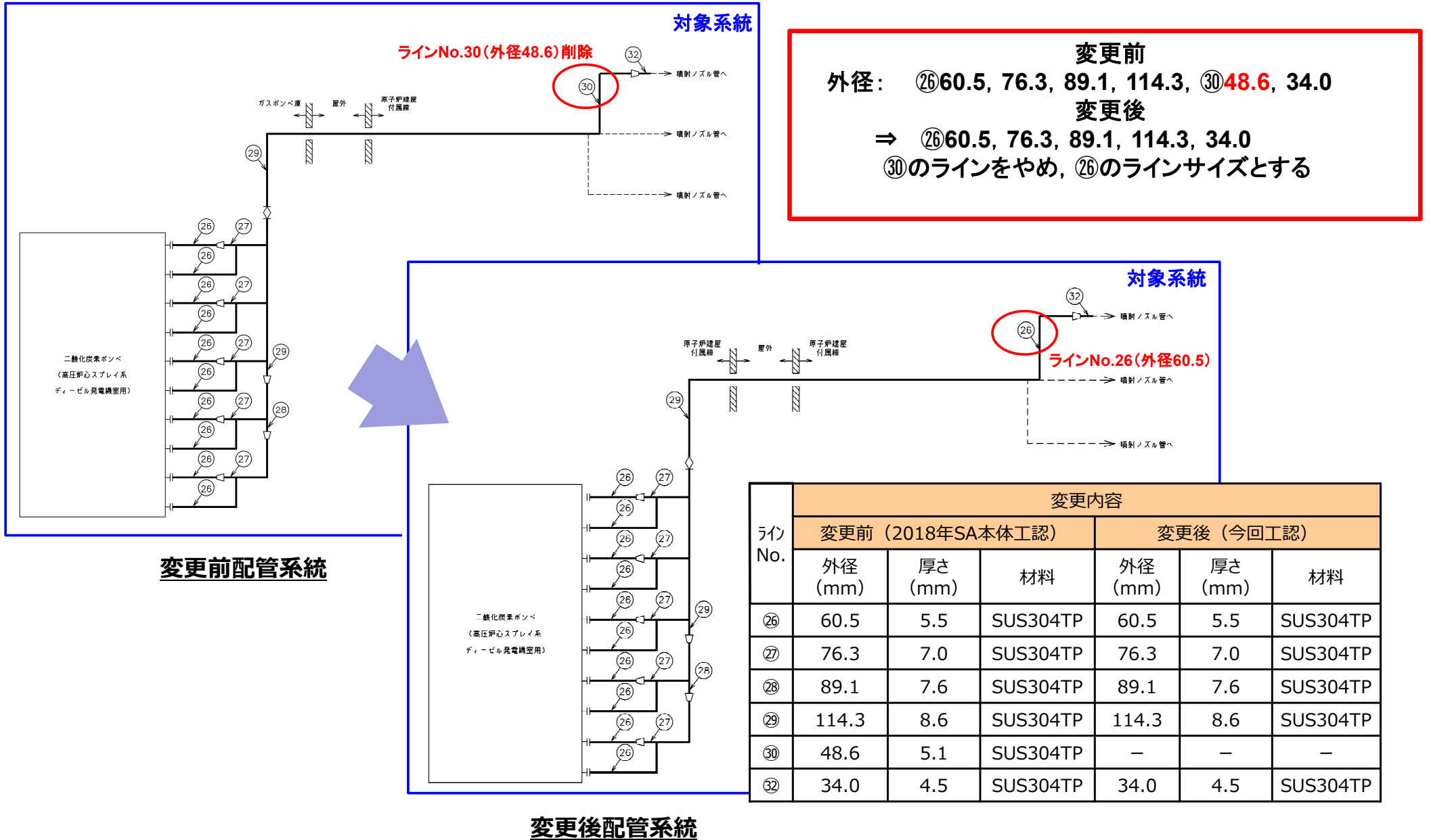
図7 高圧炉心スプレィ系ディーゼル発電機室用配管系統の変更前後
