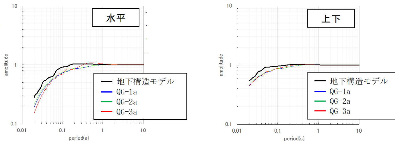
ボーリング孔内減衰測定結果と地下構造モデルの伝達関数による比較結果
