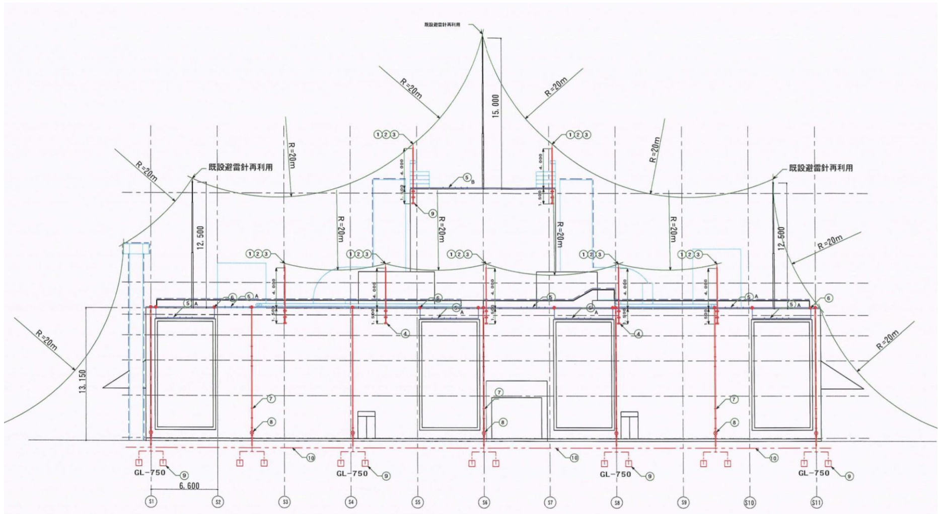
第 1 図 避雷設備の設置イメージ (2/2)
