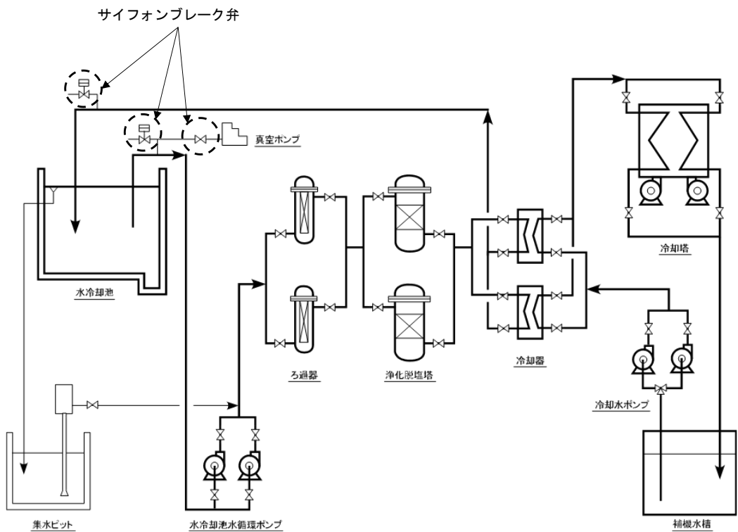
第 2.1 図 使用済燃料貯蔵設備の概要（第二使用済燃料貯蔵建物）
