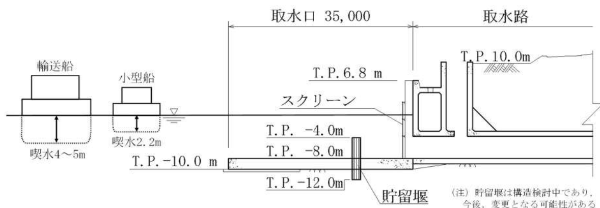
断面図 (断面 A-A')
