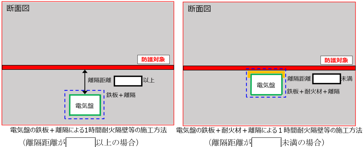
第 1-1-11 図 電気盤に隔壁等を設置する場合の施工方法 (例)
