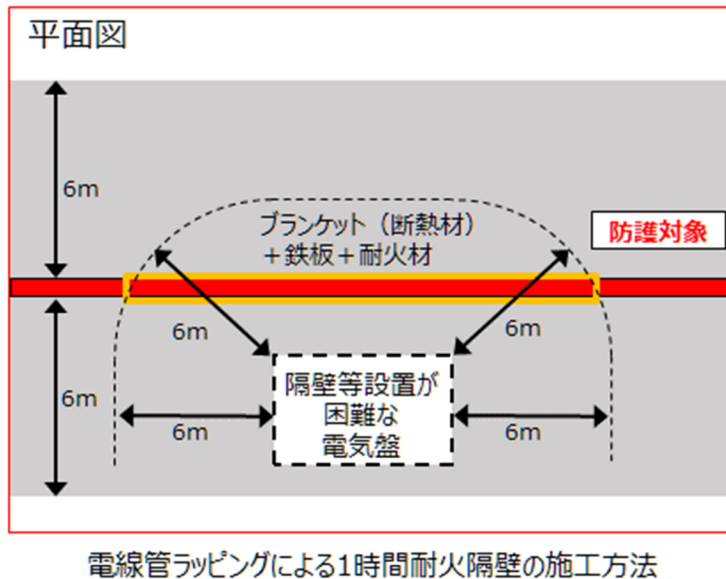
第 1-1-12 図 電気盤に隔壁等の設置が困難な場合の施工方法 (例)
