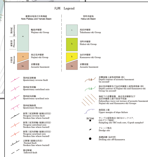
能登半島西方海底地質図 (岡村(2007)に一部加筆)
