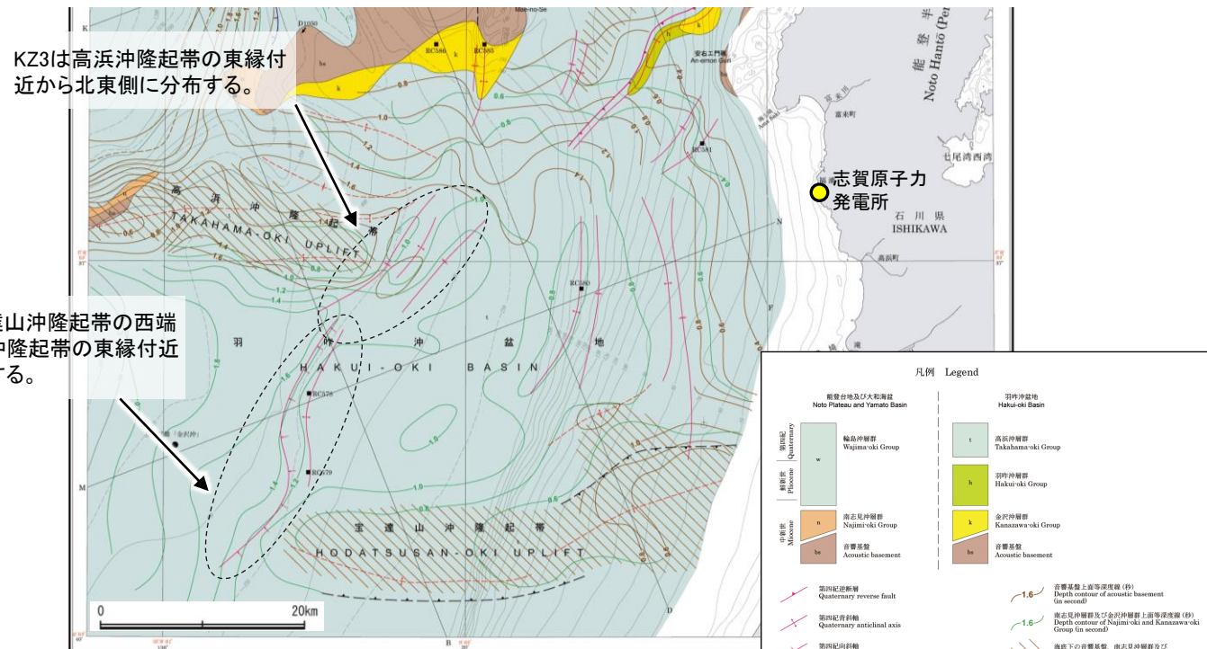
能登半島西方海底地質図 (岡村(2007)に一部加筆)
