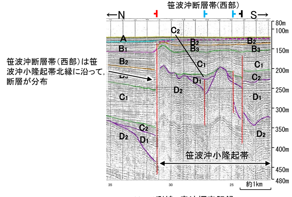
No.105-1測線 音波探査記録
