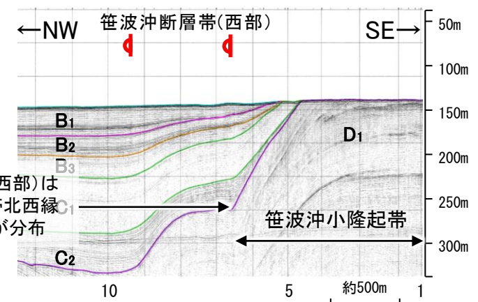
K16-2測線 音波探査記録
