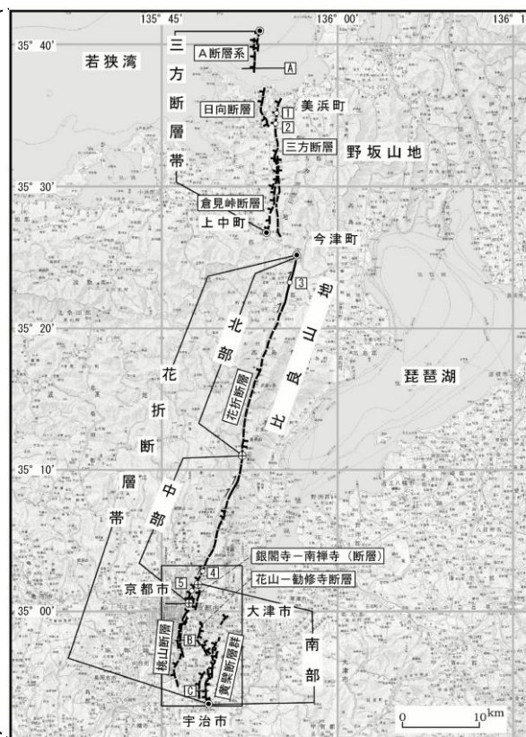
図2-1 三方・花折断層帯の活断層位置と主な調査地点 1: 久々子地点 2: 氣山地点 3: 途中谷地点 4: 修学院地点 5: 今出川地点 A: 文献6 B: 文献7 C: 文献4 活断層の位置は文献2及び10に基づく ●: 断層帯の北端と南端 中: 花折断層帯の北部・中部・南部の境界 基図は国土地理院発行数値地図200000「岐阜」、「名古屋」、「宮津」及び「京都及大阪」を使用。 (長方形は図2-2の範囲)
