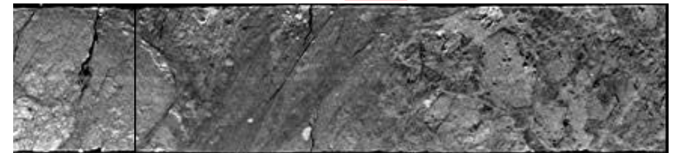
拡大図(上:コア写真, 下:CT画像)
