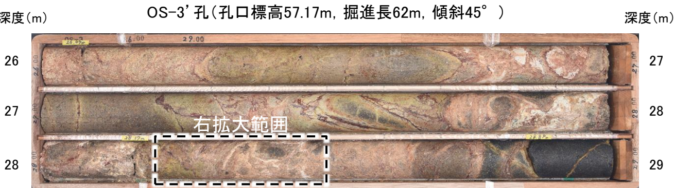
コア写真(26~29m)
