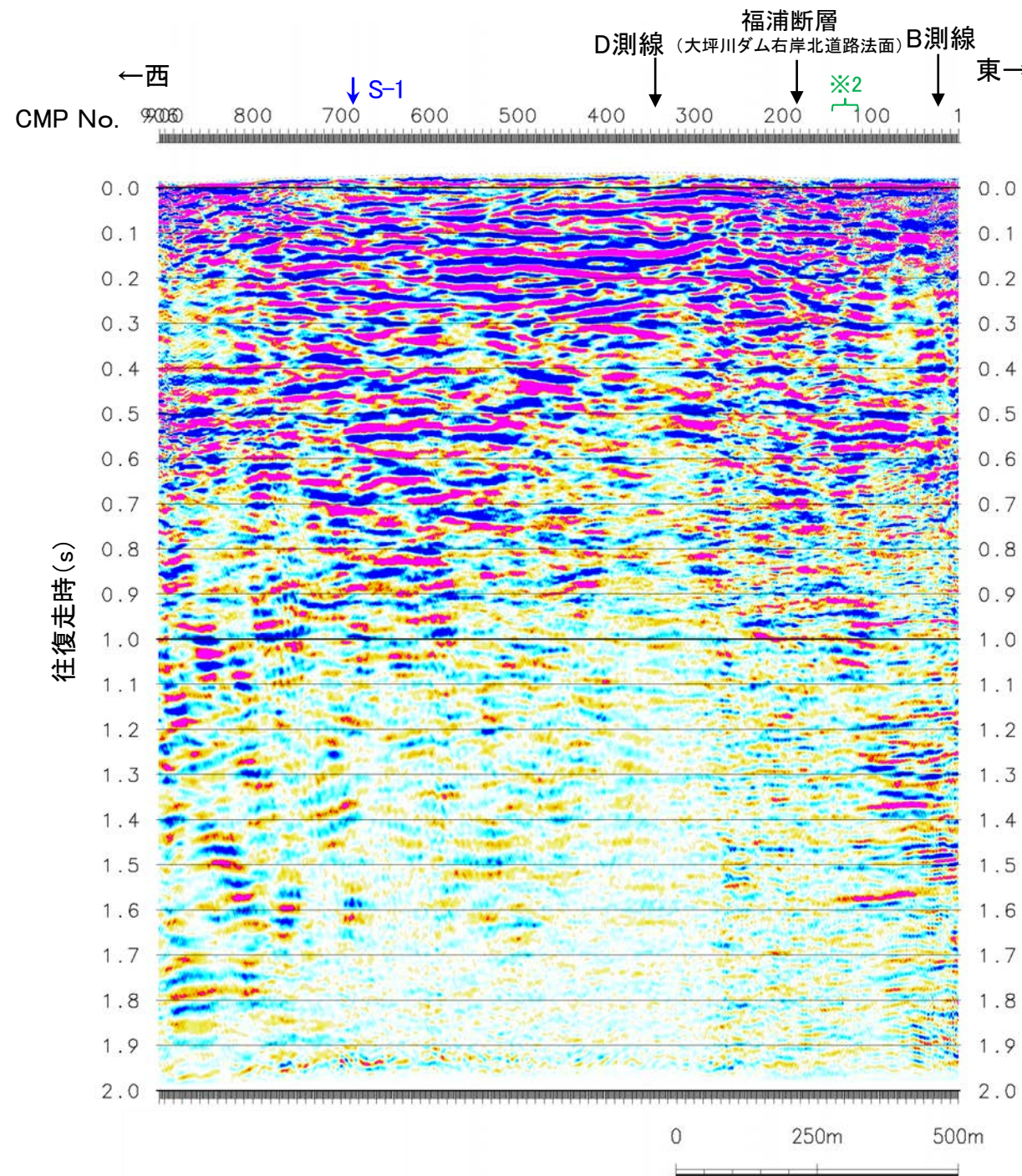
C測線
