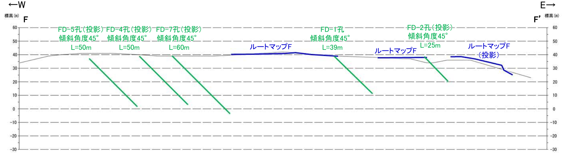
断面図(H:V=1:1)
