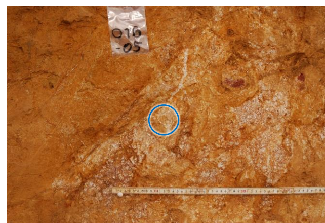
試料採取箇所写真(OTB-05)
