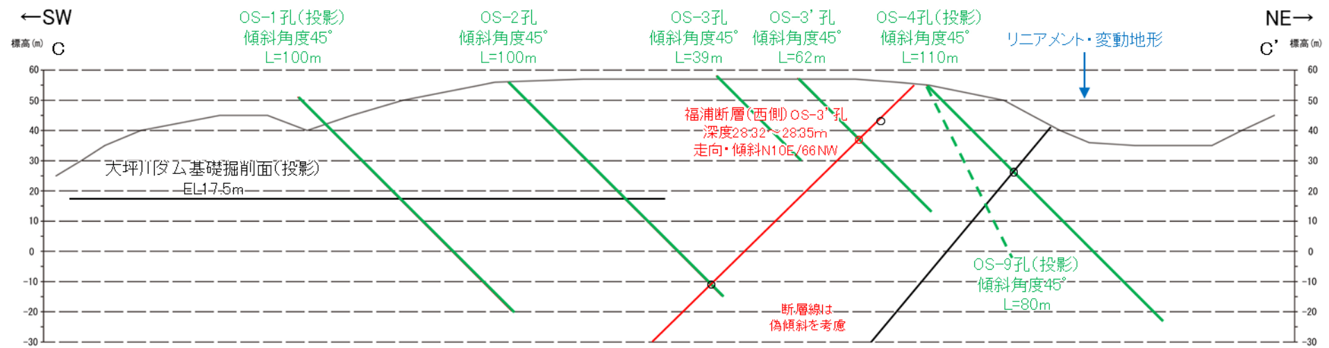
断面図(C-C' 断面) (H:V=1:1)
