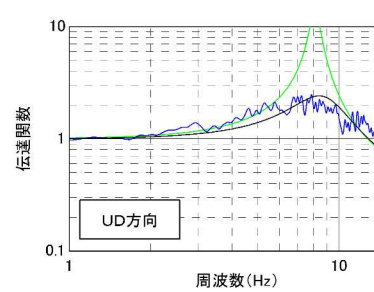
伝達関数の比較 (EL.-17.0m/EL.-90.0m)
