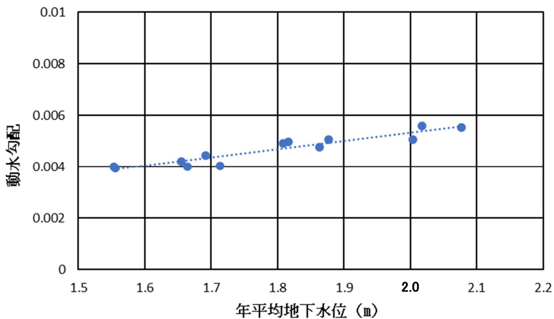
第 14 図 年平均地下水位と年間の動水勾配の相関
