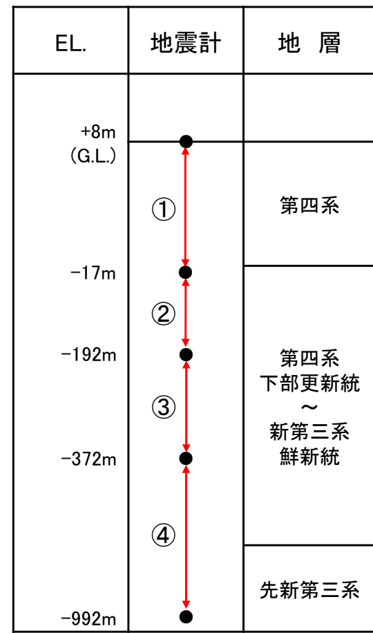
地震計の設置深さ
