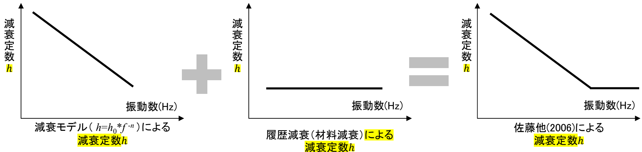
逆解析に用いる減衰モデル h のイメージ図
