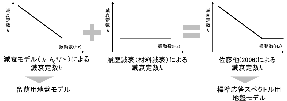
同定解析に用いる減衰モデル h のイメージ図
