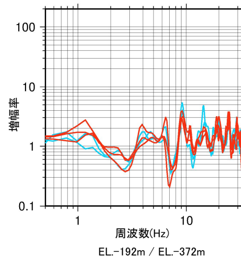
選定した5地震の伝達関数(UD方向)
