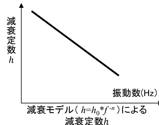
同定解析に用いる減衰モデル h のイメージ図
