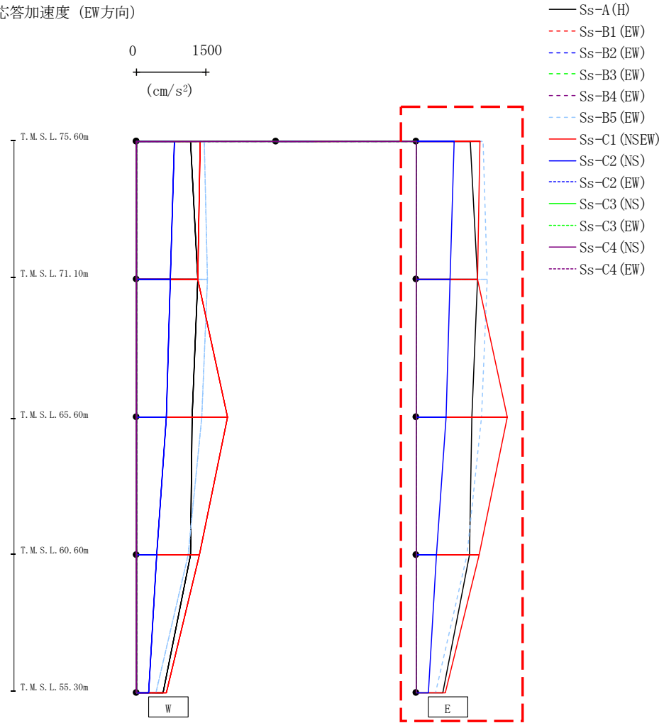
第4.2.1-29図 支持架構の最大応答加速度(+1σ地盤, EW断面③, 全応力解析) (2/2)
