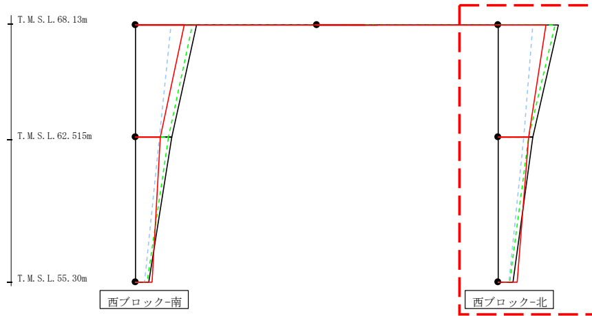
第4.2.2-25図 支持架構の最大応答加速度(-1σ地盤, NS断面①, 全応力解析) (2/2)
