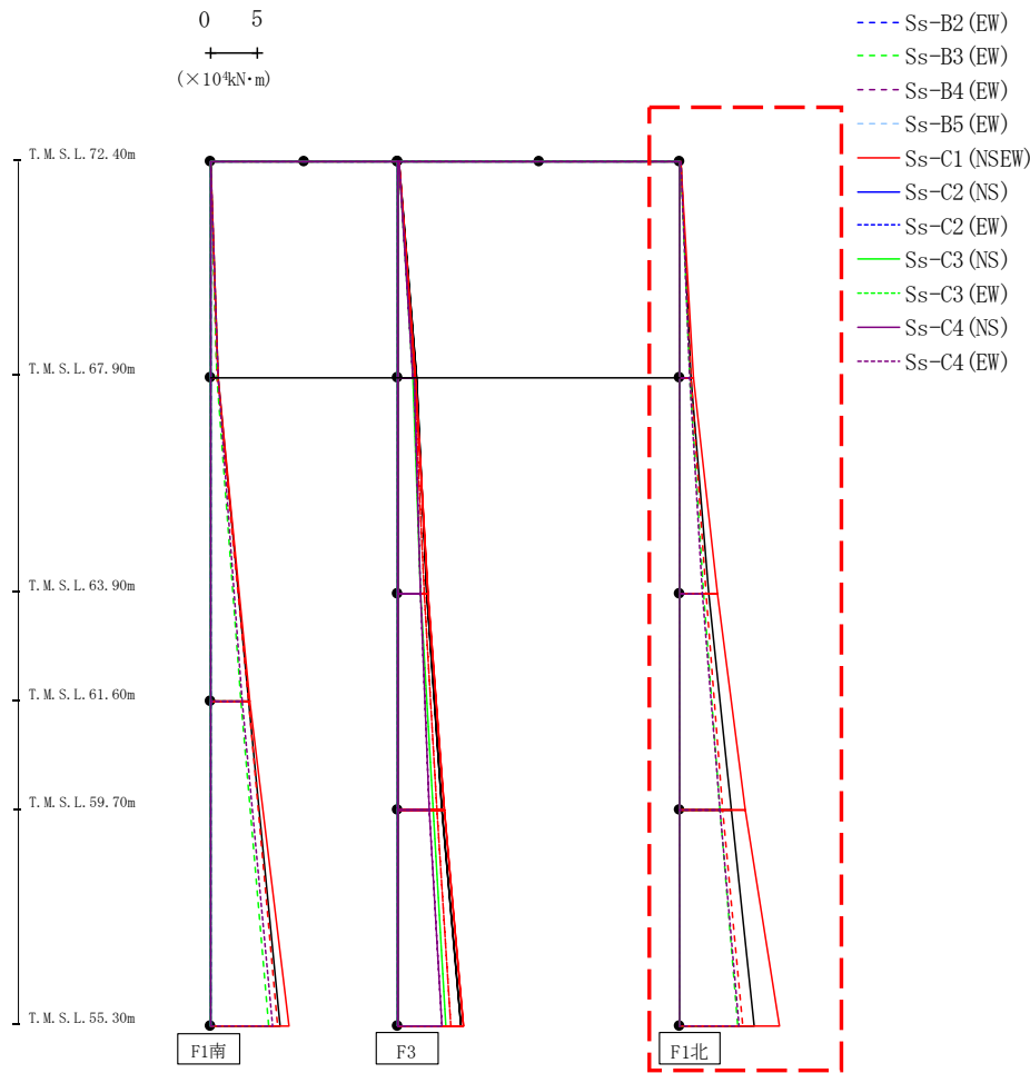
第4.2.2-31図 支持架構の最大応答曲げモーメント (G10B防護ネット架構, -1σ地盤, EW断面①) (3/3)
