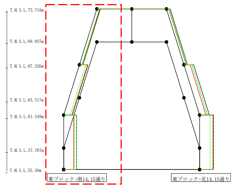
第4.2.1-26図 支持架構の最大応答せん断力(-1σ地盤, NS断面②, 全応力解析)(1/4)
