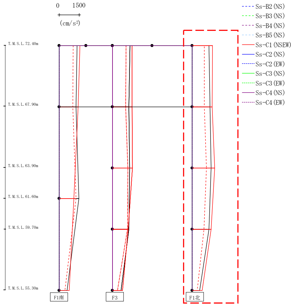
第4.2.1-25図 支持架構の最大応答加速度(G10A防護ネット架構, -1σ地盤, NS断面①)(3/3)
