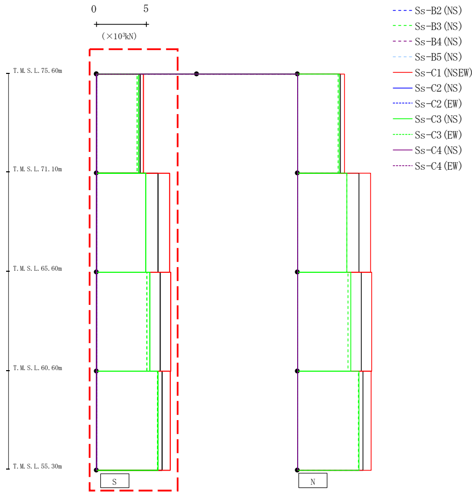
第4.2.1-38図 支持架構の最大応答せん断力(-1σ地盤, NS断面③, 全応力解析) (1/2)
