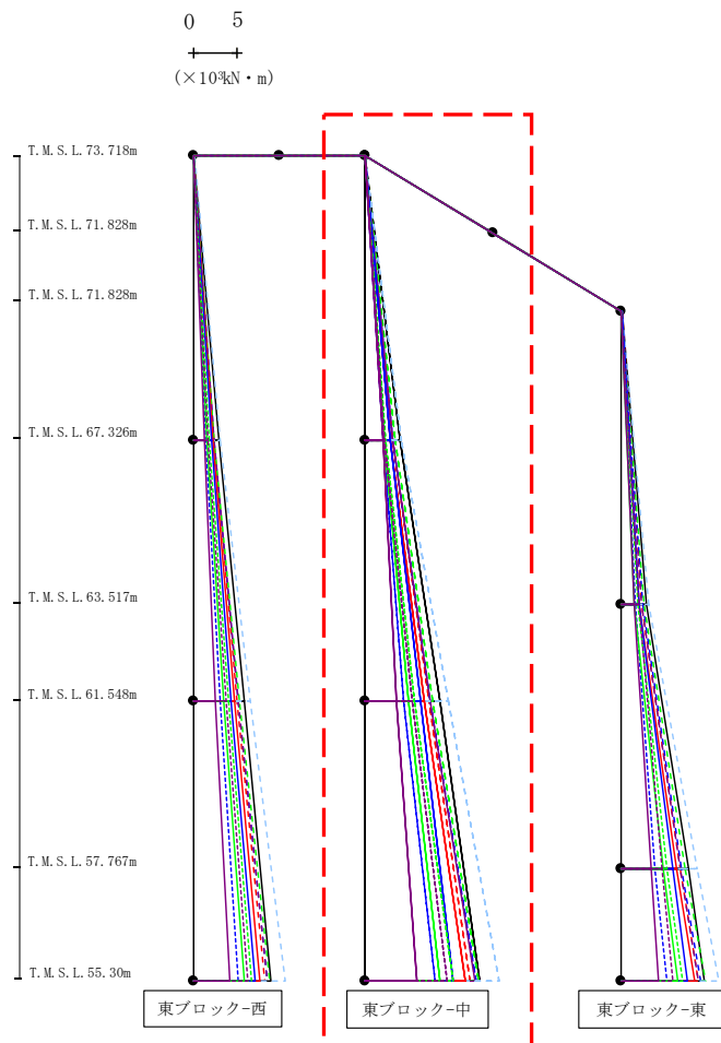
第4.2.1-43図 支持架構の最大応答曲げモーメント(基本ケース, EW断面③, 有効応力解析) (2/3)
