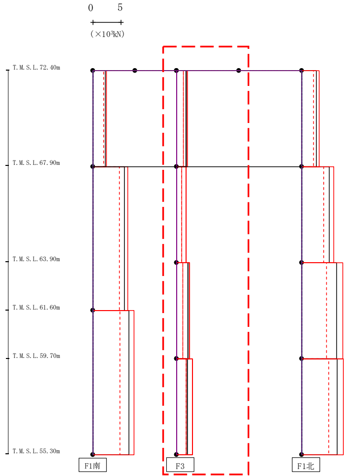
第4.2.1-14図 支持架構の最大応答せん断力(G10A防護ネット架構, +1σ地盤, NS断面①) (2/3)
