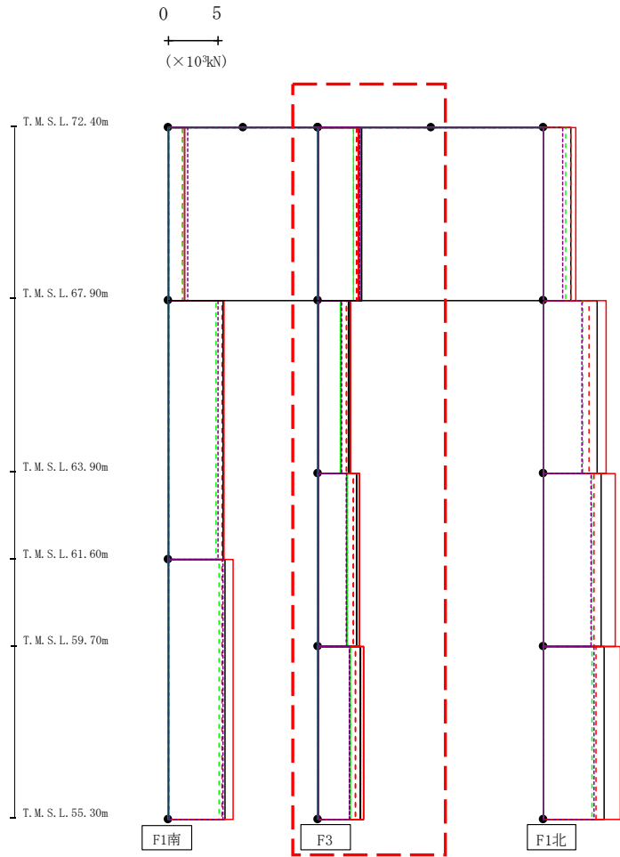
第4.2.2-18図 支持架構の最大応答せん断力(G10B防護ネット架構, +1σ地盤, EW断面①) (2/3)
