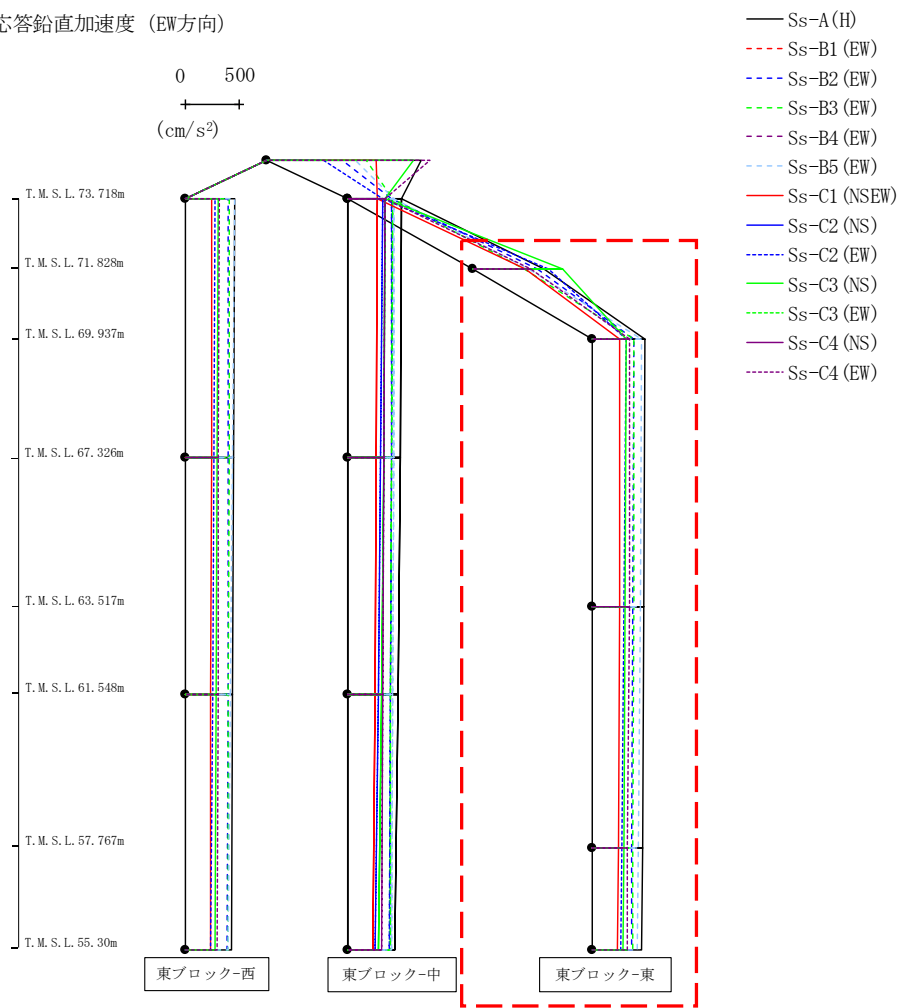
第4.2.1-68図 支持架構の最大応答鉛直加速度(-1σ地盤, EW断面③, 有効応力解析) (3/3)
