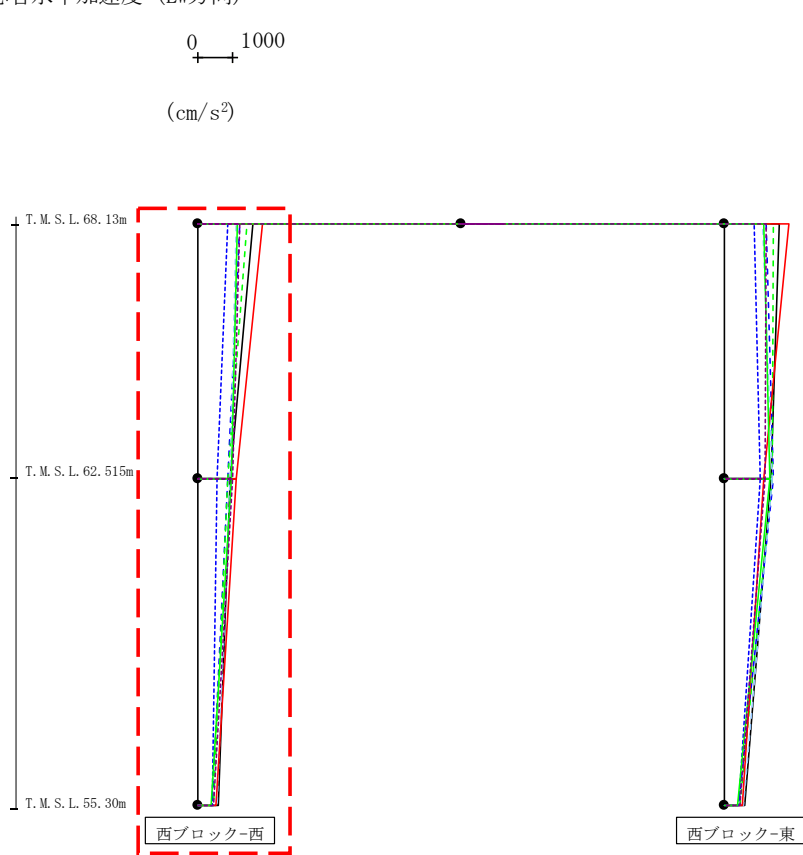
第4.2.2-53図 支持架構の最大応答加速度(+1σ地盤, EW断面③, 有効応力解析) (1/2)
