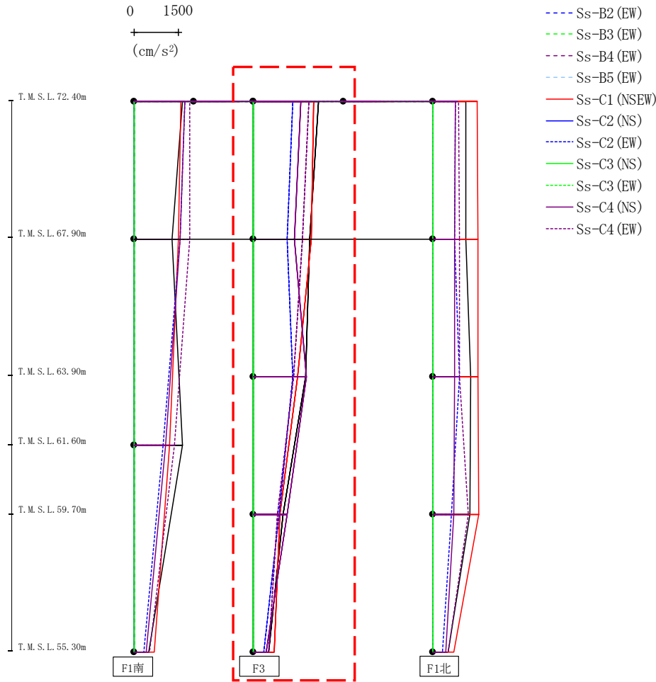
第4.2.2-21図 支持架構の最大応答加速度(G10B防護ネット架構, +1σ地盤, EW断面②)(2/3)
