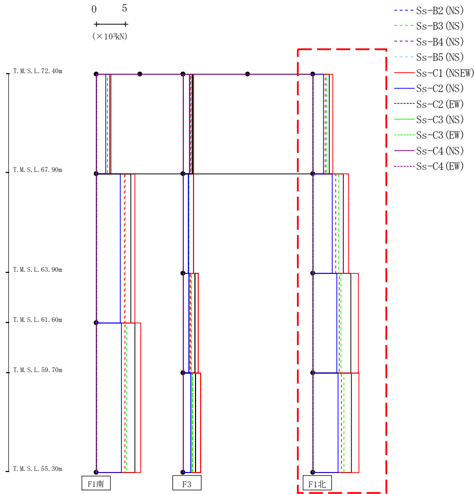
第4.2.2-26図 支持架構の最大応答せん断力(G10B防護ネット架構, -1σ地盤, NS断面②) (3/3)
