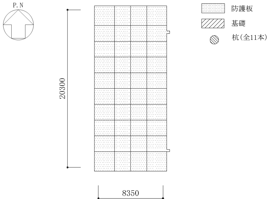
(a) 屋根伏図
