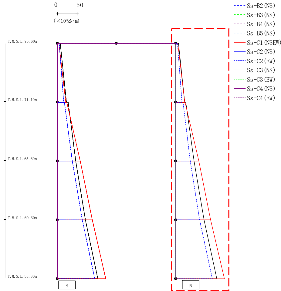
第4.2.1-35図 支持架構の最大応答曲げモーメント(-1σ地盤, NS断面①, 全応力解析)(2/2)
