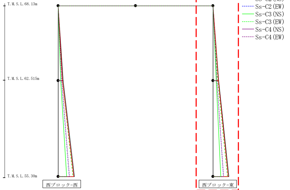
第4.2.2-35図 支持架構の最大応答曲げモーメント(-1σ地盤, EW断面④, 全応力解析) (2/2)
