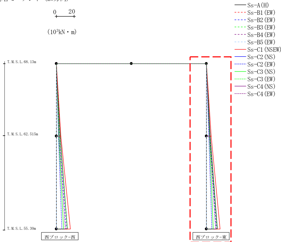
第4.2.2-55図 支持架構の最大応答曲げモーメント(+1σ地盤, EW断面③, 有効応力解析) (2/2)
