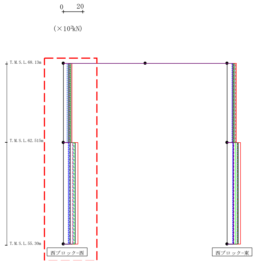
第4.2.2-42図 支持架構の最大応答せん断力(基本ケース, EW断面③, 有効応力解析)(1/2)
