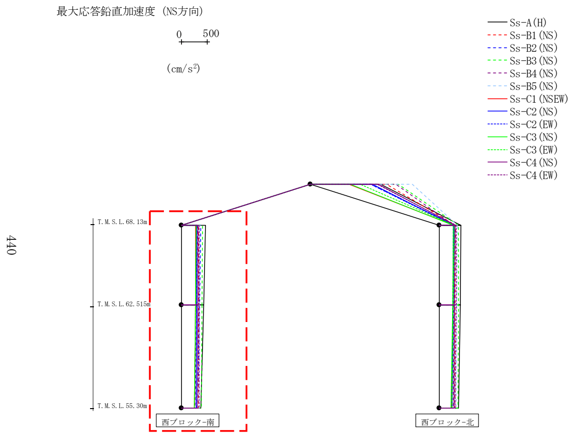
第4.2.2-40図 支持架構の最大応答鉛直加速度(基本ケース, NS断面①, 有効応力解析)(1/2)
