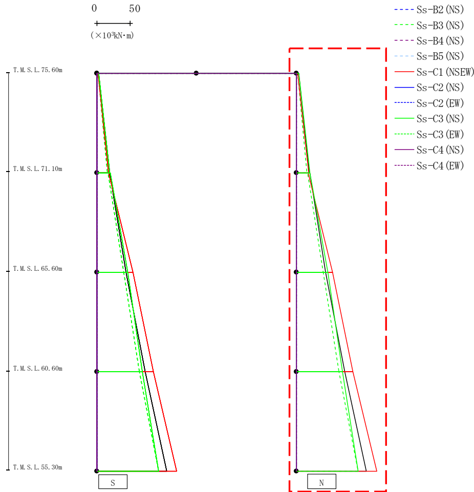
第4.2.1-23図 支持架構の最大応答曲げモーメント(+1σ地盤, NS断面③, 全応力解析)(2/2)
