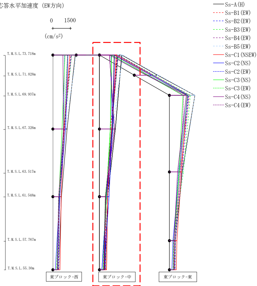
第4.2.1-41図 支持架構の最大応答加速度(基本ケース, EW断面③, 有効応力解析)(2/3)
