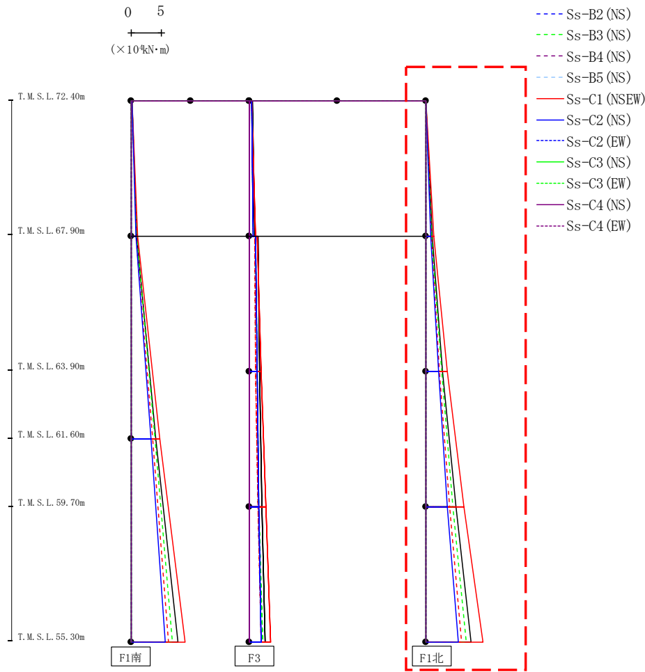
第4.2.2-15図 支持架構の最大応答曲げモーメント (G10B防護ネット架構, +1σ地盤, NS断面②) (3/3)
