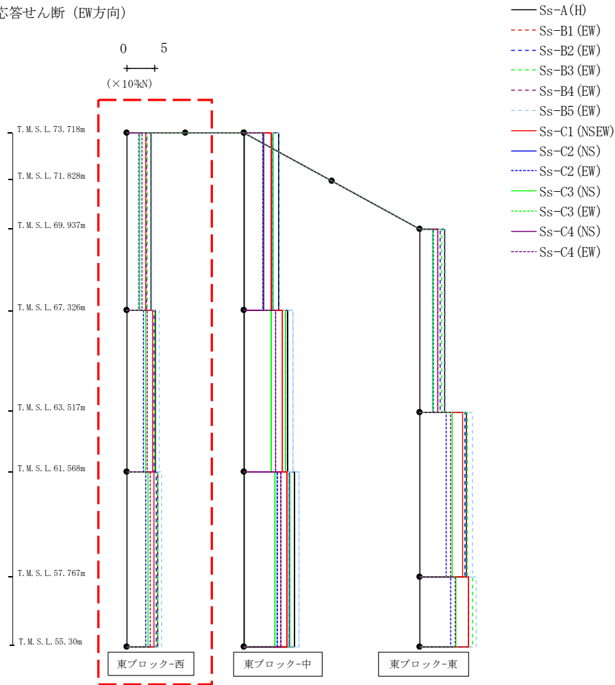
第4.2.1-54図 支持架構の最大応答せん断力(+1σ地盤, EW断面③, 有効応力解析) (1/3)
