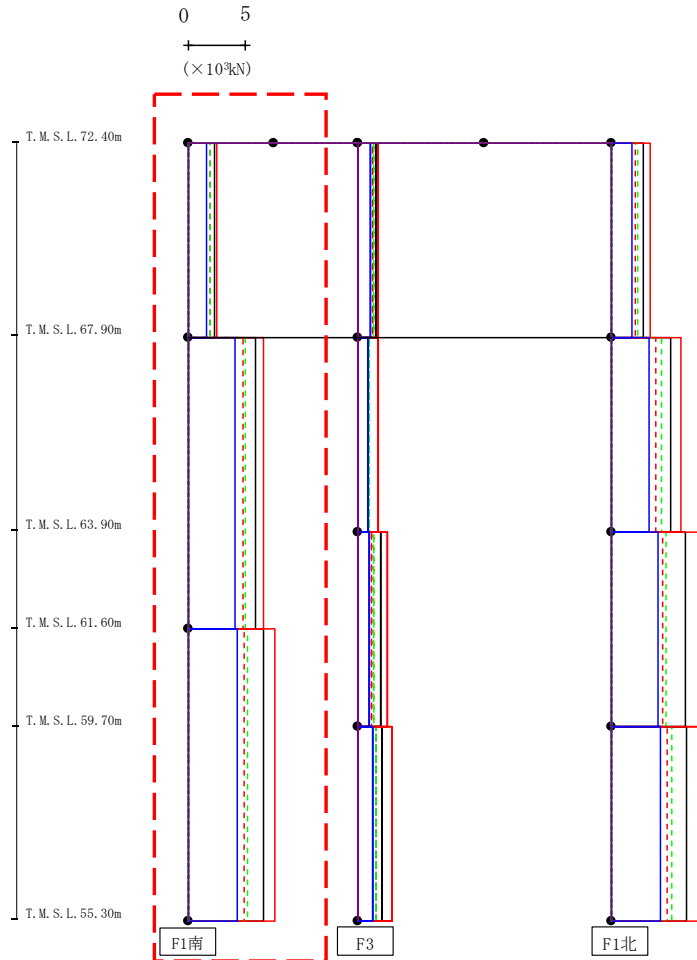
第4.2.2-26図 支持架構の最大応答せん断力(G10B防護ネット架構, -1σ地盤, NS断面②) (1/3)
