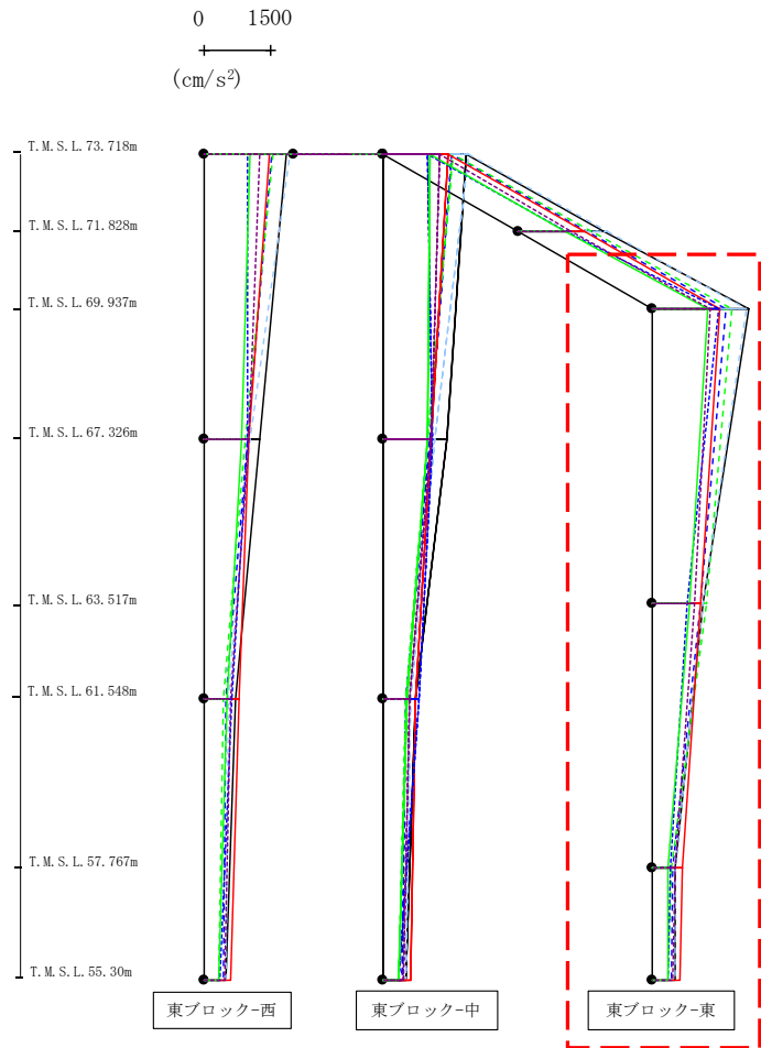
第4.2.1-53図 支持架構の最大応答加速度(+1σ地盤, EW断面③, 有効応力解析) (3/3)
