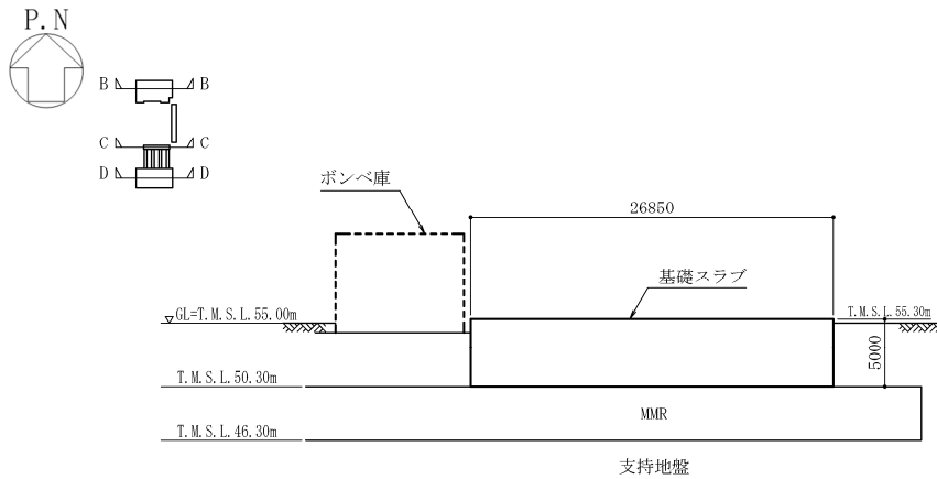
(b) B-B断面図(EW方向)
