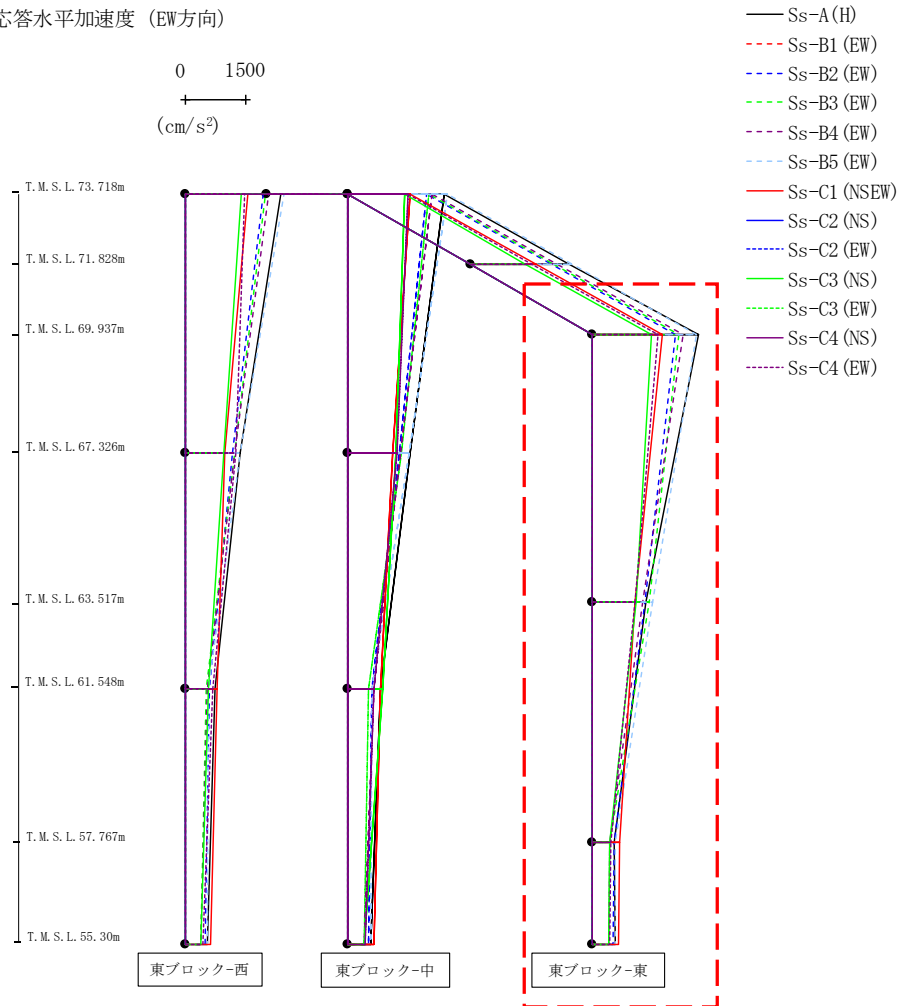
第4.2.1-69図 支持架構の最大応答加速度(-1σ地盤, EW断面④, 有効応力解析) (3/3)
