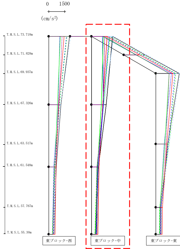
第4.2.1-65図 支持架構の最大応答加速度(-1σ地盤, EW断面③, 有効応力解析) (2/3)
