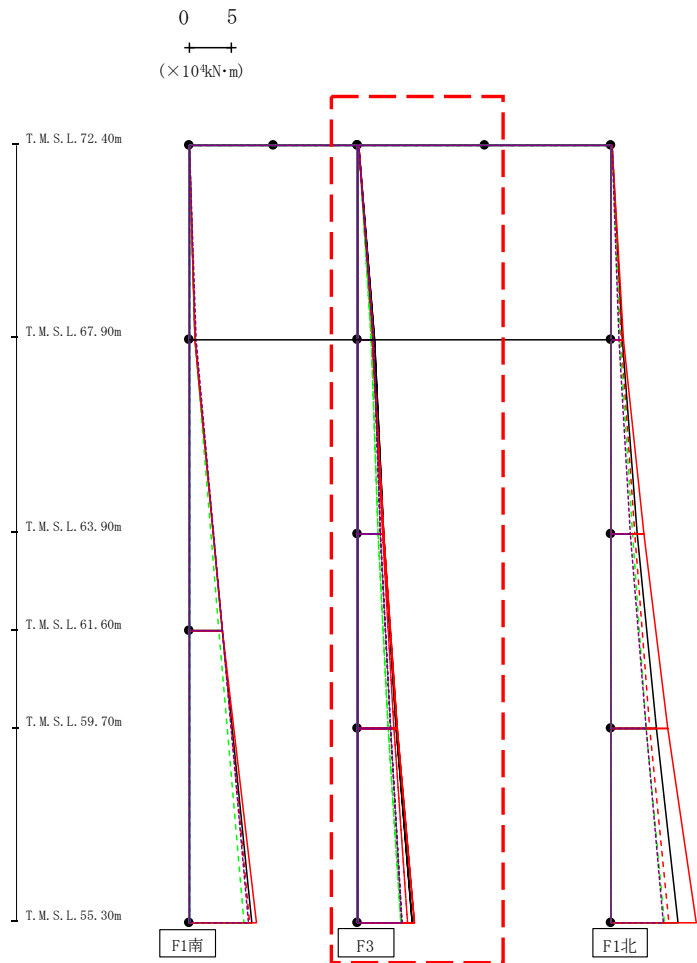
第4.2.2-19図 支持架構の最大応答曲げモーメント (G10B防護ネット架構, +1σ地盤, EW断面①) (2/3)
