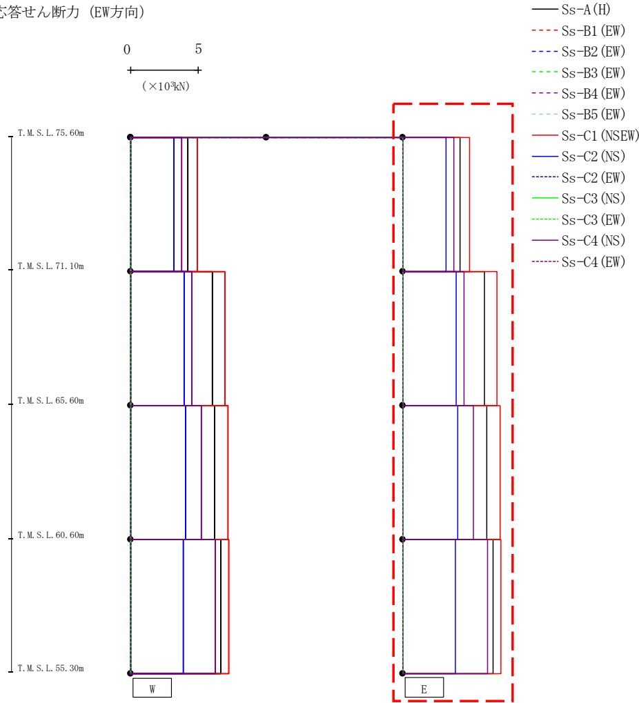
第4.2.2-30図 支持架構の最大応答せん断力(+1σ地盤, EW断面③, 有効応力解析) (2/2)
