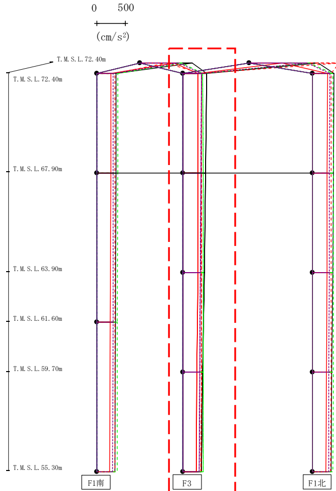
第4.2.1-24図 支持架構の最大応答鉛直加速度(G10A防護ネット架構, +1σ地盤, EW断面②)(2/3)
