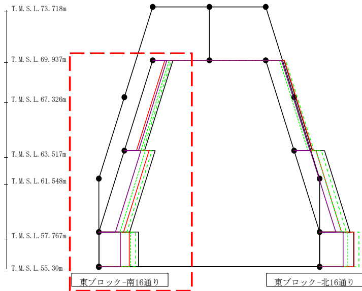
第4.2.1-50図 支持架構の最大応答せん断力(+1σ地盤, NS断面②, 有効応力解析) (3/4)
