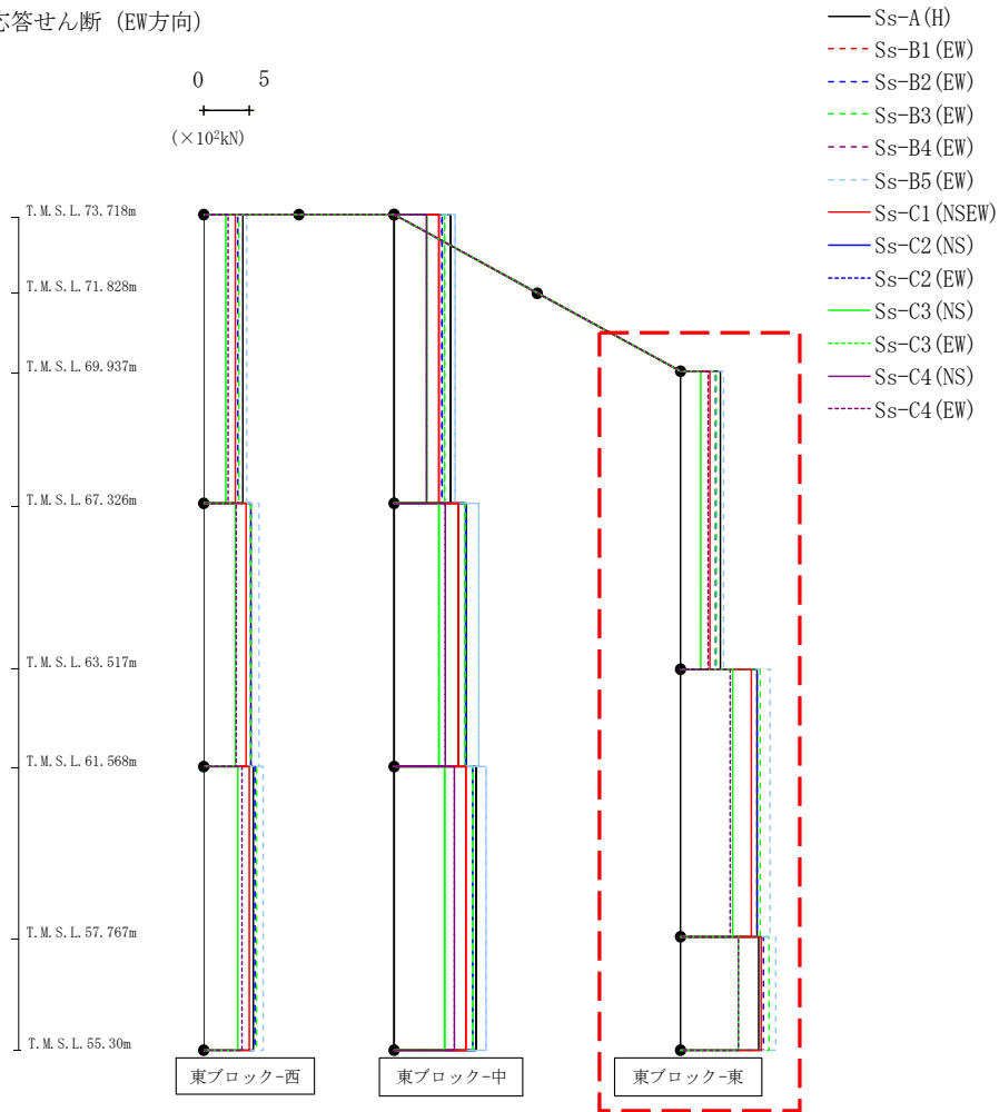
第4.2.2-18図 支持架構の最大応答せん断力(+1σ地盤, EW断面③, 全応力解析) (3/3)
