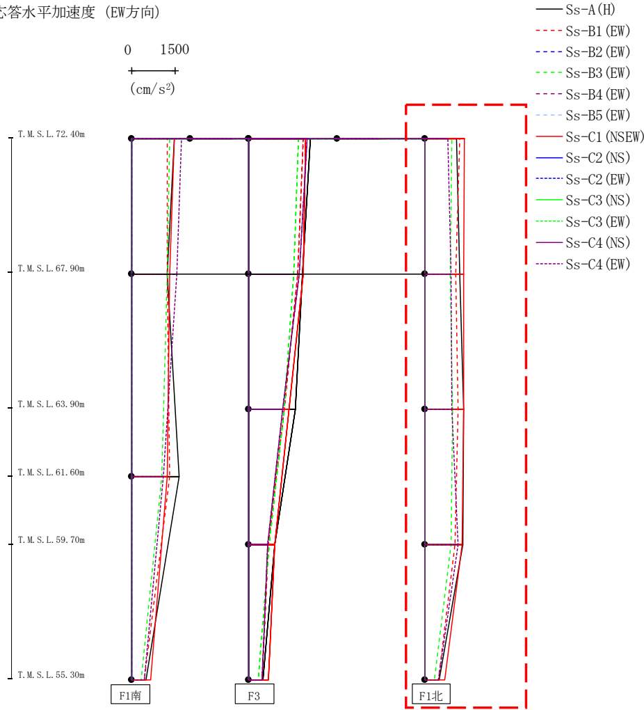
第4.2.2-17図 支持架構の最大応答加速度(G10B防護ネット架構, +1σ地盤, EW断面①) (3/3)
