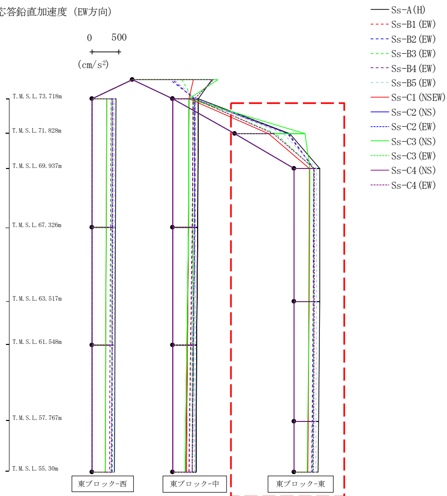
第4.2.1-72図 支持架構の最大応答鉛直加速度(-1σ地盤, EW断面④, 有効応力解析) (3/3)
