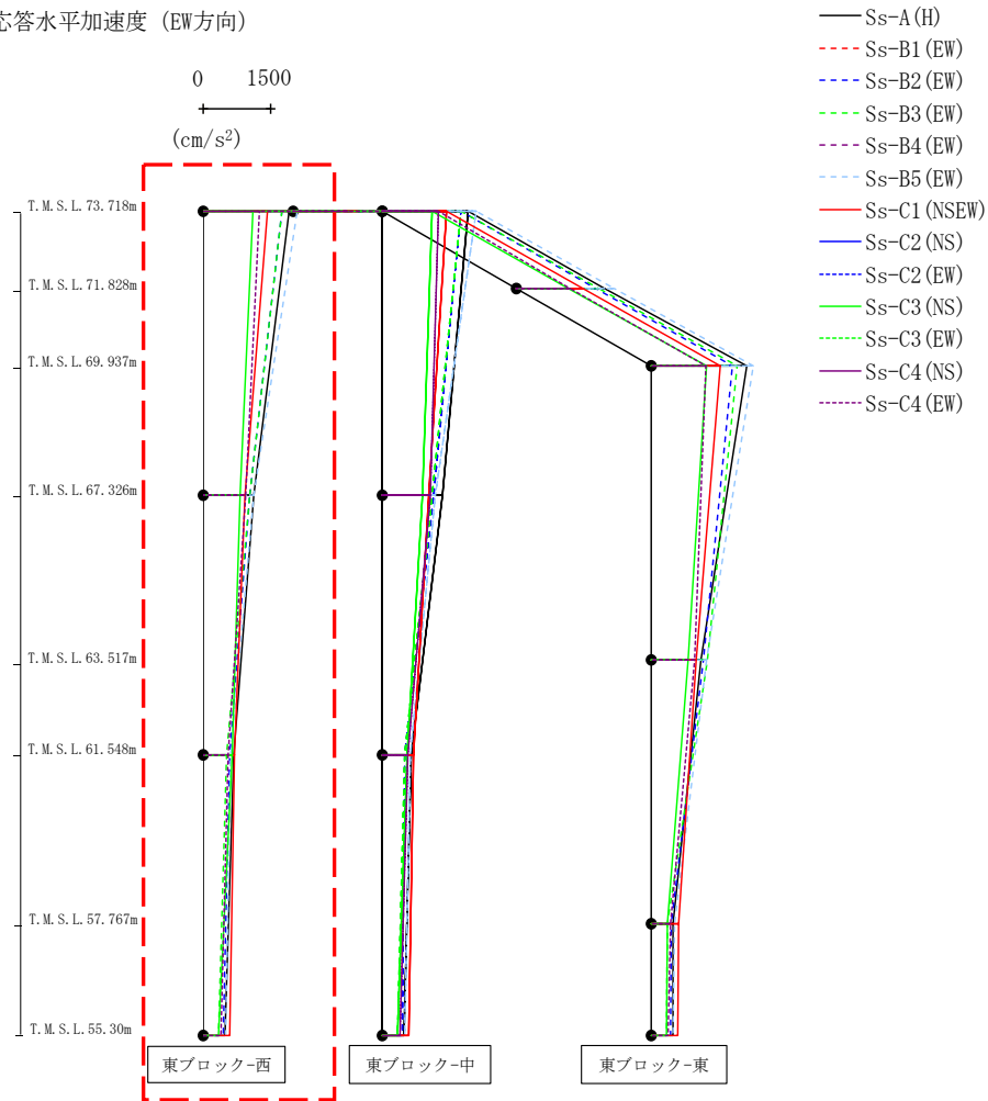
第4.2.1-29図 支持架構の最大応答加速度(-1σ地盤, EW断面③, 全応力解析) (1/3)
