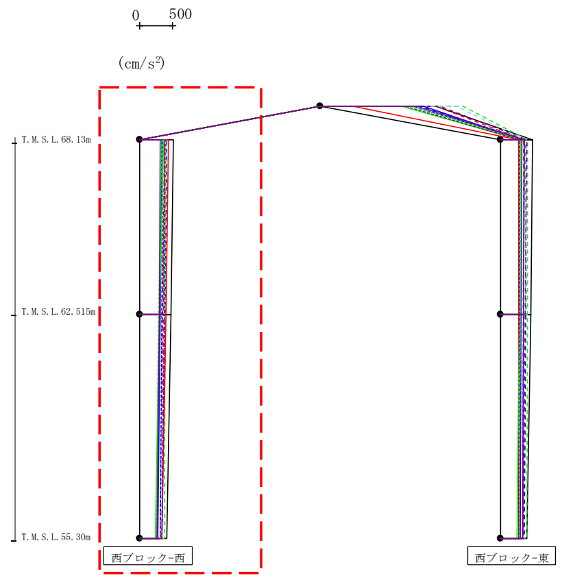
第4.2.2-48図 支持架構の最大応答鉛直加速度(基本ケース, EW断面④, 有効応力解析)(1/2)
