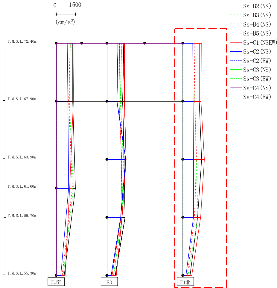
第4.2.2-25図 支持架構の最大応答加速度(G10B防護ネット架構, -1σ地盤, NS断面②) (3/3)
