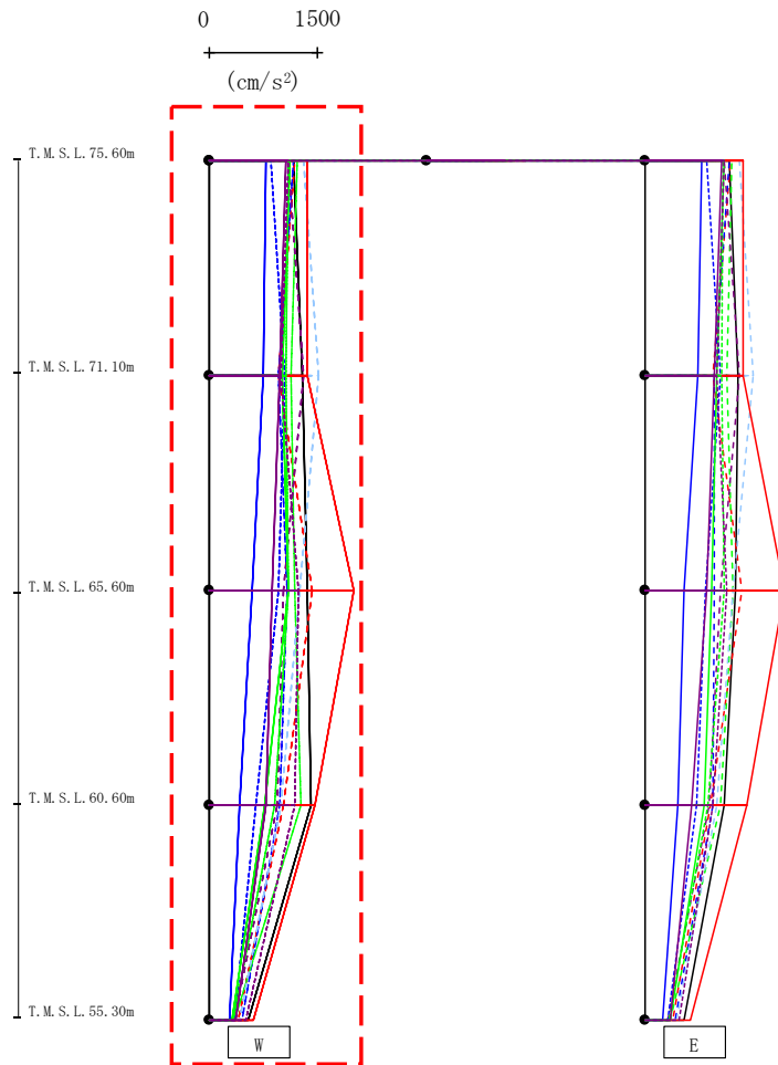
第4.2.2-9図 支持架構の最大応答加速度(基本ケース, EW断面①, 有効応力解析)(1/2)
