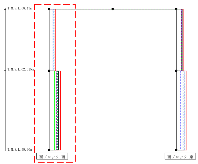
第4.2.2-66図 支持架構の最大応答せん断力(-1σ地盤, EW断面③, 有効応力解析) (1/2)
