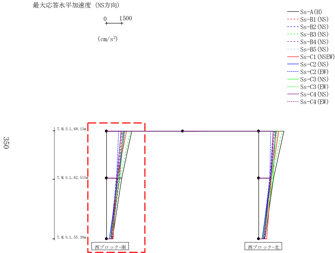
第4.2.2-1図 支持架構の最大応答加速度(基本ケース, NS断面①, 全応力解析) (1/2)
