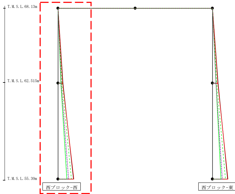
第4.2.2-23図 支持架構の最大応答曲げモーメント(+1σ地盤, EW断面④, 全応力解析)(1/2)
