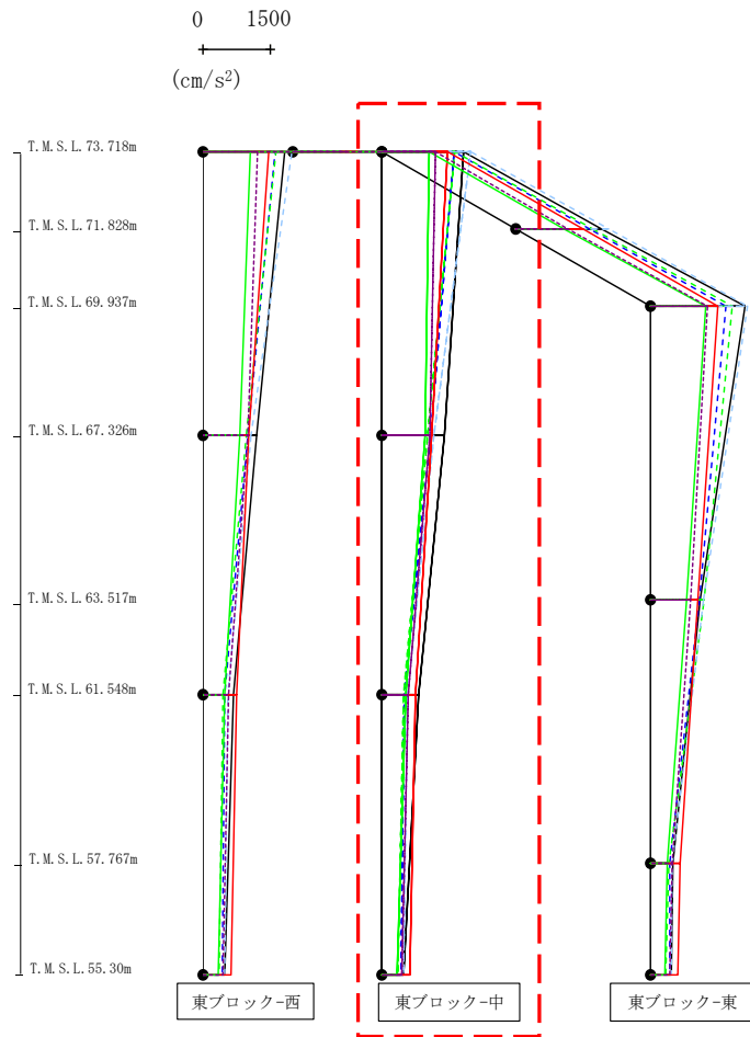
第4.2.1-17図 支持架構の最大応答加速度(+1σ地盤, EW断面③, 全応力解析) (2/3)
