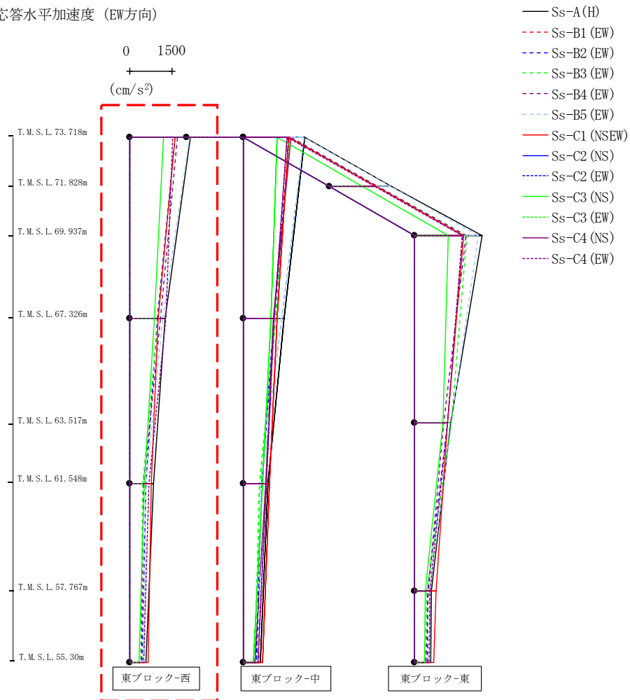
第4.2.1-57図 支持架構の最大応答加速度(+1σ地盤, EW断面④, 有効応力解析) (1/3)
