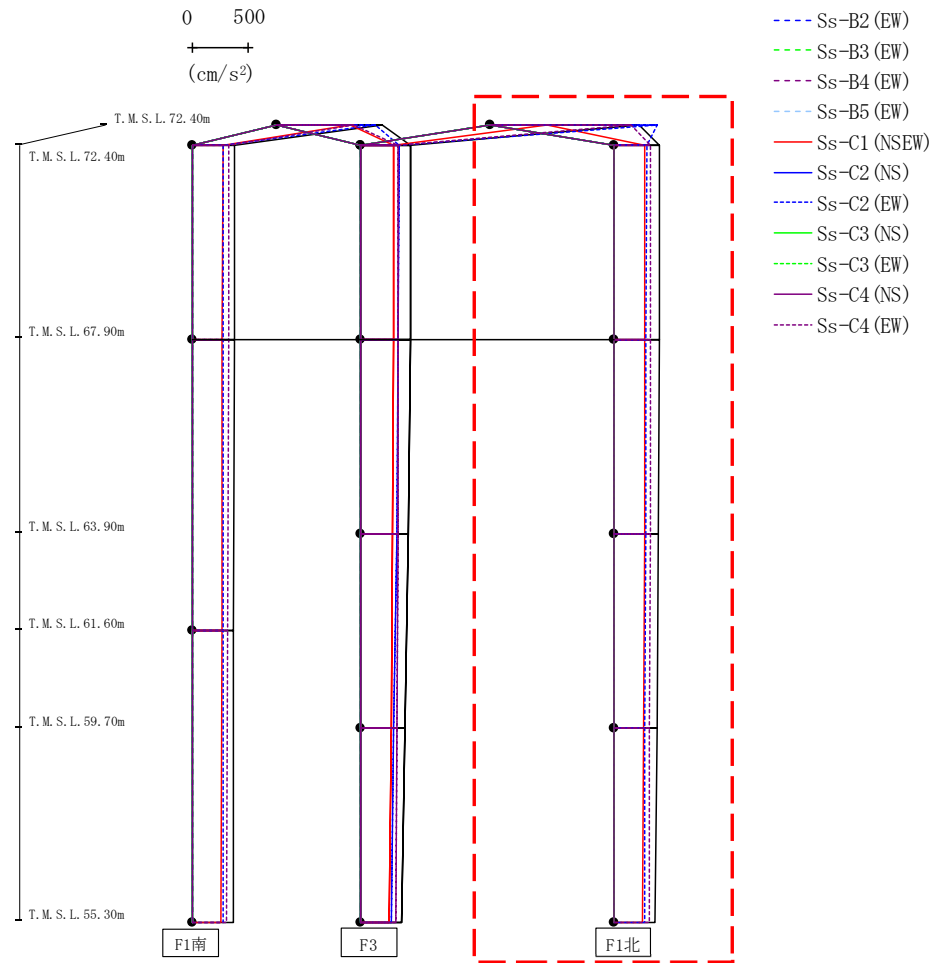
第4.2.1-32図 支持架構の最大応答鉛直加速度(G10A防護ネット架構, -1σ地盤, EW断面①)(3/3)
