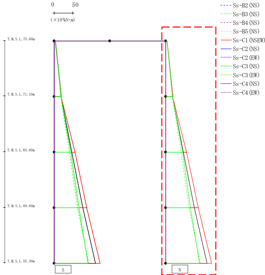
第4.2.1-39図 支持架構の最大応答曲げモーメント(-1σ地盤, NS断面③, 全応力解析)(2/2)
