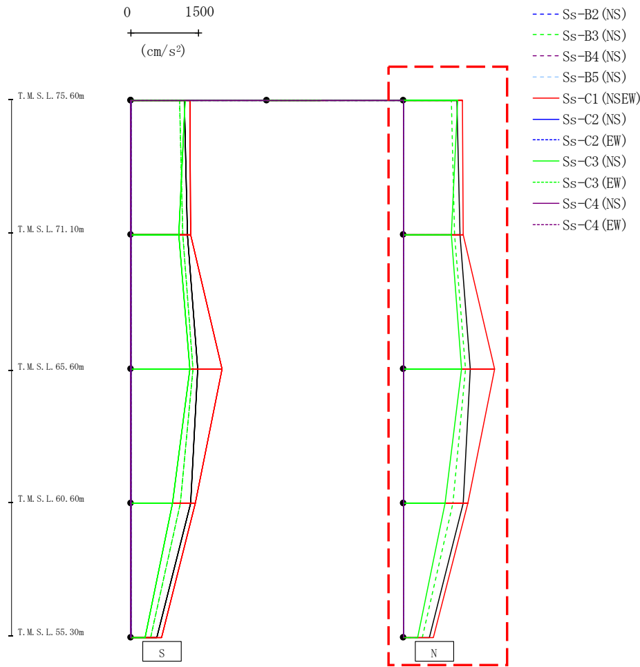
第4.2.2-21図 支持架構の最大応答加速度(+1σ地盤, NS断面③, 有効応力解析)(2/2)
