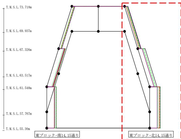
第4.2.1-50図 支持架構の最大応答せん断力(+1 \sigma 地盤, NS断面②, 有効応力解析) (2/4)
