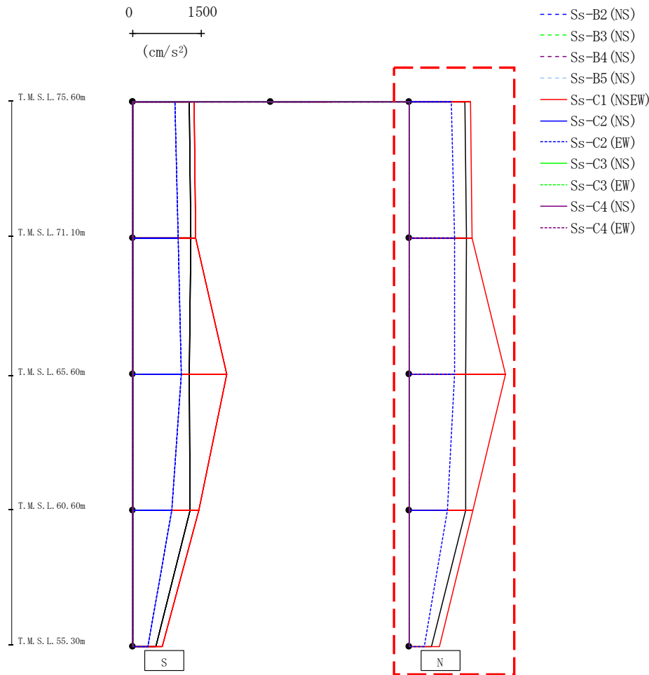
第4.2.2-17図 支持架構の最大応答加速度(+1σ地盤, NS断面①, 有効応力解析)(2/2)
