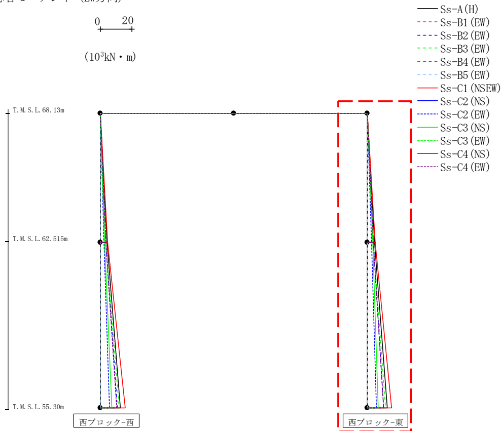
第4.2.2-67図 支持架構の最大応答曲げモーメント(-1σ地盤, EW断面③, 有効応力解析) (2/2)
