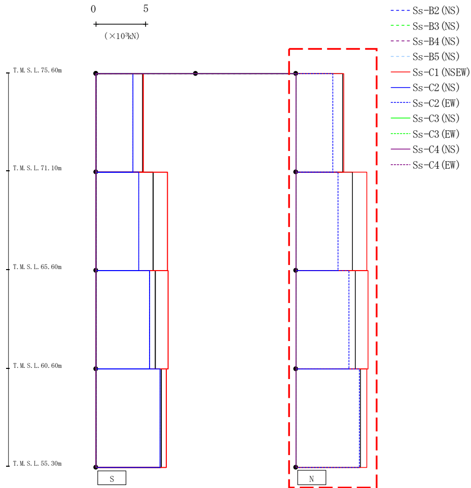
第4.2.2-34図 支持架構の最大応答せん断力(-1σ地盤, NS断面①, 有効応力解析) (2/2)
