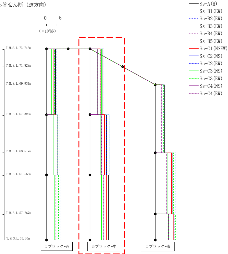
第4.2.1-18図 支持架構の最大応答せん断力(+1σ地盤, EW断面③, 全応力解析) (2/3)
