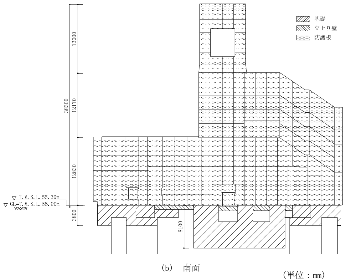
第2.2-4図 飛来物防護板架構の概略側面図(2/4)
