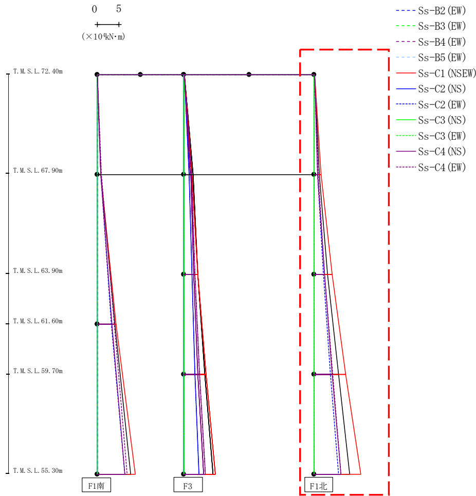
第4.2.2-23図 支持架構の最大応答曲げモーメント (G10B防護ネット架構, +1σ地盤, EW断面②) (3/3)
