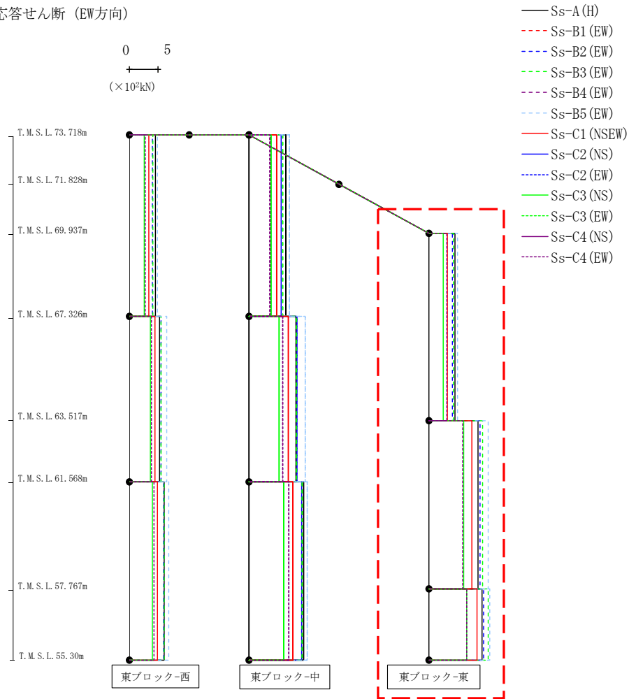
第4.2.1-30図 支持架構の最大応答せん断力(-1σ地盤, EW断面③, 全応力解析) (3/3)
