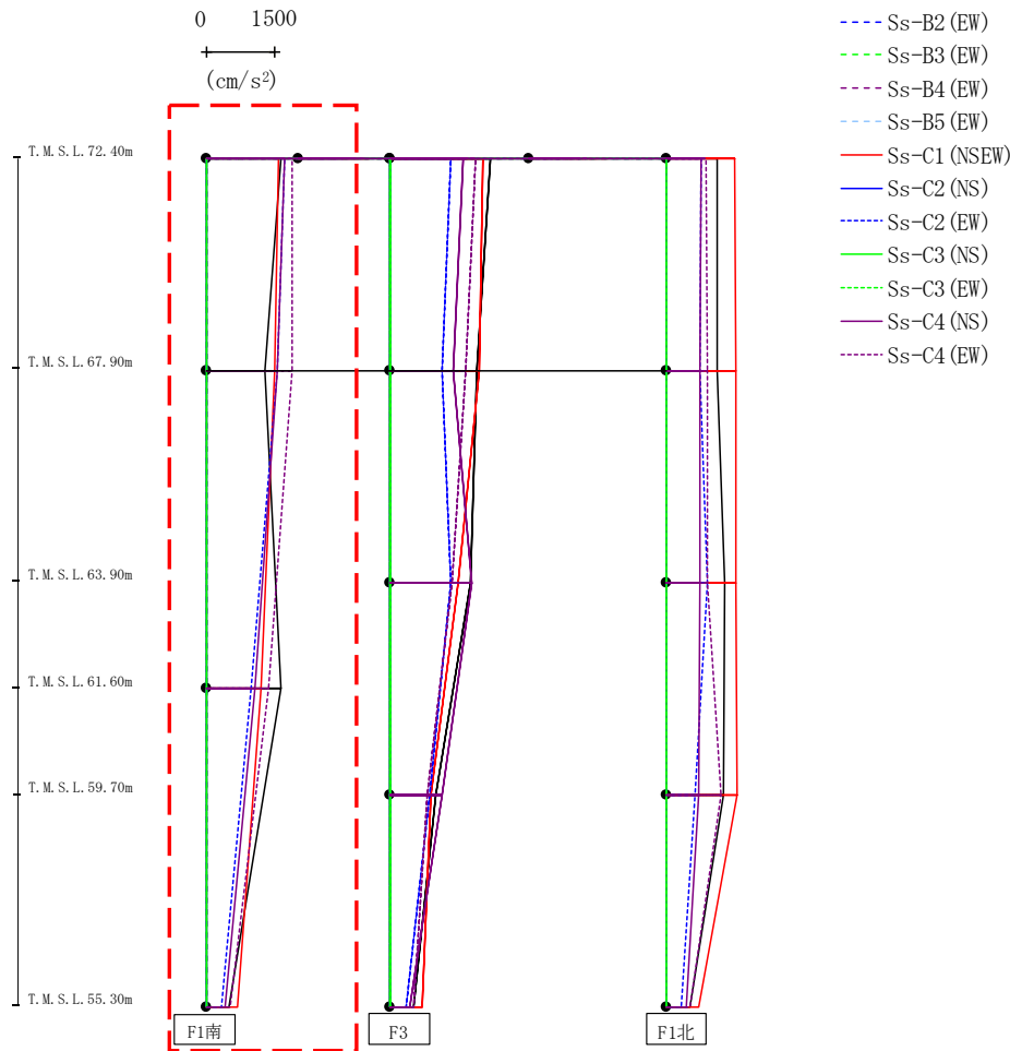
第4.2.2-21図 支持架構の最大応答加速度(G10B防護ネット架構, +1σ地盤, EW断面②)(1/3)
