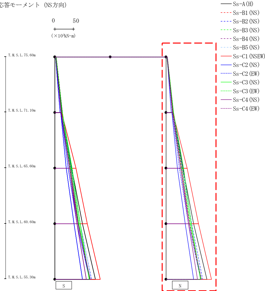
第4.2.1-7図 支持架構の最大応答曲げモーメント(基本ケース, NS断面③, 全応力解析)(2/2)
