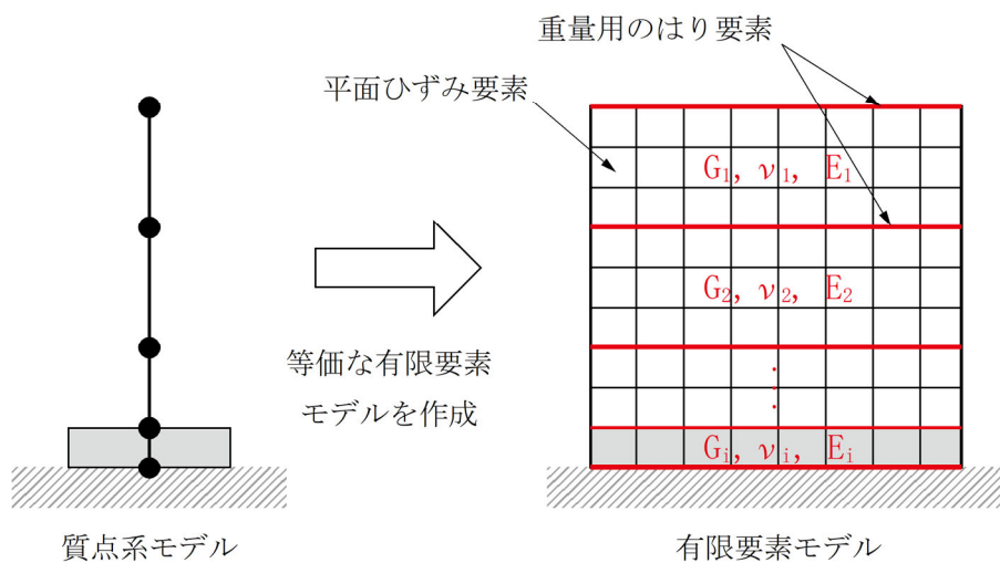
第3.2.3-1図 前処理建屋のモデル化手法概念図
