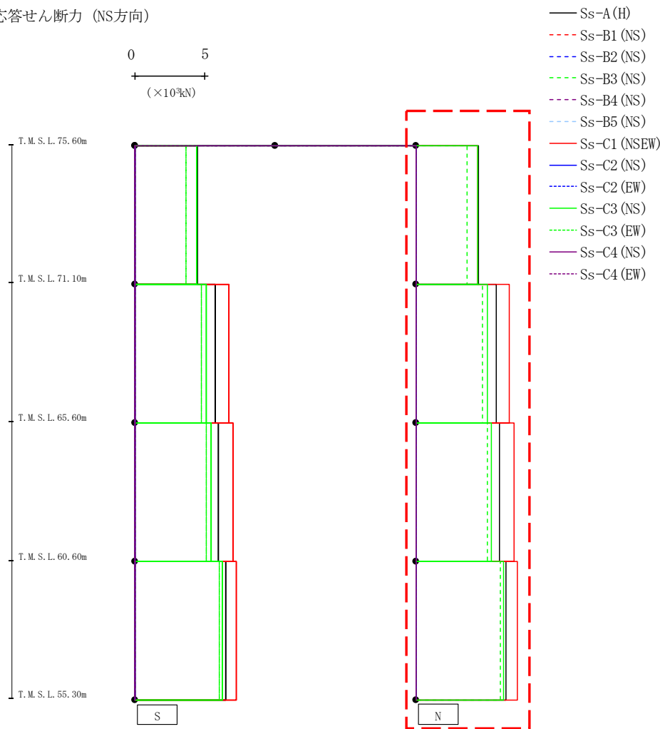
第4.2.1-22図 支持架構の最大応答せん断力(+1σ地盤, NS断面③, 全応力解析) (2/2)
