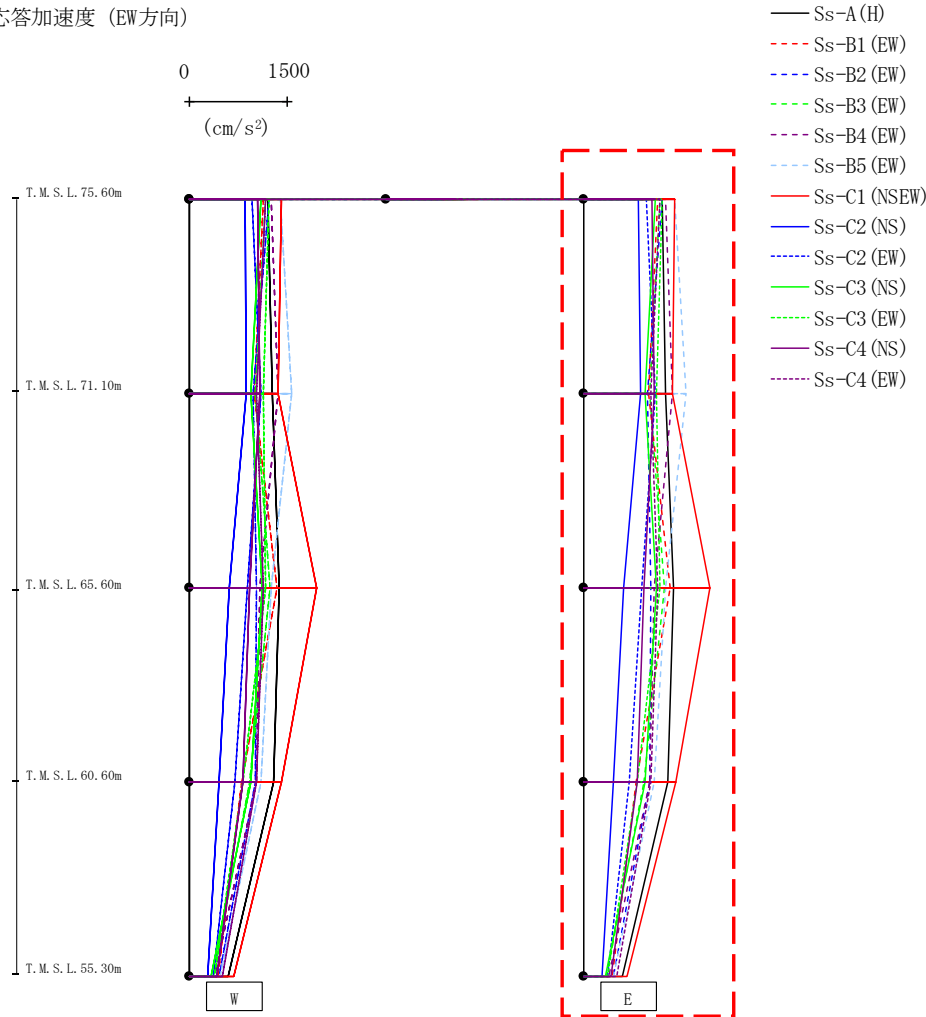
第4.2.1-13図 支持架構の最大応答加速度(基本ケース, EW断面③, 全応力解析)(2/2)
