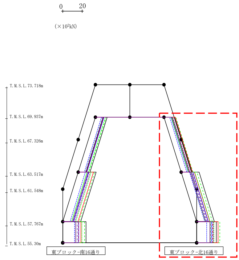
第4.2.1-2図 支持架構の最大応答せん断力(基本ケース, NS断面②, 全応力解析) (4/4)
