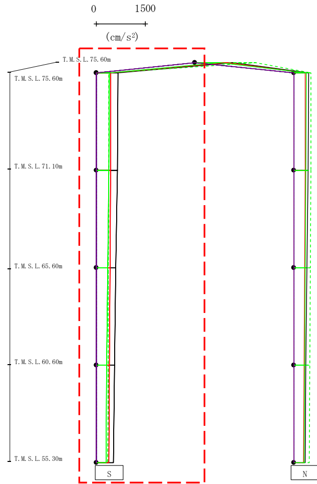
第4.2.1-40図 支持架構の最大応答鉛直加速度(-1σ地盤, NS断面③, 全応力解析)(1/2)
