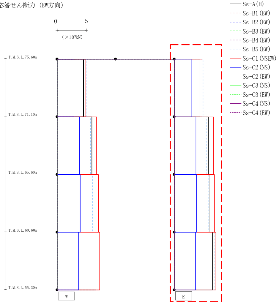
第4.2.2-26図 支持架構の最大応答せん断力(+1σ地盤, EW断面①, 有効応力解析) (2/2)
