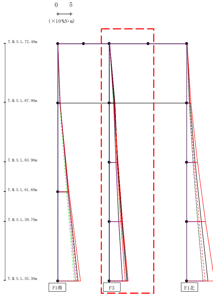
第4.2.1-23図 支持架構の最大応答曲げモーメント(G10A防護ネット架構, +1σ地盤, EW断面②) (2/3)
