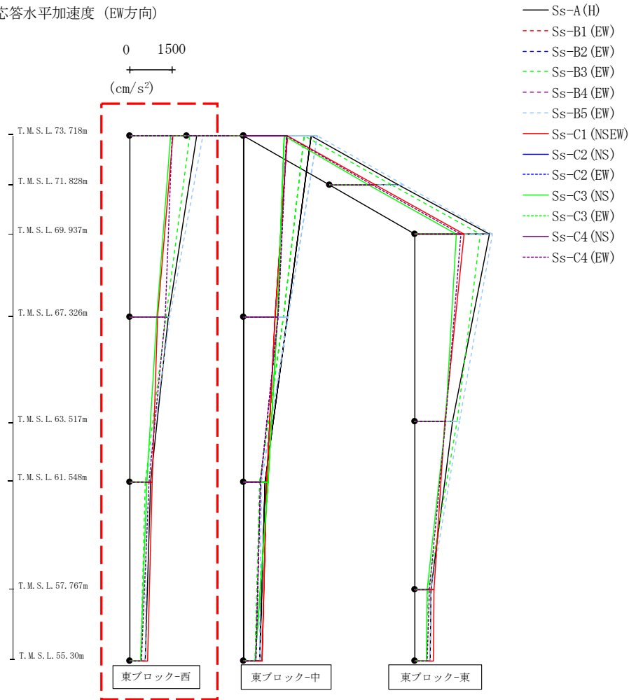
第4. 2. 1-33図 支持架構の最大応答加速度(-1σ地盤, EW断面④, 全応力解析) (1/3)
