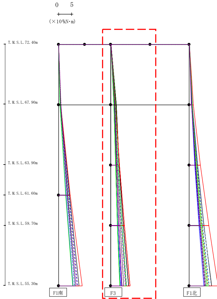
第4.2.2-11図 支持架構の最大応答曲げモーメント (G10B防護ネット架構, 基本ケース, EW断面②) (2/3)
