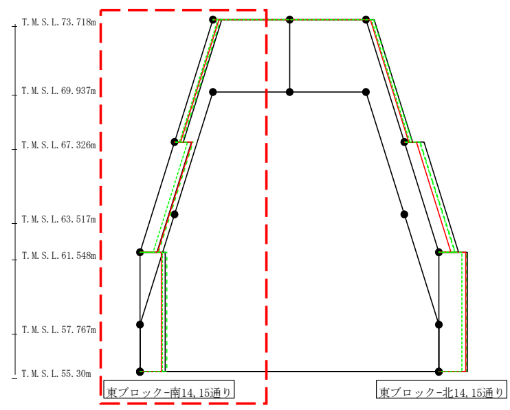
第4.2.1-14図 支持架構の最大応答せん断力(+1σ地盤, NS断面②, 全応力解析)(1/4)
