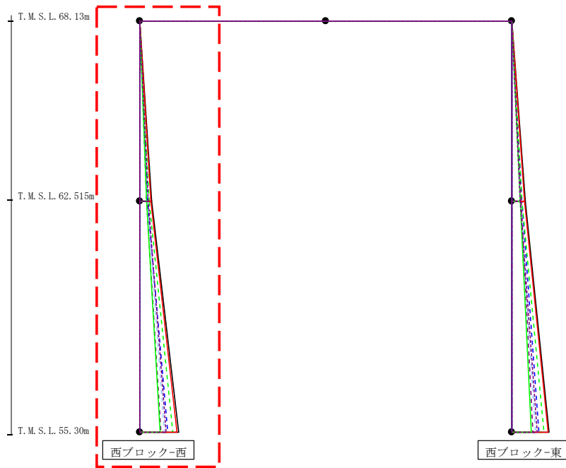
第4.2.2-71図 支持架構の最大応答曲げモーメント(-1σ地盤, EW断面④, 有効応力解析) (1/2)
