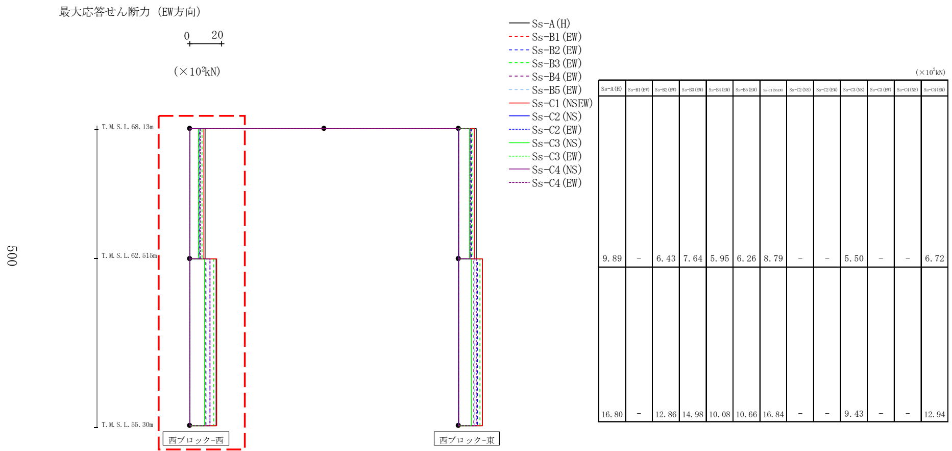
第4.2.2-70図 支持架構の最大応答せん断力(-1σ地盤, EW断面④, 有効応力解析) (1/2)
