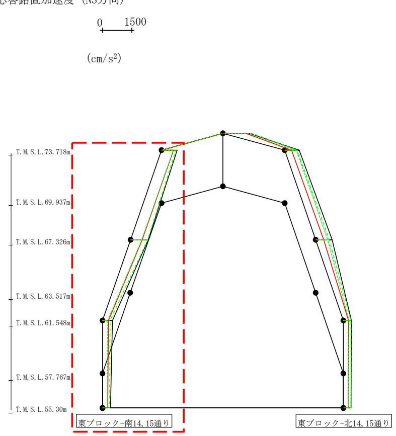
第4.2.1-16図 支持架構の最大応答鉛直加速度(+1σ地盤, NS断面②, 全応力解析) (1/4)
