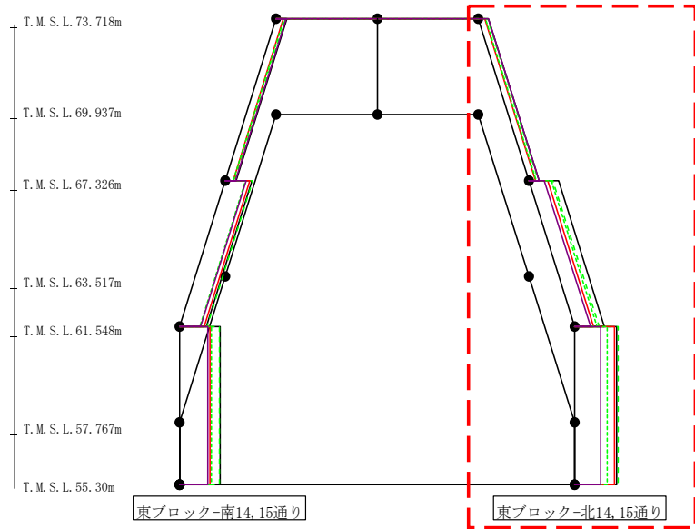
第4.2.1-62図 支持架構の最大応答せん断力(-1σ地盤, NS断面②, 有効応力解析) (2/4)
