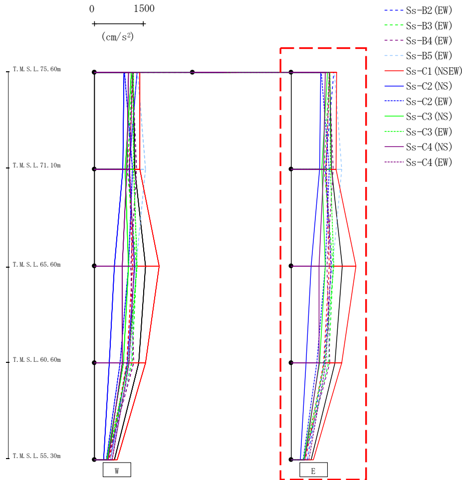
第4.2.2-13図 支持架構の最大応答加速度(基本ケース, EW断面③, 有効応力解析)(2/2)
