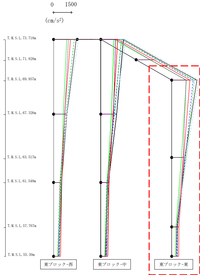
第4.2.1-29図 支持架構の最大応答加速度(-1σ地盤, EW断面③, 全応力解析) (3/3)
