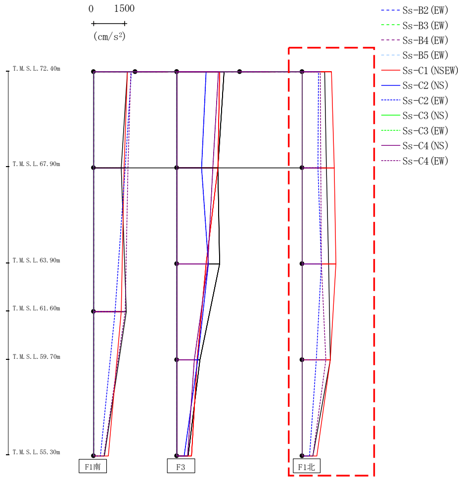
第4.2.1-17図 支持架構の最大応答加速度(G10A防護ネット架構, +1σ地盤, EW断面①) (3/3)
