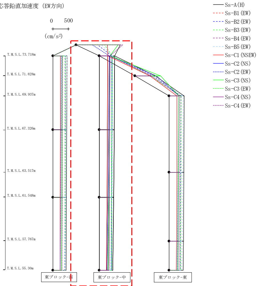
第4.2.1-68図 支持架構の最大応答鉛直加速度(-1σ地盤, EW断面③, 有効応力解析) (2/3)
