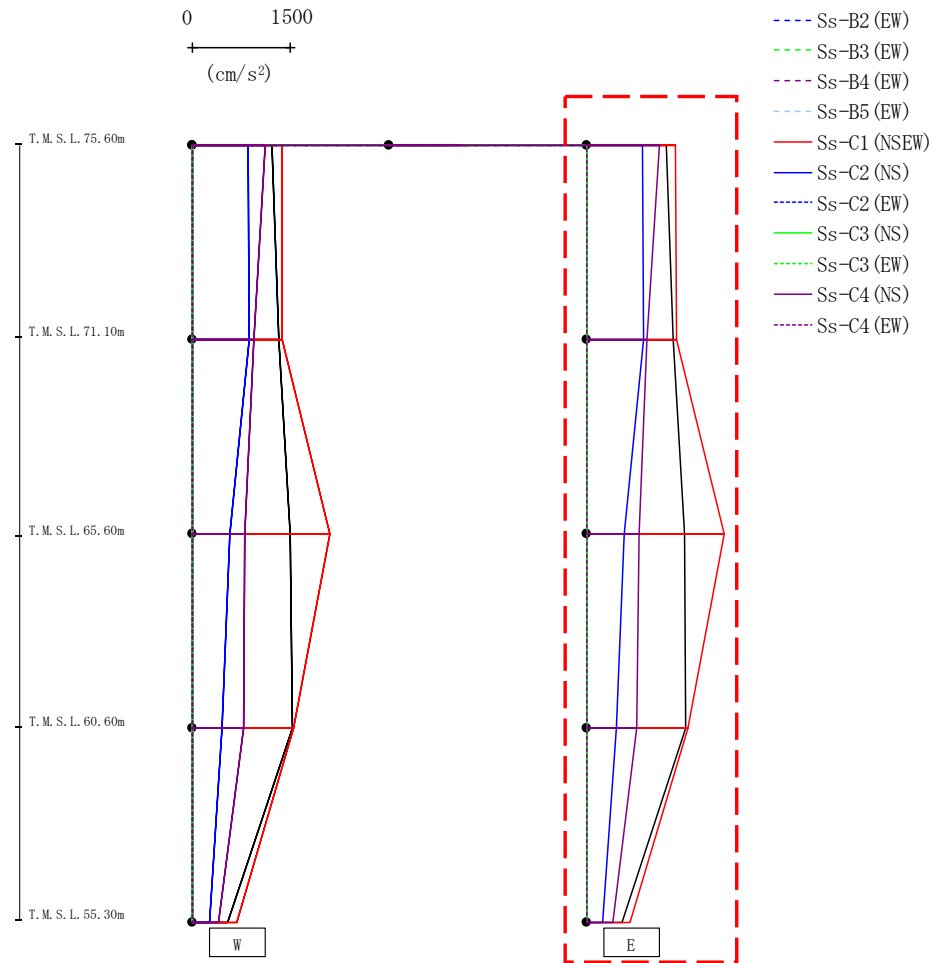
第4.2.2-45図 支持架構の最大応答加速度(-1σ地盤, EW断面③, 有効応力解析)(2/2)
