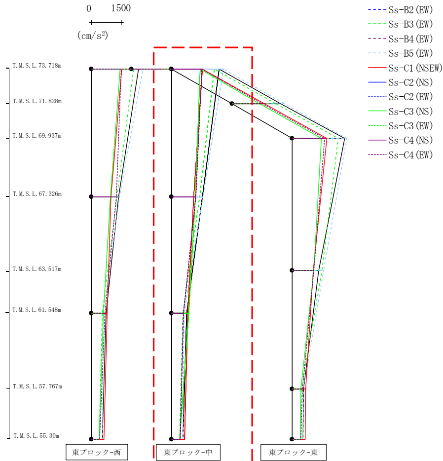
第4.2.1-33図 支持架構の最大応答加速度(-1σ地盤, EW断面④, 全応力解析) (2/3)
