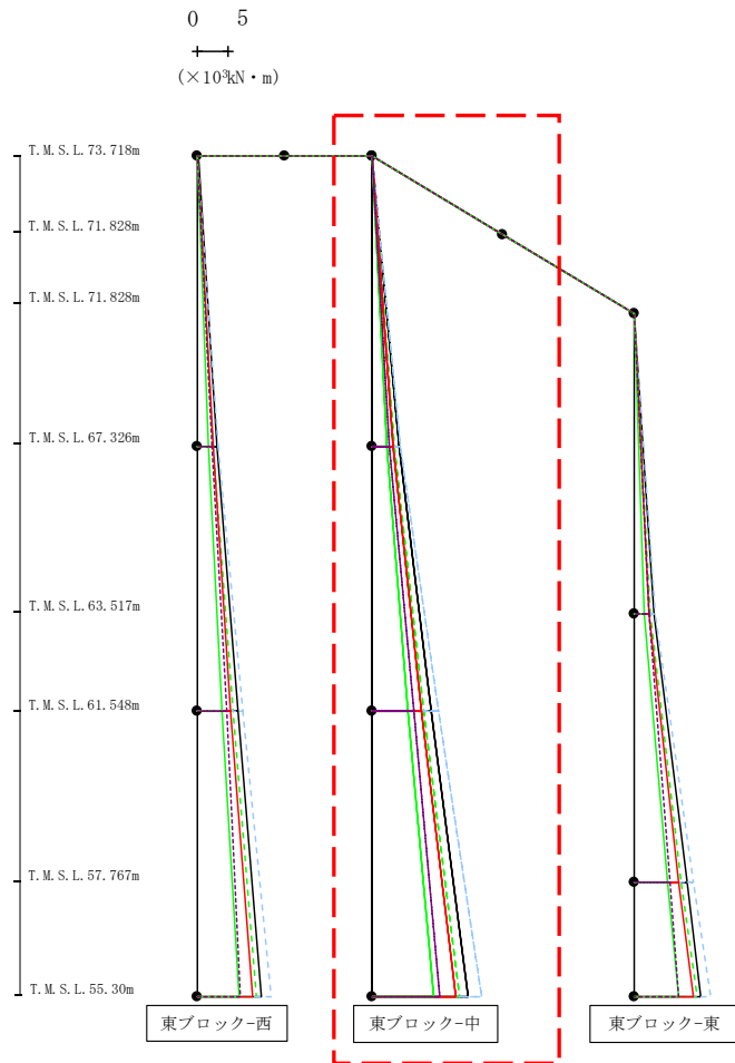
第4.2.1-23図 支持架構の最大応答曲げモーメント(+1σ地盤, EW断面④, 全応力解析) (2/3)
