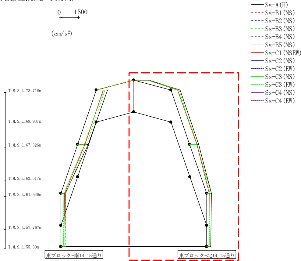
第4.2.1-28図 支持架構の最大応答鉛直加速度(-1σ地盤, NS断面②, 全応力解析) (2/4)
