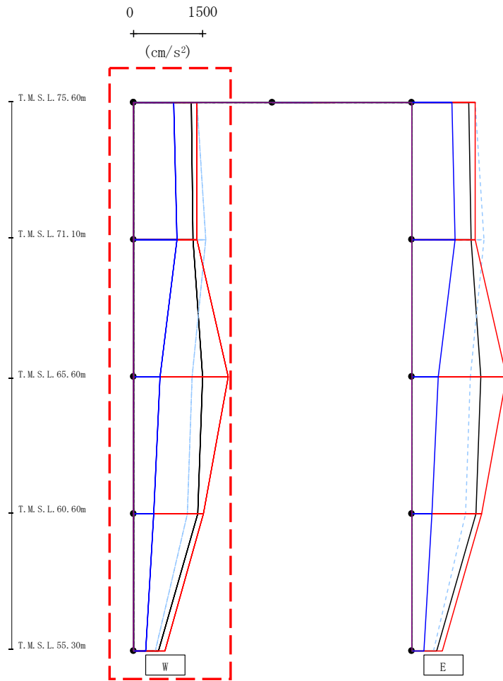
第4.2.1-45図 支持架構の最大応答加速度(-1σ地盤, EW断面③, 全応力解析)(1/2)
