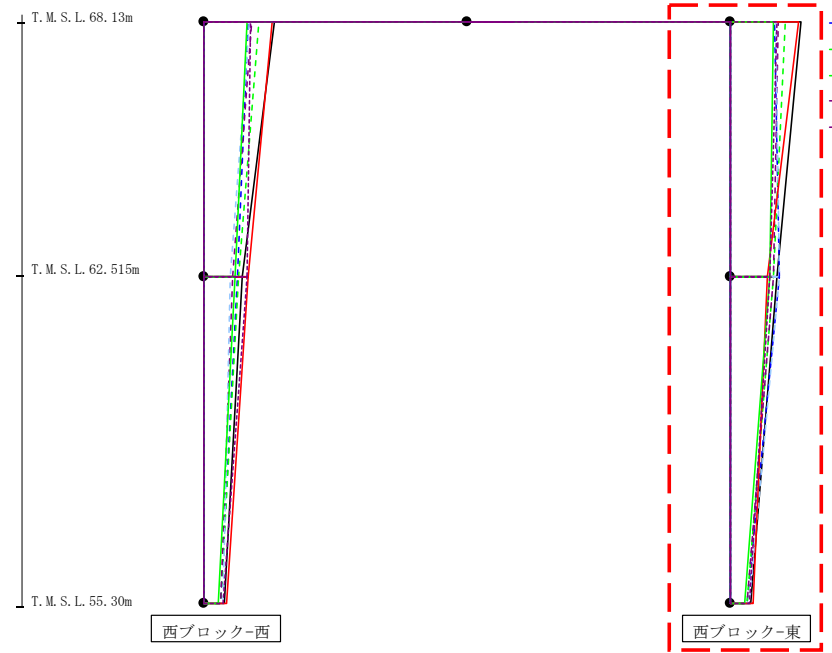
第4.2.2-57図 支持架構の最大応答加速度(+1σ地盤, EW断面④, 有効応力解析)(2/2)
