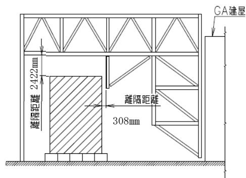
(A-A断面)
