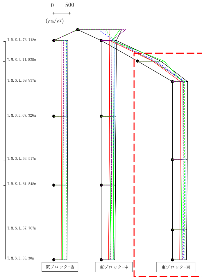
第4.2.1-32図 支持架構の最大応答鉛直加速度(-1σ地盤, EW断面③, 全応力解析) (3/3)
