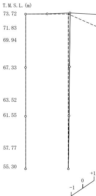
第4.1.1-2図 刺激関数図(EW方向モデル, EW断面③)(3/3)
