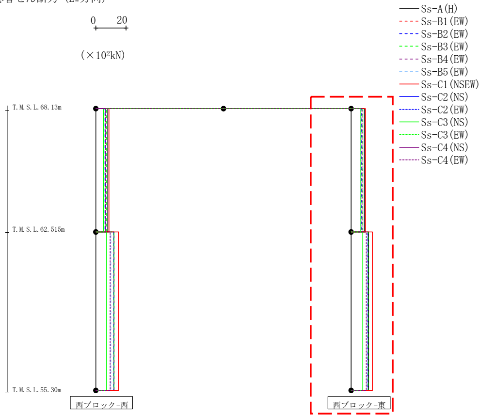
第4.2.2-30図 支持架構の最大応答せん断力(-1σ地盤, EW断面③, 全応力解析) (2/2)
