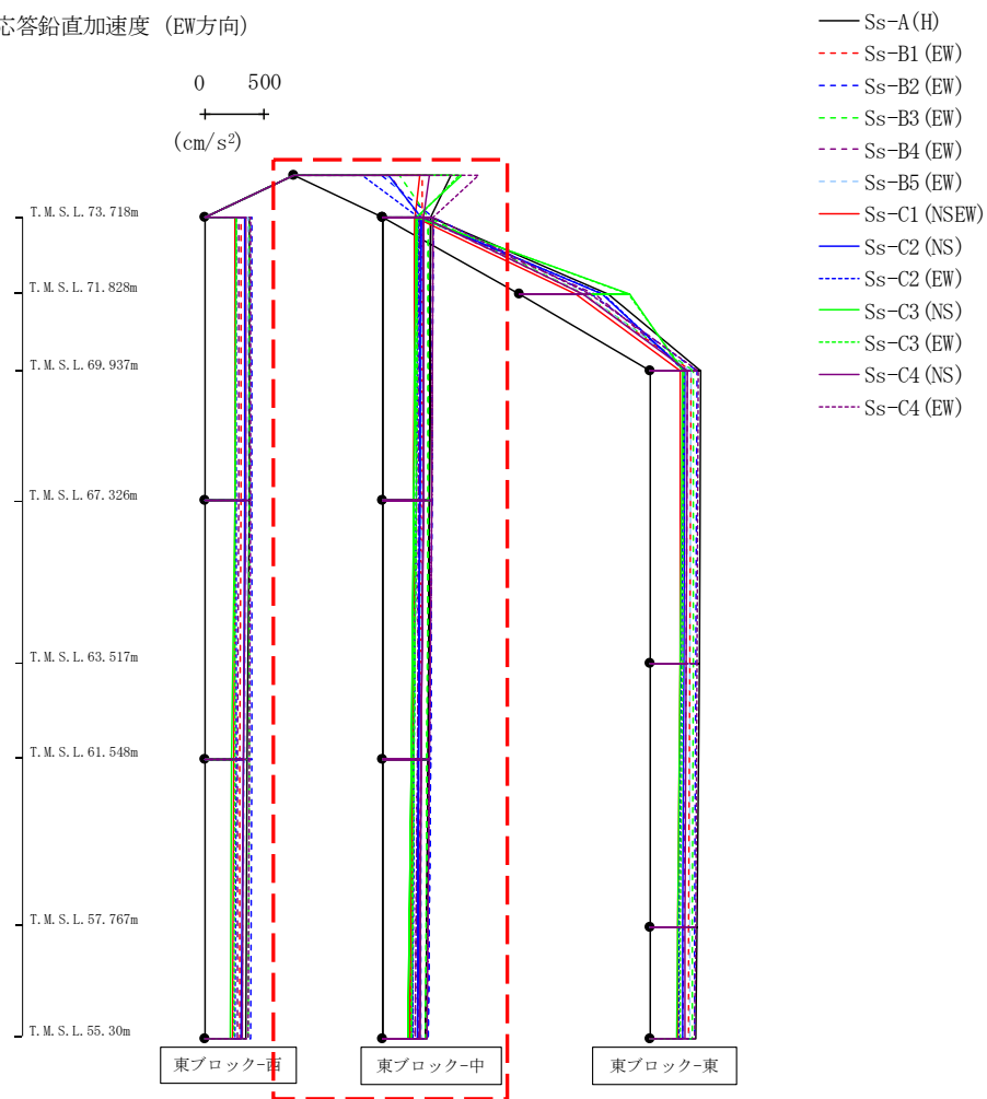
第4.2.1-44図 支持架構の最大応答鉛直加速度(基本ケース, EW断面③, 有効応力解析)(2/3)
