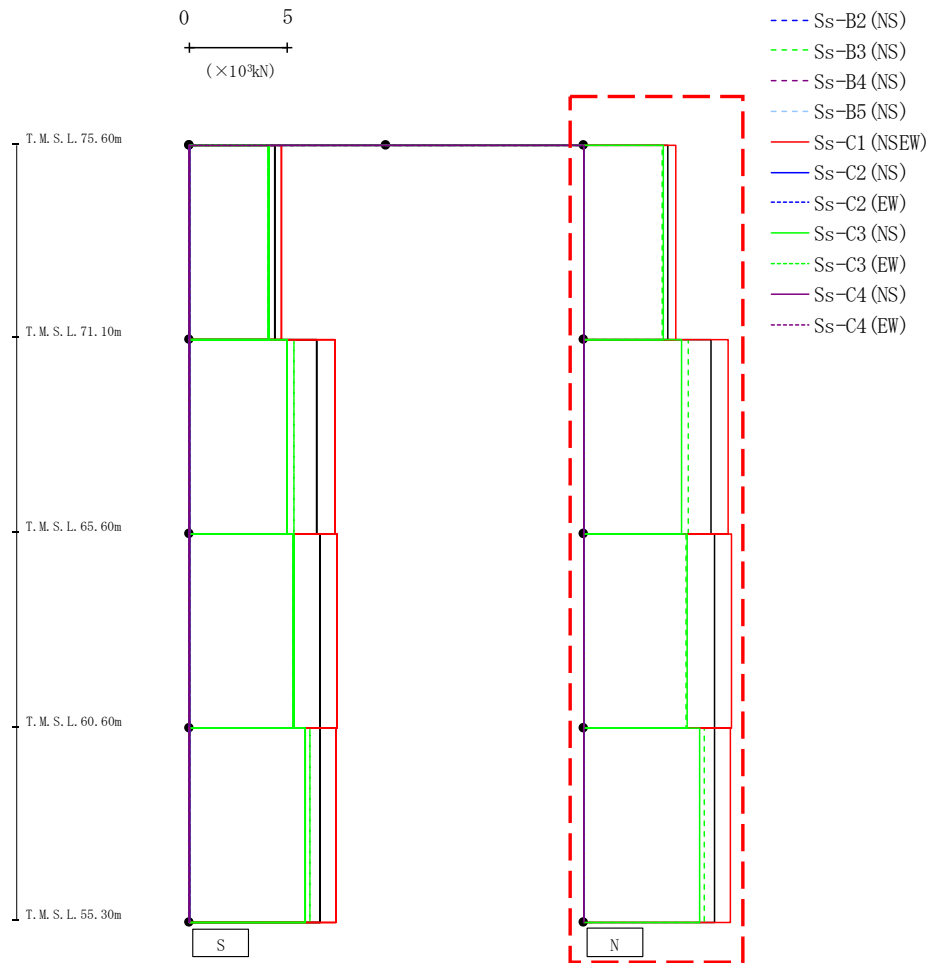
第4.2.2-38図 支持架構の最大応答せん断力(-1σ地盤, NS断面③, 有効応力解析) (2/2)
