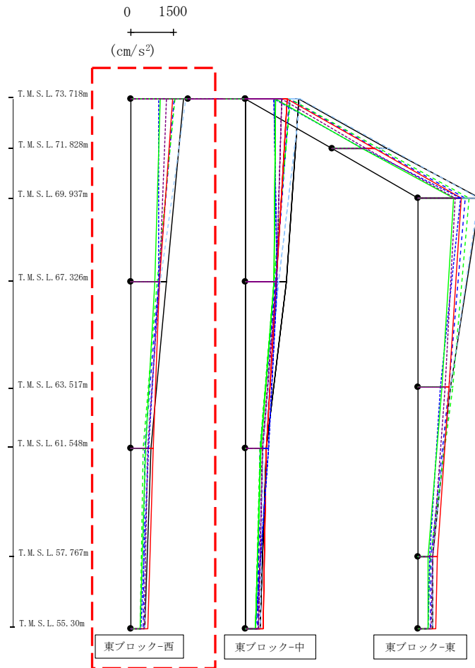
第4.2.1-53図 支持架構の最大応答加速度(+1σ地盤, EW断面③, 有効応力解析) (1/3)
