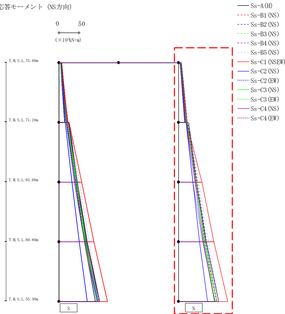
第4.2.1-3図 支持架構の最大応答曲げモーメント(基本ケース, NS断面①, 全応力解析) (2/2)
