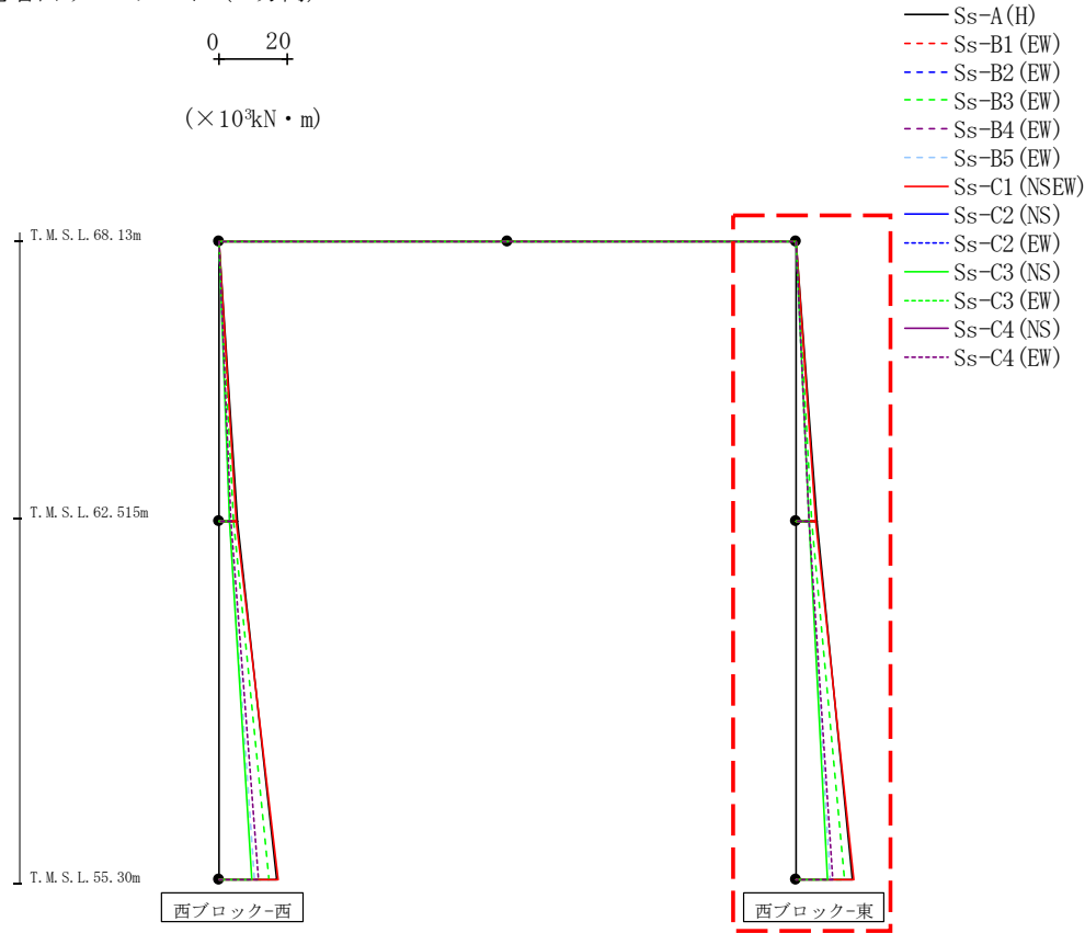
第4.2.2-23図 支持架構の最大応答曲げモーメント(+1 \sigma 地盤, EW断面④, 全応力解析) (2/2)
