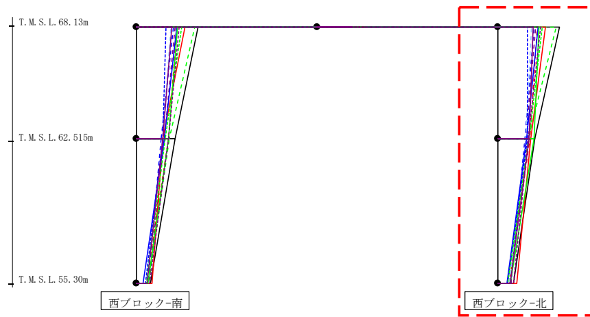
第4.2.2-37図 支持架構の最大応答加速度 (基本ケース, NS断面①, 有効応力解析) (2/2)
