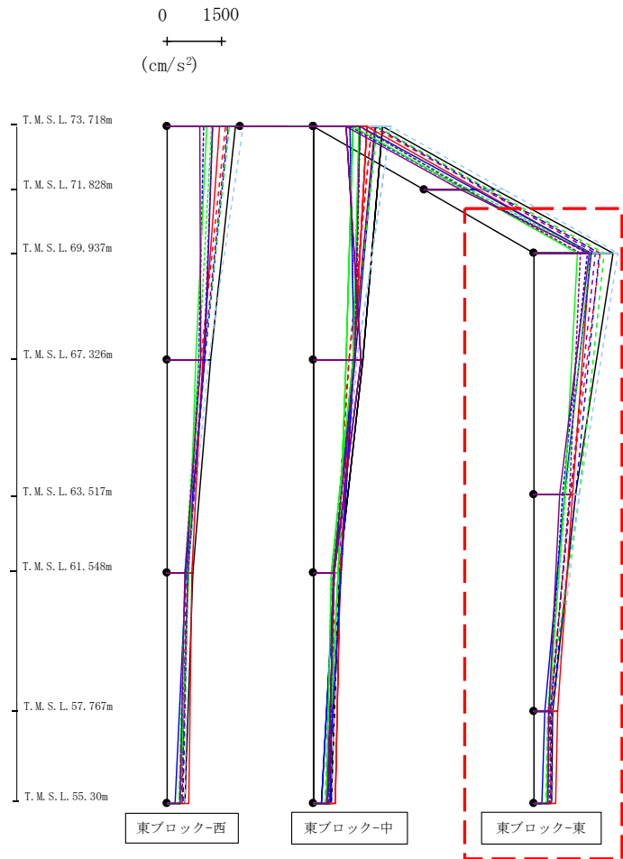
第4.2.1-5図 支持架構の最大応答加速度(基本ケース, EW断面③, 全応力解析) (3/3)
