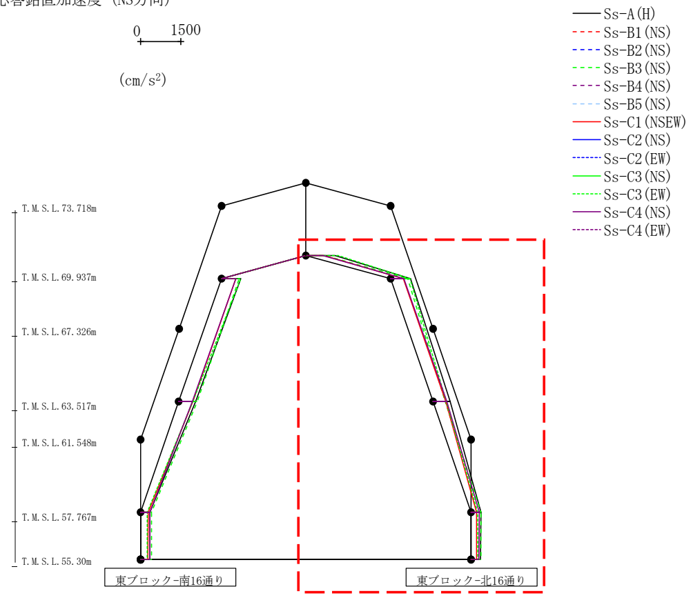
第4.2.1-28図 支持架構の最大応答鉛直加速度(-1σ地盤, NS断面②, 全応力解析) (4/4)
