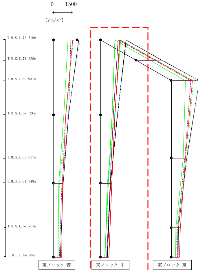
第4.2.1-21図 支持架構の最大応答加速度(+1σ地盤, EW断面④, 全応力解析) (2/3)
