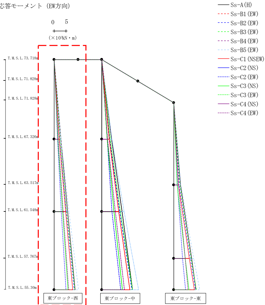
第4.2.1-55図 支持架構の最大応答曲げモーメント(+1σ地盤, EW断面③, 有効応力解析)(1/3)
