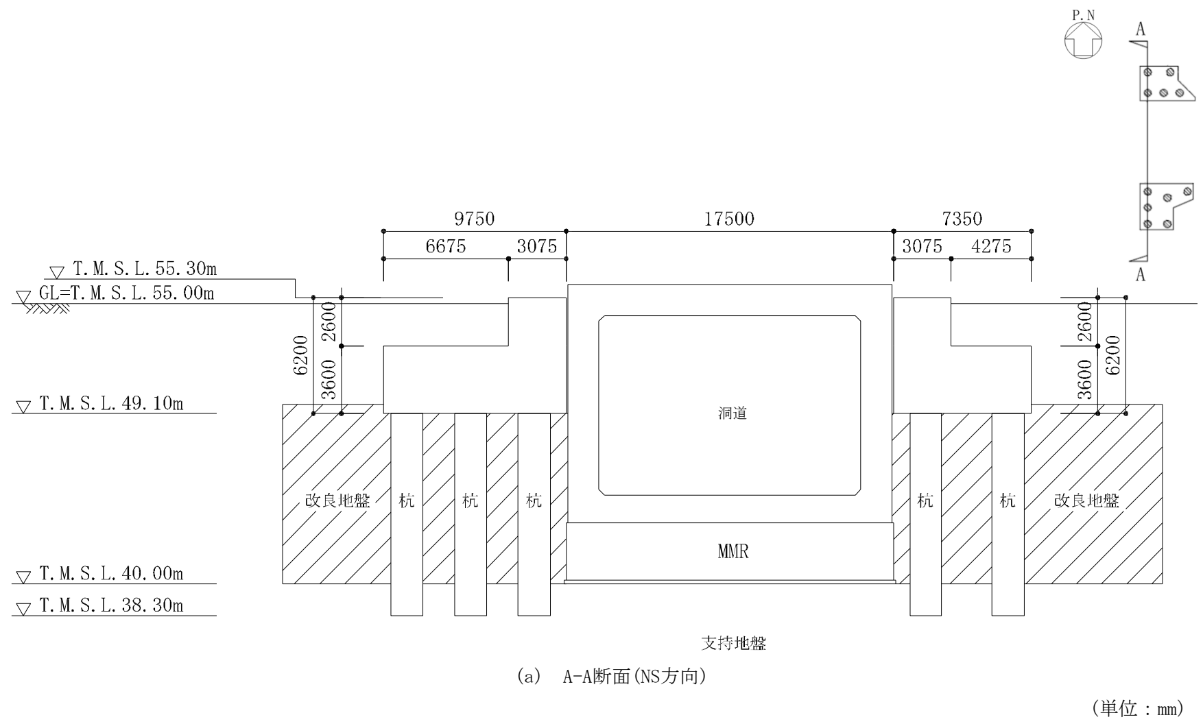
第2.2-8図 A1(西)防護板架構の基礎及び杭の断面図(1/2)
