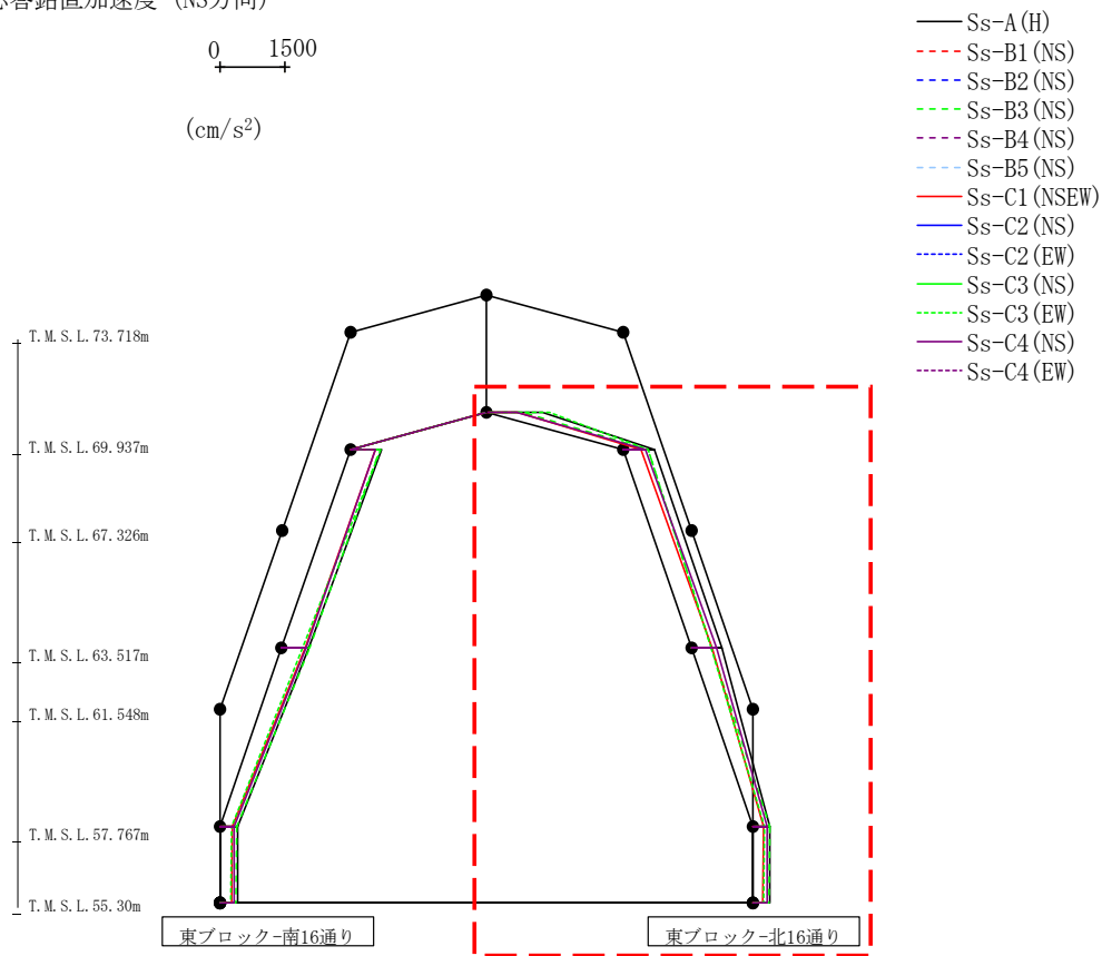
第4.2.1-52図 支持架構の最大応答鉛直加速度(+1σ地盤, NS断面②, 有効応力解析)(4/4)
