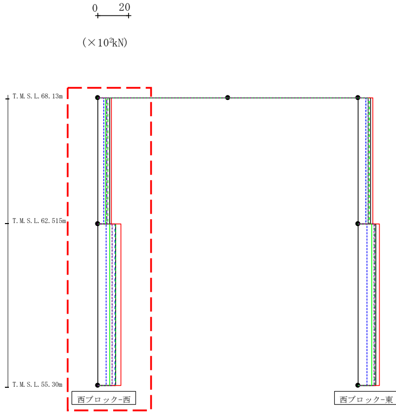
第4.2.2-54図 支持架構の最大応答せん断力(+1σ地盤, EW断面③, 有効応力解析) (1/2)
