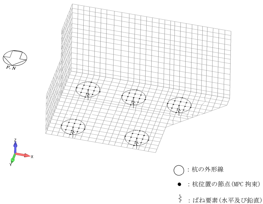
(b) 鳥瞰図(底面)
