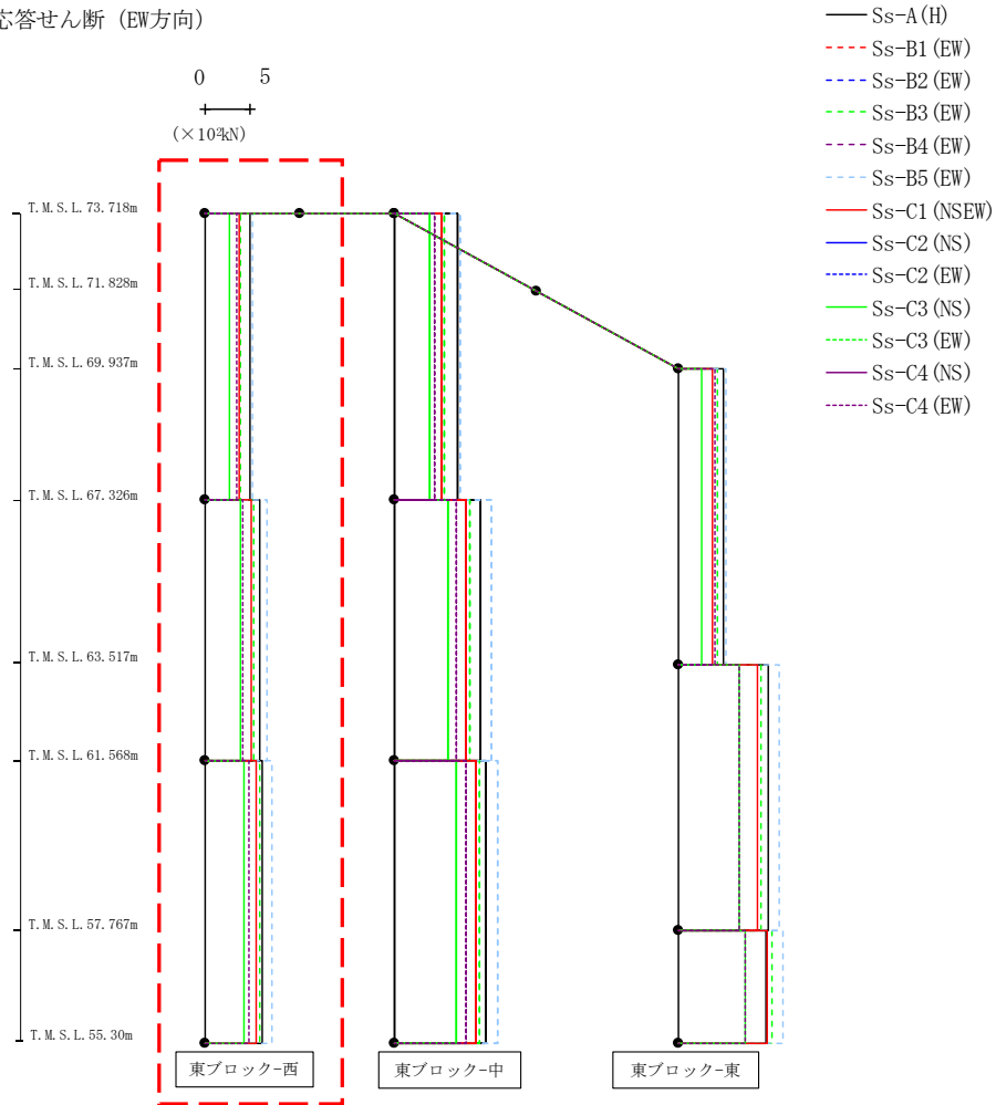
第4.2.1-22図 支持架構の最大応答せん断力(+1σ地盤, EW断面④, 全応力解析) (1/3)
