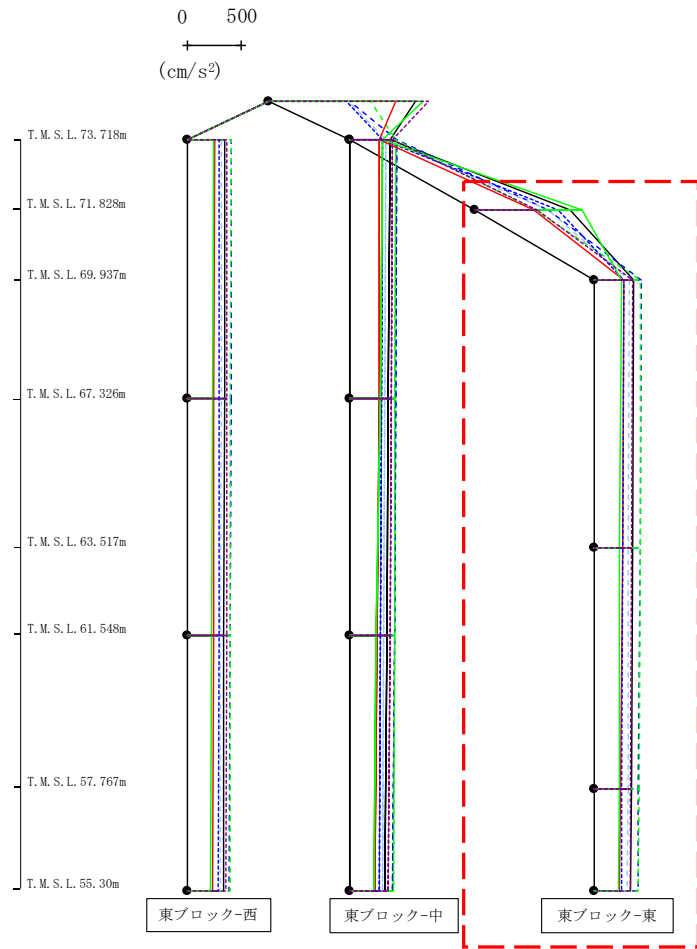
第4.2.1-56図 支持架構の最大応答鉛直加速度(+1σ地盤, EW断面③, 有効応力解析) (3/3)
