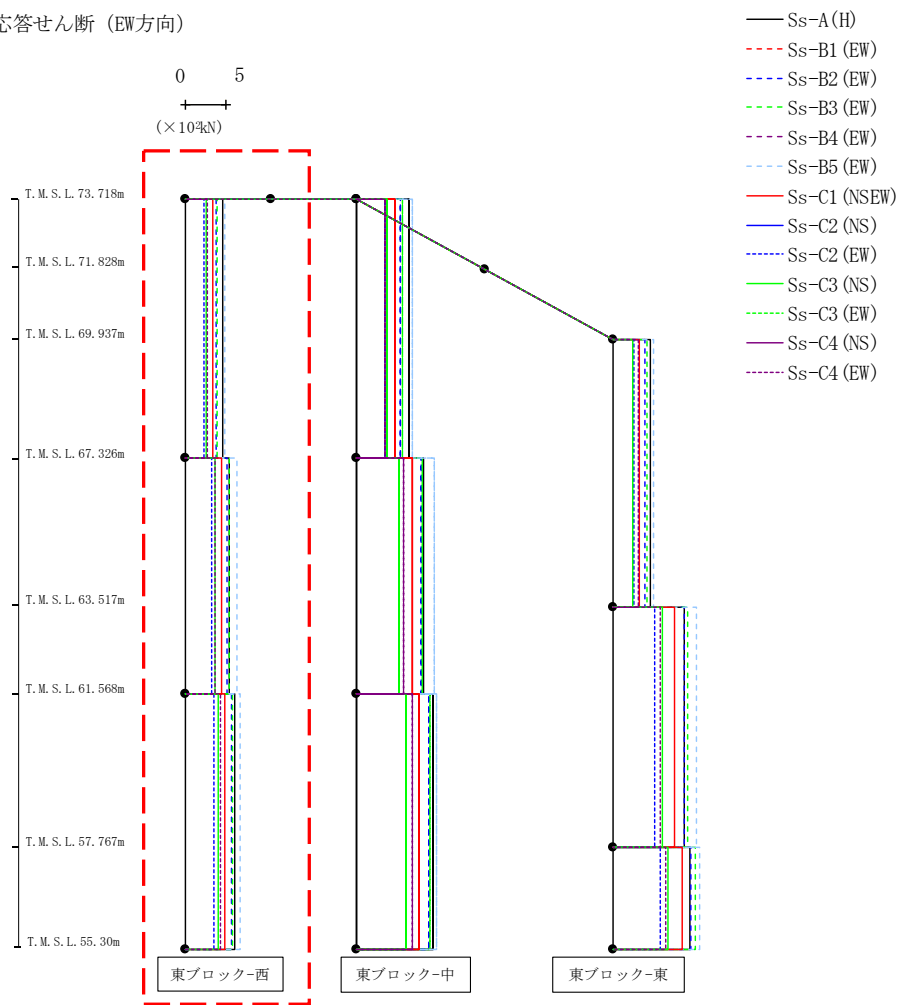
第4.2.1-66図 支持架構の最大応答せん断力(-1σ地盤, EW断面③, 有効応力解析) (1/3)
