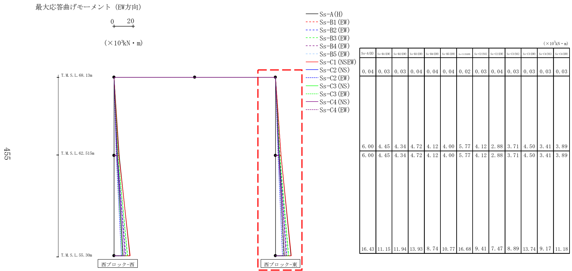
第4.2.2-47図 支持架構の最大応答曲げモーメント(基本ケース, EW断面④, 有効応力解析) (2/2)
