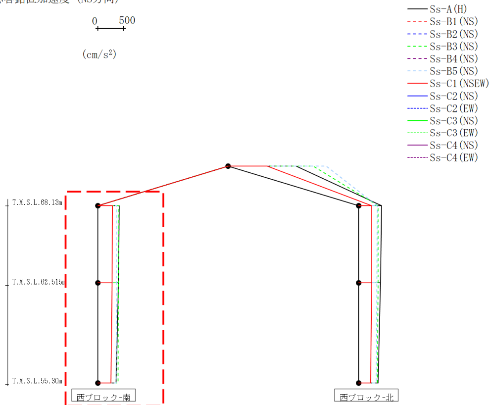
第4.2.2-64図 支持架構の最大応答鉛直加速度(-1σ地盤, NS断面①, 有効応力解析)(1/2)
