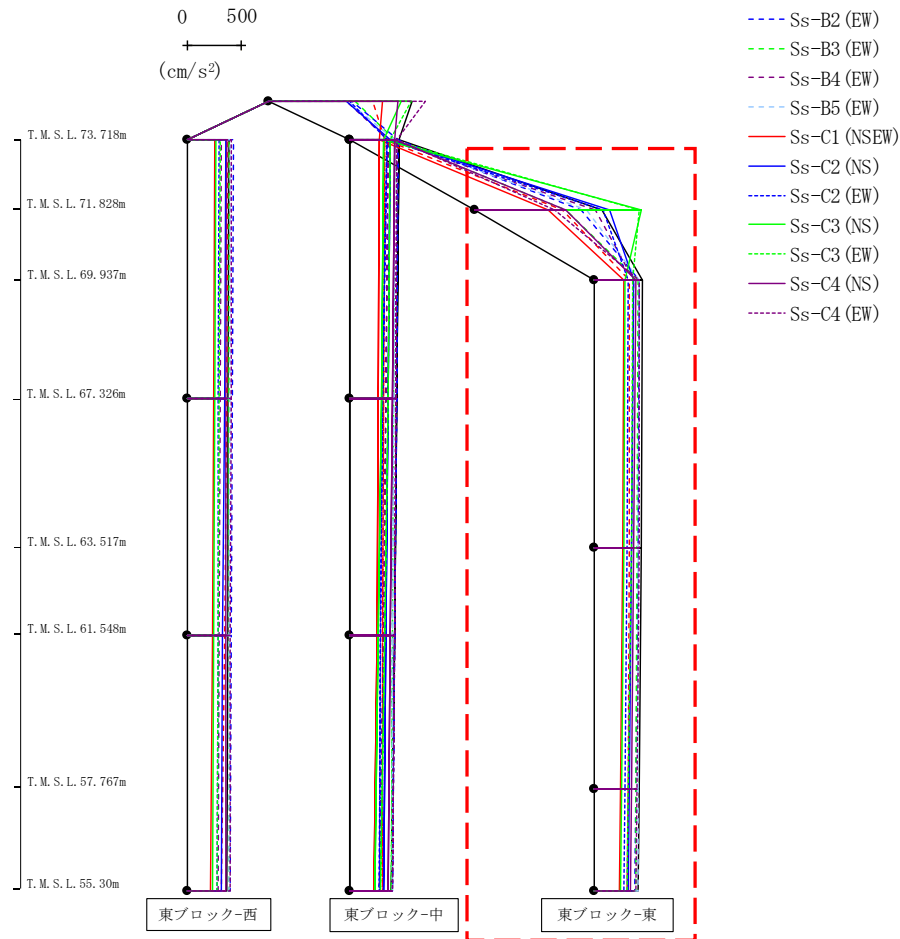
第4.2.1-48図 支持架構の最大応答鉛直加速度(基本ケース, EW断面④, 有効応力解析)(3/3)
