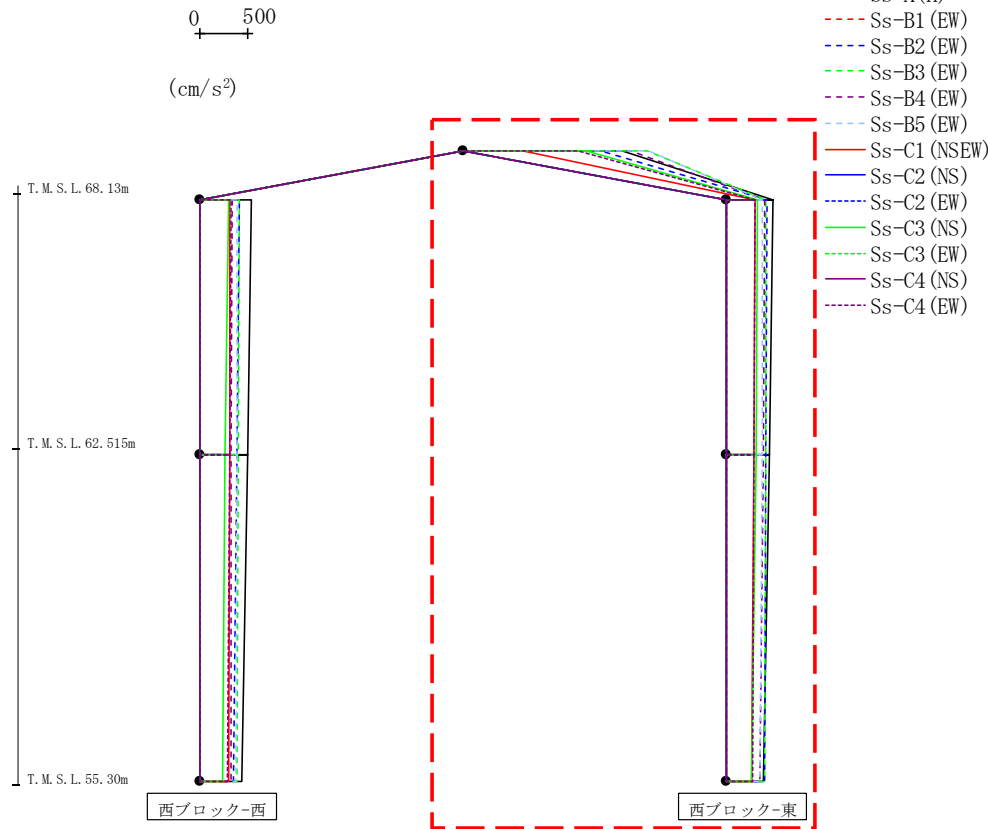
第4.2.2-72図 支持架構の最大応答鉛直加速度(-1σ地盤, EW断面④, 有効応力解析) (2/2)
