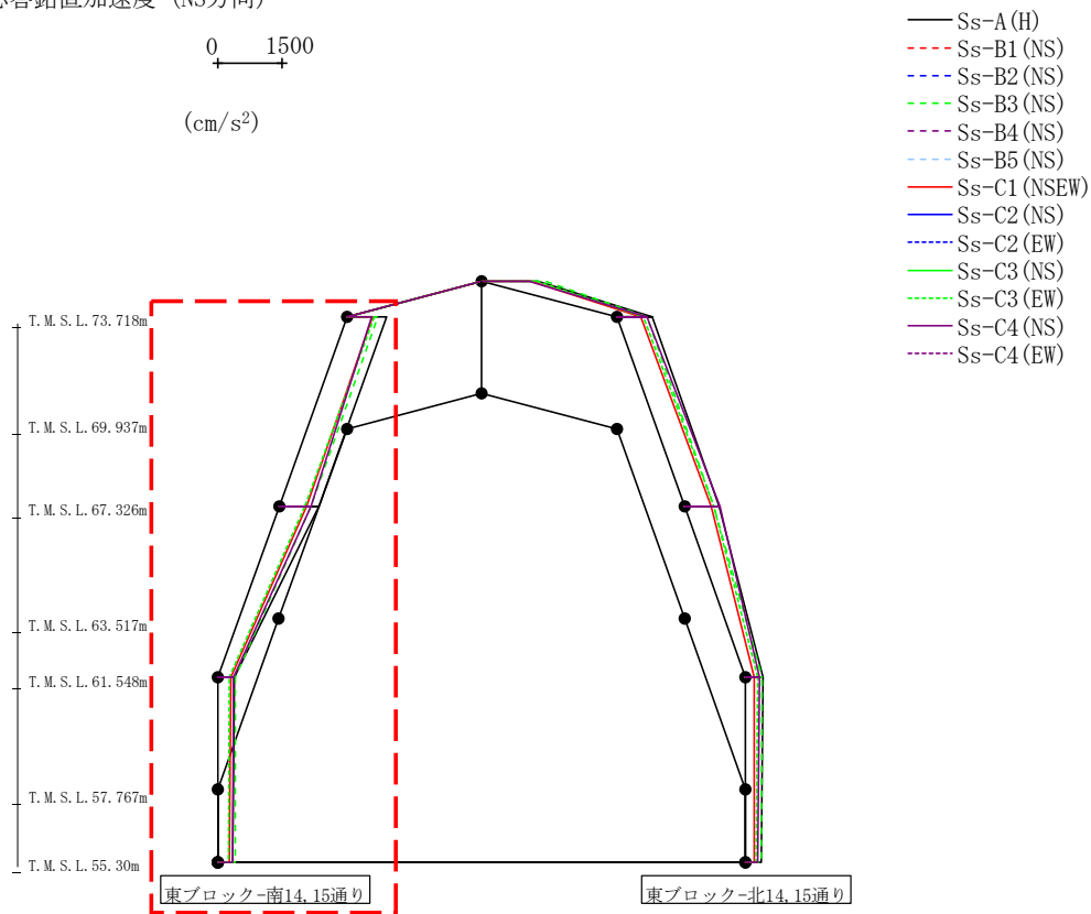
第4.2.1-64図 支持架構の最大応答鉛直加速度(-1σ地盤, NS断面②, 有効応力解析)(1/4)
