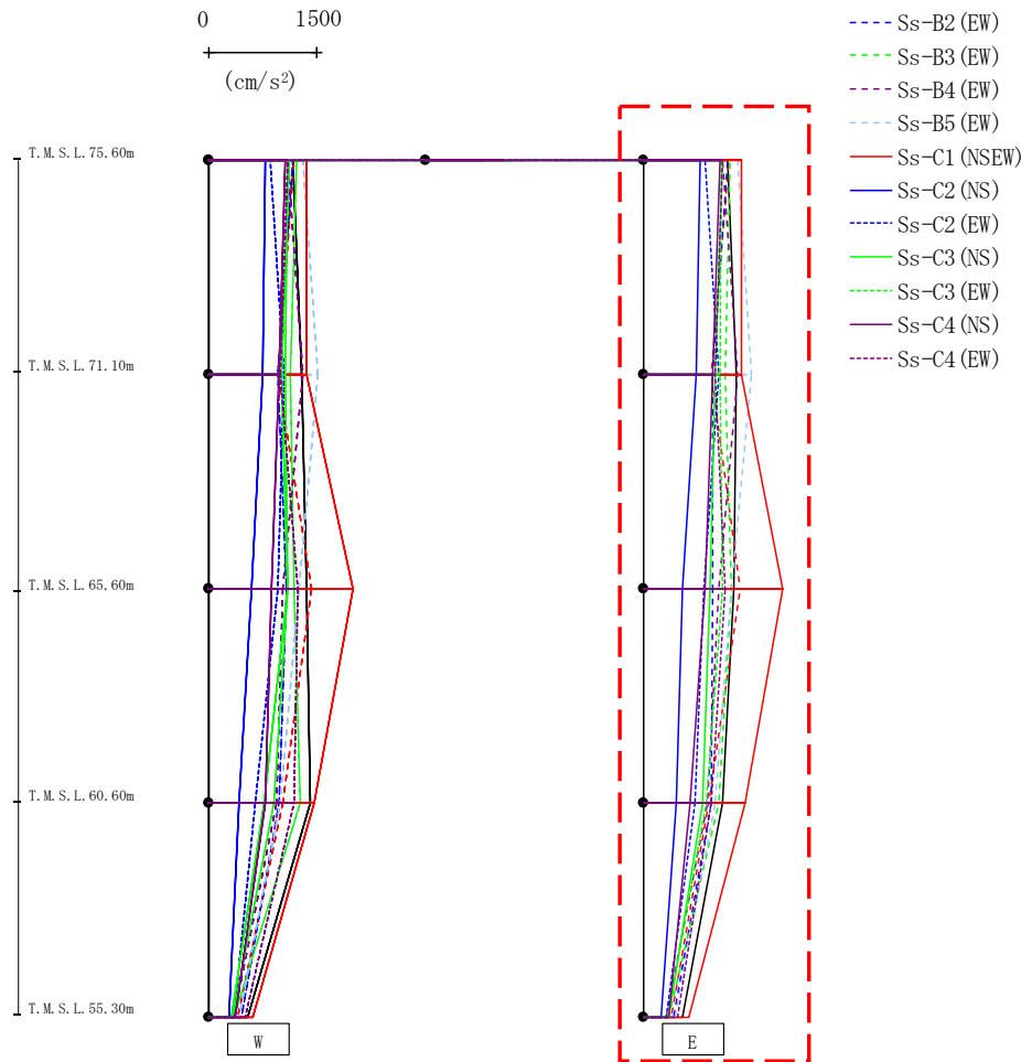
第4.2.2-9図 支持架構の最大応答加速度(基本ケース, EW断面①, 有効応力解析)(2/2)
