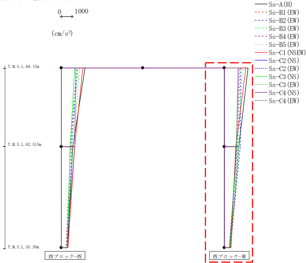
第4.2.2-69図 支持架構の最大応答加速度(-1σ地盤, EW断面④, 有効応力解析)(2/2)
