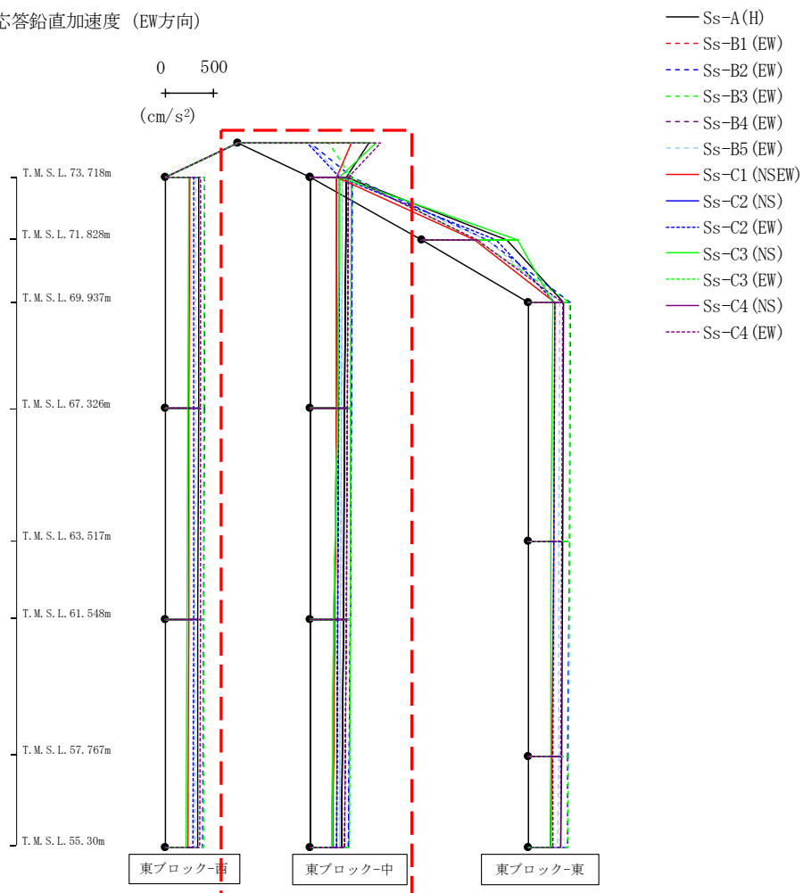
第4.2.1-56図 支持架構の最大応答鉛直加速度(+1σ地盤, EW断面③, 有効応力解析) (2/3)
