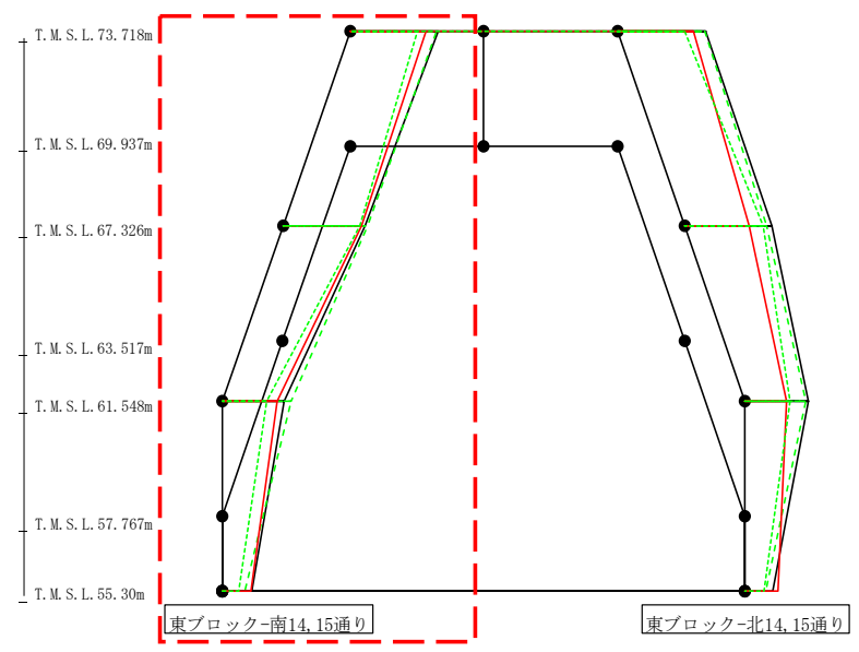
第4.2.1-13図 支持架構の最大応答加速度(+1σ地盤, NS断面②, 全応力解析) (1/4)
