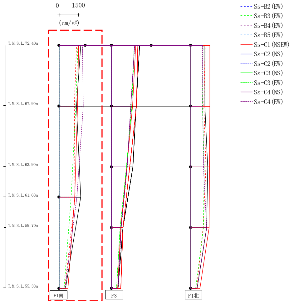
第4.2.2-29図 支持架構の最大応答加速度(G10B防護ネット架構, -1σ地盤, EW断面①)(1/3)
