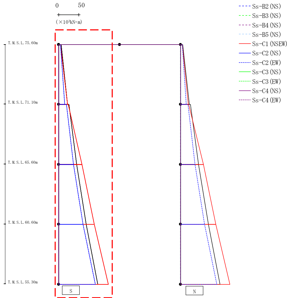
第4.2.1-19図 支持架構の最大応答曲げモーメント(+1σ地盤, NS断面①, 全応力解析)(1/2)
