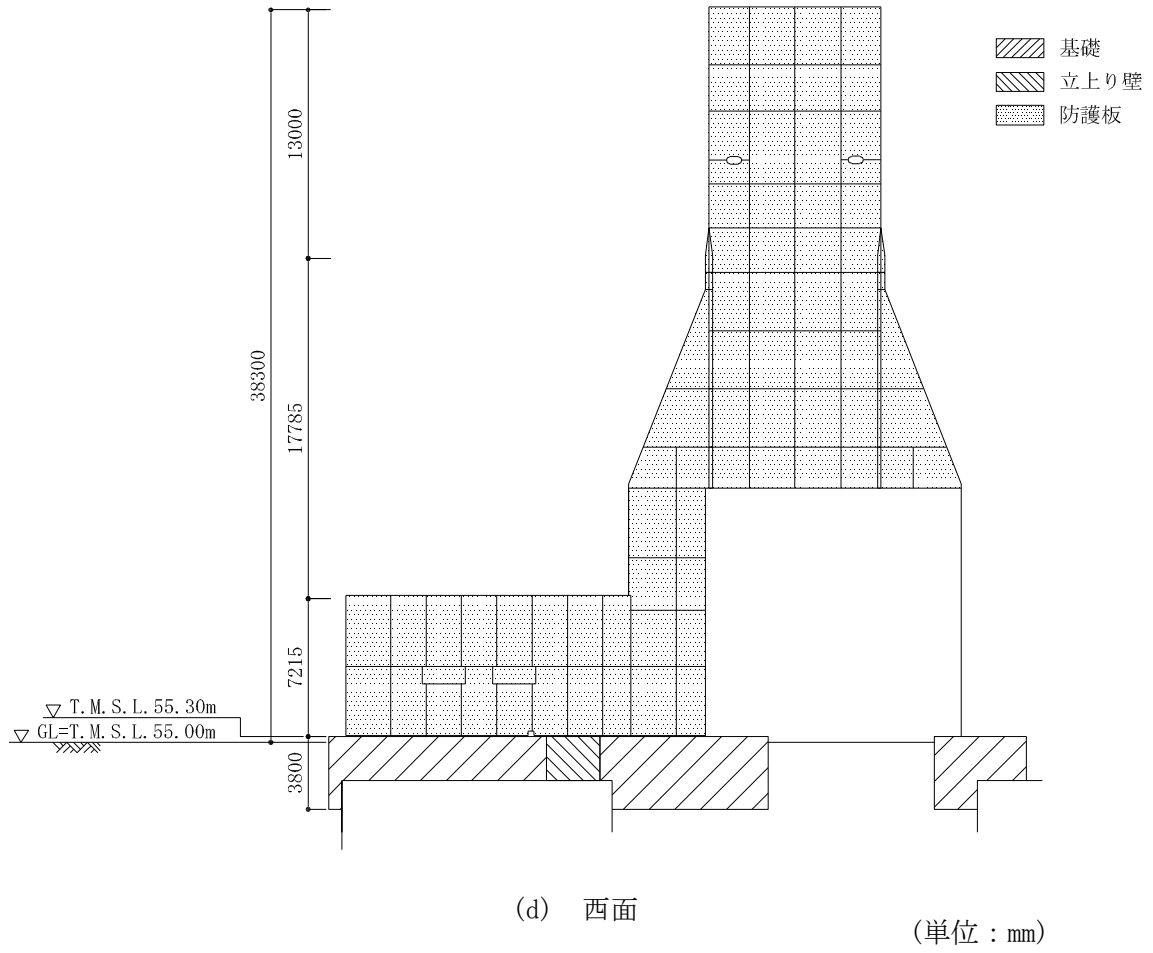
第2.2-4図 飛来物防護板架構の概略側面図(4/4)
