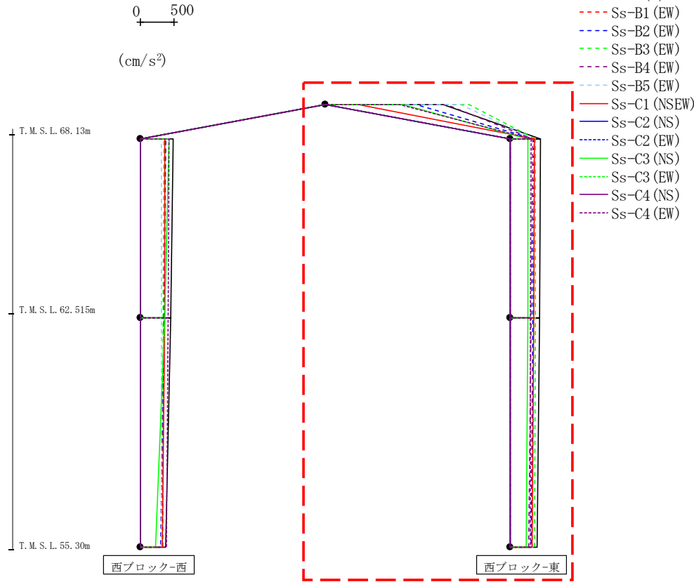
第4.2.2-60図 支持架構の最大応答鉛直加速度(+1σ地盤, EW断面④, 有効応力解析)(2/2)
