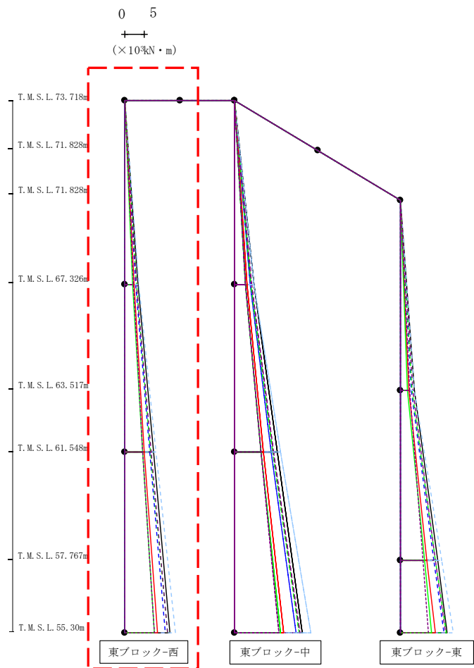
第4.2.1-71図 支持架構の最大応答曲げモーメント(-1σ地盤, EW断面④, 有効応力解析)(1/3)
