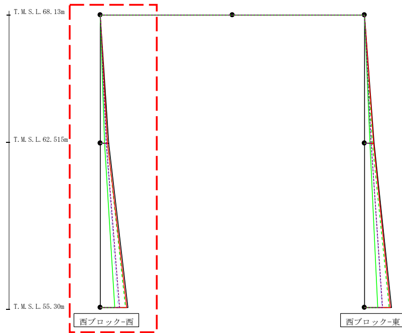
第4.2.2-35図 支持架構の最大応答曲げモーメント(-1σ地盤, EW断面④, 全応力解析)(1/2)
