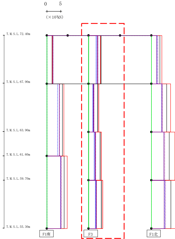
第4.2.2-34図 支持架構の最大応答せん断力(G10B防護ネット架構, -1σ地盤, EW断面②) (2/3)
