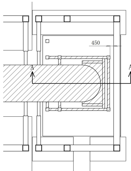
(平面)
