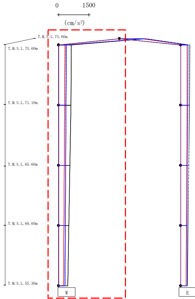
第4.2.1-48図 支持架構の最大応答鉛直加速度(-1σ地盤, EW断面③, 全応力解析) (1/2)
