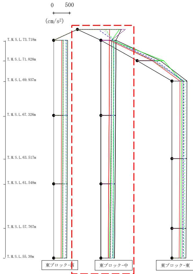
第4.2.1-32図 支持架構の最大応答鉛直加速度(-1σ地盤, EW断面③, 全応力解析) (2/3)
