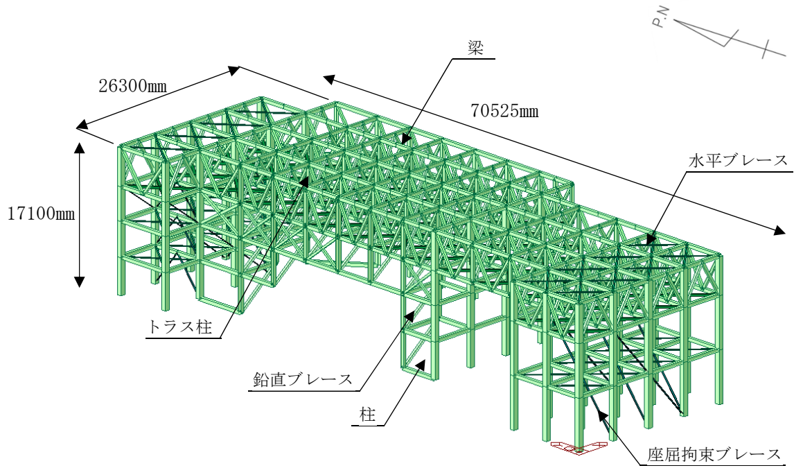
第2.2-6図 支持架構の全景(G10B防護ネット)
