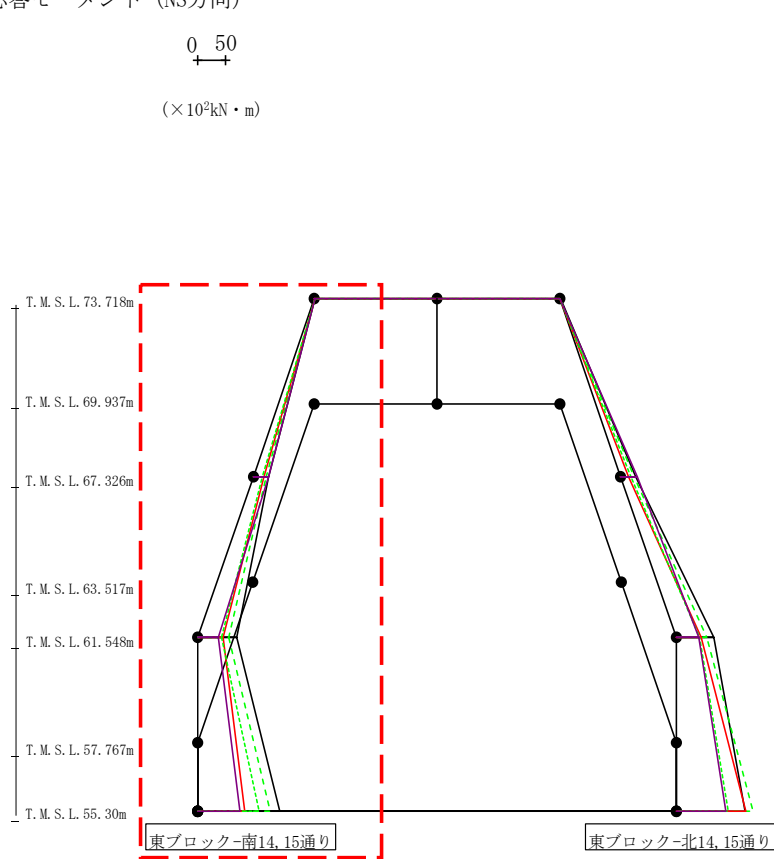
第4.2.1-51図 支持架構の最大応答曲げモーメント(+1σ地盤, NS断面②, 有効応力解析) (1/4)
