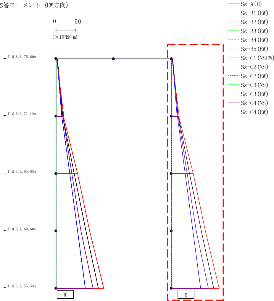
第4.2.2-31図 支持架構の最大応答曲げモーメント(+1σ地盤, EW断面③, 有効応力解析)(2/2)
