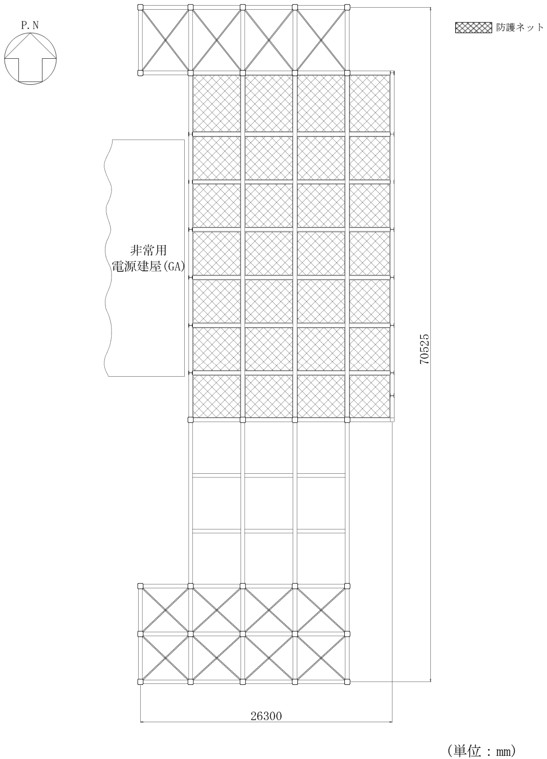
第2.2-7図 G10B防護ネット架構の屋根伏図
