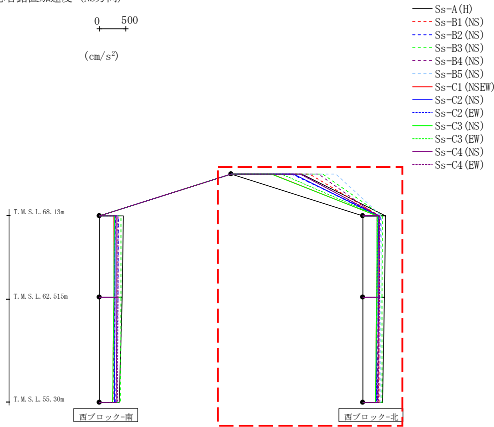
第4.2.2-4図 支持架構の最大応答鉛直加速度(基本ケース, NS断面①, 全応力解析) (2/2)
