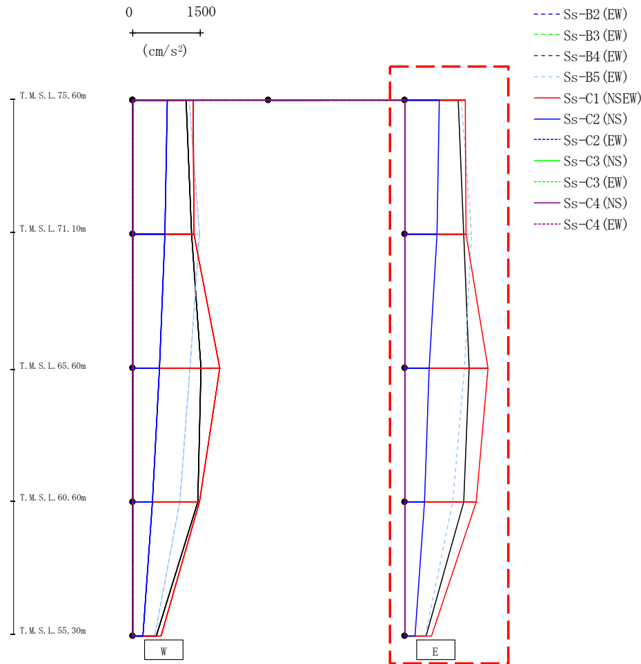
第4.2.2-41図 支持架構の最大応答加速度(-1σ地盤, EW断面①, 有効応力解析)(2/2)
