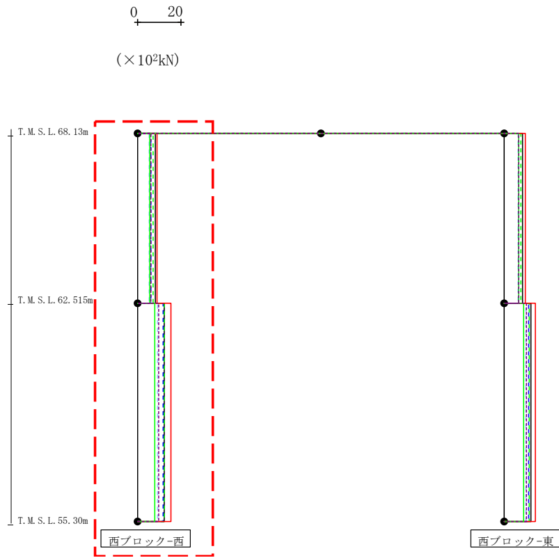
第4.2.2-18図 支持架構の最大応答せん断力(+1σ地盤, EW断面③, 全応力解析) (1/2)
