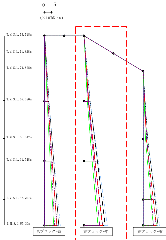
第4.2.1-59図 支持架構の最大応答曲げモーメント(+1σ地盤, EW断面④, 有効応力解析) (2/3)
