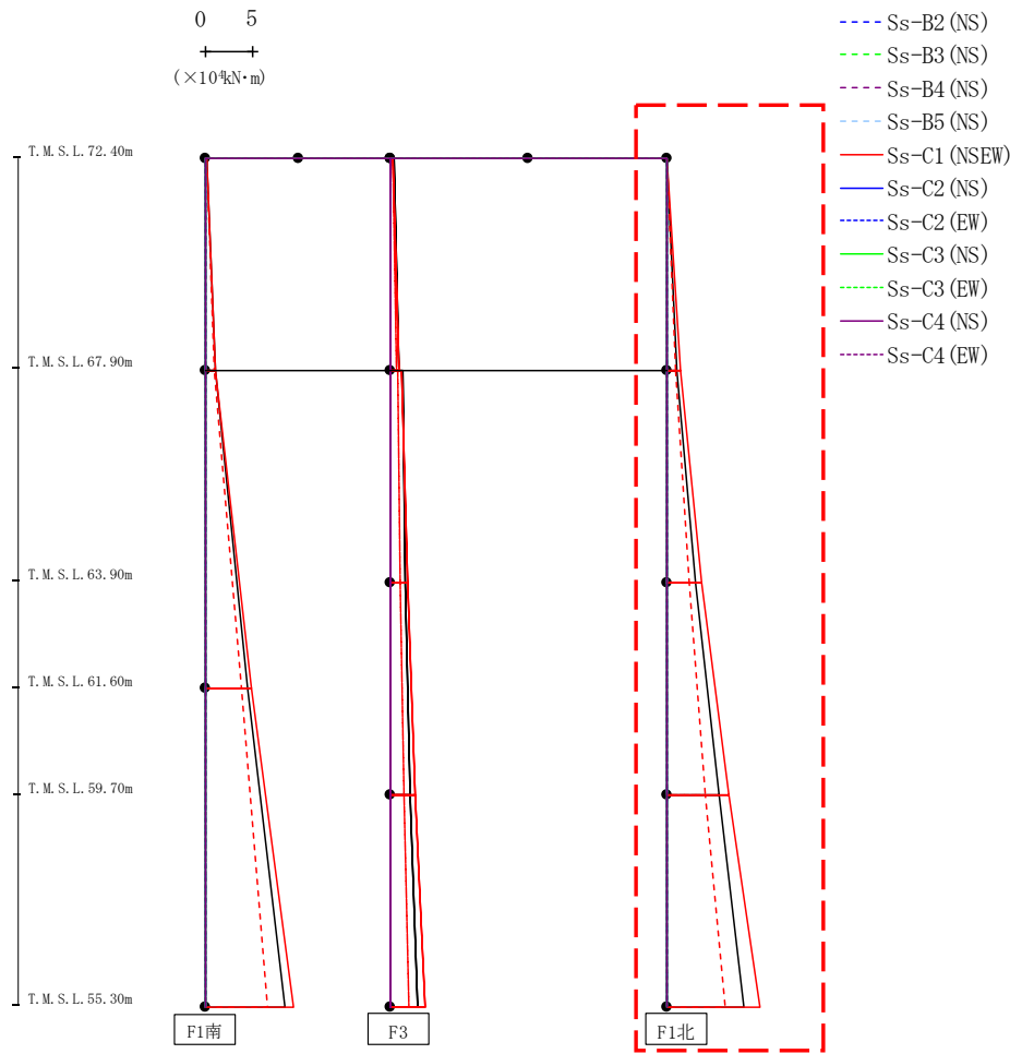
第4.2.1-15図 支持架構の最大応答曲げモーメント(G10A防護ネット架構, +1σ地盤, NS断面①) (3/3)
