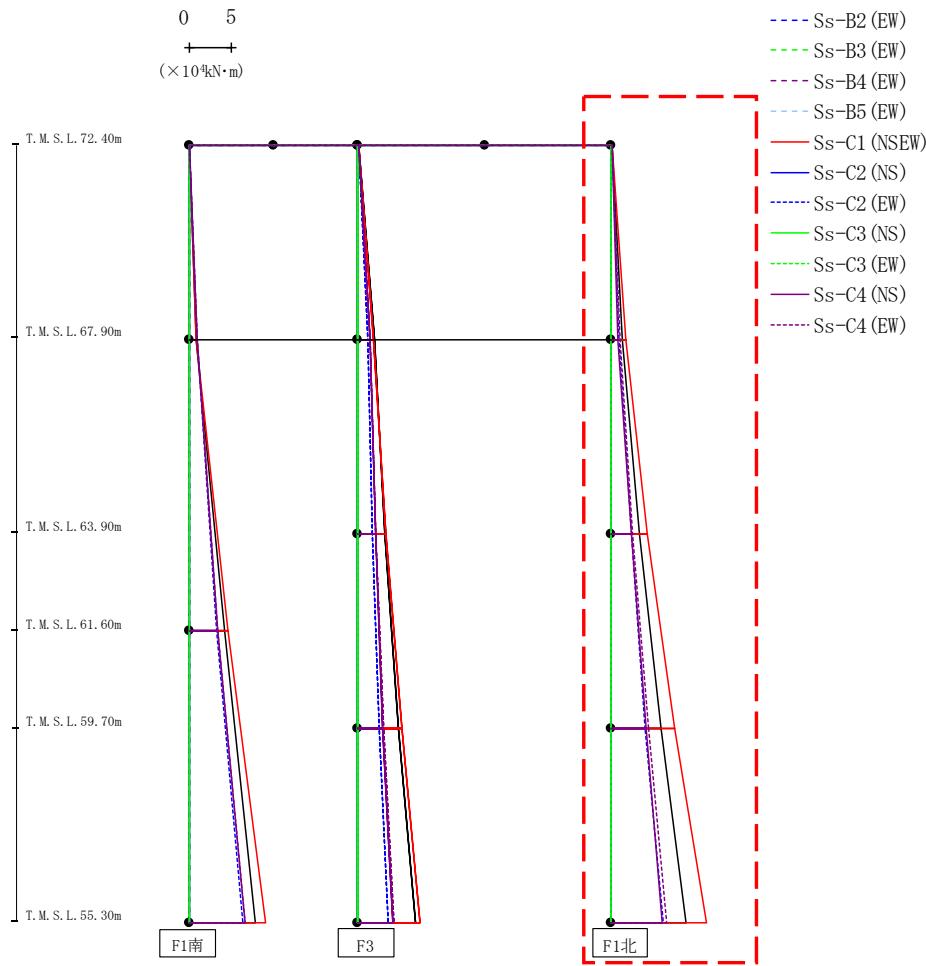
第4.2.2-35図 支持架構の最大応答曲げモーメント (G10B防護ネット架構, -1σ地盤, EW断面②) (3/3)
