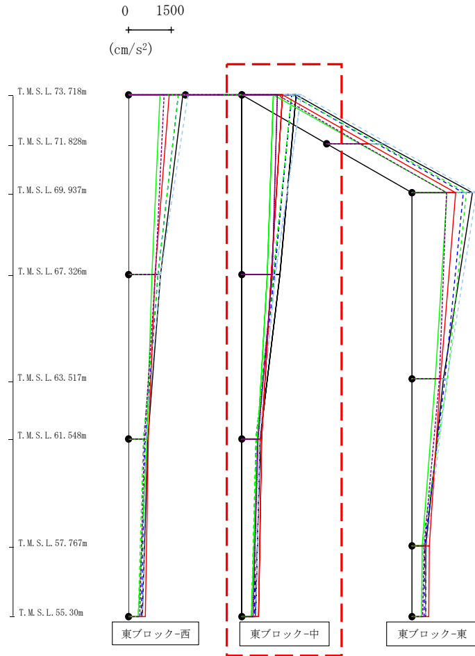
第4.2.1-29図 支持架構の最大応答加速度(-1σ地盤, EW断面③, 全応力解析) (2/3)
