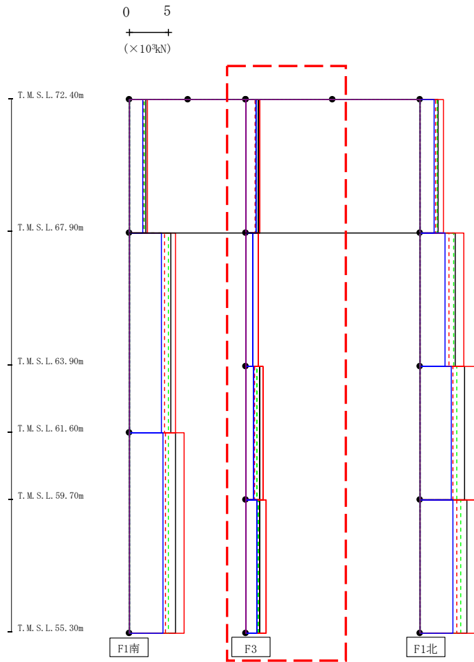
第4.2.2-14図 支持架構の最大応答せん断力(G10B防護ネット架構, +1σ地盤, NS断面②) (2/3)
