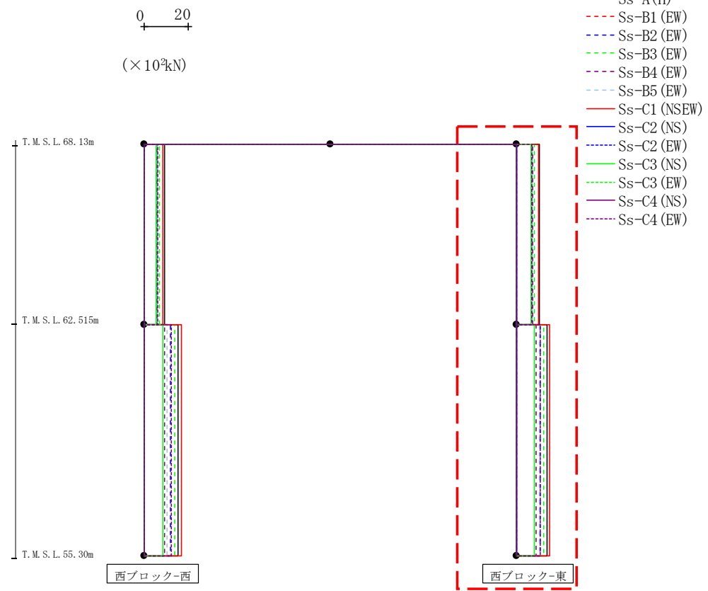
第4.2.2-58図 支持架構の最大応答せん断力(+1σ地盤, EW断面④, 有効応力解析) (2/2)
