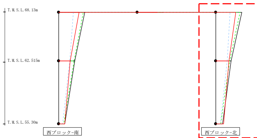
第4.2.2-49図 支持架構の最大応答加速度(+1σ地盤, NS断面①, 有効応力解析)(2/2)
