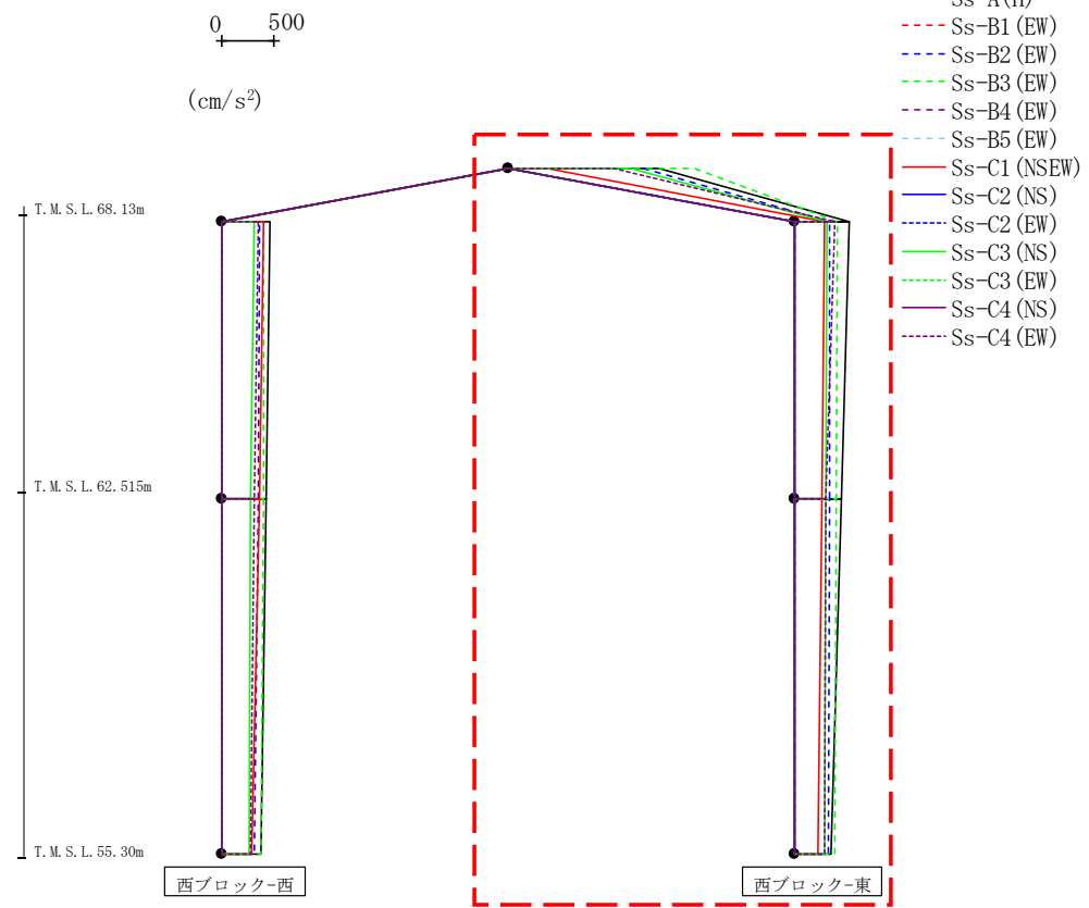
第4.2.2-44図 支持架構の最大応答鉛直加速度(基本ケース, EW断面③, 有効応力解析) (2/2)
