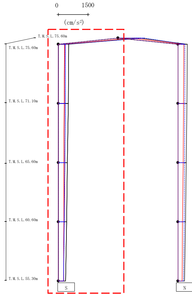
第4.2.2-20図 支持架構の最大応答鉛直加速度(+1σ地盤, NS断面①, 有効応力解析)(1/2)
