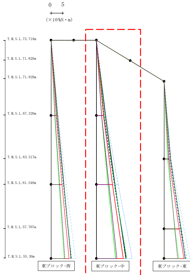
第4.2.2-19図 支持架構の最大応答曲げモーメント(+1σ地盤, EW断面③, 全応力解析) (2/3)
