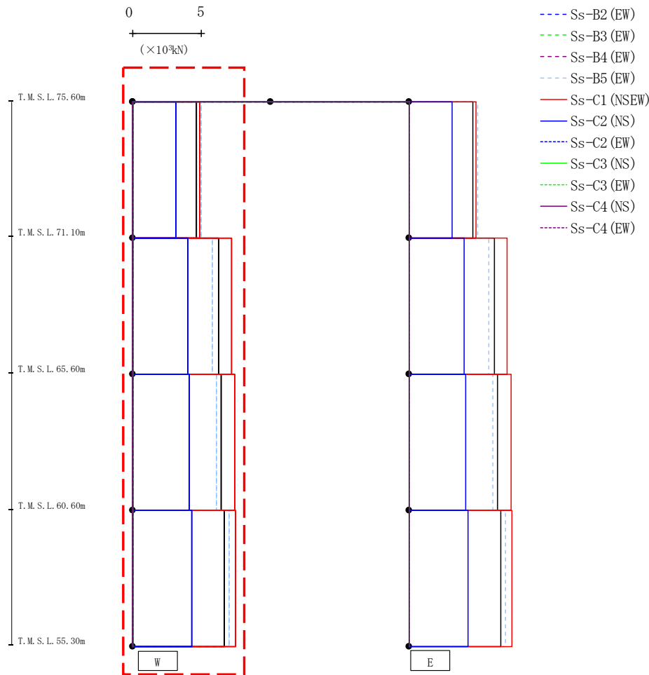
第4.2.1-46図 支持架構の最大応答せん断力(-1σ地盤, EW断面③, 全応力解析) (1/2)
