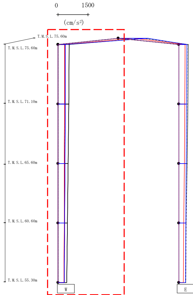
第4.2.2-28図 支持架構の最大応答鉛直加速度(+1σ地盤, EW断面①, 有効応力解析)(1/2)
