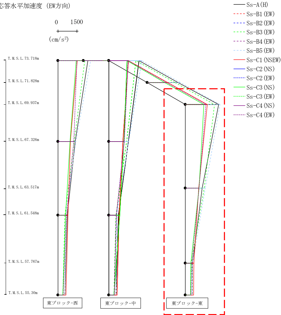
第4.2.1-33図 支持架構の最大応答加速度(-1σ地盤, EW断面④, 全応力解析) (3/3)
