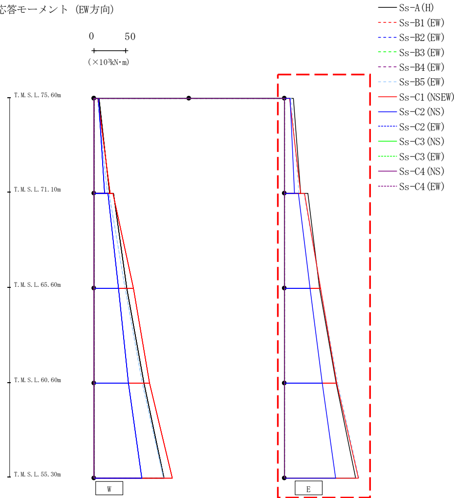
第4.2.2-43図 支持架構の最大応答曲げモーメント(-1σ地盤, EW断面①, 有効応力解析)(2/2)
