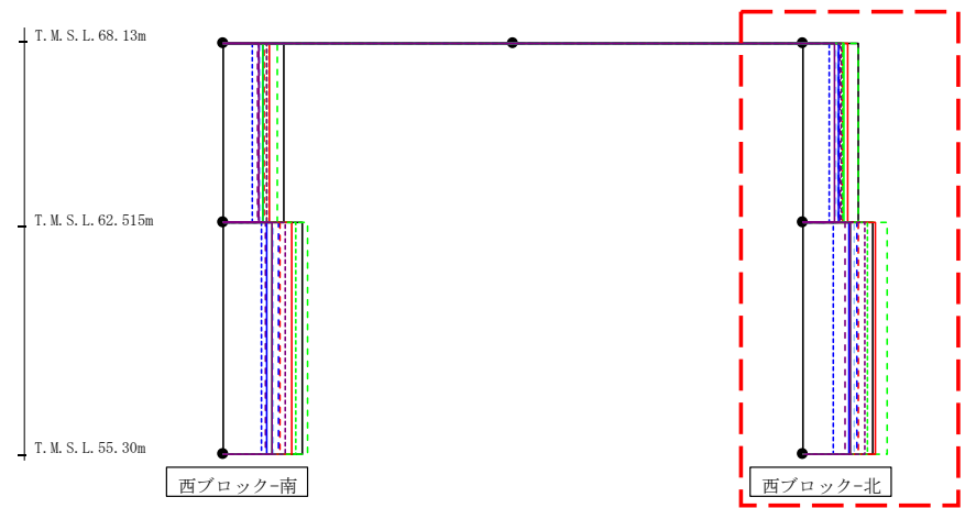
第4.2.2-38図 支持架構の最大応答せん断力(基本ケース, NS断面①, 有効応力解析)(2/2)
