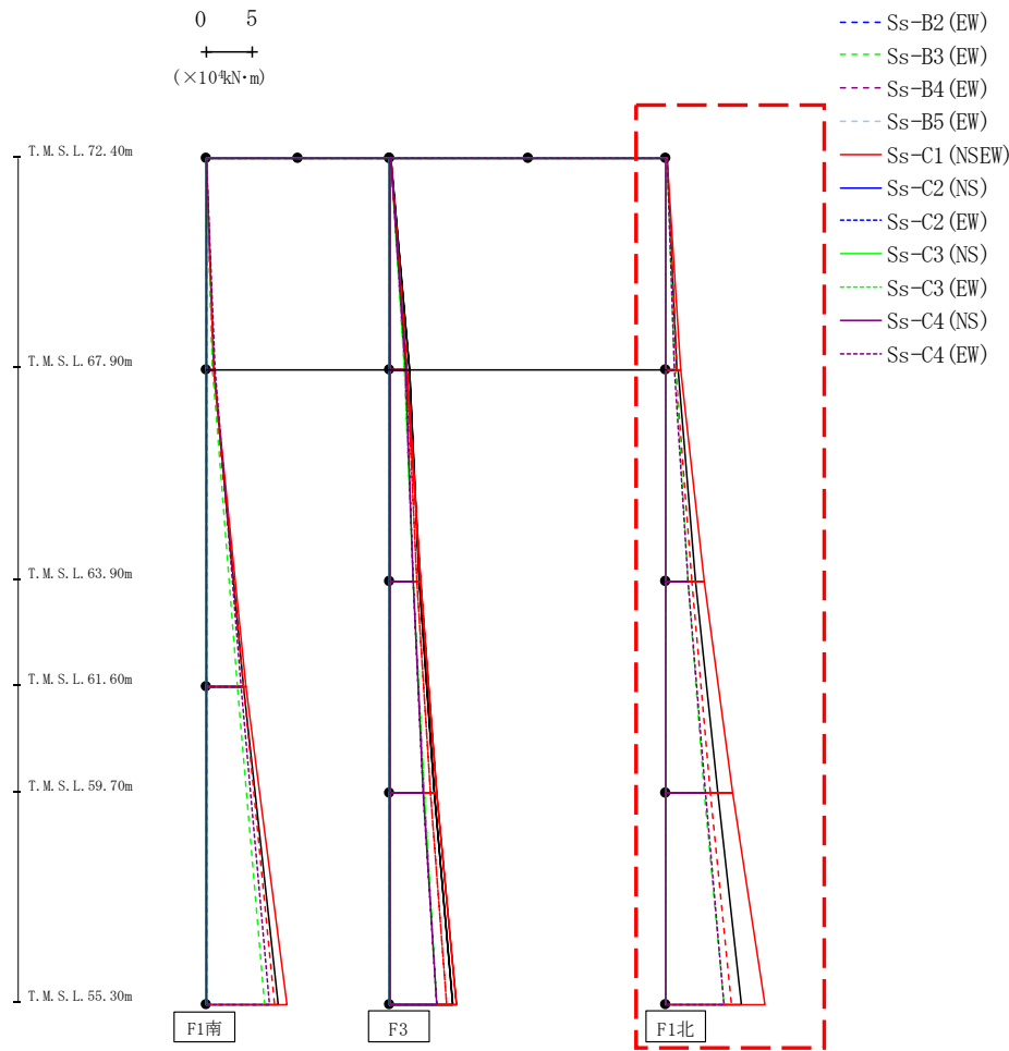
第4.2.1-23図 支持架構の最大応答曲げモーメント (G10A防護ネット架構, +1σ地盤, EW断面②) (3/3)
