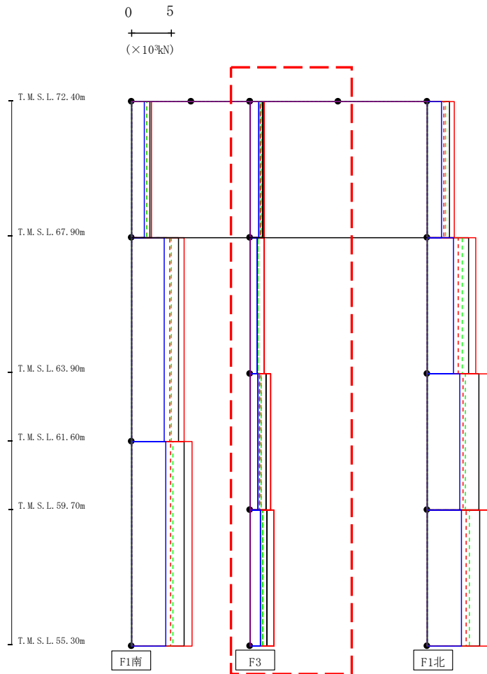
第4.2.2-26図 支持架構の最大応答せん断力(G10B防護ネット架構, -1σ地盤, NS断面②) (2/3)
