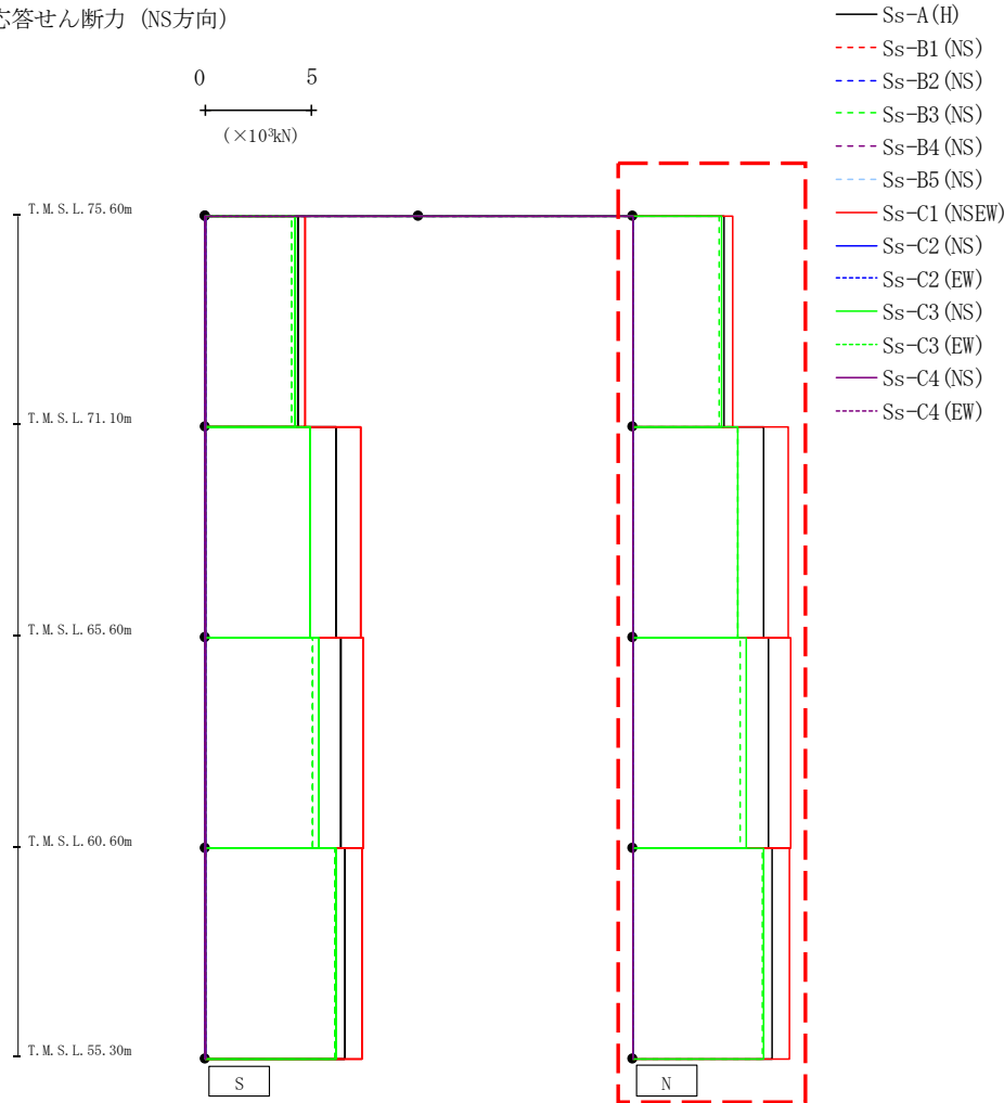
第4.2.1-38図 支持架構の最大応答せん断力(-1σ地盤, NS断面③, 全応力解析) (2/2)
