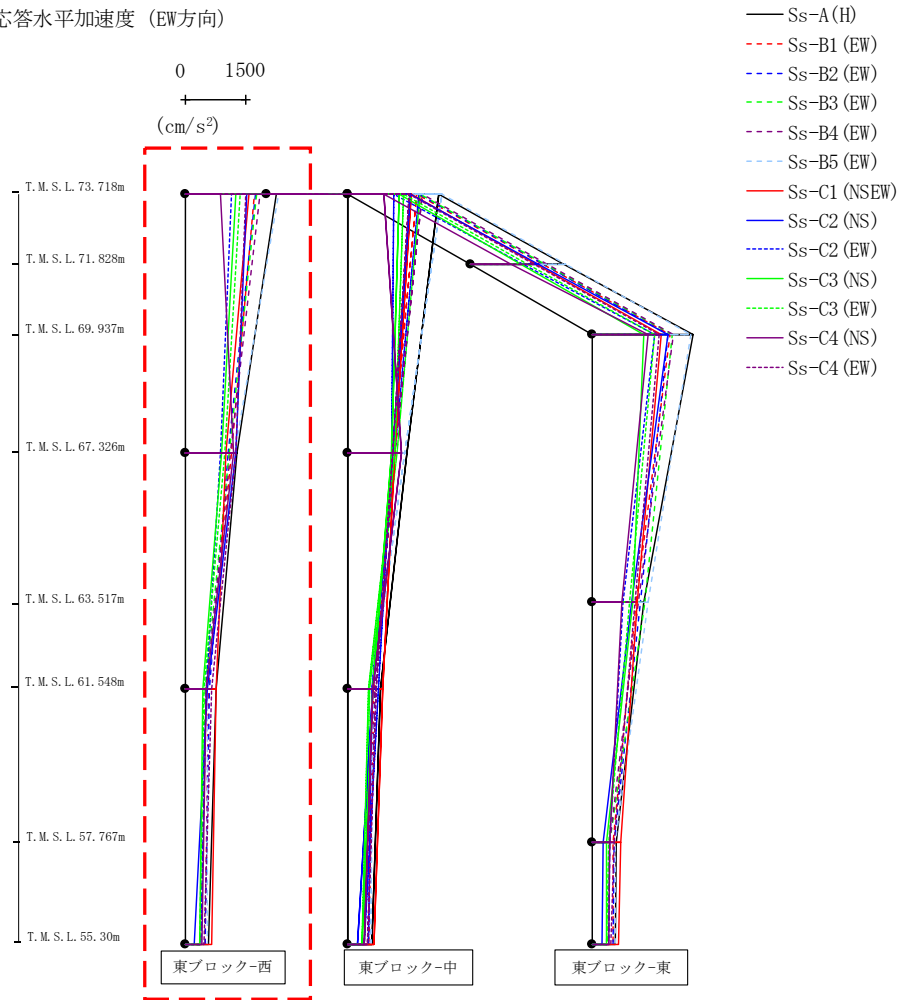
第4.2.1-45図 支持架構の最大応答加速度(基本ケース, EW断面④, 有効応力解析)(1/3)
