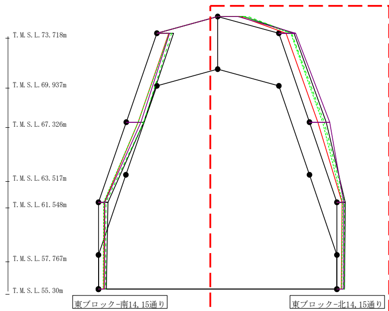
第4.2.1-52図 支持架構の最大応答鉛直加速度(+1σ地盤, NS断面②, 有効応力解析) (2/4)
