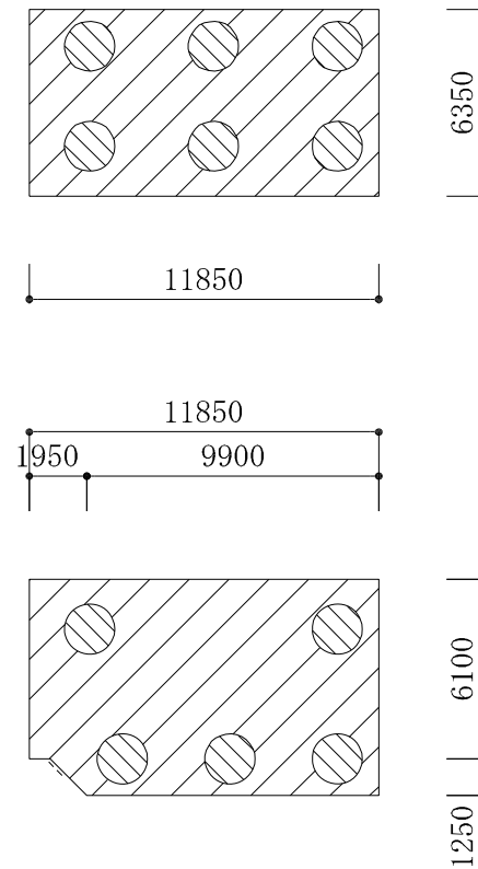
(b) 杭伏図
