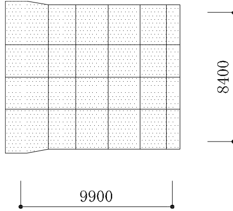
(a) 屋根伏図
