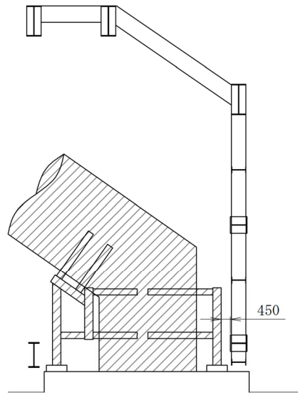
(A-A断面)
