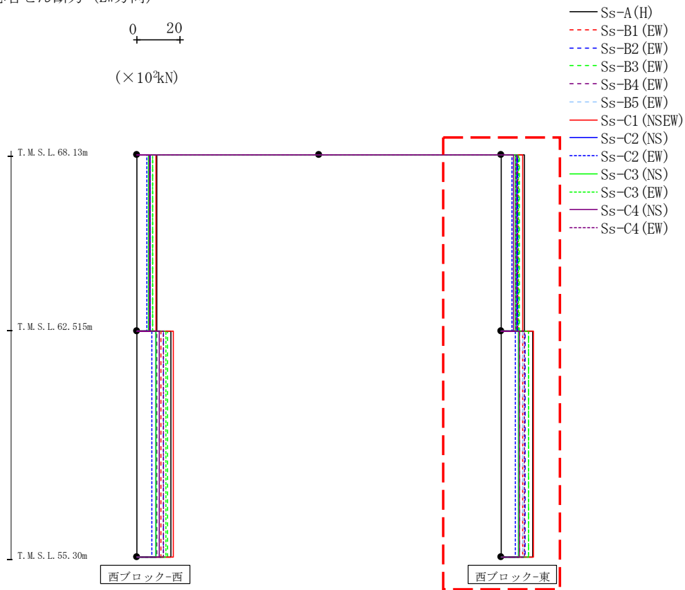
第4.2.2-46図 支持架構の最大応答せん断力(基本ケース, EW断面④, 有効応力解析) (2/2)
