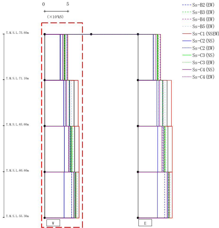
第4.2.2-14図 支持架構の最大応答せん断力(基本ケース, EW断面③, 有効応力解析)(1/2)
