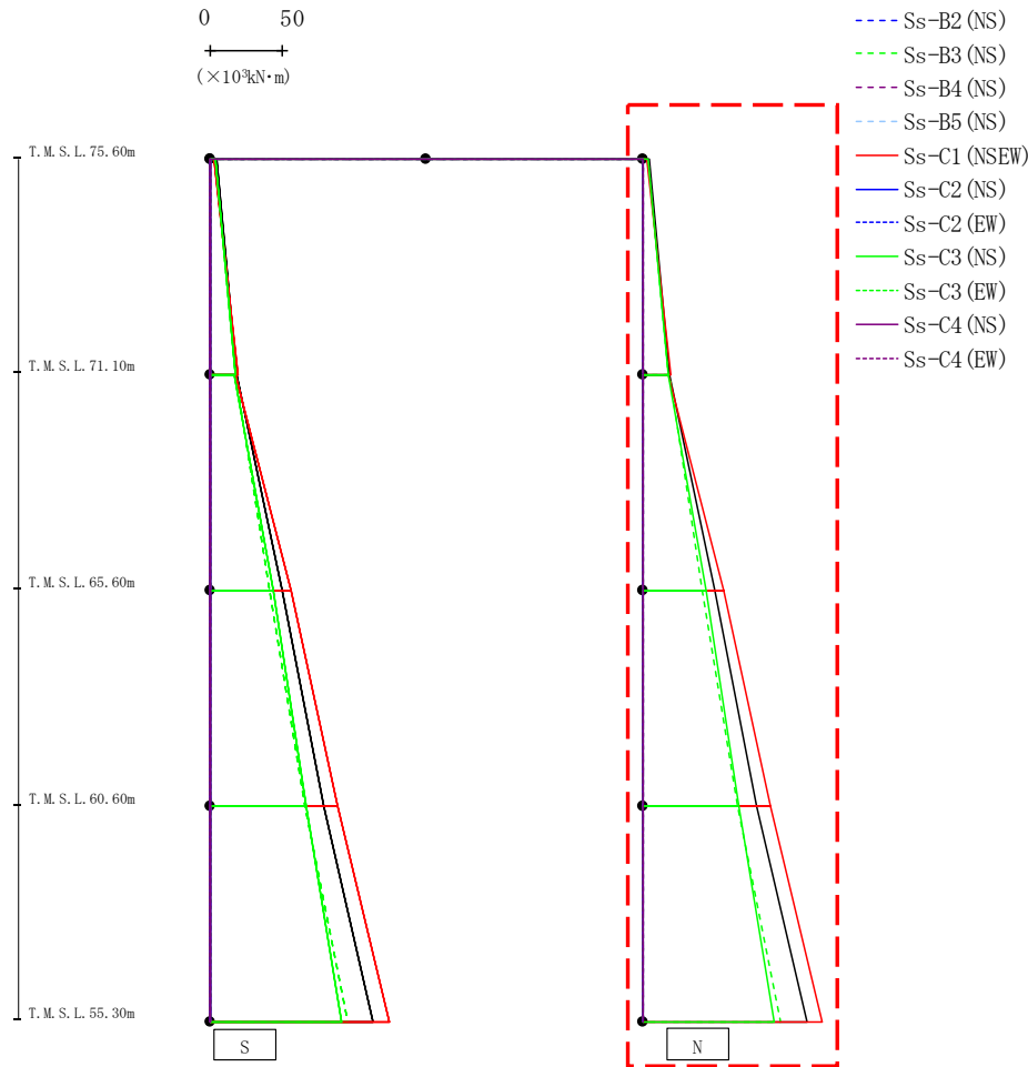
第4.2.2-39図 支持架構の最大応答曲げモーメント(-1σ地盤, NS断面③, 有効応力解析) (2/2)
