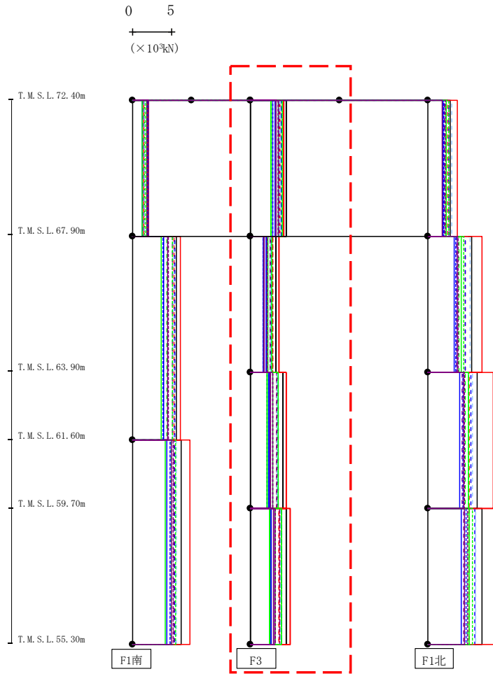
第4.2.2-10図 支持架構の最大応答せん断力 (G10B防護ネット架構, 基本ケース, EW断面②) (2/3)
