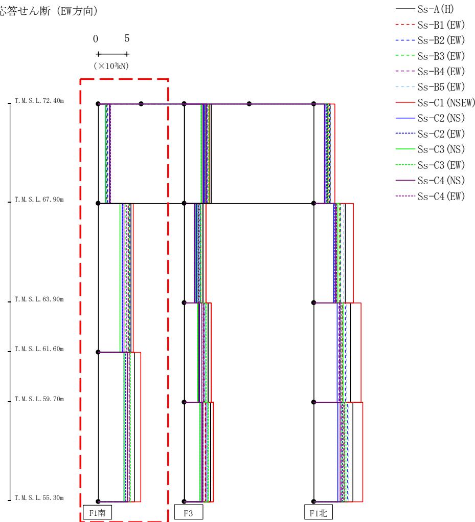
第4.2.1-6図 支持架構の最大応答せん断力(G10A防護ネット架構, 基本ケース, EW断面①) (1/3)
