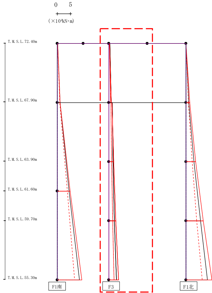
第4.2.1-15図 支持架構の最大応答曲げモーメント(G10A防護ネット架構, +1σ地盤, NS断面①) (2/3)
