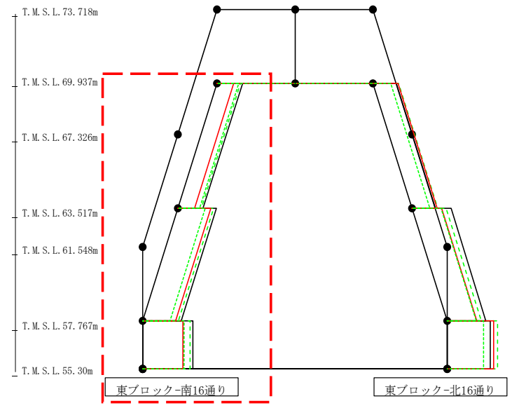
第4. 2. 1-14図 支持架構の最大応答せん断力(+1σ地盤, NS断面②, 全応力解析) (3/4)
