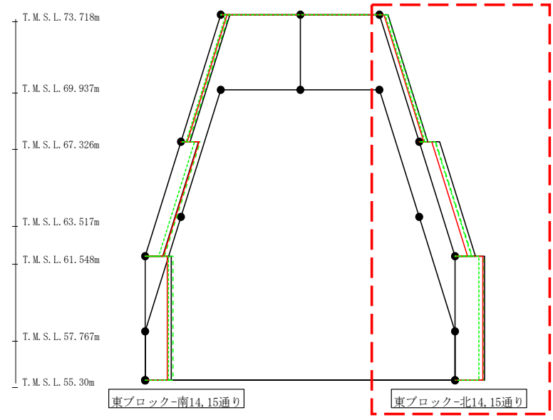
第4.2.1-14図 支持架構の最大応答せん断力(+1 \sigma 地盤, NS断面②, 全応力解析)(2/4)
