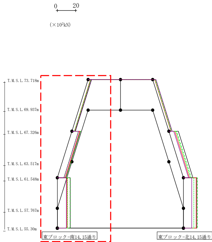
第4.2.1-62図 支持架構の最大応答せん断力(-1σ地盤, NS断面②, 有効応力解析) (1/4)
