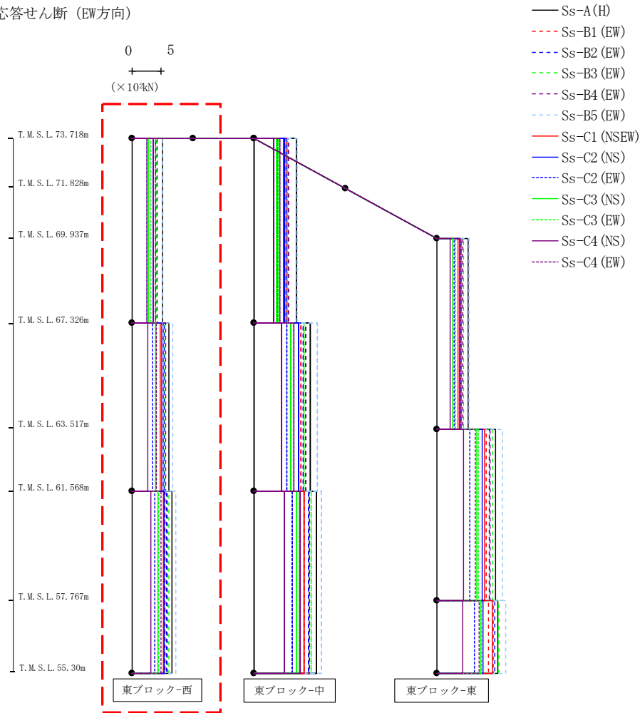
第4.2.1-46図 支持架構の最大応答せん断力(基本ケース, EW断面④, 有効応力解析)(1/3)
