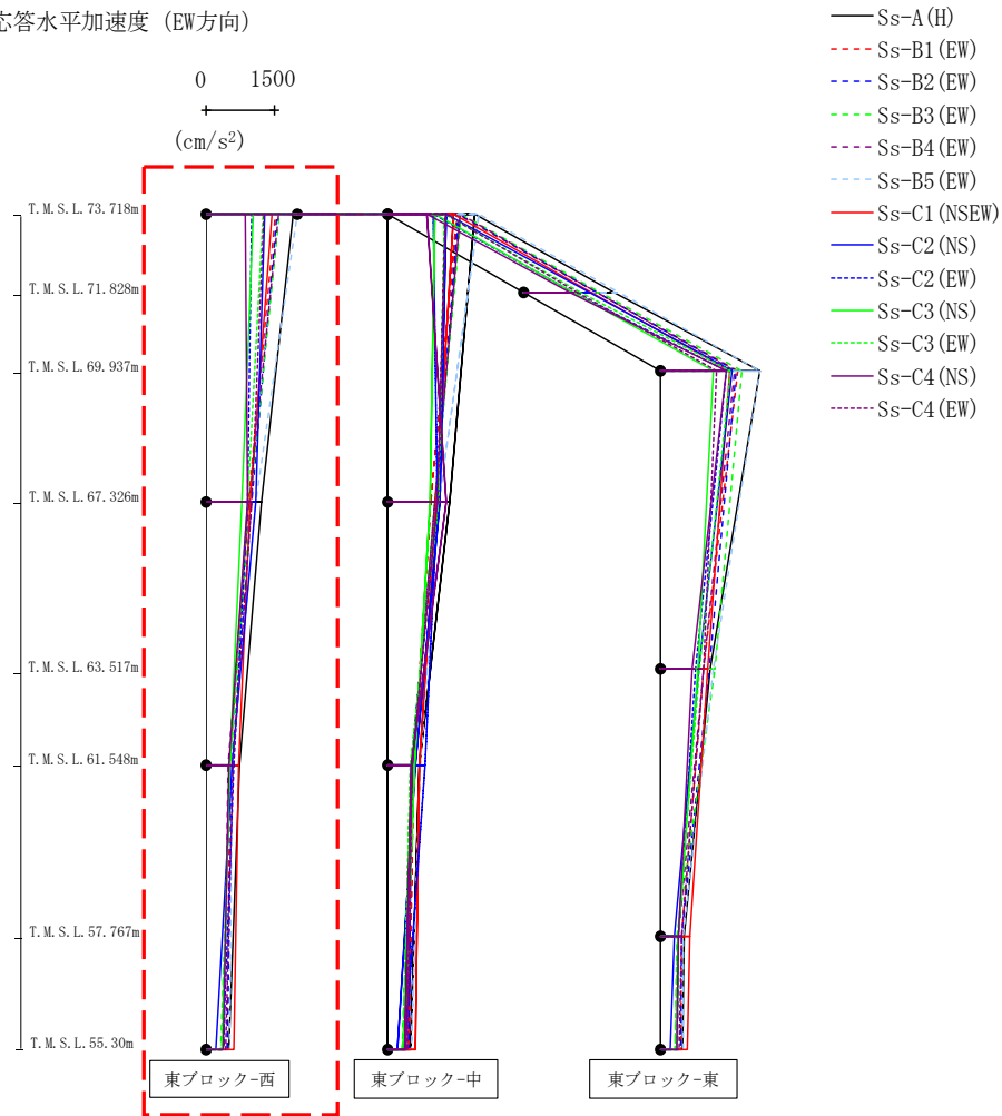
第4.2.1-41図 支持架構の最大応答加速度(基本ケース, EW断面③, 有効応力解析)(1/3)
