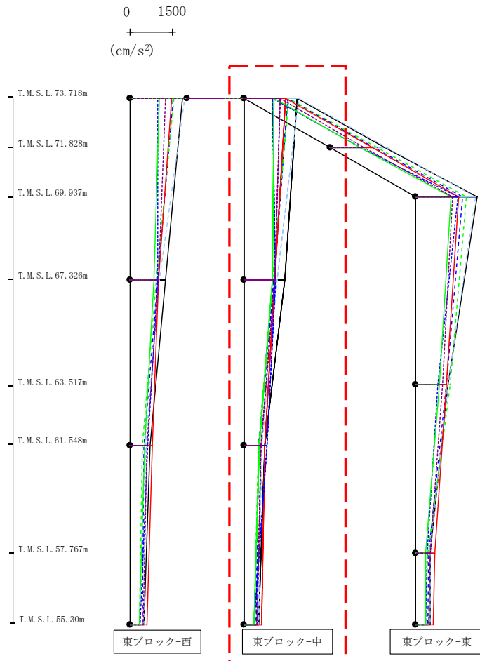
第4.2.1-53図 支持架構の最大応答加速度(+1σ地盤, EW断面③, 有効応力解析) (2/3)
