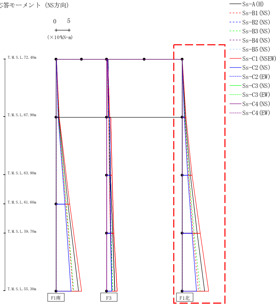
第4.2.2-27図 支持架構の最大応答曲げモーメント(G10B防護ネット架構, -1σ地盤, NS断面②) (3/3)
