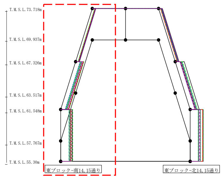
第4.2.1-2図 支持架構の最大応答せん断力(基本ケース, NS断面②, 全応力解析) (1/4)
