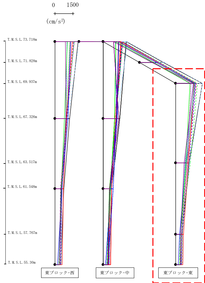
第4.2.1-41図 支持架構の最大応答加速度(基本ケース, EW断面③, 有効応力解析) (3/3)
