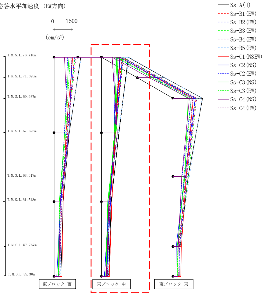
第4.2.1-45図 支持架構の最大応答加速度(基本ケース, EW断面④, 有効応力解析)(2/3)
