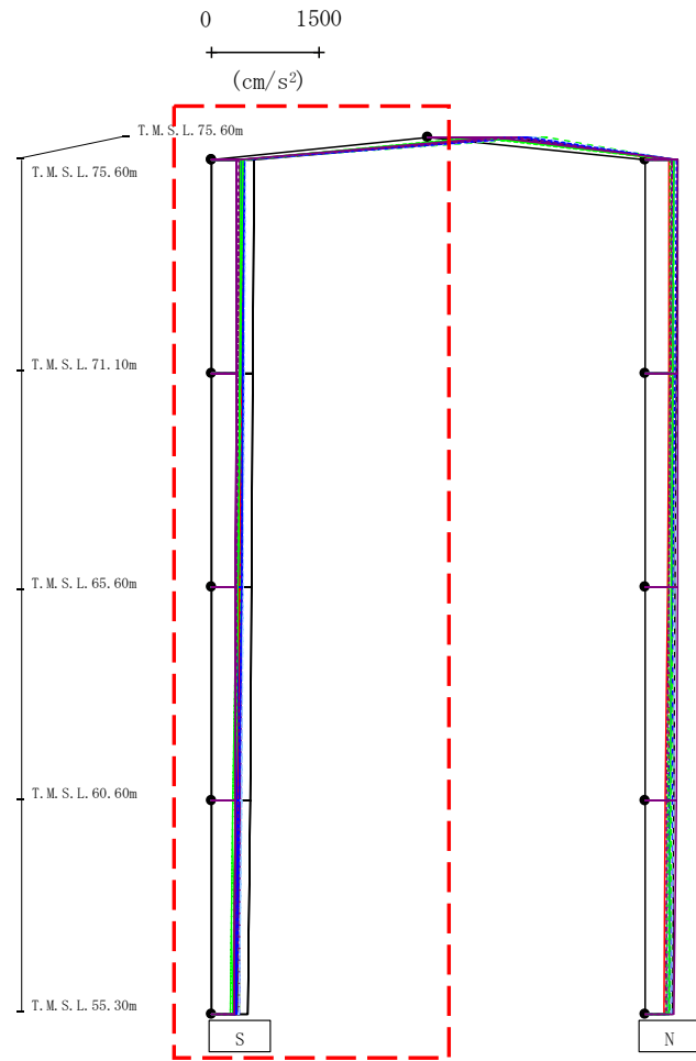
第4.2.1-8図 支持架構の最大応答鉛直加速度(基本ケース, NS断面③, 全応力解析) (1/2)
