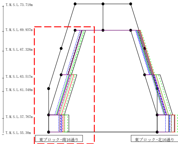
第4.2.1-38図 支持架構の最大応答せん断力(基本ケース, NS断面②, 有効応力解析)(3/4)
