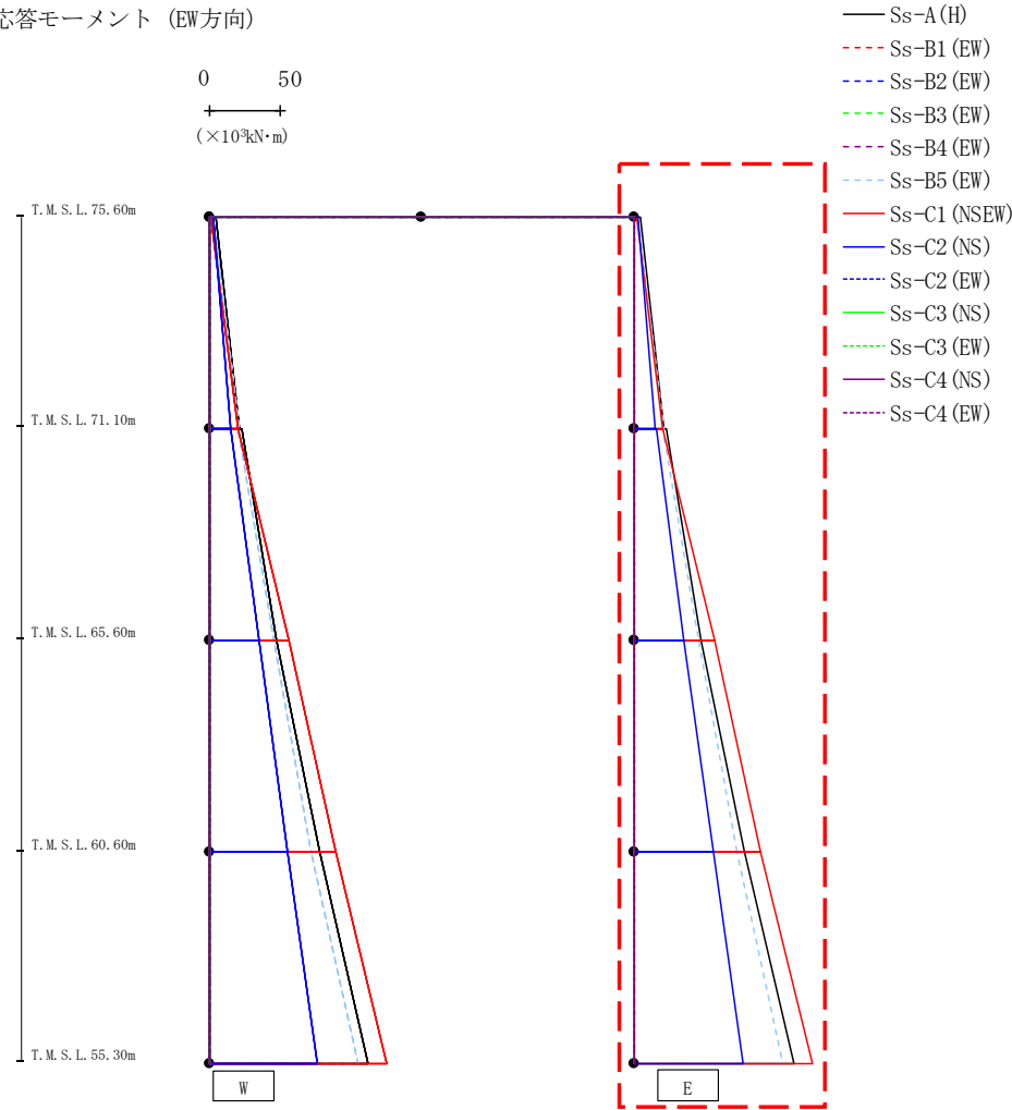
第4.2.1-47図 支持架構の最大応答曲げモーメント(-1σ地盤, EW断面③, 全応力解析) (2/2)
