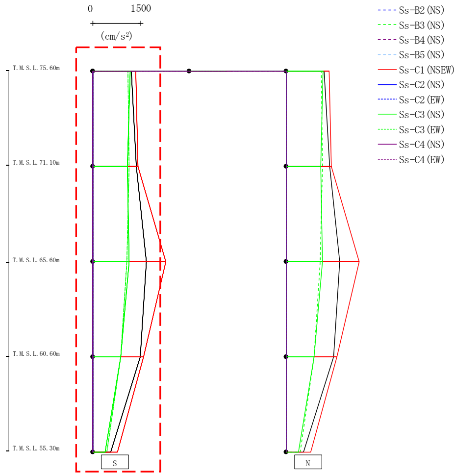
第4.2.1-37図 支持架構の最大応答加速度(-1σ地盤, NS断面③, 全応力解析) (1/2)
