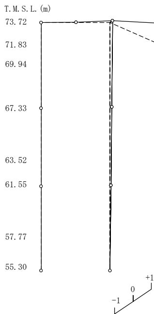
第4.1.1-3図 刺激関数図(EW方向モデル, EW断面④) (3/3)
