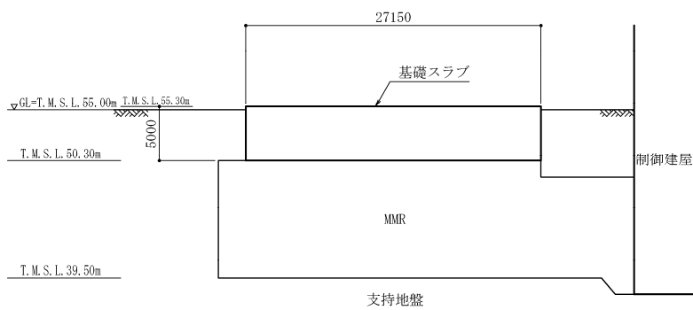
(d) D-D断面図(EW方向)
