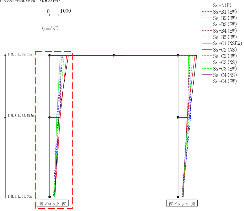
第4.2.2-69図 支持架構の最大応答加速度(-1σ地盤, EW断面④, 有効応力解析)(1/2)
