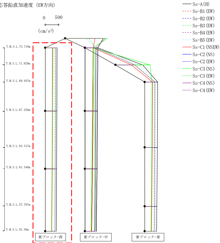
第4.2.1-36図 支持架構の最大応答鉛直加速度(-1σ地盤, EW断面④, 全応力解析) (1/3)
