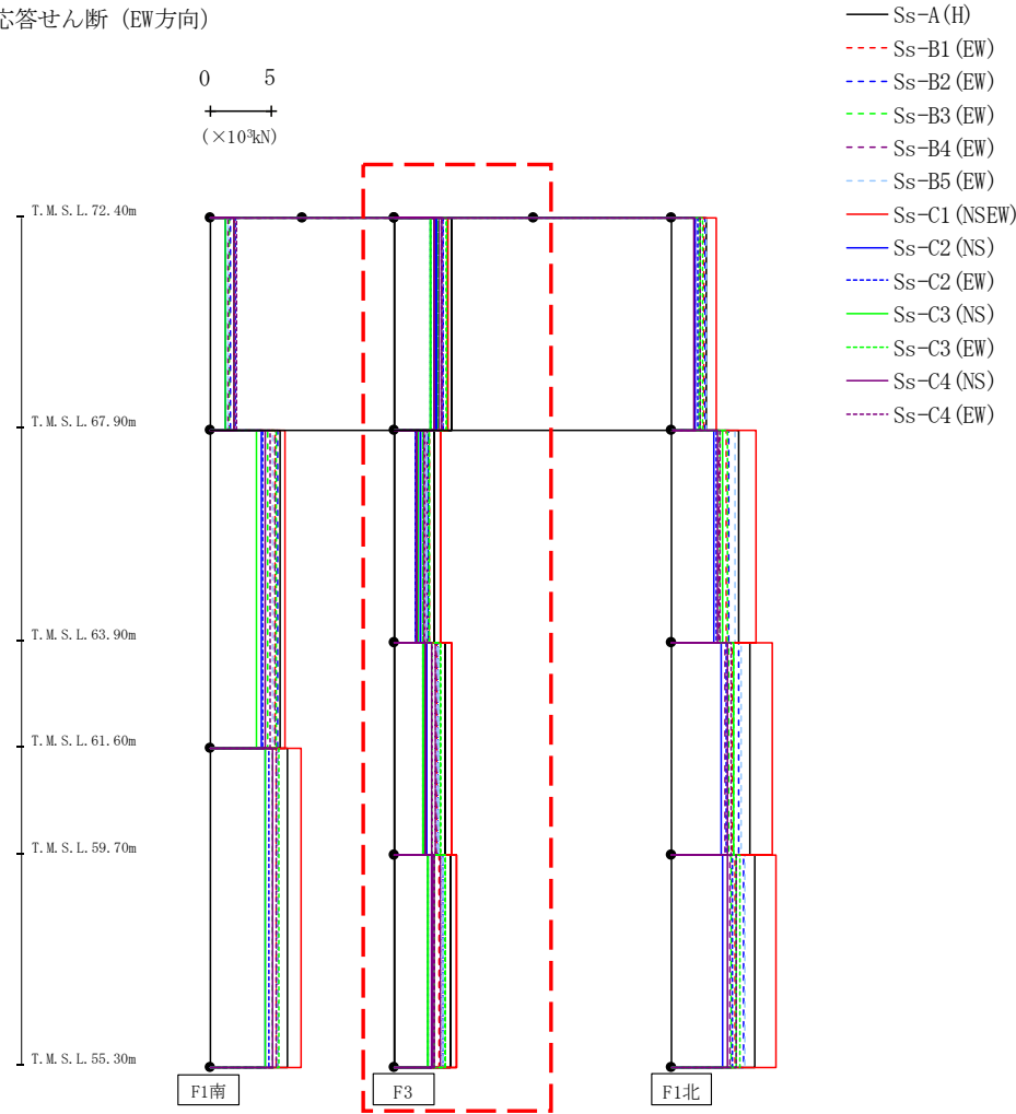
第4.2.1-6図 支持架構の最大応答せん断力(G10A防護ネット架構, 基本ケース, EW断面①) (2/3)
