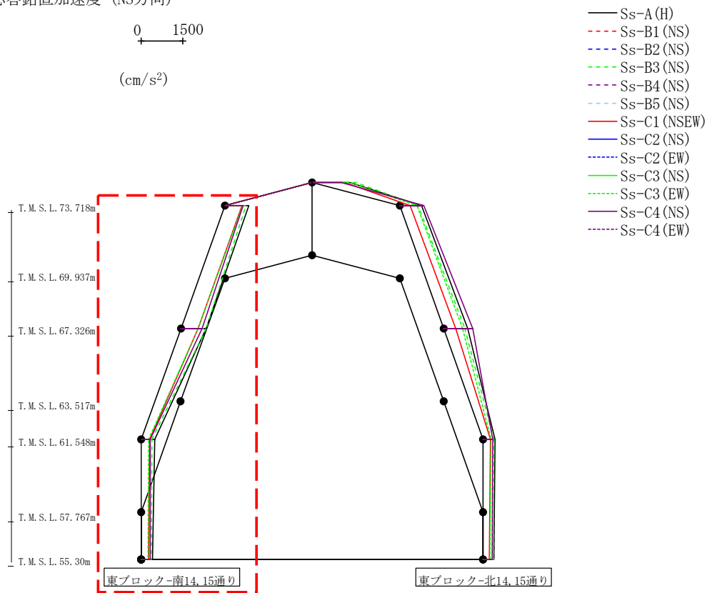
第4.2.1-52図 支持架構の最大応答鉛直加速度(+1σ地盤, NS断面②, 有効応力解析)(1/4)
