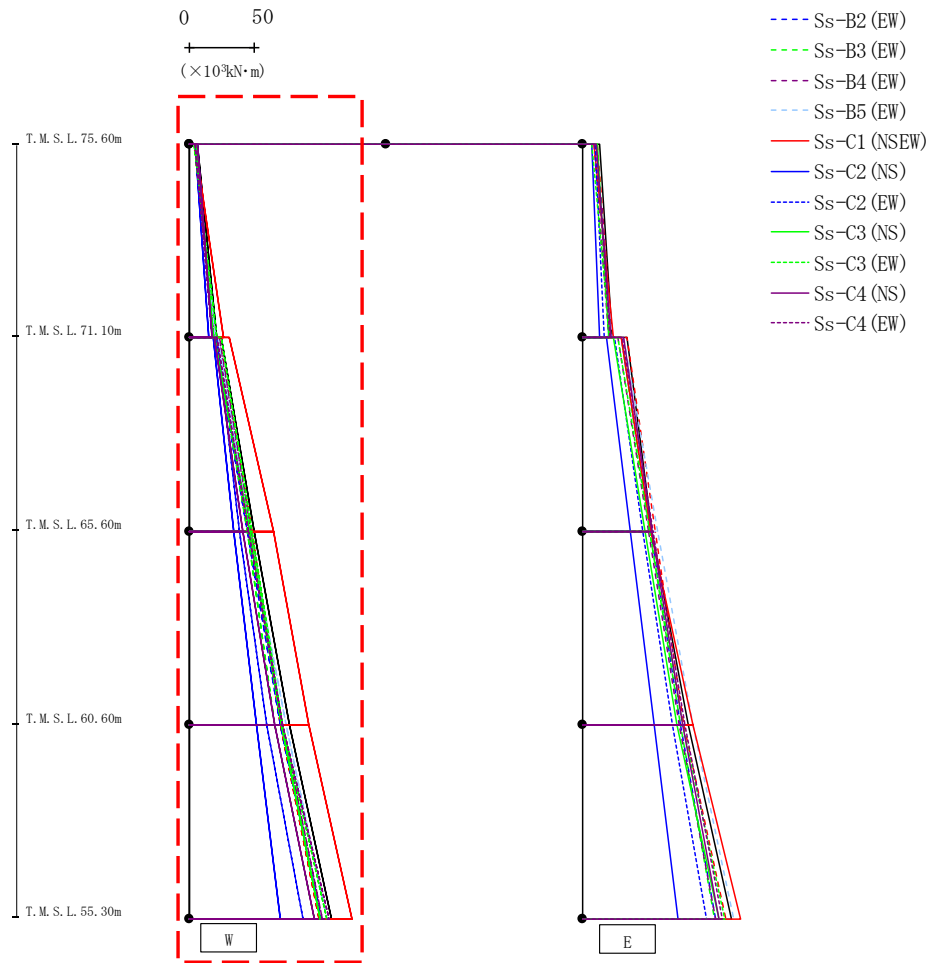
第4.2.1-11図 支持架構の最大応答曲げモーメント(基本ケース, EW断面①, 全応力解析) (1/2)
