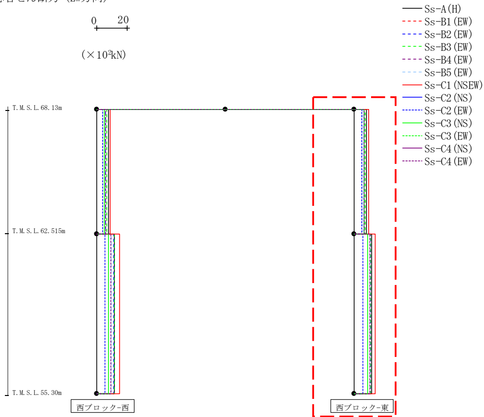
第4.2.2-54図 支持架構の最大応答せん断力(+1σ地盤, EW断面③, 有効応力解析) (2/2)
