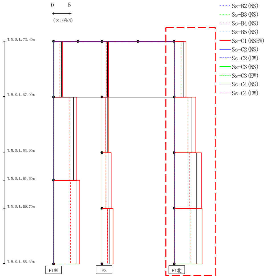
第4.2.1-26図 支持架構の最大応答せん断力(G10A防護ネット架構, -1σ地盤, NS断面①) (3/3)
