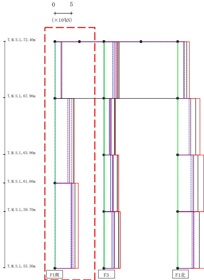
第4.2.2-22図 支持架構の最大応答せん断力(G10B防護ネット架構, +1σ地盤, EW断面②) (1/3)
