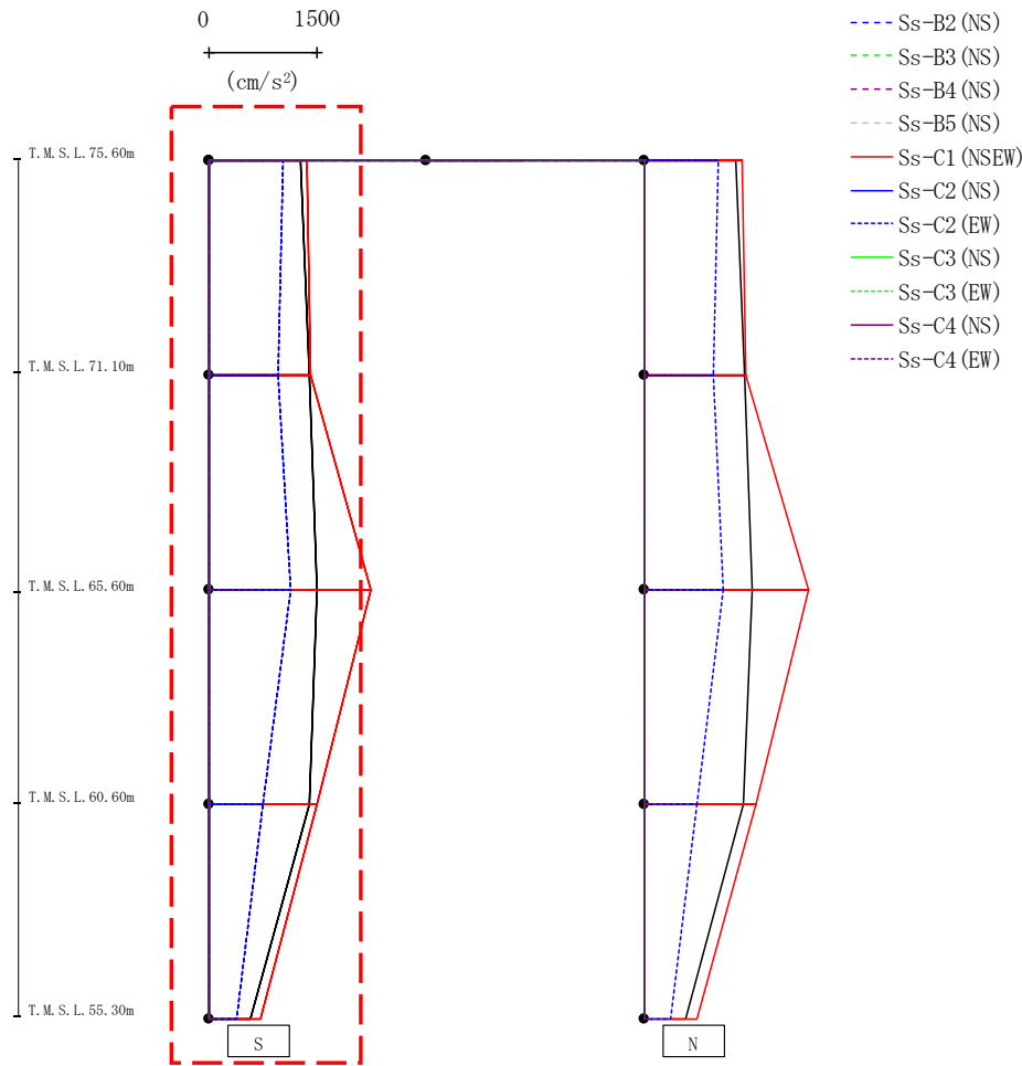
第4.2.2-33図 支持架構の最大応答加速度(-1σ地盤, NS断面①, 有効応力解析)(1/2)
