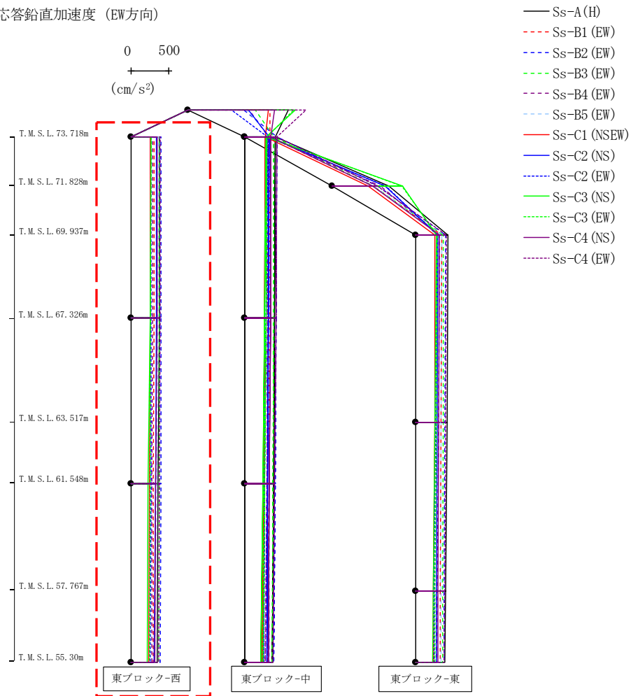
第4.2.1-44図 支持架構の最大応答鉛直加速度(基本ケース, EW断面③, 有効応力解析)(1/3)
