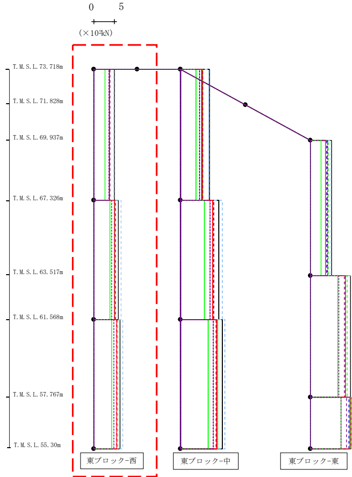
第4.2.1-58図 支持架構の最大応答せん断力(+1σ地盤, EW断面④, 有効応力解析) (1/3)
