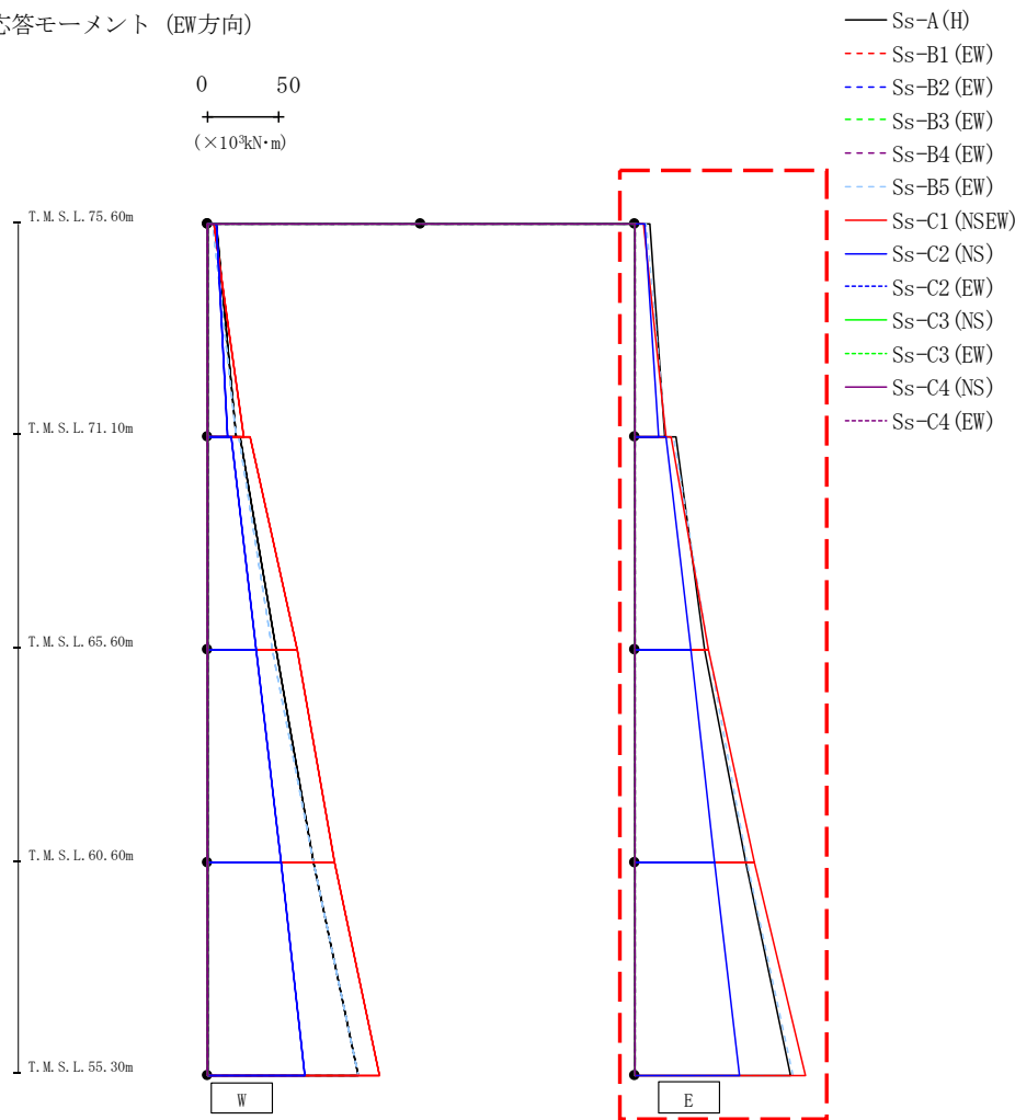
第4.2.1-27図 支持架構の最大応答曲げモーメント(+1σ地盤, EW断面①, 全応力解析)(2/2)
