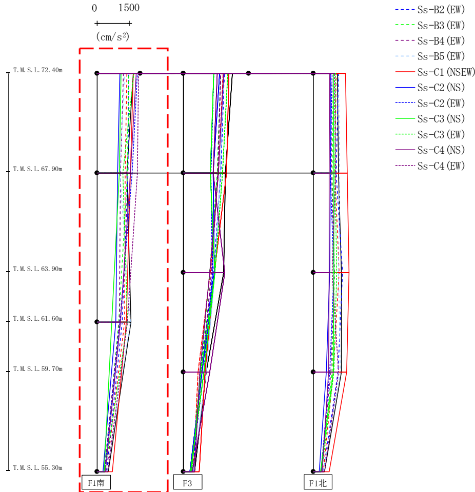
第4.2.1-5図 支持架構の最大応答加速度(G10A防護ネット架構, 基本ケース, EW断面①) (1/3)
