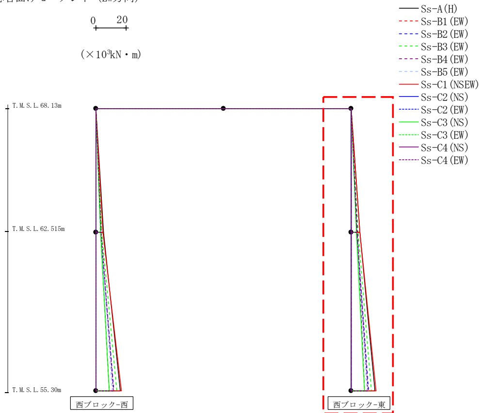
第4.2.2-59図 支持架構の最大応答曲げモーメント(+1σ地盤, EW断面④, 有効応力解析) (2/2)
