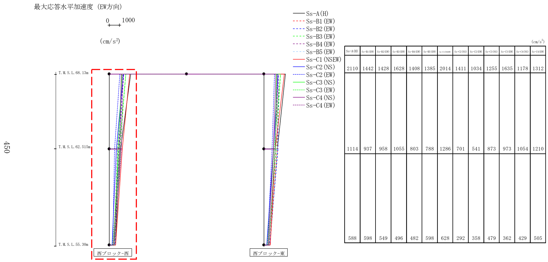
第4.2.2-45図 支持架構の最大応答加速度(基本ケース, EW断面④, 有効応力解析)(1/2)
