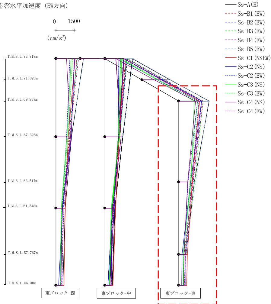
第4.2.1-45図 支持架構の最大応答加速度(基本ケース, EW断面④, 有効応力解析)(3/3)
