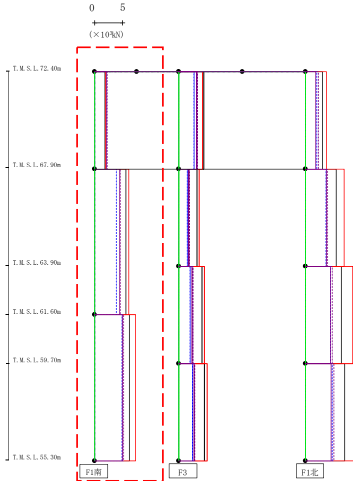
第4.2.2-34図 支持架構の最大応答せん断力(G10B防護ネット架構, -1σ地盤, EW断面②) (1/3)
