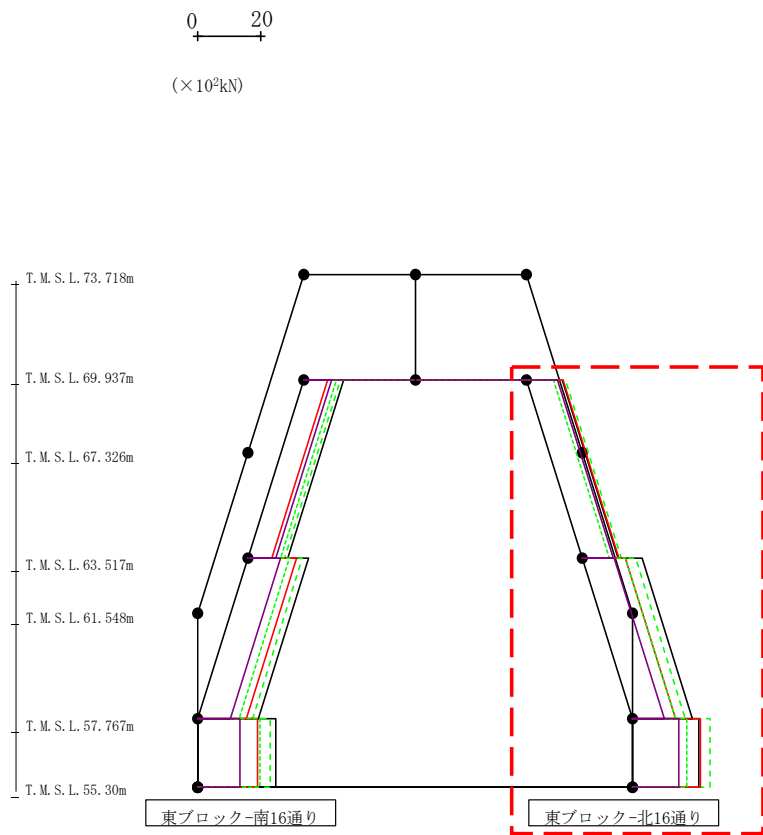
第4.2.1-50図 支持架構の最大応答せん断力(+1σ地盤, NS断面②, 有効応力解析) (4/4)
