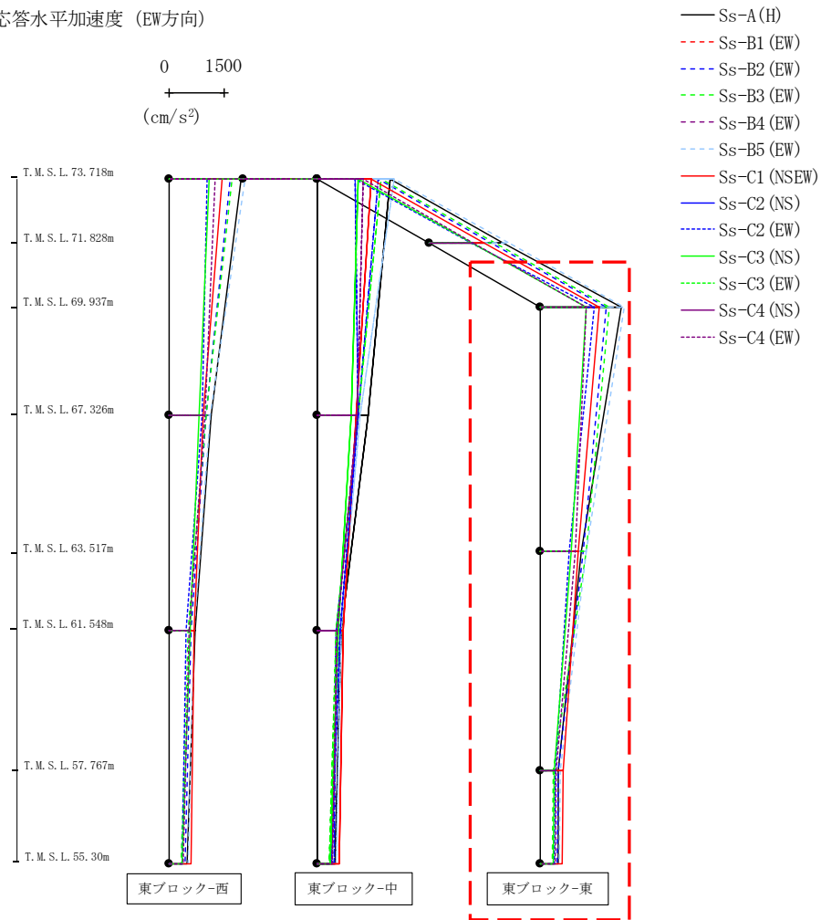
第4.2.1-65図 支持架構の最大応答加速度(-1σ地盤, EW断面③, 有効応力解析) (3/3)
