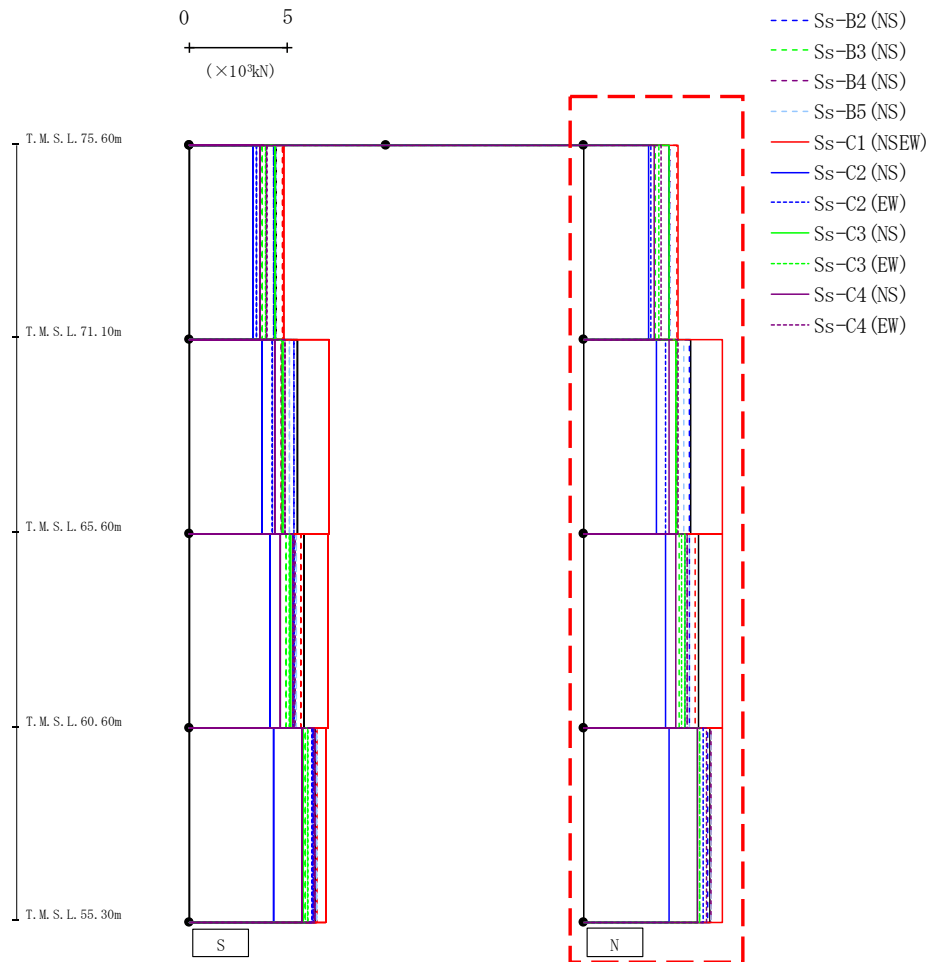
第4.2.2-2図 支持架構の最大応答せん断力(基本ケース, NS断面①, 有効応力解析)(2/2)
