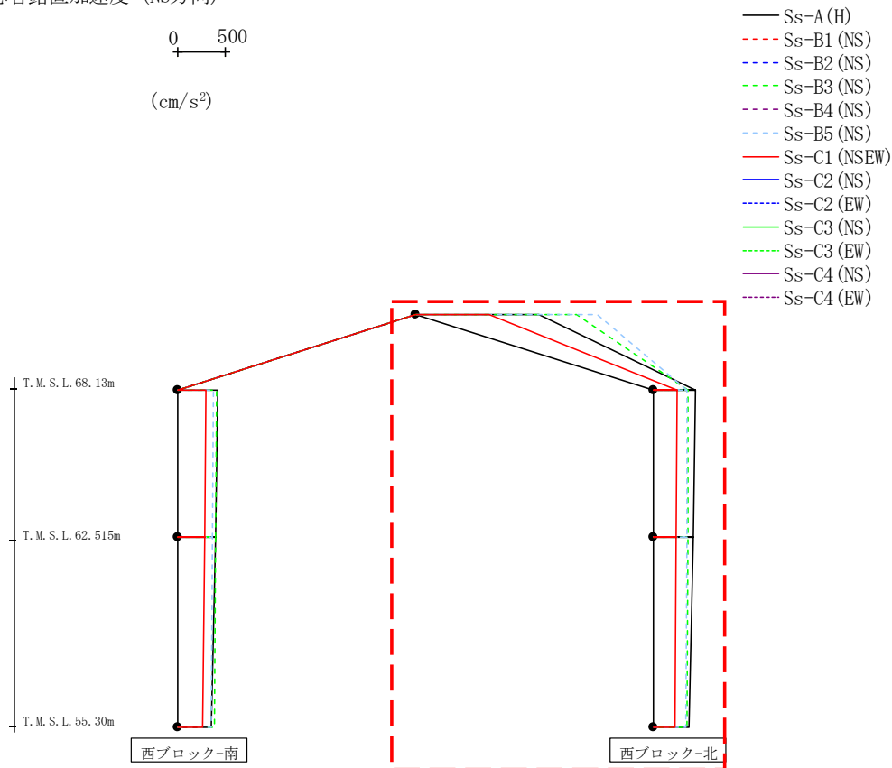
第4.2.2-28図 支持架構の最大応答鉛直加速度(-1σ地盤, NS断面①, 全応力解析)(2/2)
