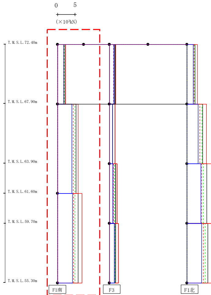
第4.2.2-14図 支持架構の最大応答せん断力(G10B防護ネット架構, +1σ地盤, NS断面②) (1/3)
