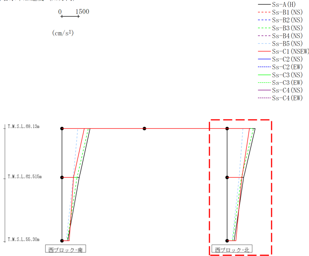
第4.2.2-61図 支持架構の最大応答加速度(-1σ地盤, NS断面①, 有効応力解析)(2/2)
