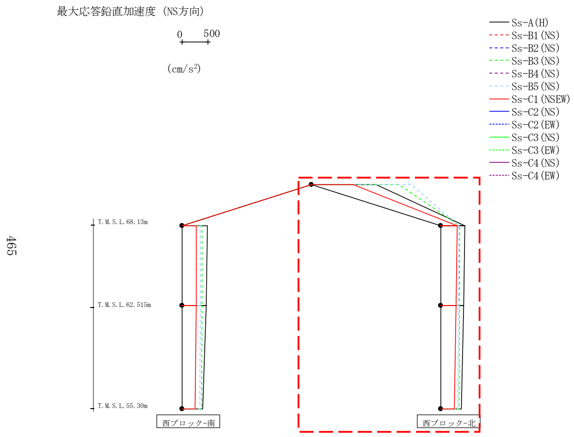
第4.2.2-52図 支持架構の最大応答鉛直加速度(+1σ地盤, NS断面①, 有効応力解析)(2/2)
