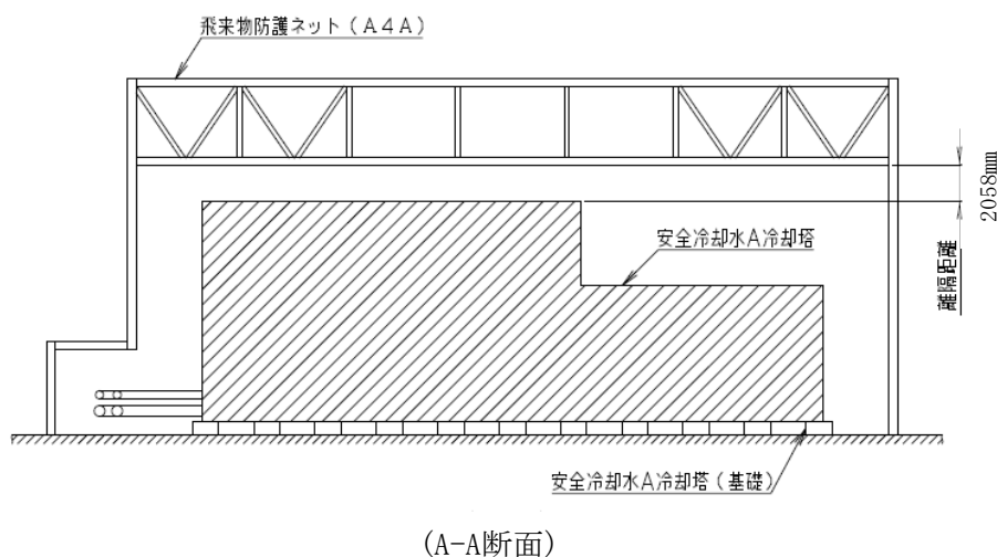
(a) 飛来物防護ネット架構と冷却塔
