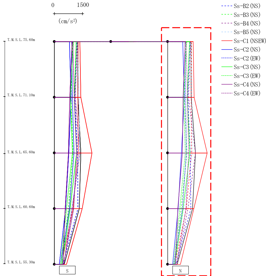
第4.2.1-1図 支持架構の最大応答加速度(基本ケース, NS断面①, 全応力解析) (2/2)
