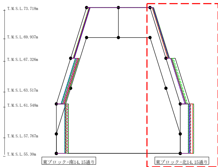
第4.2.1-38図 支持架構の最大応答せん断力(基本ケース, NS断面②, 有効応力解析)(2/4)
