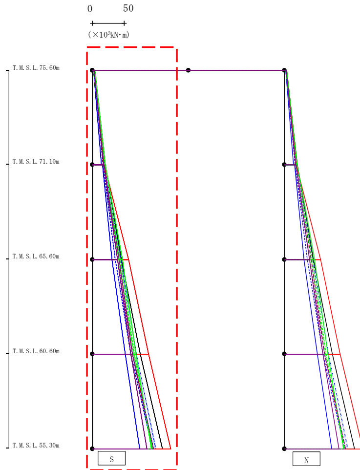
第4.2.1-7図 支持架構の最大応答曲げモーメント(基本ケース, NS断面③, 全応力解析)(1/2)
