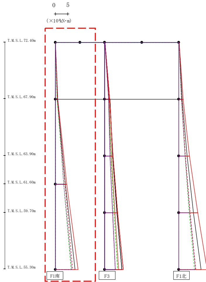
第4.2.1-35図 支持架構の最大応答曲げモーメント (G10A防護ネット架構, -1\sigma 地盤, EW断面②) (1/3)
