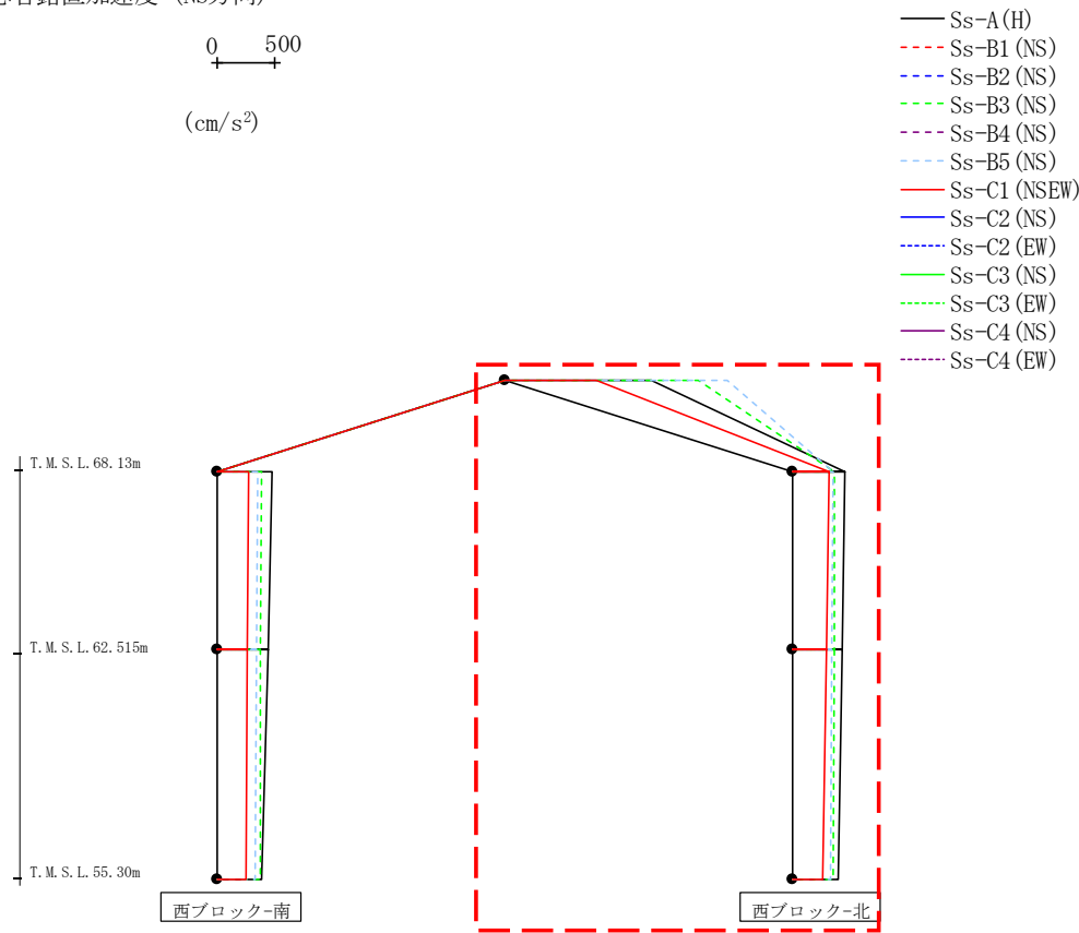
第4.2.2-16図 支持架構の最大応答鉛直加速度(+1σ地盤, NS断面①, 全応力解析) (2/2)
