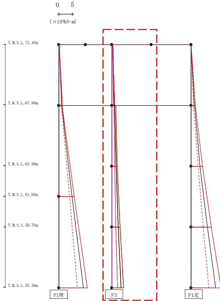
第4.2.1-27図 支持架構の最大応答曲げモーメント (G10A防護ネット架構, -1σ地盤, NS断面①) (2/3)
