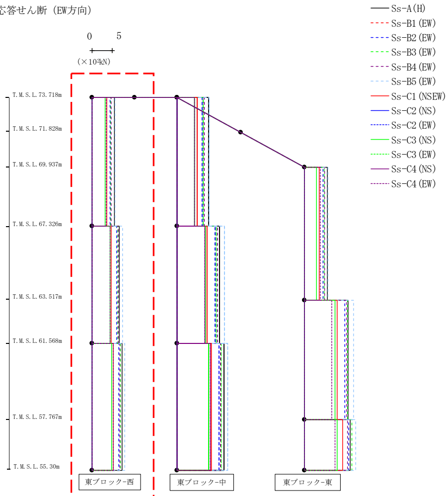
第4.2.1-70図 支持架構の最大応答せん断力(-1σ地盤, EW断面④, 有効応力解析) (1/3)
