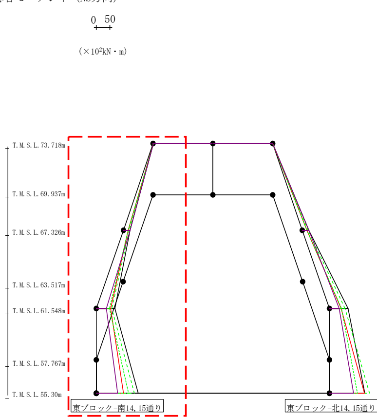
第4.2.1-63図 支持架構の最大応答曲げモーメント(-1σ地盤, NS断面②, 有効応力解析) (1/4)
