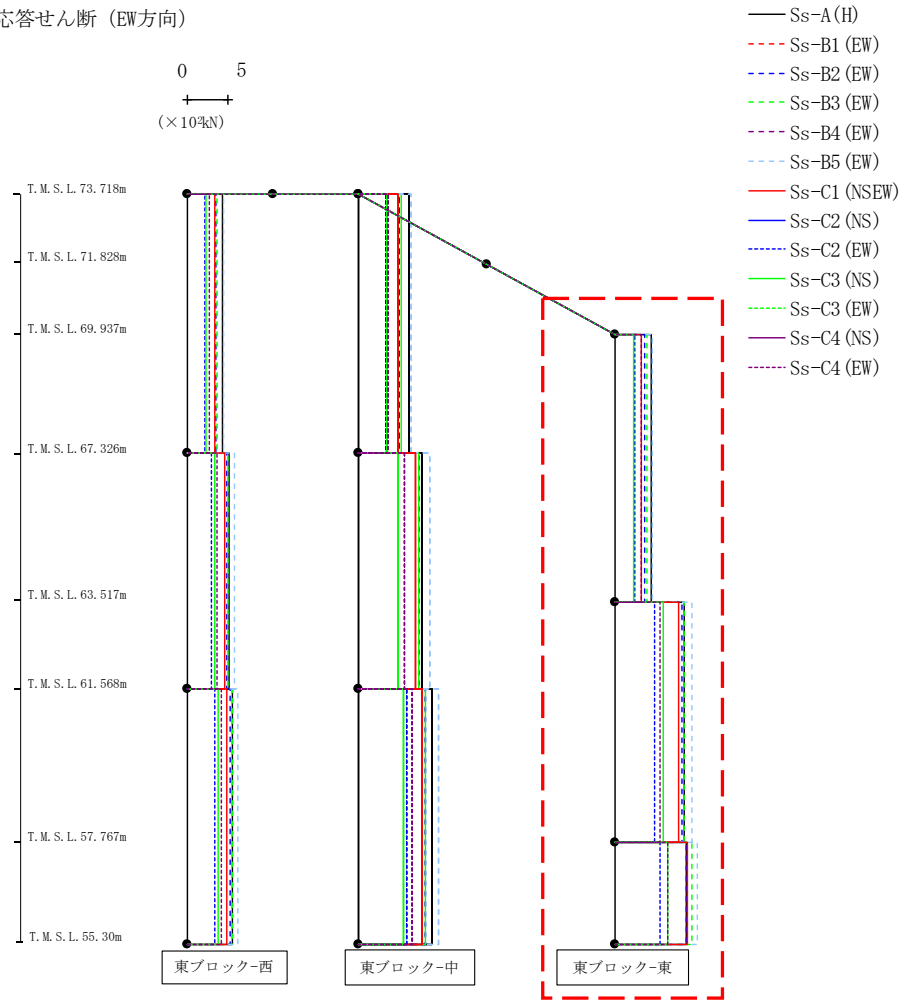
第4.2.1-54図 支持架構の最大応答せん断力(+1σ地盤, EW断面③, 有効応力解析) (3/3)
