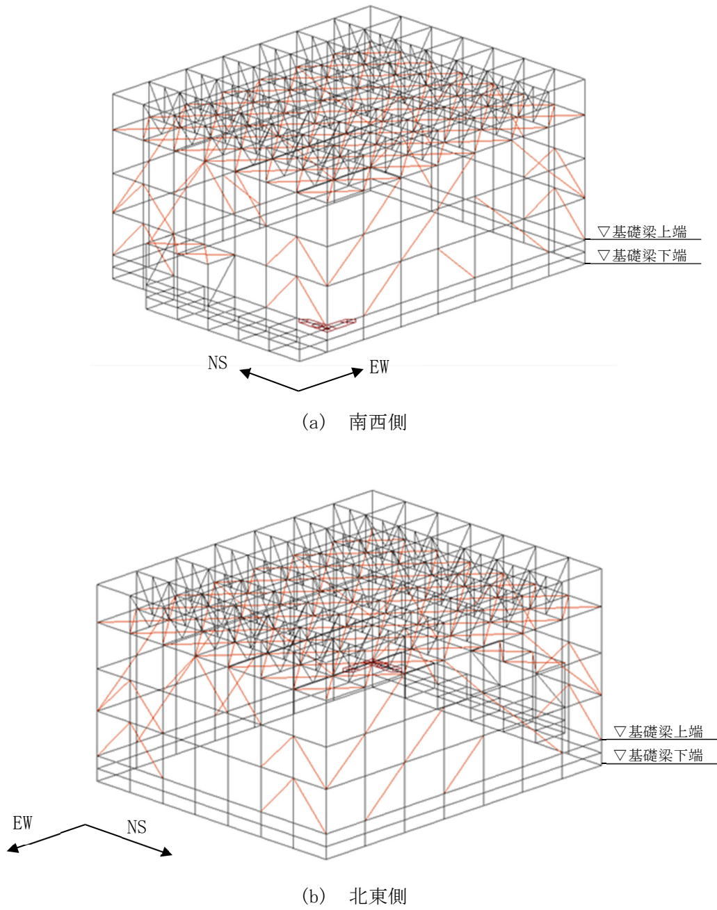
第3.1.4-1図 支持架構の解析モデル
