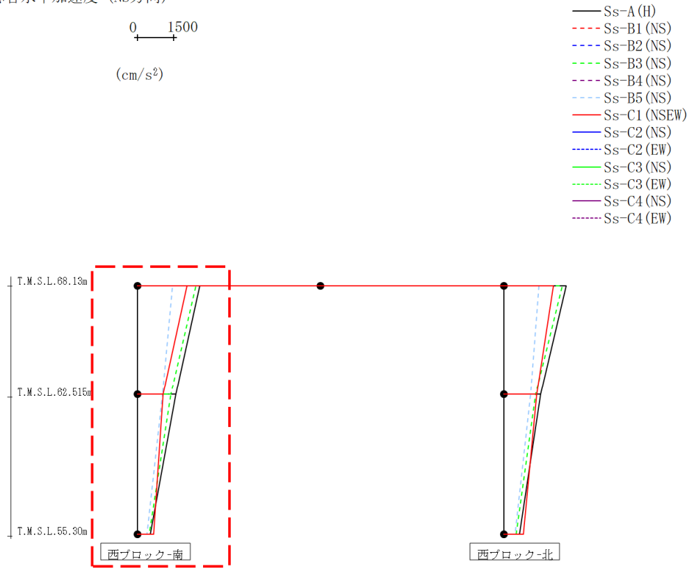
第4.2.2-61図 支持架構の最大応答加速度(-1σ地盤, NS断面①, 有効応力解析)(1/2)
