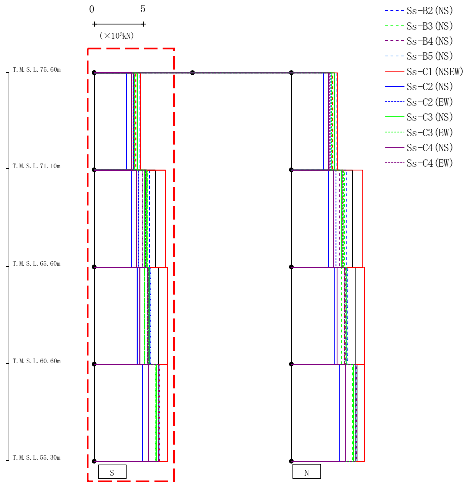
第4.2.2-6図 支持架構の最大応答せん断力(基本ケース, NS断面③, 有効応力解析) (1/2)
