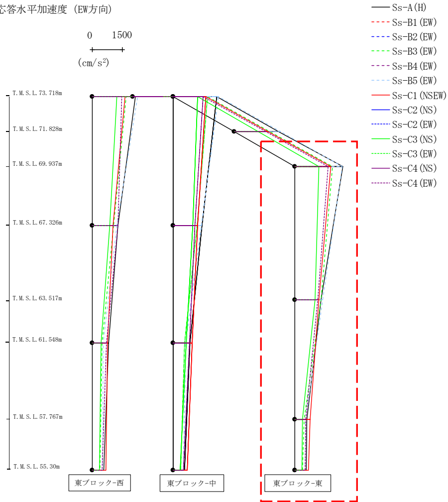
第4.2.1-21図 支持架構の最大応答加速度(+1σ地盤, EW断面④, 全応力解析) (3/3)
