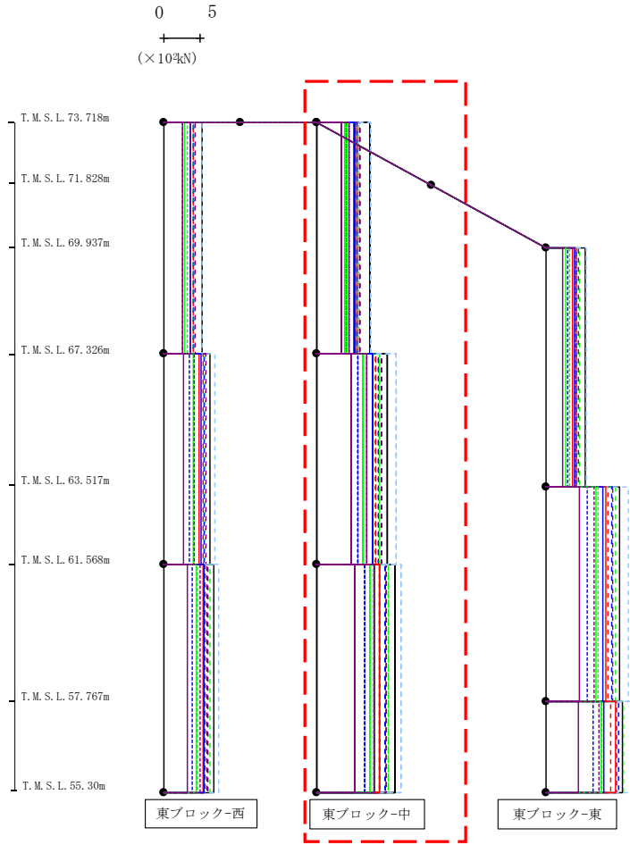
第4.2.1-46図 支持架構の最大応答せん断力(基本ケース, EW断面④, 有効応力解析)(2/3)
