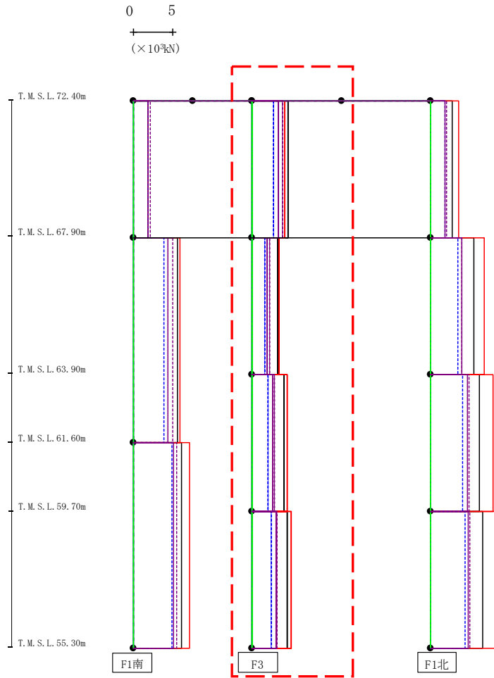
第4.2.2-22図 支持架構の最大応答せん断力(G10B防護ネット架構, +1σ地盤, EW断面②) (2/3)
