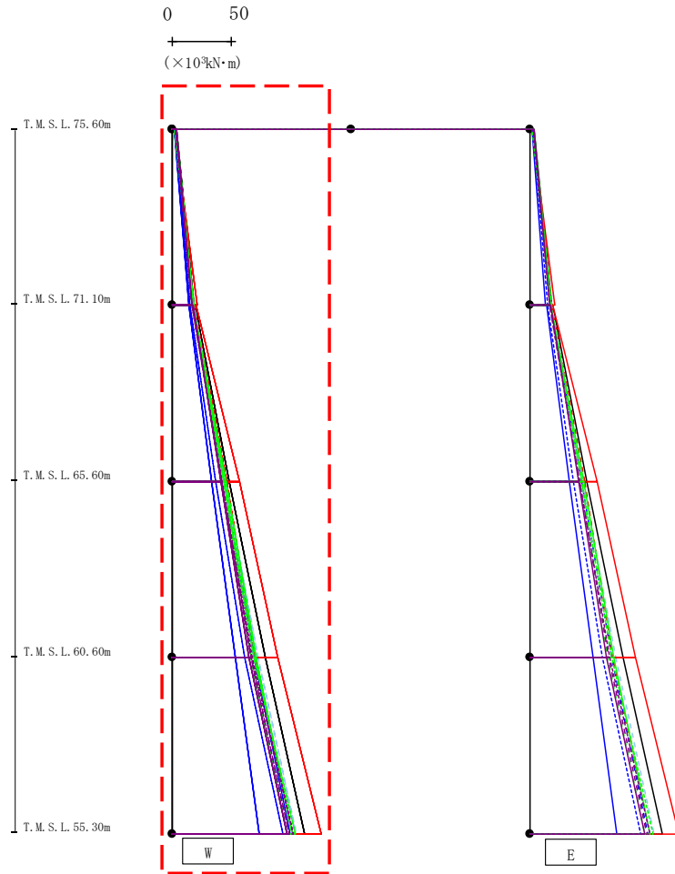
第4.2.1-15図 支持架構の最大応答曲げモーメント(基本ケース, EW断面③, 全応力解析)(1/2)
