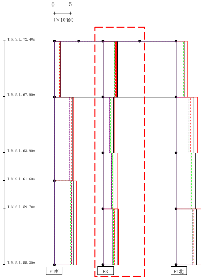
第4.2.2-30図 支持架構の最大応答せん断力(G10B防護ネット架構, -1σ地盤, EW断面①) (2/3)
