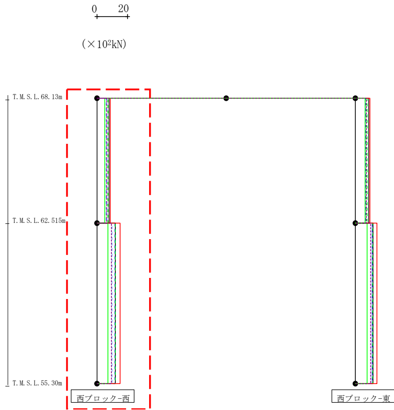
第4.2.2-30図 支持架構の最大応答せん断力(-1σ地盤, EW断面③, 全応力解析) (1/2)
