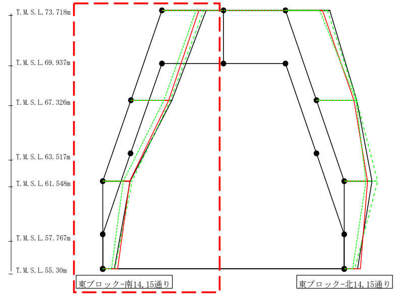
第4.2.1-25図 支持架構の最大応答加速度(-1σ地盤, NS断面②, 全応力解析) (1/4)
