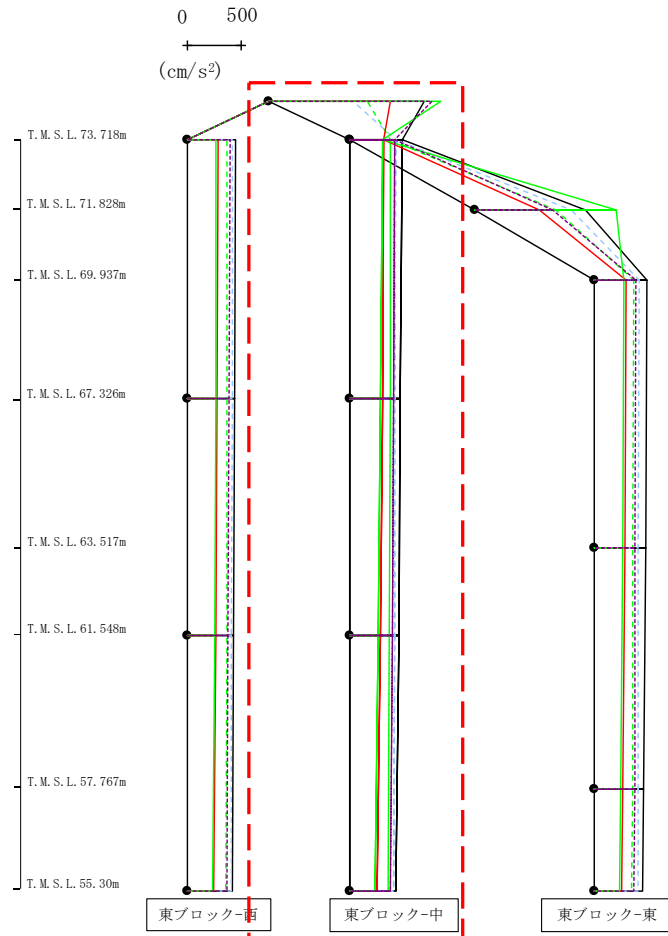
第4.2.1-36図 支持架構の最大応答鉛直加速度(-1σ地盤, EW断面④, 全応力解析) (2/3)
