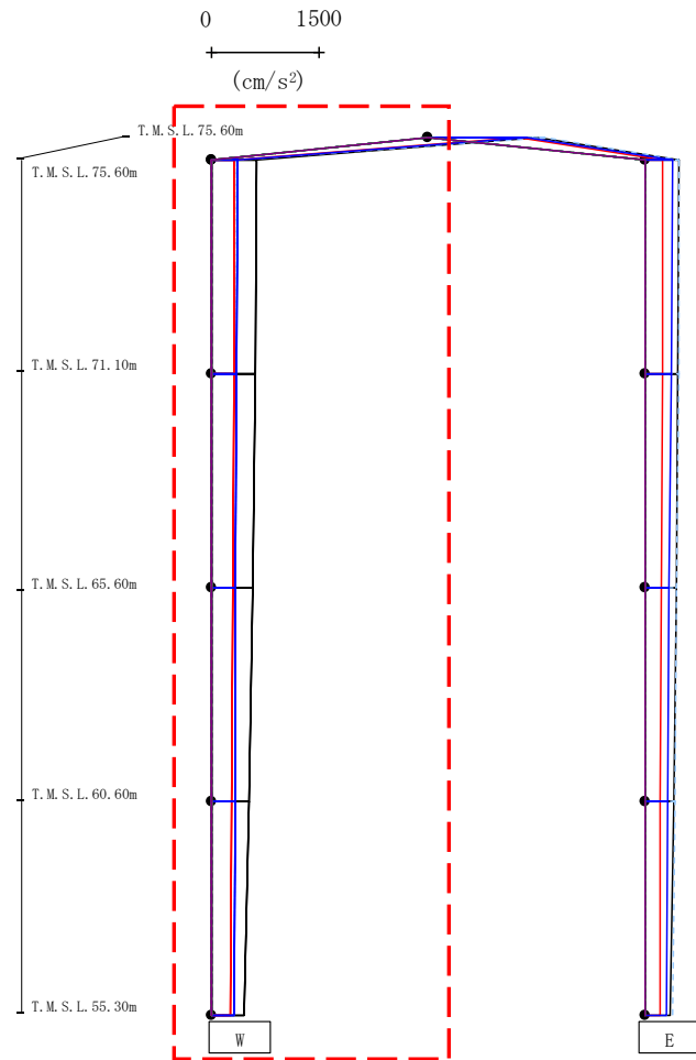
第4.2.2-44図 支持架構の最大応答鉛直加速度(-1σ地盤, EW断面①, 有効応力解析)(1/2)
