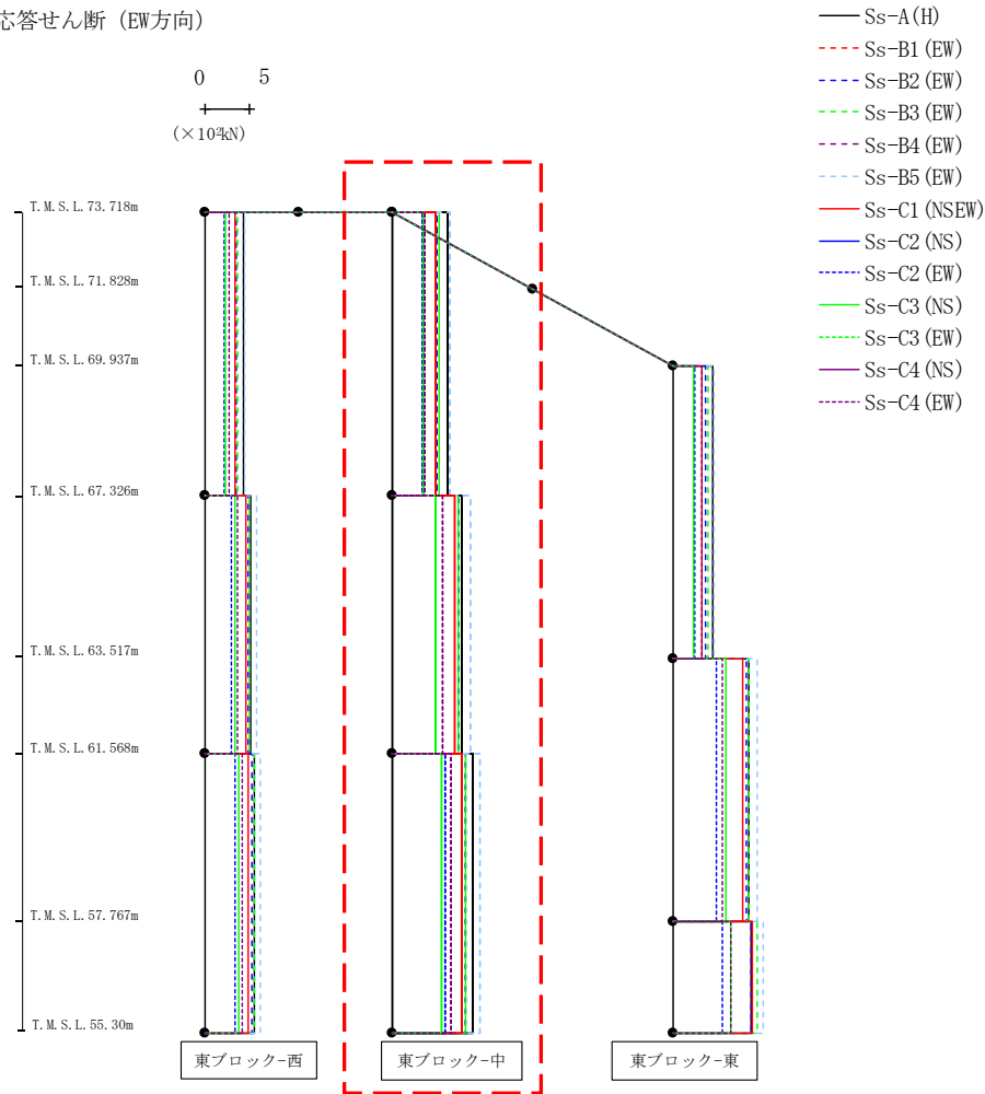
第4.2.1-54図 支持架構の最大応答せん断力(+1σ地盤, EW断面③, 有効応力解析) (2/3)
