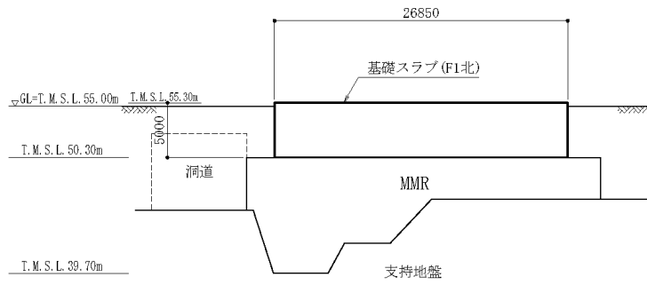
(b) B-B断面 (EW方向)
