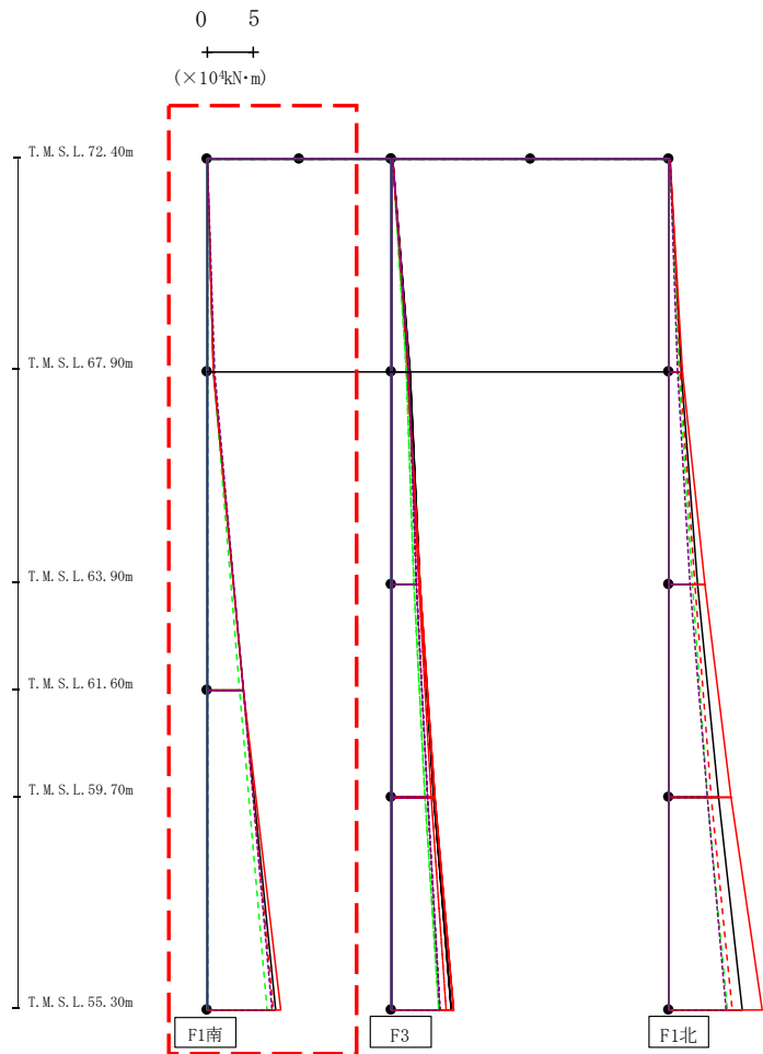
第4.2.2-19図 支持架構の最大応答曲げモーメント (G10B防護ネット架構, +1σ地盤, EW断面①) (1/3)
