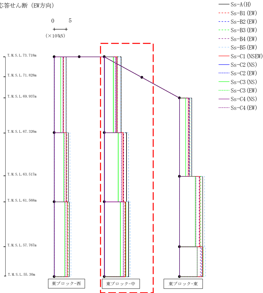
第4.2.1-58図 支持架構の最大応答せん断力(+1σ地盤, EW断面④, 有効応力解析) (2/3)
