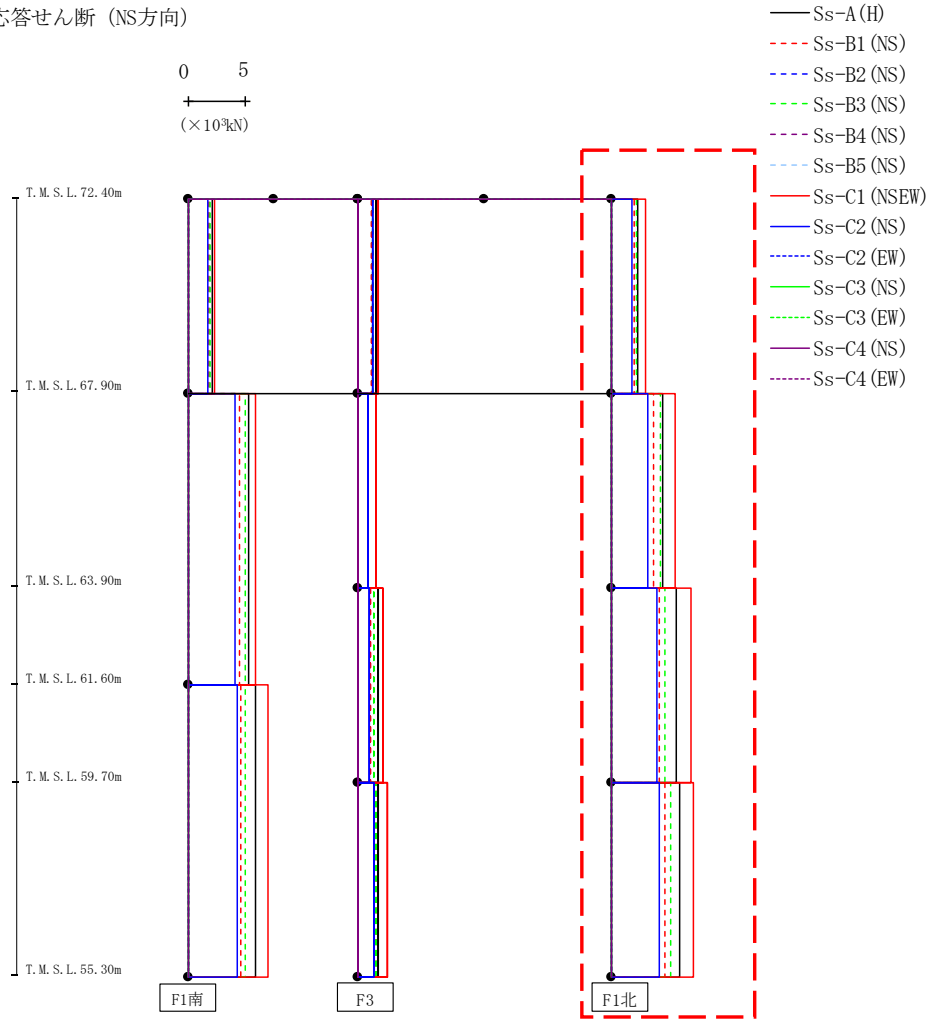
第4.2.2-14図 支持架構の最大応答せん断力(G10B防護ネット架構, +1σ地盤, NS断面②) (3/3)
