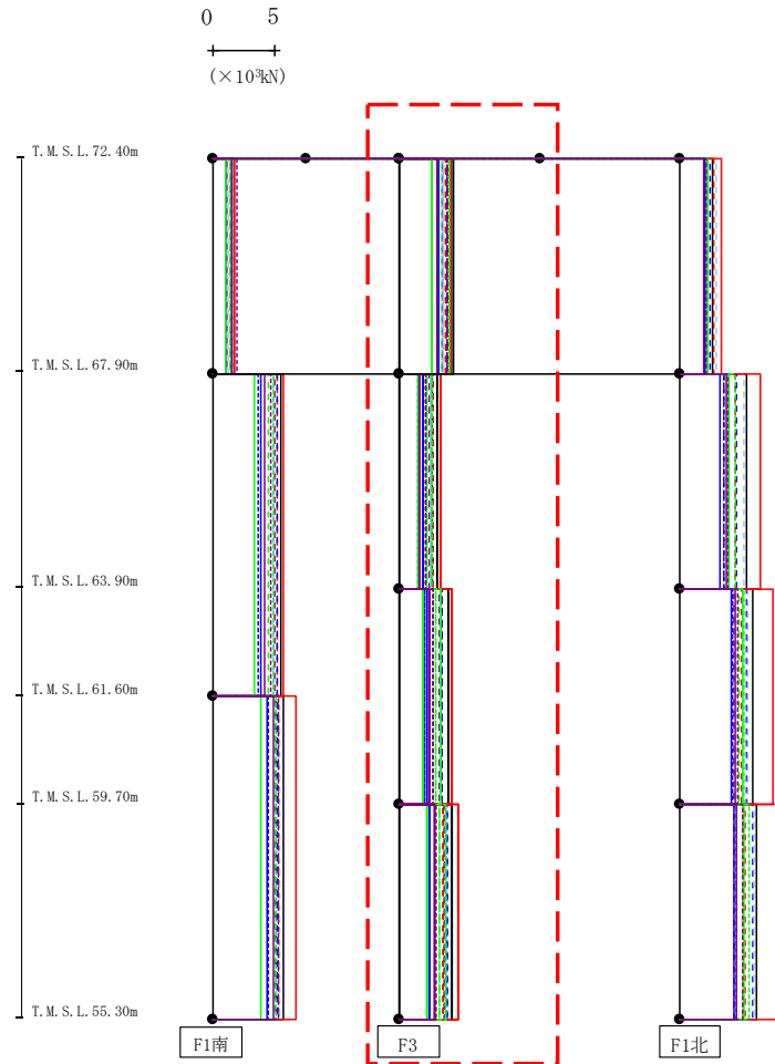
第4.2.2-6図 支持架構の最大応答せん断力(G10B防護ネット架構, 基本ケース, EW断面①) (2/3)
