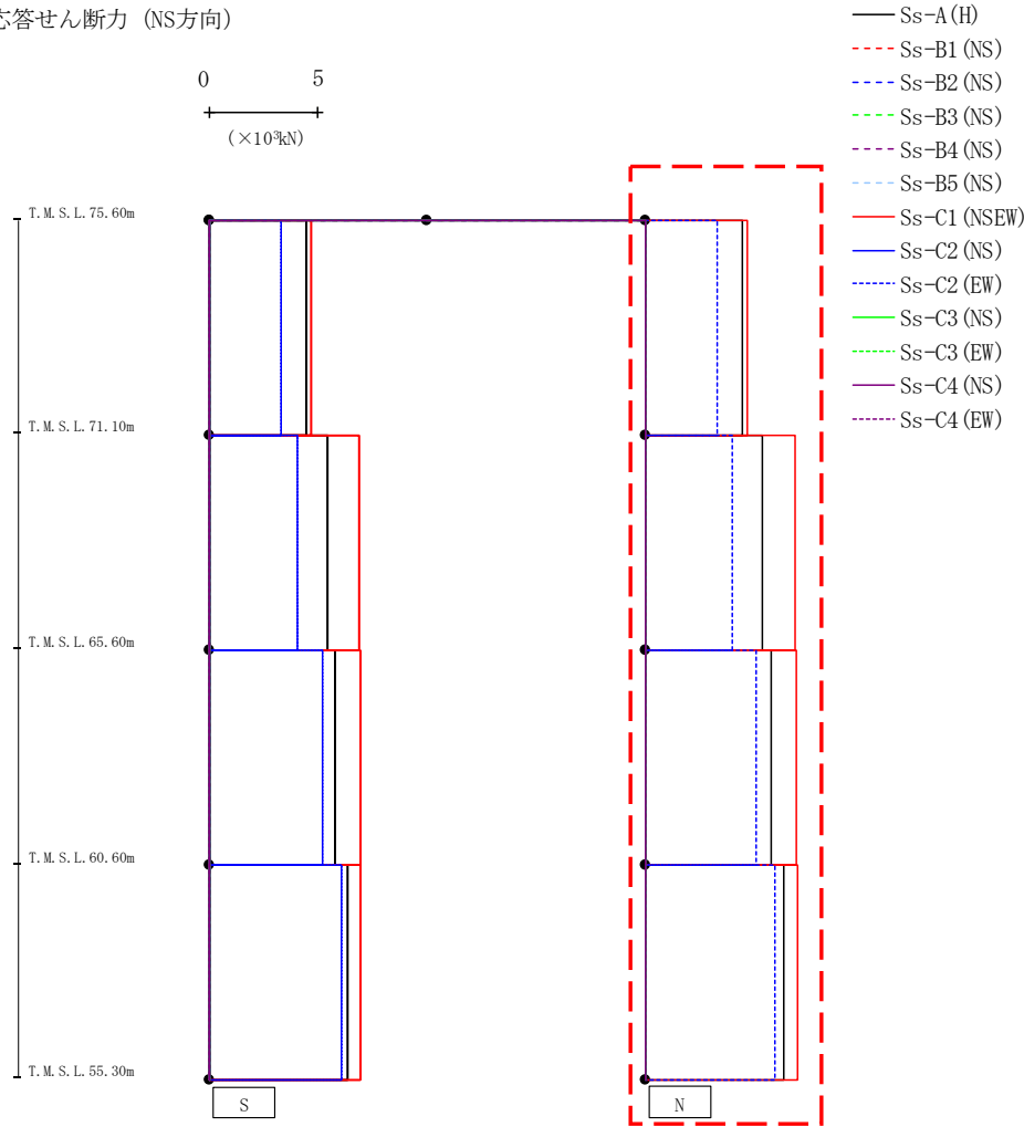
第4.2.2-18図 支持架構の最大応答せん断力(+1 \sigma 地盤, NS断面①, 有効応力解析) (2/2)
