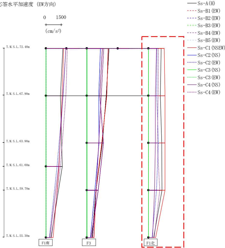
第4.2.2-33図 支持架構の最大応答加速度(G10B防護ネット架構, -1σ地盤, EW断面②) (3/3)
