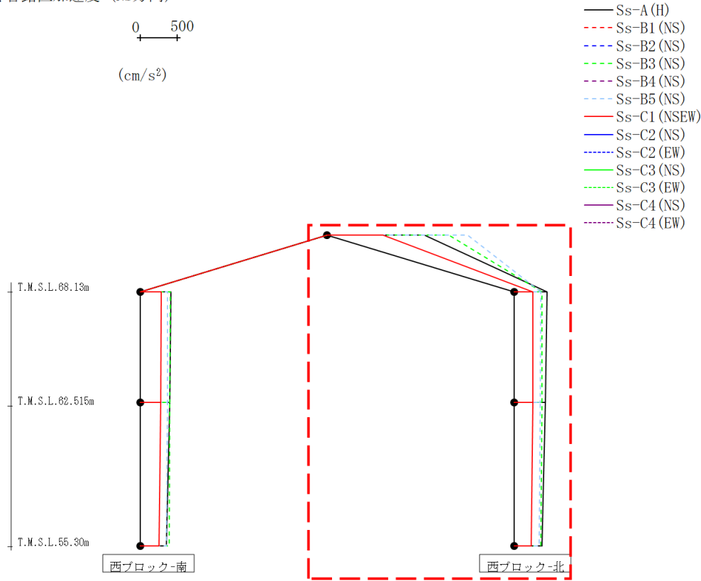
第4.2.2-64図 支持架構の最大応答鉛直加速度(-1σ地盤, NS断面①, 有効応力解析)(2/2)
