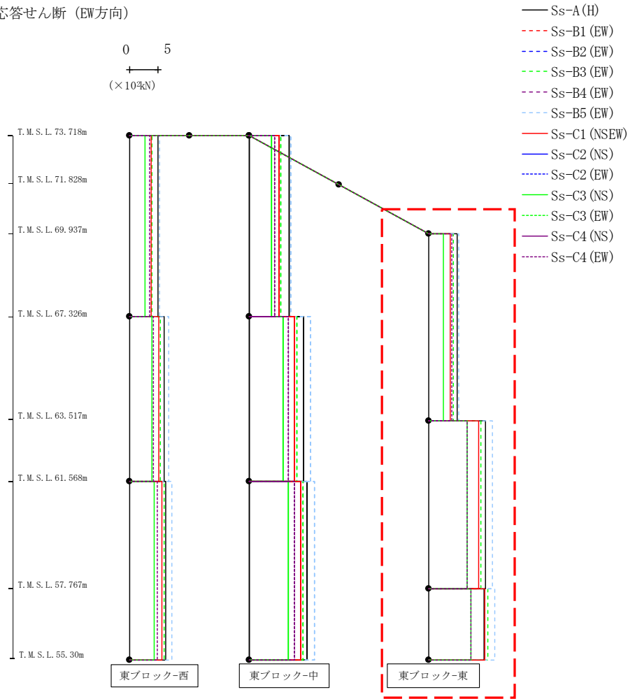
第4.2.1-22図 支持架構の最大応答せん断力(+1σ地盤, EW断面④, 全応力解析) (3/3)
