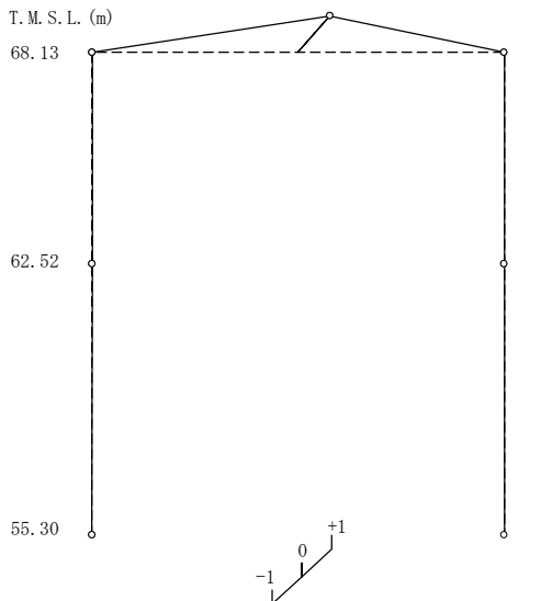
第4.1.2-2図 刺激関数図(EW方向モデル, EW断面③)(1/2)
