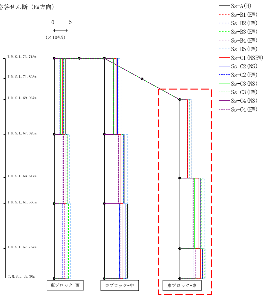
第4.2.1-66図 支持架構の最大応答せん断力(-1σ地盤, EW断面③, 有効応力解析) (3/3)
