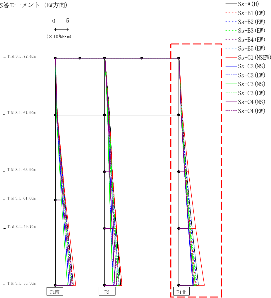
第4.2.2-7図 支持架構の最大応答曲げモーメント(G10B防護ネット架構, 基本ケース, EW断面①) (3/3)
