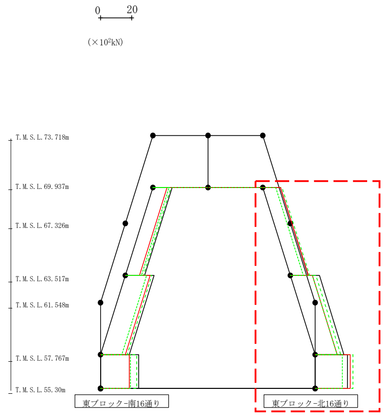
第4.2.1-26図 支持架構の最大応答せん断力(-1σ地盤, NS断面②, 全応力解析) (4/4)
