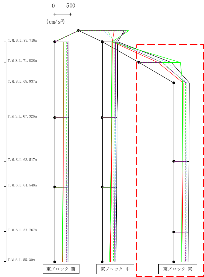
第4.2.1-36図 支持架構の最大応答鉛直加速度(-1σ地盤, EW断面④, 全応力解析) (3/3)
