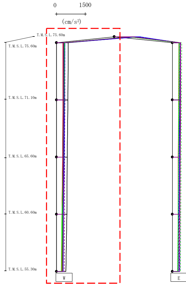
第4.2.1-16図 支持架構の最大応答鉛直加速度(基本ケース, EW断面③, 全応力解析)(1/2)
