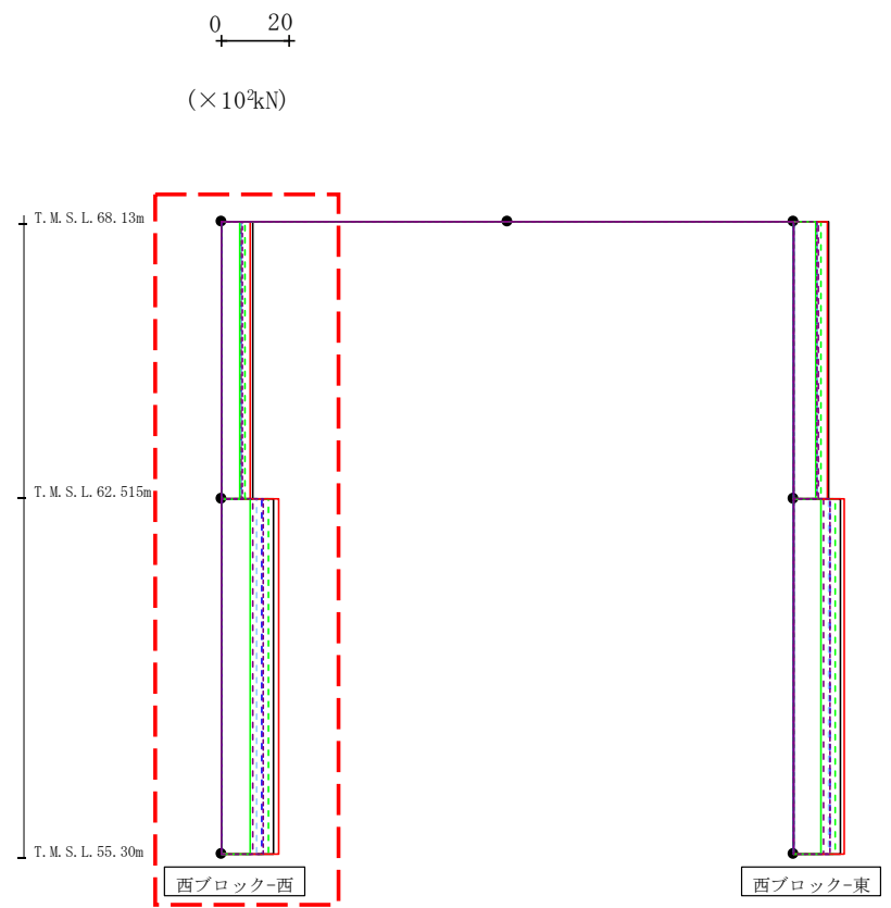
第4.2.2-58図 支持架構の最大応答せん断力(+1σ地盤, EW断面④, 有効応力解析) (1/2)
