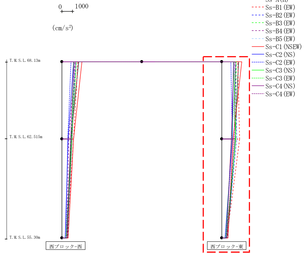
第4.2.2-41図 支持架構の最大応答加速度(基本ケース, EW断面③, 有効応力解析)(2/2)
