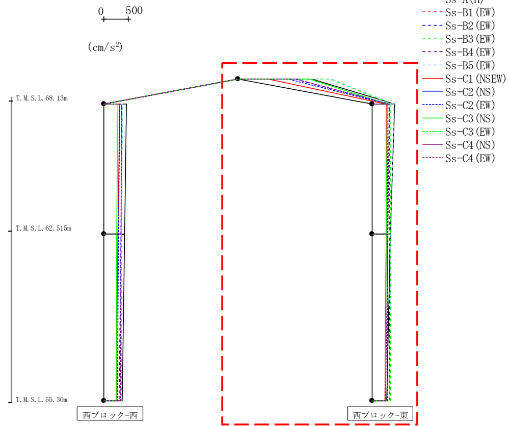
第4.2.2-68図 支持架構の最大応答鉛直加速度(-1σ地盤, EW断面③, 有効応力解析)(2/2)
