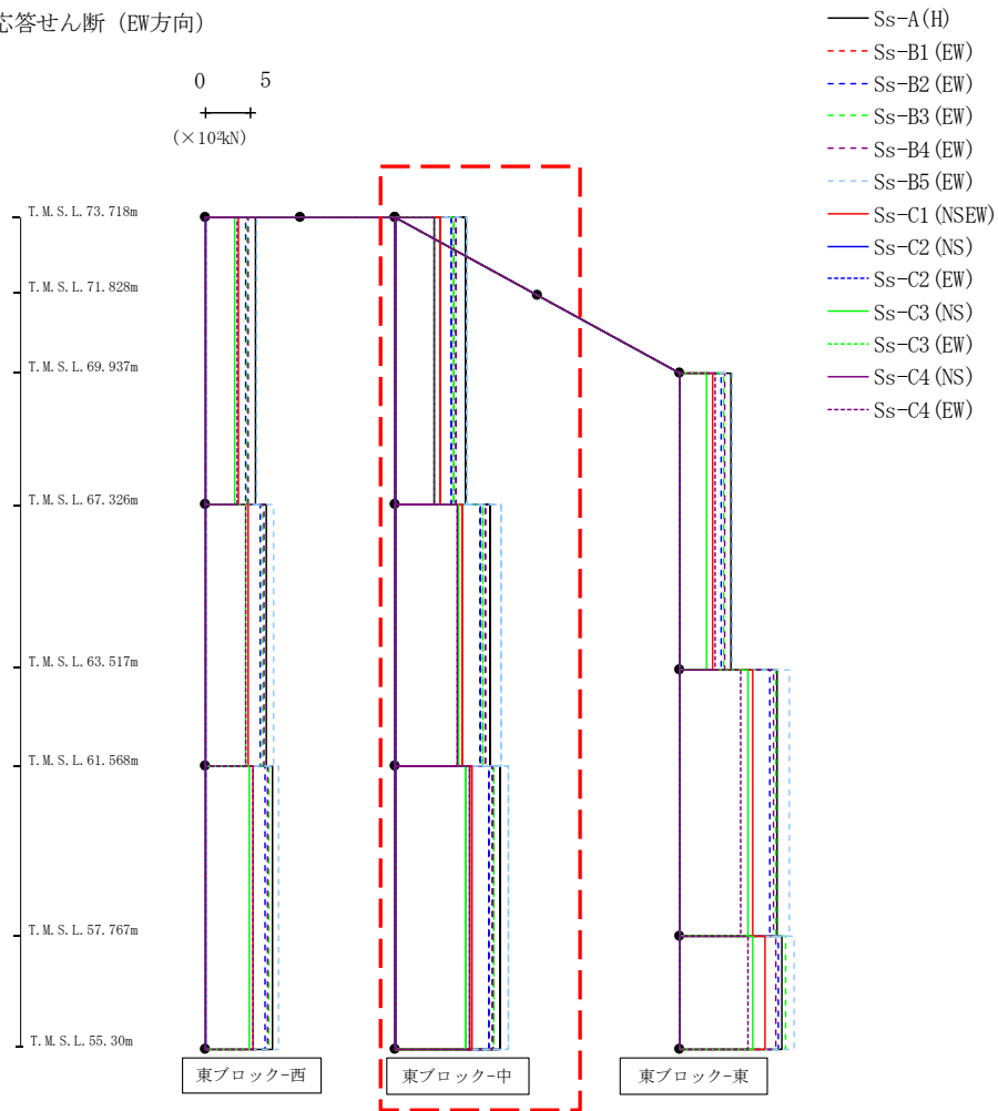
第4.2.1-70図 支持架構の最大応答せん断力(-1σ地盤, EW断面④, 有効応力解析) (2/3)
