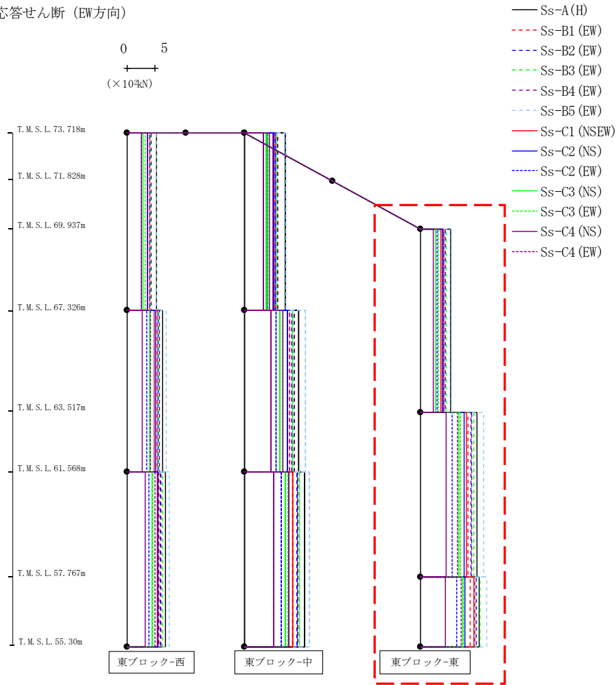
第4.2.1-46図 支持架構の最大応答せん断力(基本ケース, EW断面④, 有効応力解析)(3/3)
