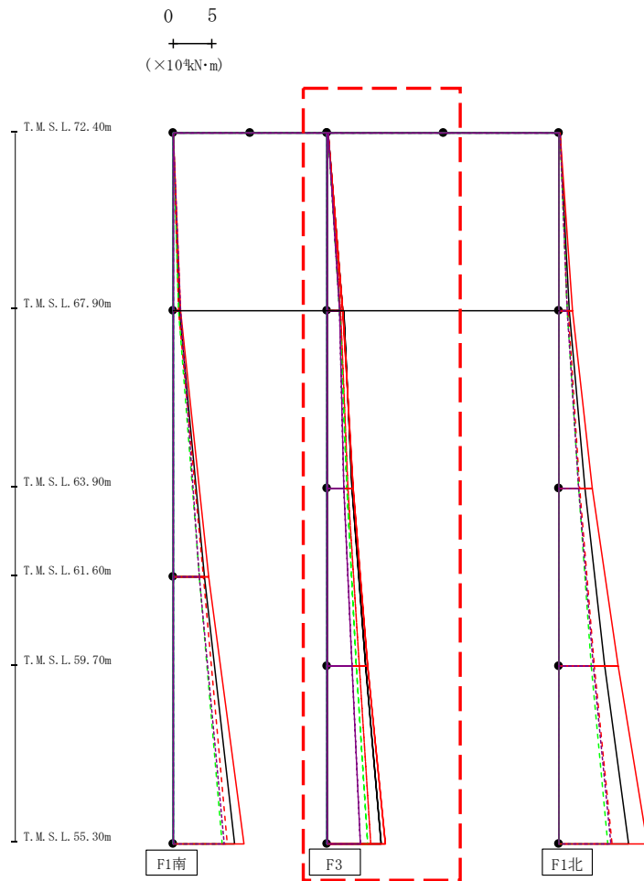
第4.2.1-35図 支持架構の最大応答曲げモーメント(G10A防護ネット架構, -1σ地盤, EW断面②) (2/3)
