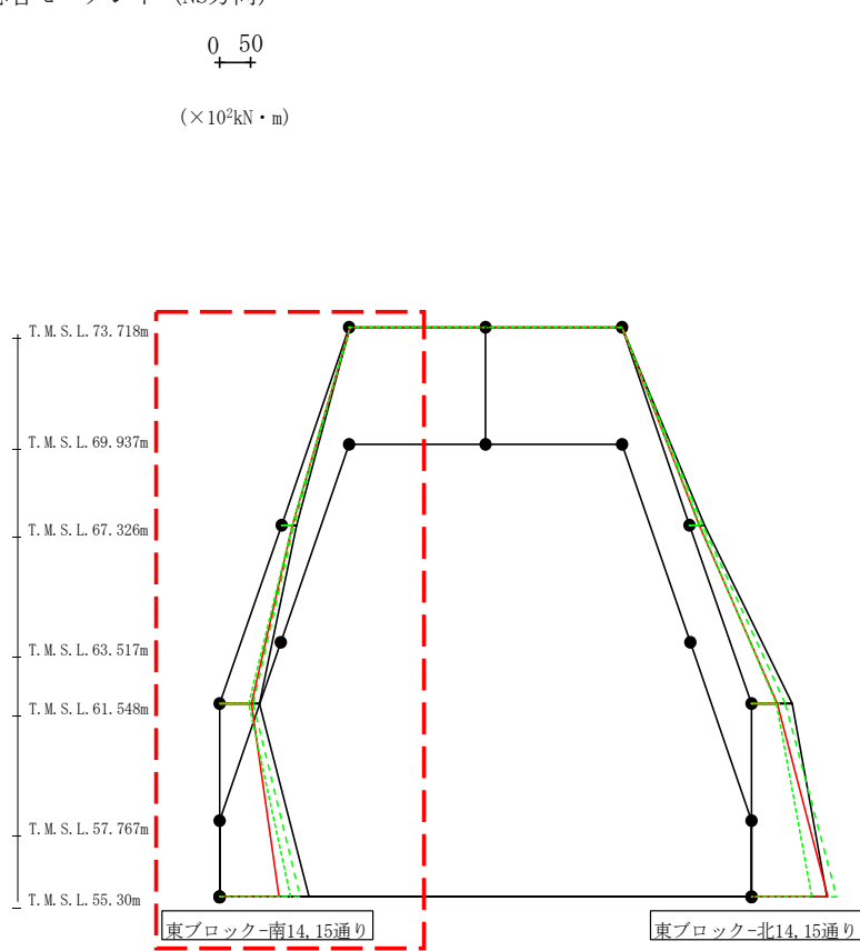
第4.2.1-27図 支持架構の最大応答曲げモーメント(-1σ地盤, NS断面②, 全応力解析)(1/4)
