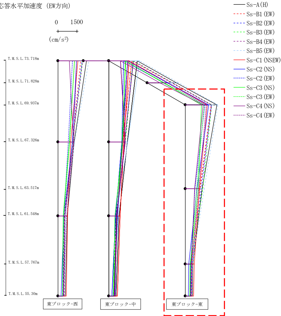
第4.2.1-9図 支持架構の最大応答加速度(基本ケース, EW断面④, 全応力解析) (3/3)
