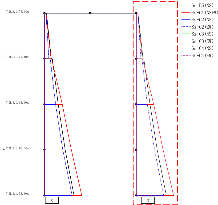
第4.2.1-19図 支持架構の最大応答曲げモーメント(+1σ地盤, NS断面①, 全応力解析)(2/2)
