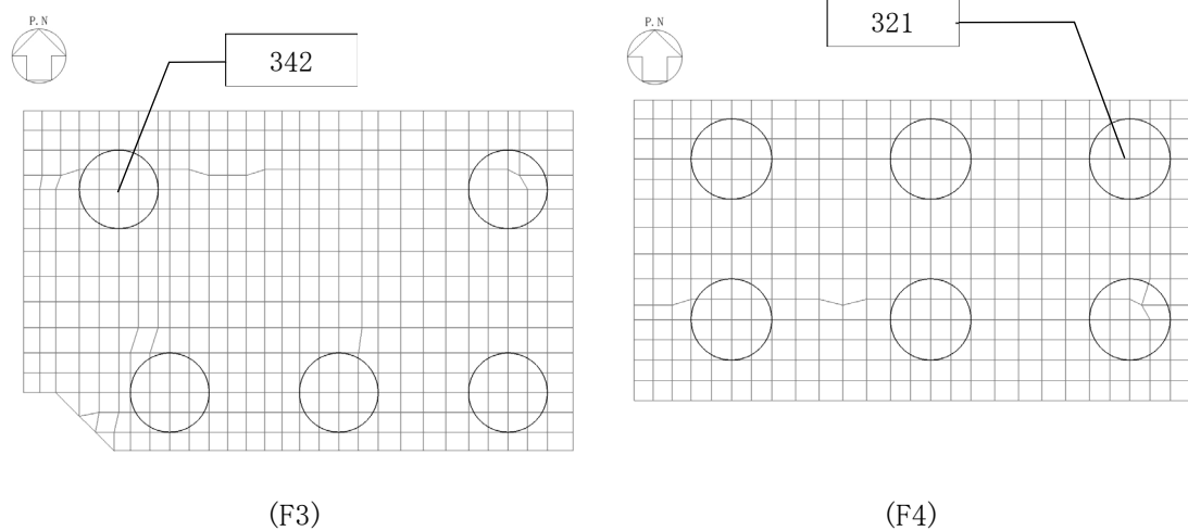
第4.3.2-1図 評価結果を記載する杭の位置
