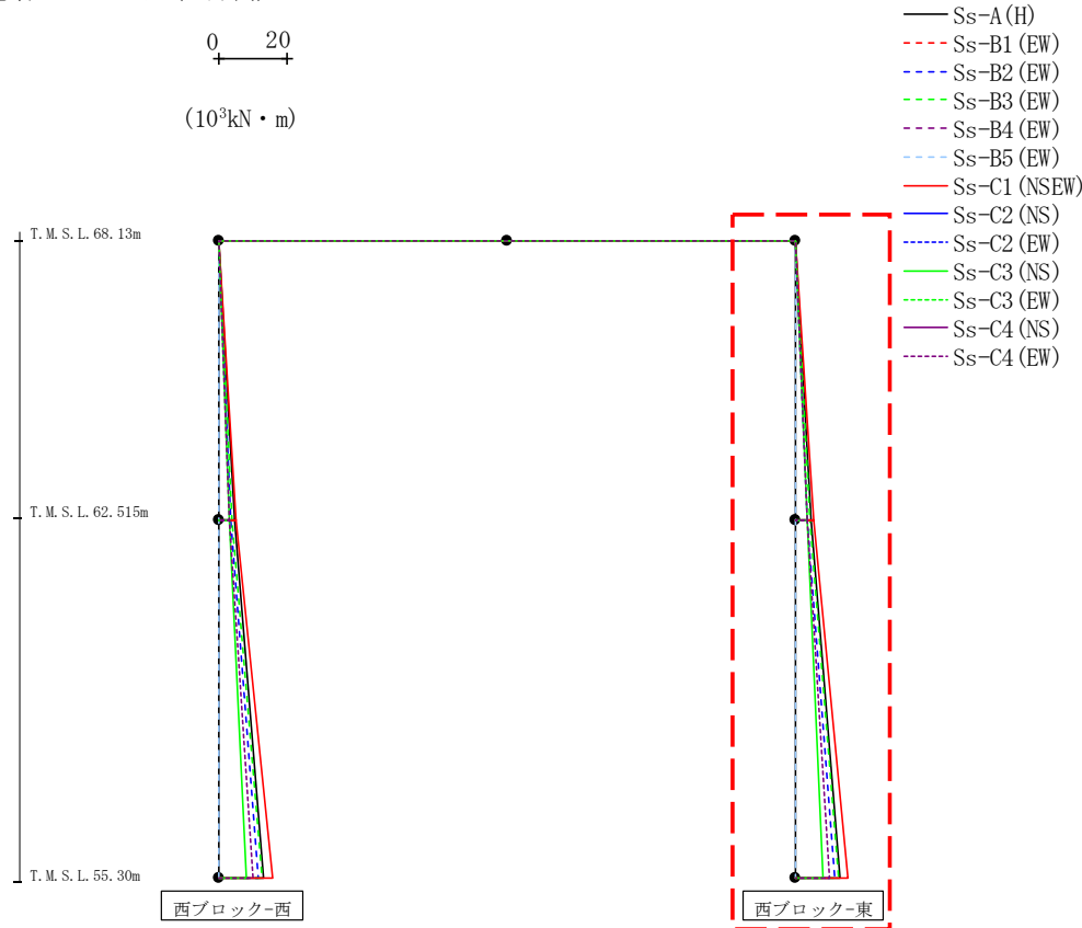
第4.2.2-19図 支持架構の最大応答曲げモーメント(+1σ地盤, EW断面③, 全応力解析) (2/2)
