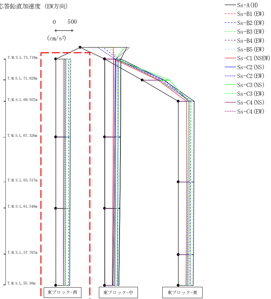
第4.2.1-68図 支持架構の最大応答鉛直加速度(-1σ地盤, EW断面③, 有効応力解析)(1/3)
