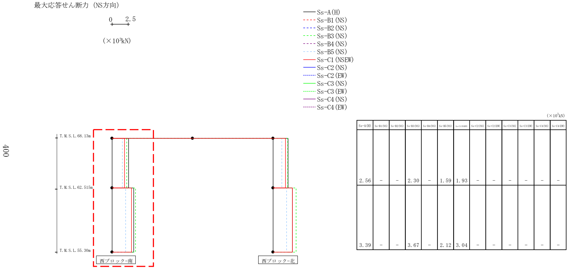
第4.2.2-26図 支持架構の最大応答せん断力(-1σ地盤, NS断面①, 全応力解析)(1/2)
