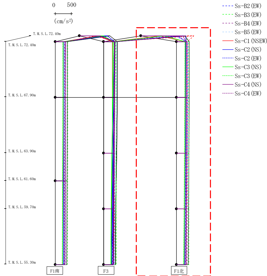
第4.2.2-8図 支持架構の最大応答鉛直加速度(G10B防護ネット架構, 基本ケース, EW断面①) (3/3)
