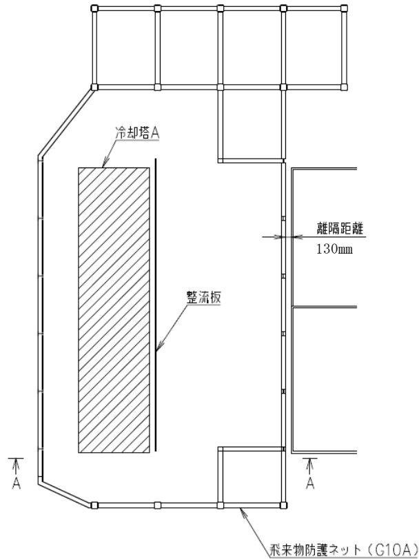
(平面)
