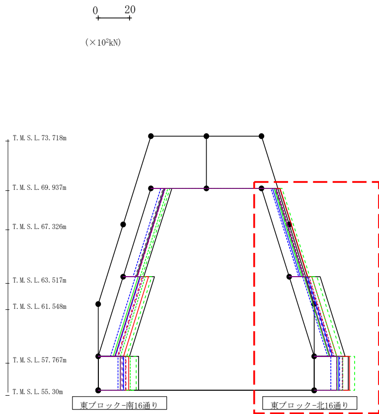
第4.2.1-38図 支持架構の最大応答せん断力(基本ケース, NS断面②, 有効応力解析)(4/4)
