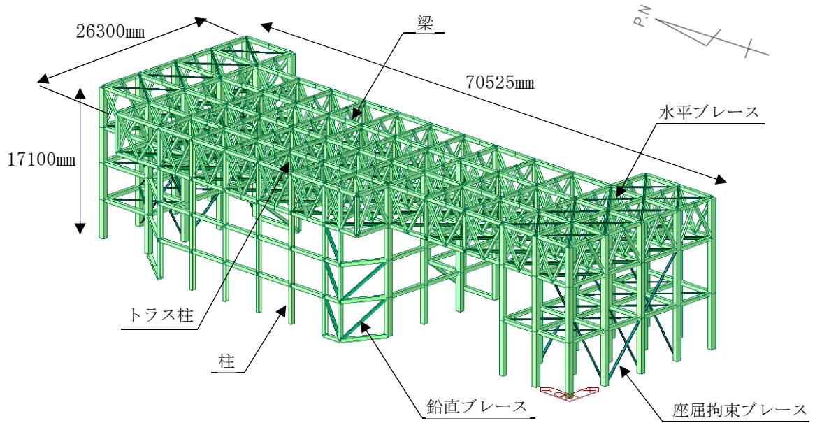
第2.2-1図 支持架構の全景(G10A防護ネット架構)
