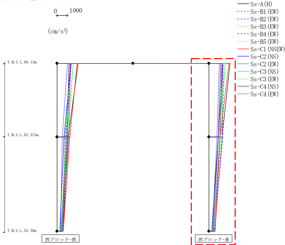
第4.2.2-45図 支持架構の最大応答加速度(基本ケース, EW断面④, 有効応力解析) (2/2)
