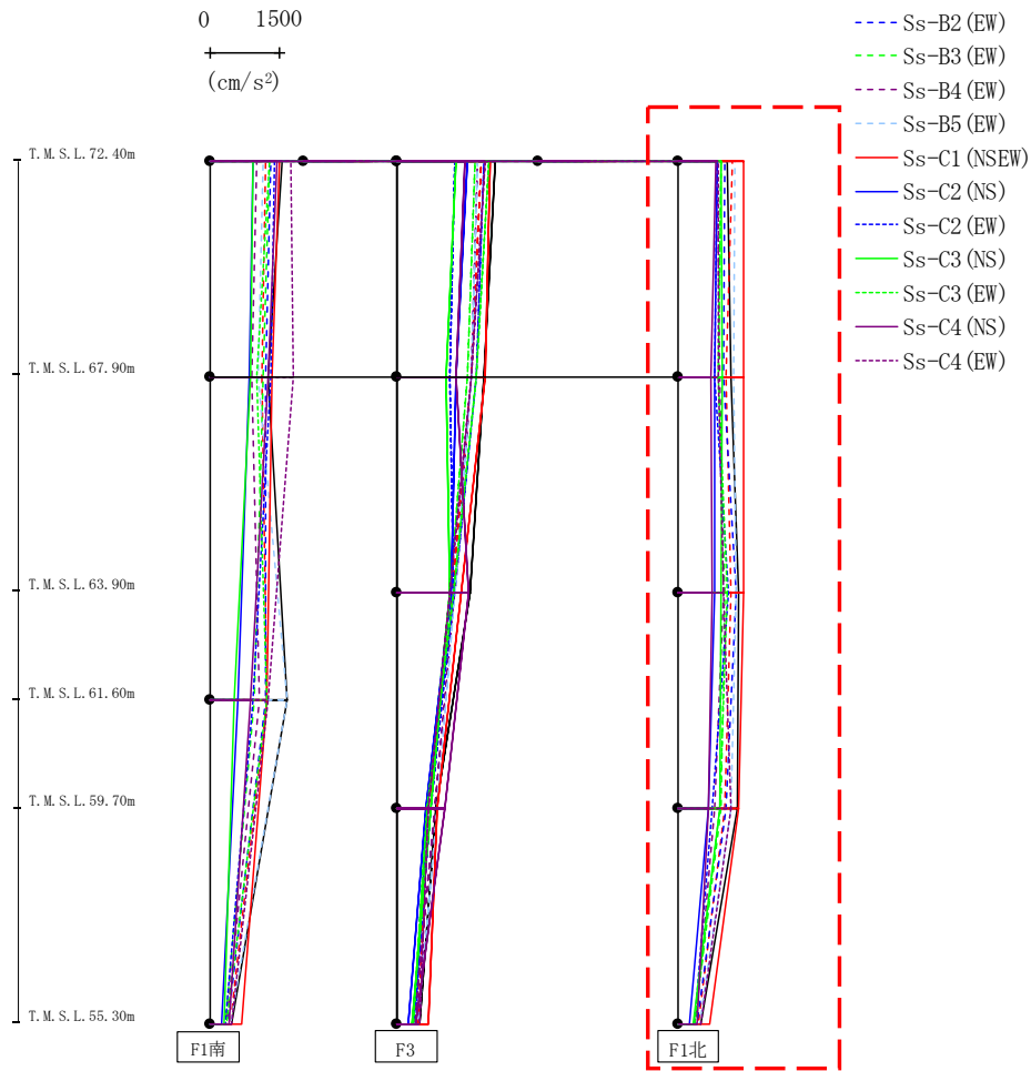
第4.2.2-5図 支持架構の最大応答加速度(G10B防護ネット架構, 基本ケース, EW断面①) (3/3)
