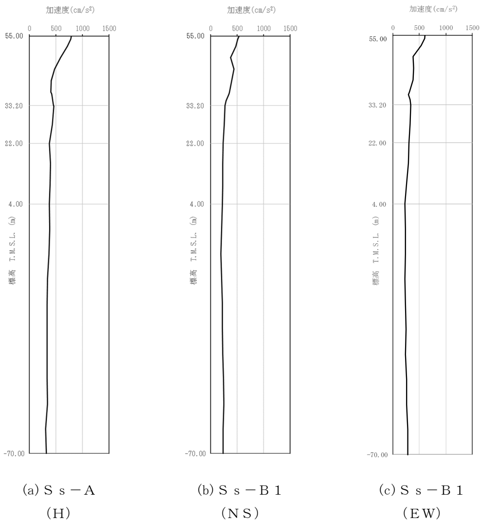
第 4-2 図 最大加速度分布 (S s) (1/8)
