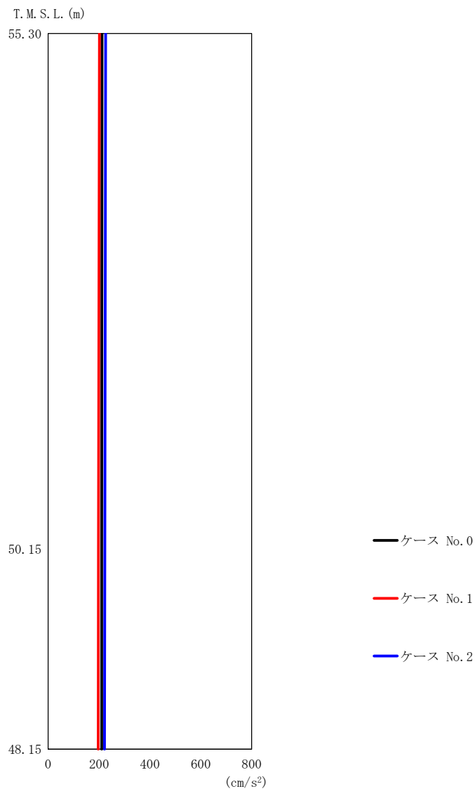
第 5.3-40 図 最大応答加速度（鉛直方向）（3/3）
