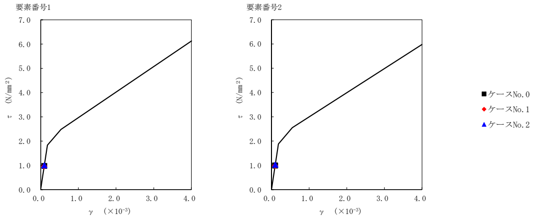
第 5.3-20 図 \tau - \gamma 関係と最大応答値 (S s - B 3 (EW) , EW 方向)
