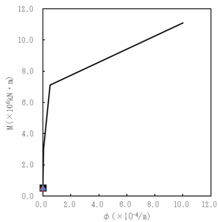
第 5.3-54 図 M- \phi 関係と最大応答値 (S d - C 4 (EW), EW 方向)
