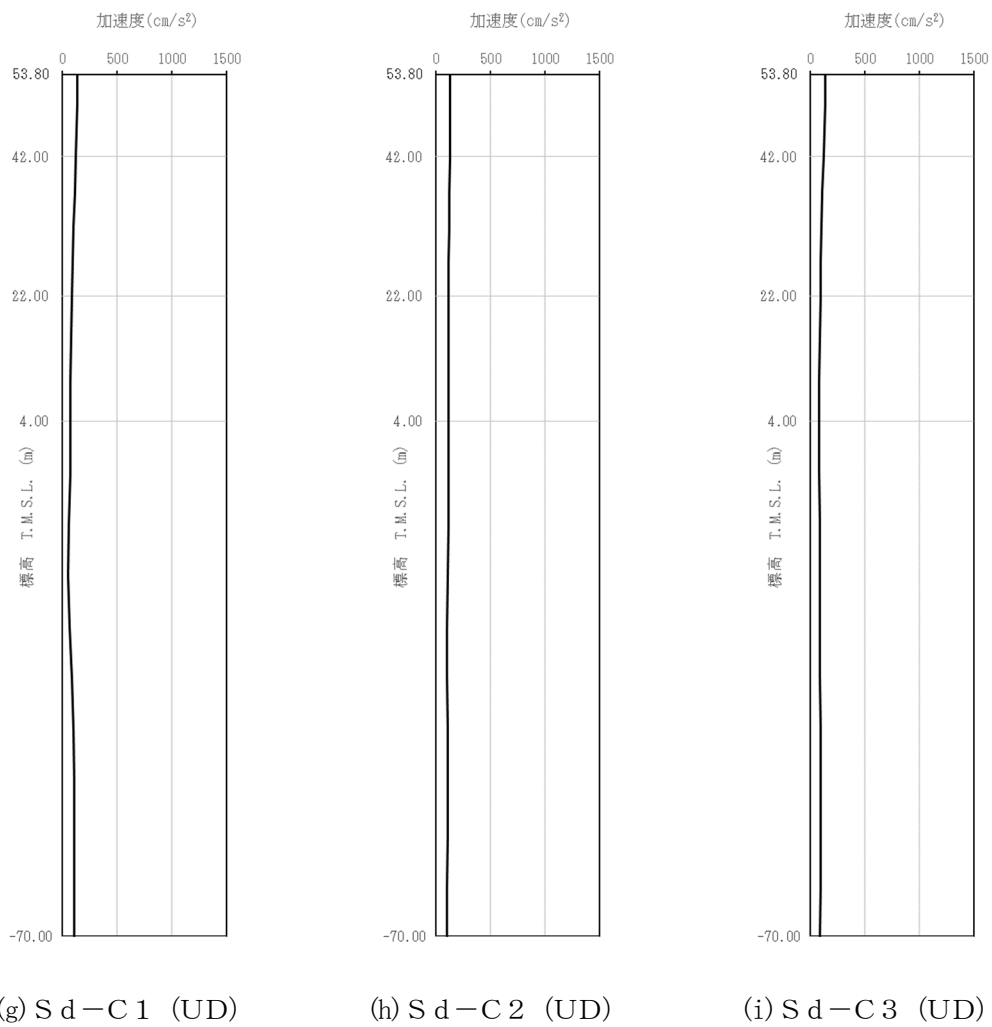
第 4-4 図 最大加速度分布 (S d) (8/8)
