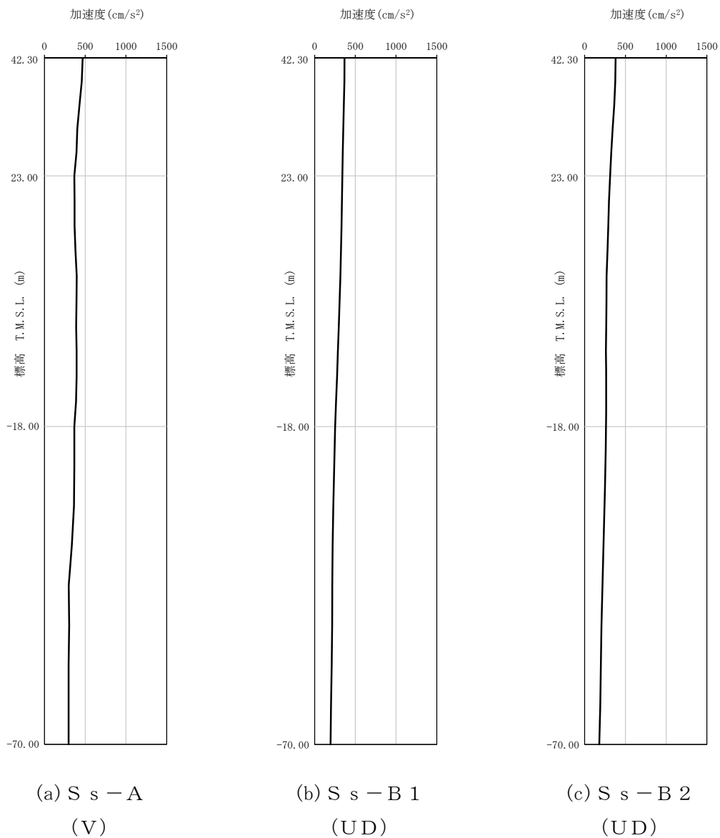
第 4-2 図 最大加速度分布 (S s) (6/8)
