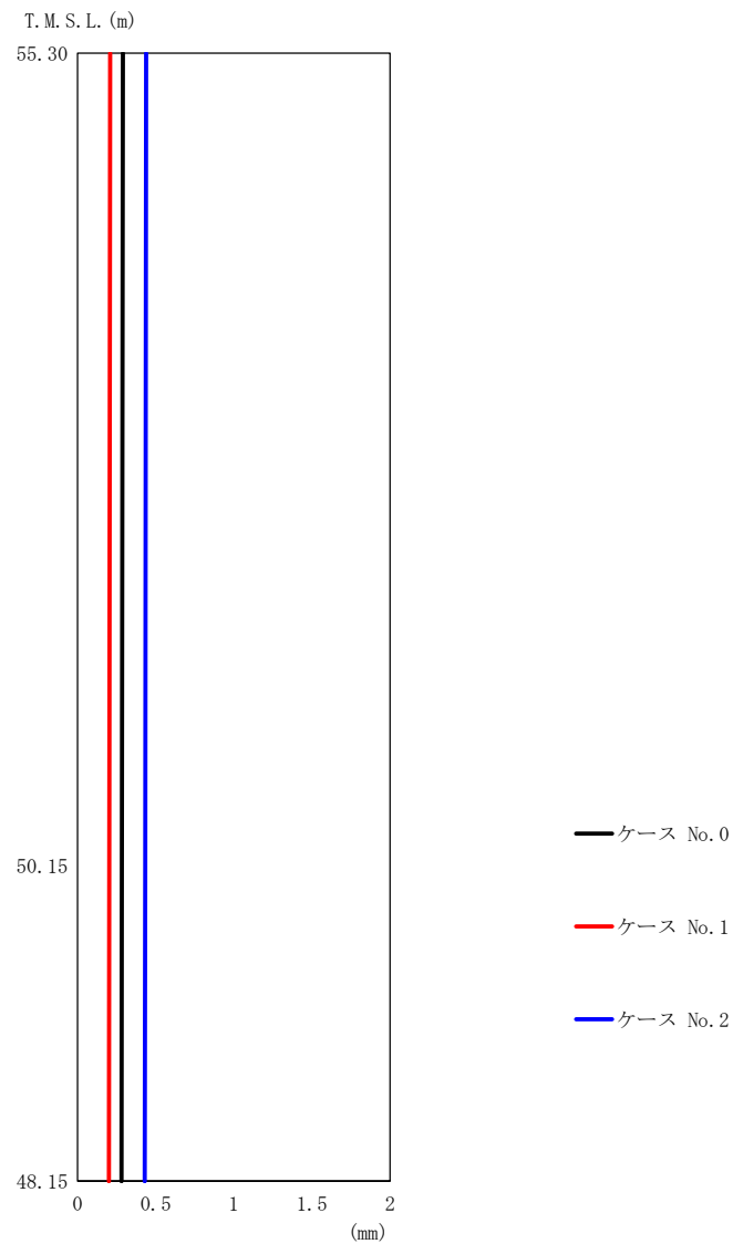
第 5.3-41 図 最大応答変位 (鉛直方向) (2/3)
