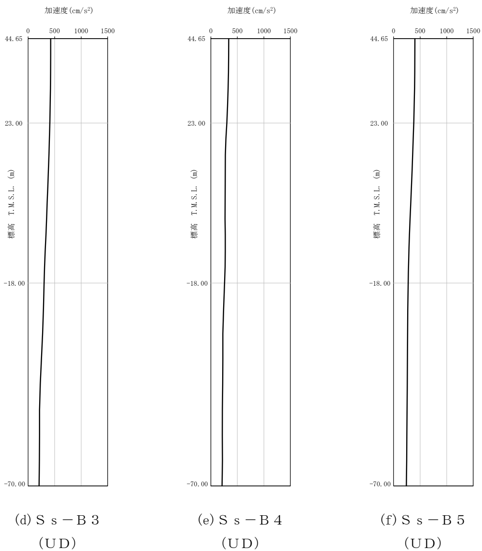
第4-2図 最大加速度分布 (S s ) (7/8)
