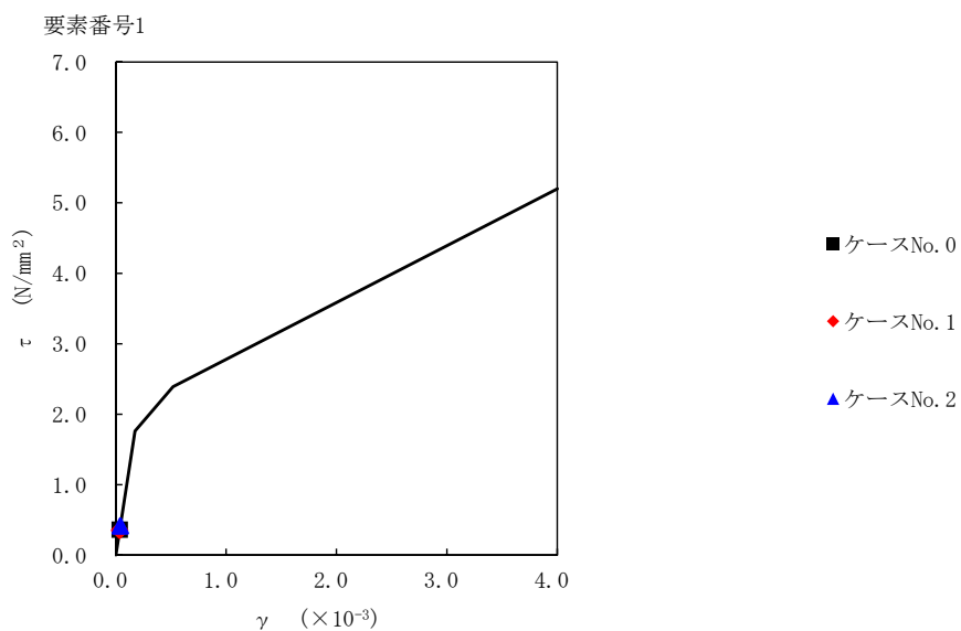
第5.3-26図 τ-γ関係と最大応答値 (S s -C4 (EW), EW方向)
