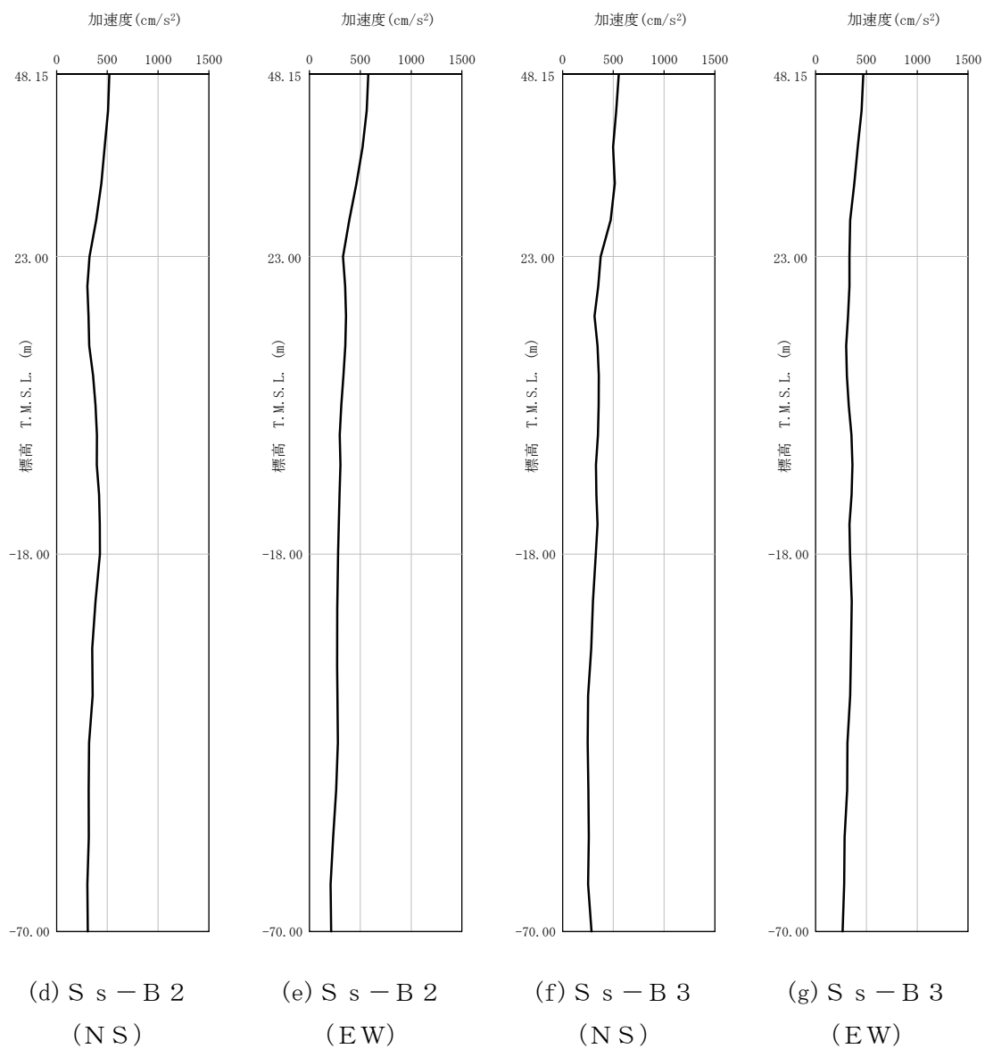
第 4-3 図 最大加速度分布 (S s ) (2/8)
