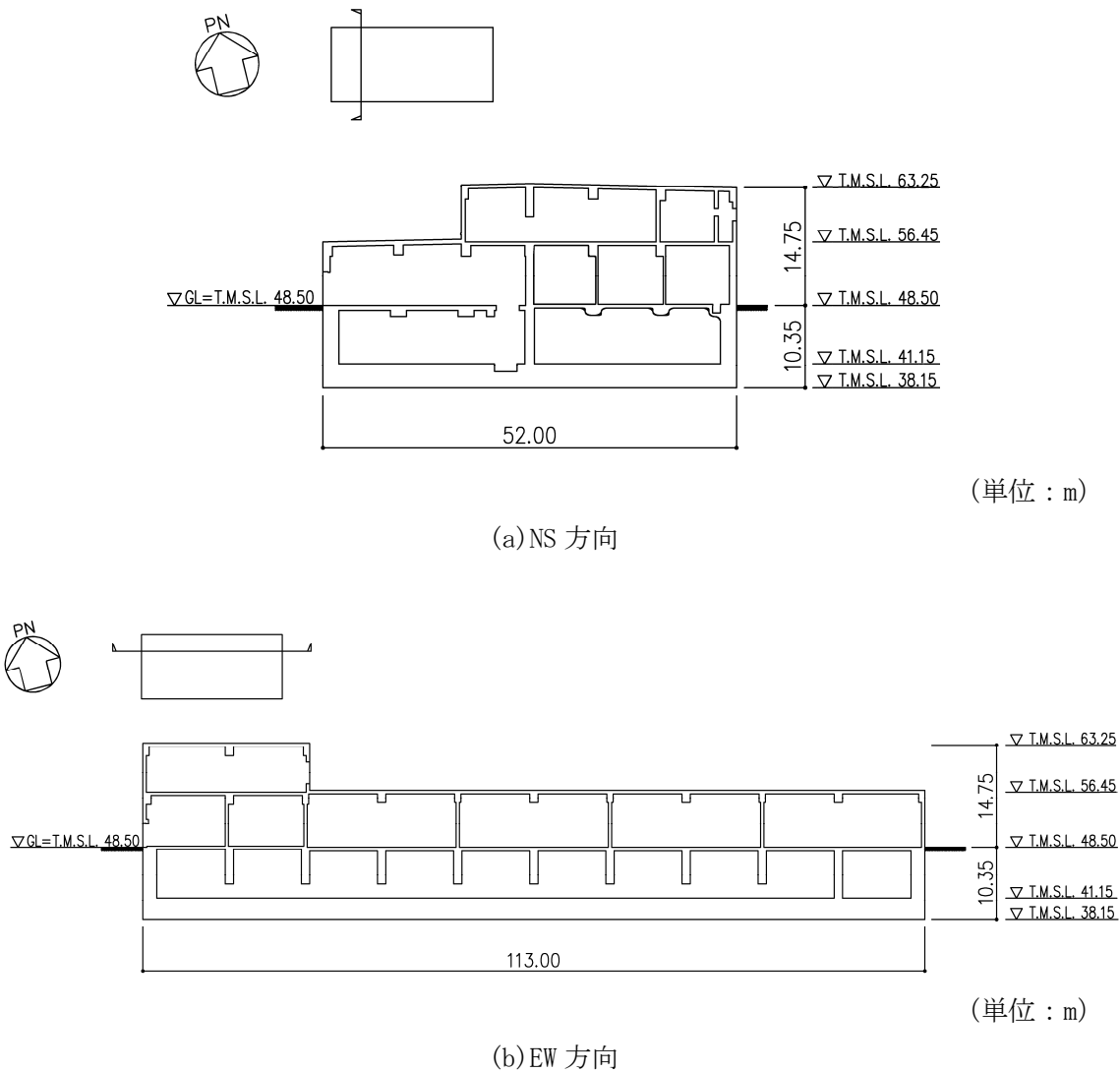
第 2.2-5 図 概略断面図
