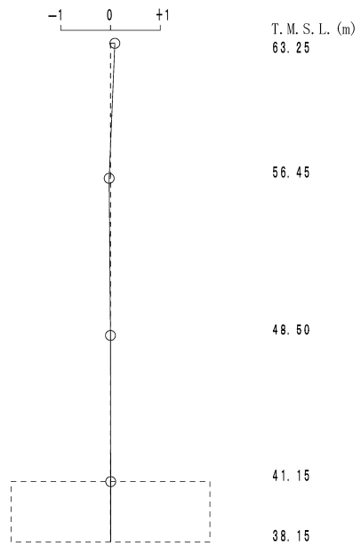
第 5.1-1 図 刺激関数図 (NS 方向)
