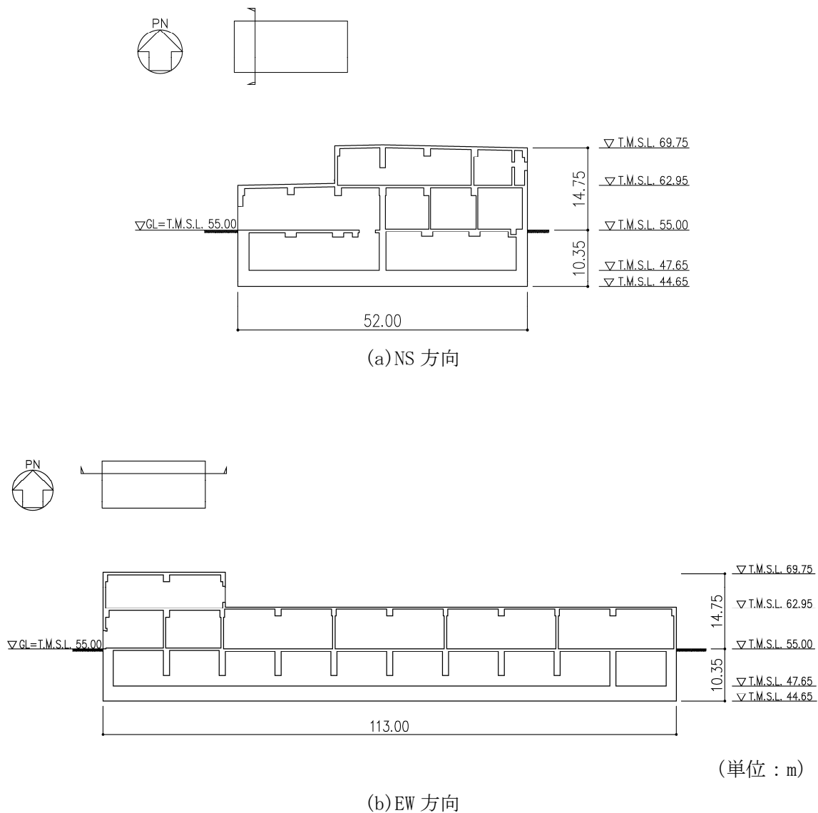
第 2.2-5 図 概略断面図
