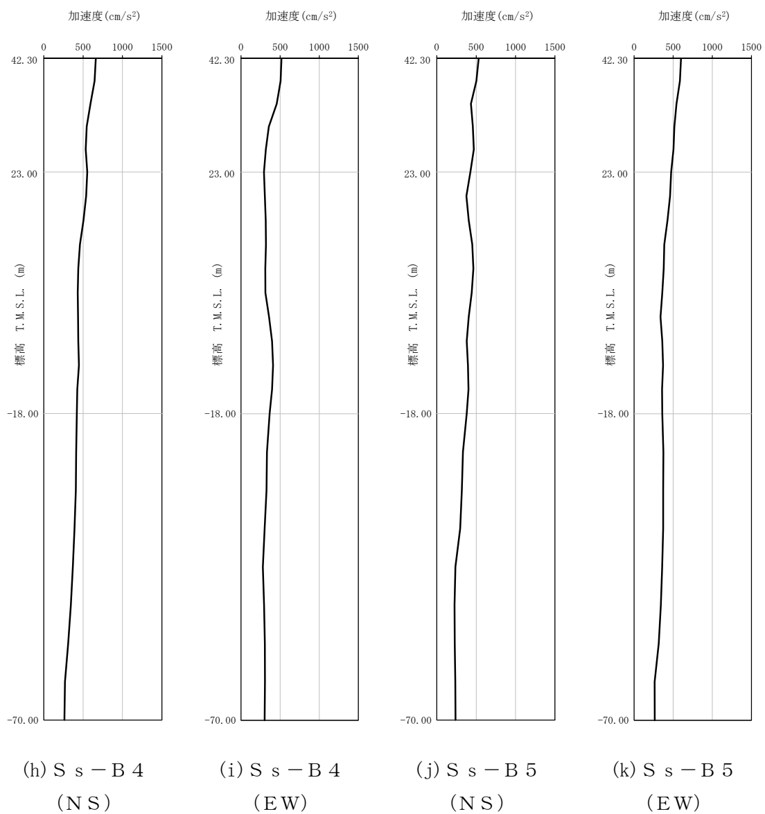
第 4-2 図 最大加速度分布 (S s ) (3/8)
