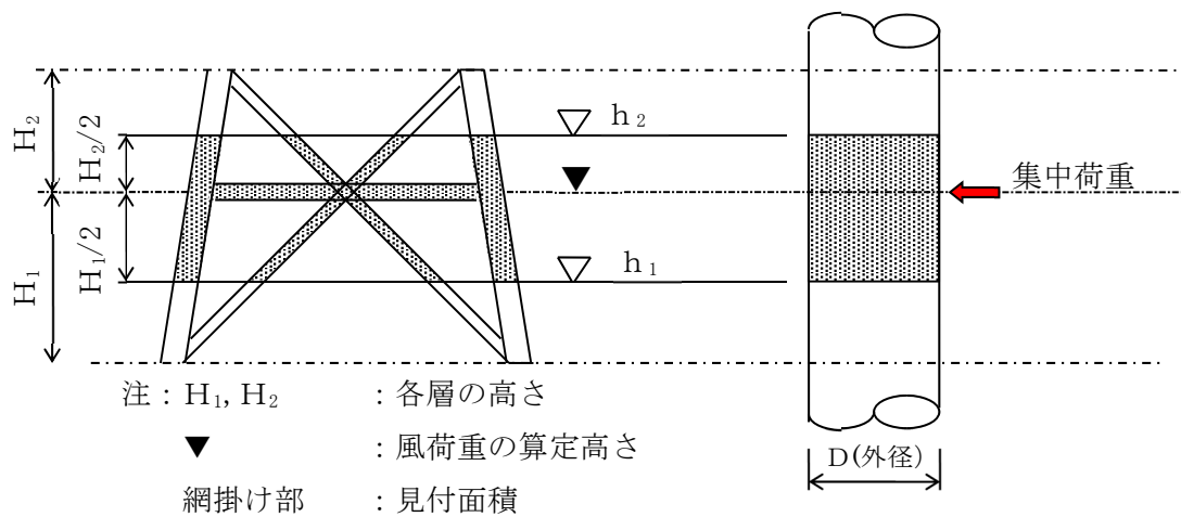
第 3.1-2 図 見付面積と風荷重の算定高さ
