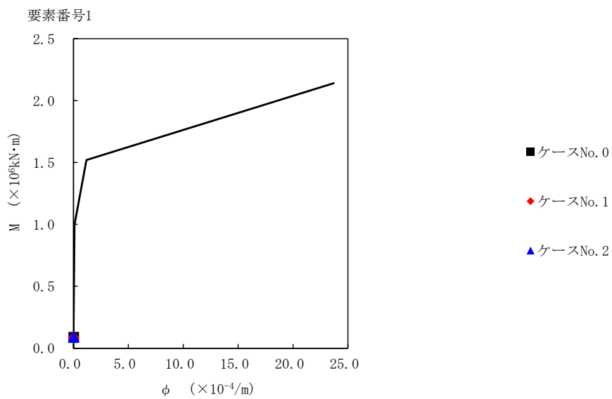
第 5.3-40 図 M-φ 関係と最大応答値 (S d-A (H), NS 方向)
