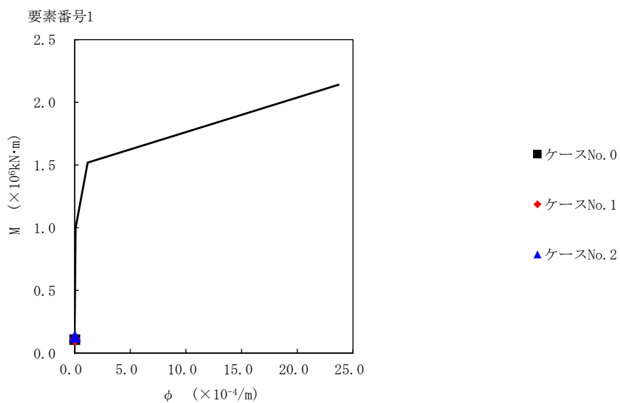
第5.3-27図 M-φ関係と最大応答値 (S s -C4 (EW), EW方向)
