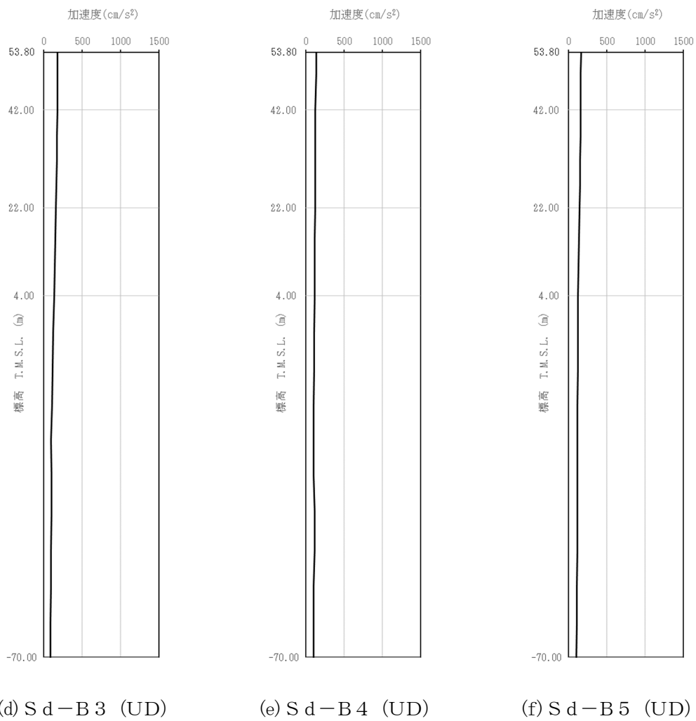
第 4-4 図 最大加速度分布 (S d) (7/8)
