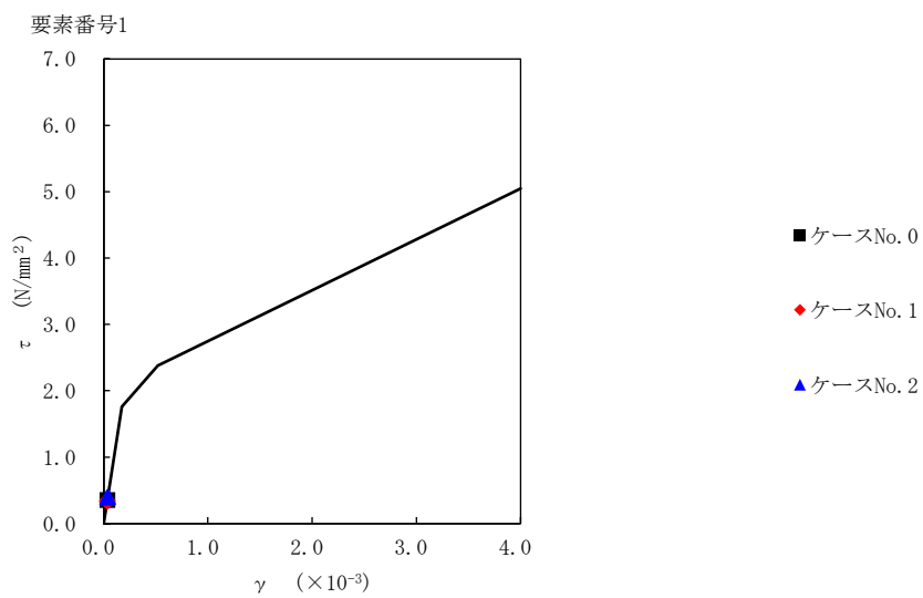
第 5.3-30 図 τ-γ 関係と最大応答値 (S s -C4 (EW), EW 方向)
