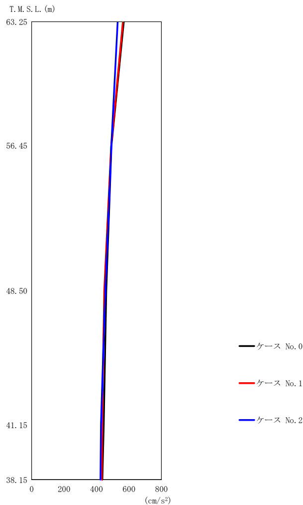
第 5.3-9 図 最大応答加速度（鉛直方向）（1/3）
