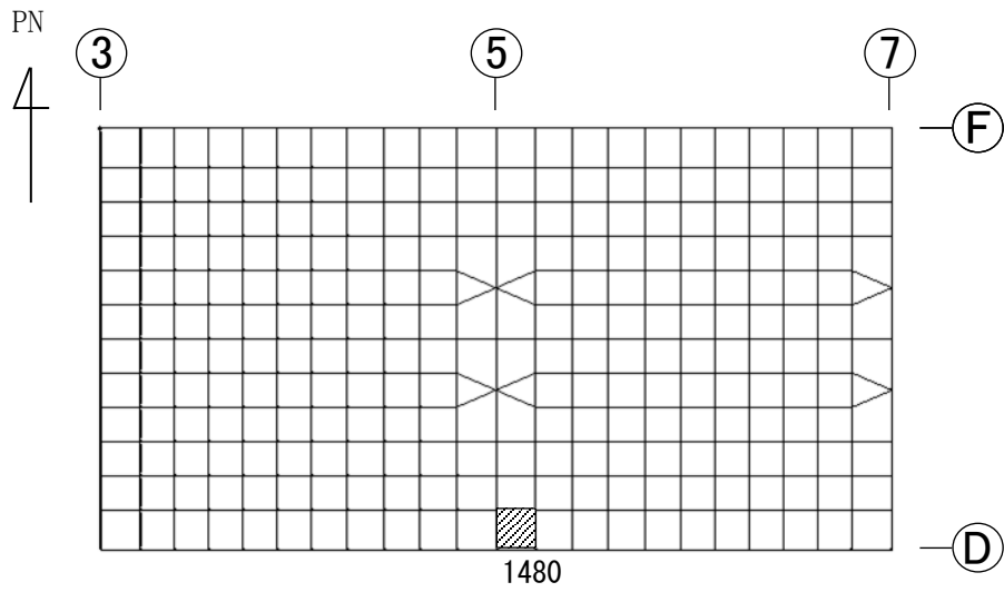
(a) NS方向 (T. M. S. L. ■■■m, 要素No. 1480)
