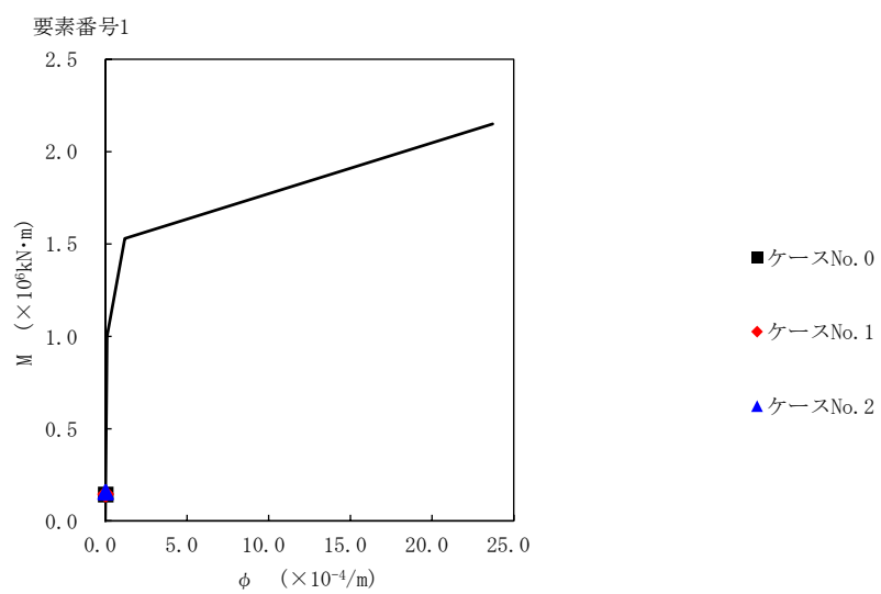
第 5.3-19 図 M-φ 関係と最大応答値 (S s -C4 (NS), NS 方向)
