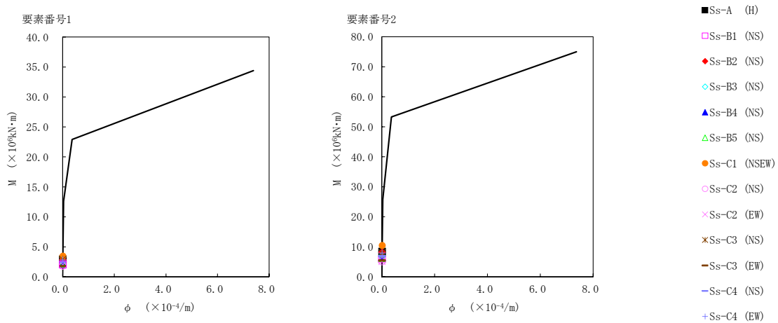
第 5.2-13 図 M - \phi 関係と最大応答値 (基準地震動 S_s , ケース No. 0, NS 方向)
