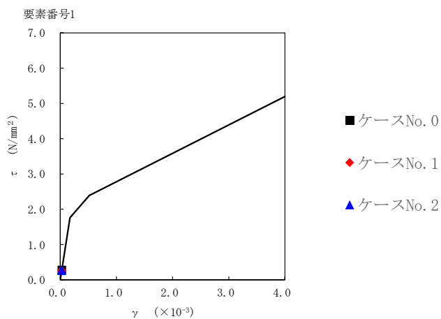
第 5.3-24 図 τ-γ 関係と最大応答値 (S s -B3 (EW), EW 方向)
