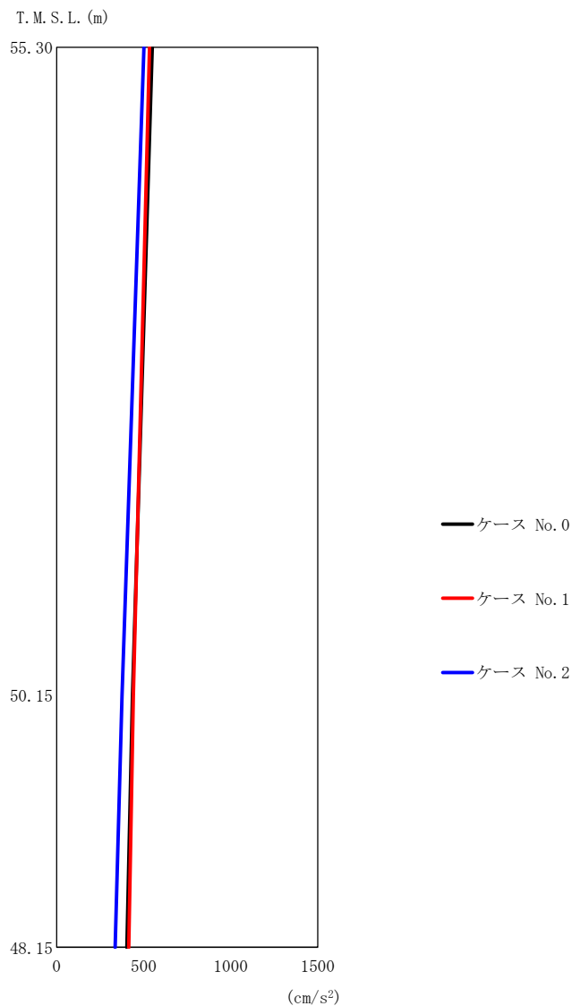
第 5.3-32 図 最大応答加速度 (NS 方向) (4/5)
