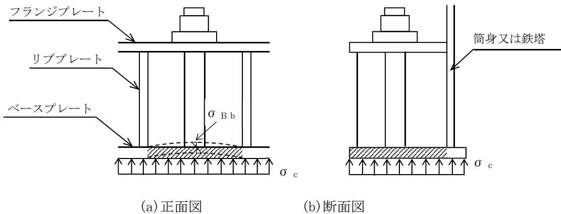
第3.2-2図 ベースプレート応力算定説明図
