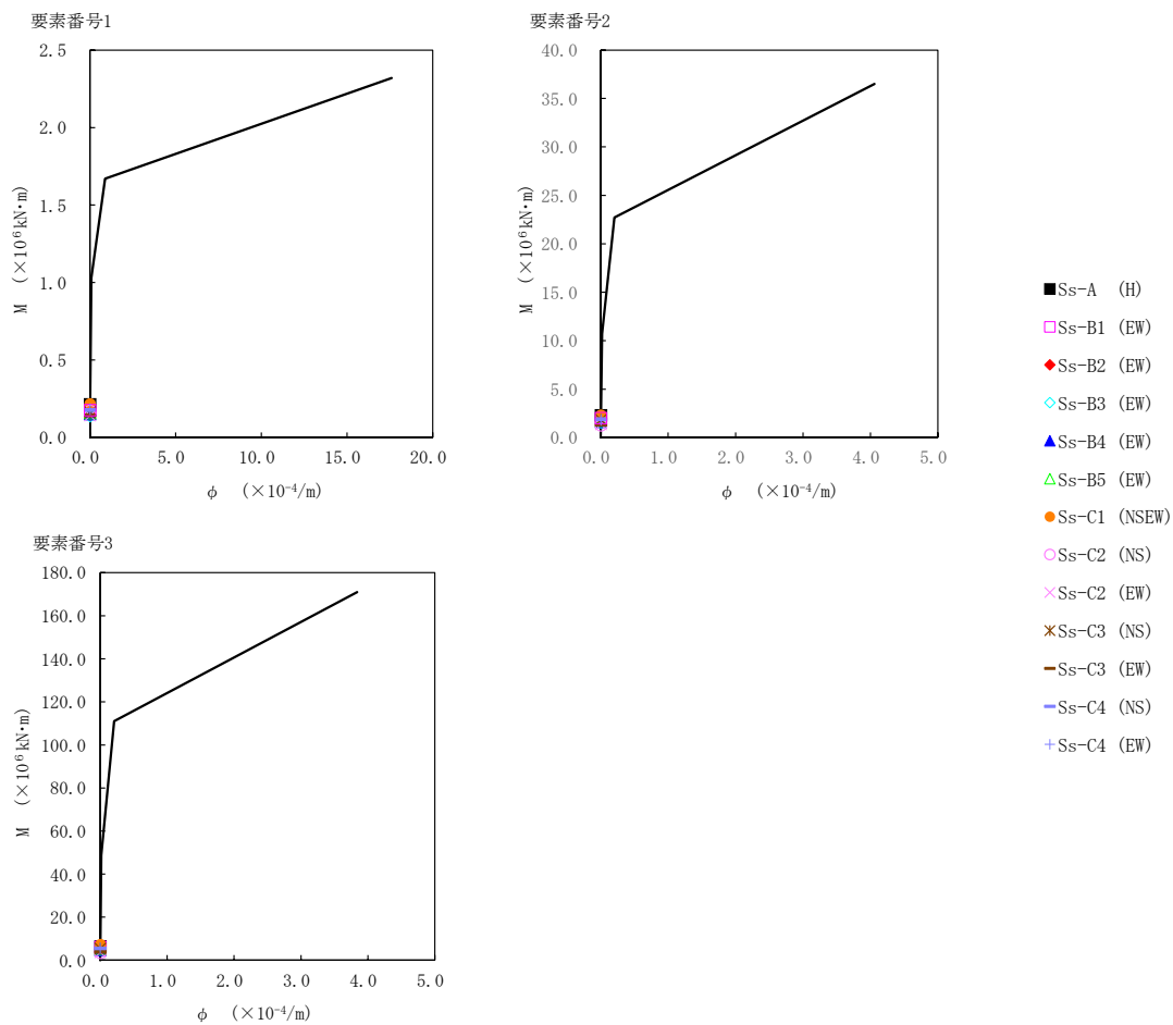
第5.2-15図 M-φ関係と最大応答値(基準地震動S s , ケースNo.0, EW方向)
