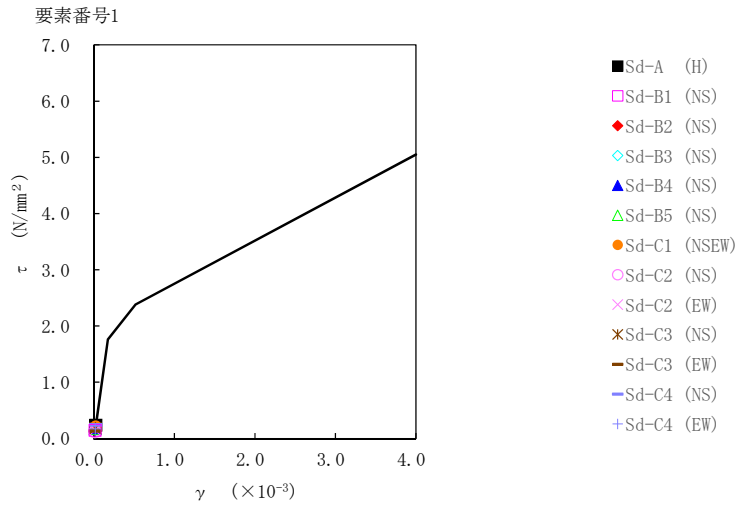
第5.2-27 図 \tau - \gamma 関係と最大応答値 (弾性設計用地震動 S d, ケース No. 0, NS 方向)
