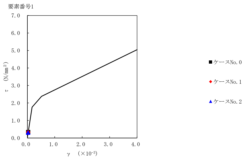
第 5.3-18 図 τ-γ 関係と最大応答値 (S s -C4 (NS), NS 方向)
