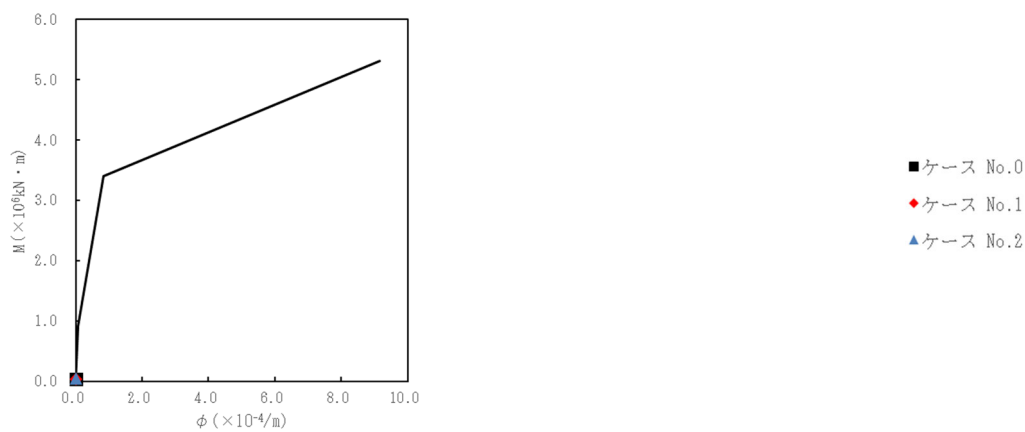
第 5.3-32 図 M-φ 関係と最大応答値 (S d - A (H) , NS 方向)
