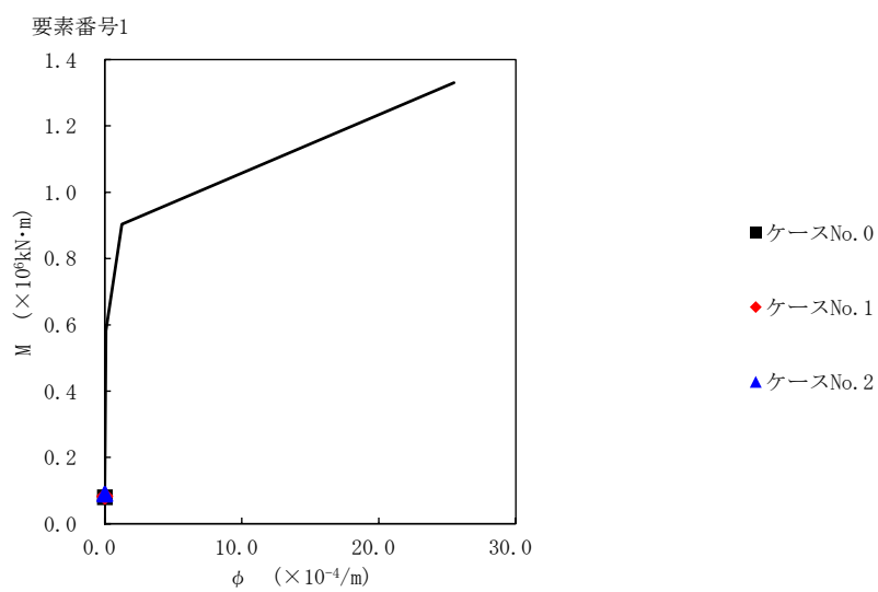
第 5.3-52 図 M-φ 関係と最大応答値 (S d - A (H) , EW 方向)
