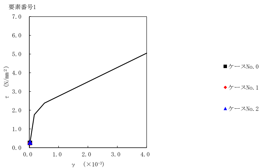
第 5.3-20 図 τ-γ 関係と最大応答値 (S s -C4 (EW), NS 方向)
