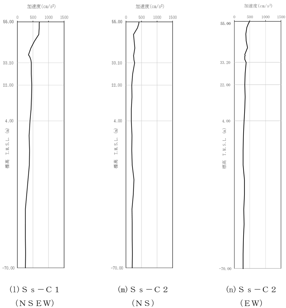
第 4-2 図 最大加速度分布 (S s ) (4/8)
