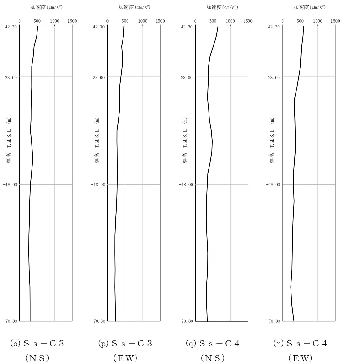
第 4-2 図 最大加速度分布 (S s ) (5/8)
