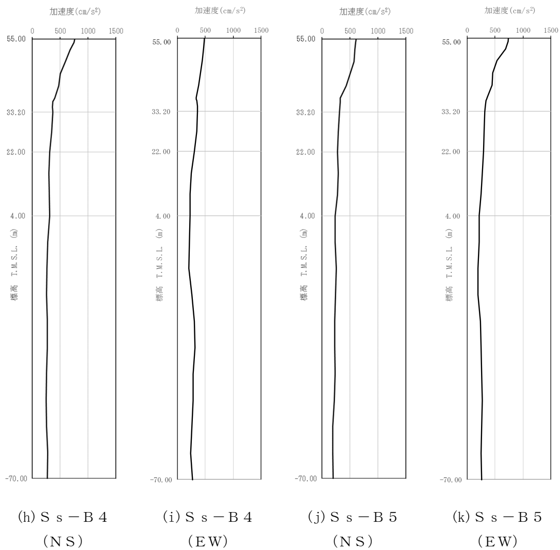
第4-2図 最大加速度分布 ( S_s ) (3/8)
