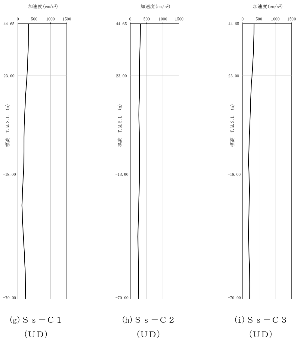
第4-2図 最大加速度分布 (S s ) (8/8)
