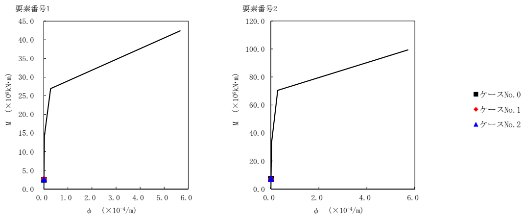
第 5.3-21 図 M - \phi 関係と最大応答値 (S s - B 3 (EW) , EW 方向)
