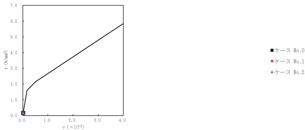
第 5.3-12 図 τ-γ 関係と最大応答値 (S s - A (H) , NS 方向)
