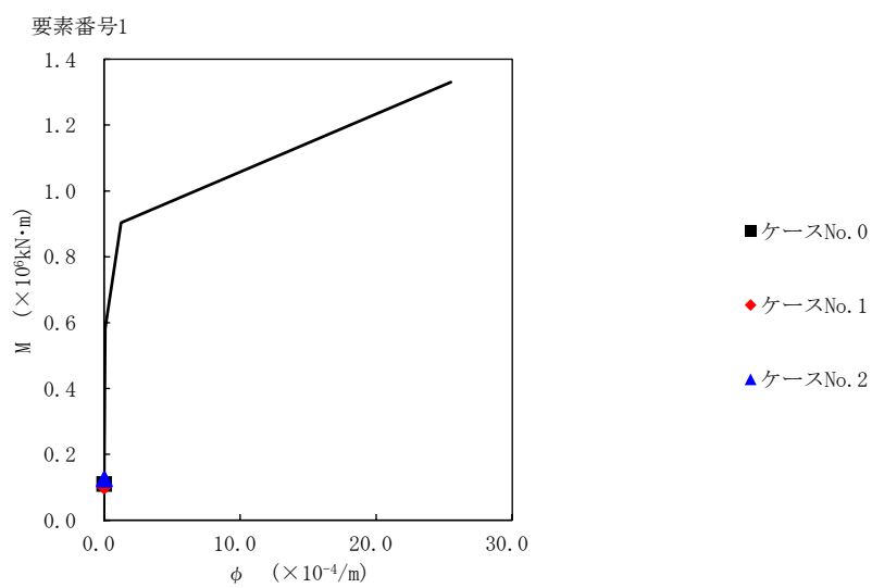
第 5.3-31 図 M-φ 関係と最大応答値 (S s -C4 (EW), EW 方向)
