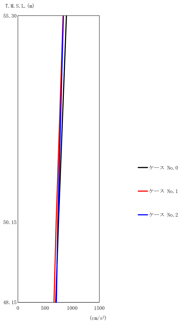
第 5.3-5 図 最大応答加速度 (EW 方向) (2/5)
