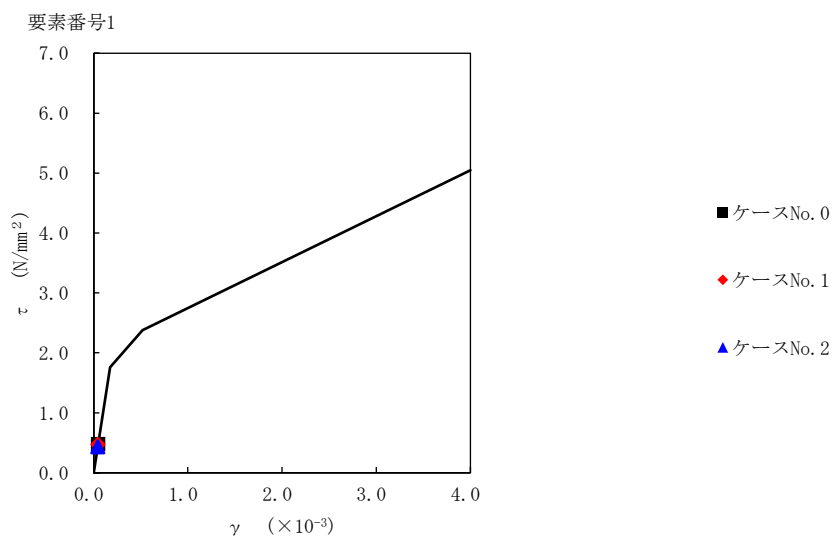
第 5.3-28 図 τ-γ 関係と最大応答値 (S s -C4 (NS), EW 方向)
