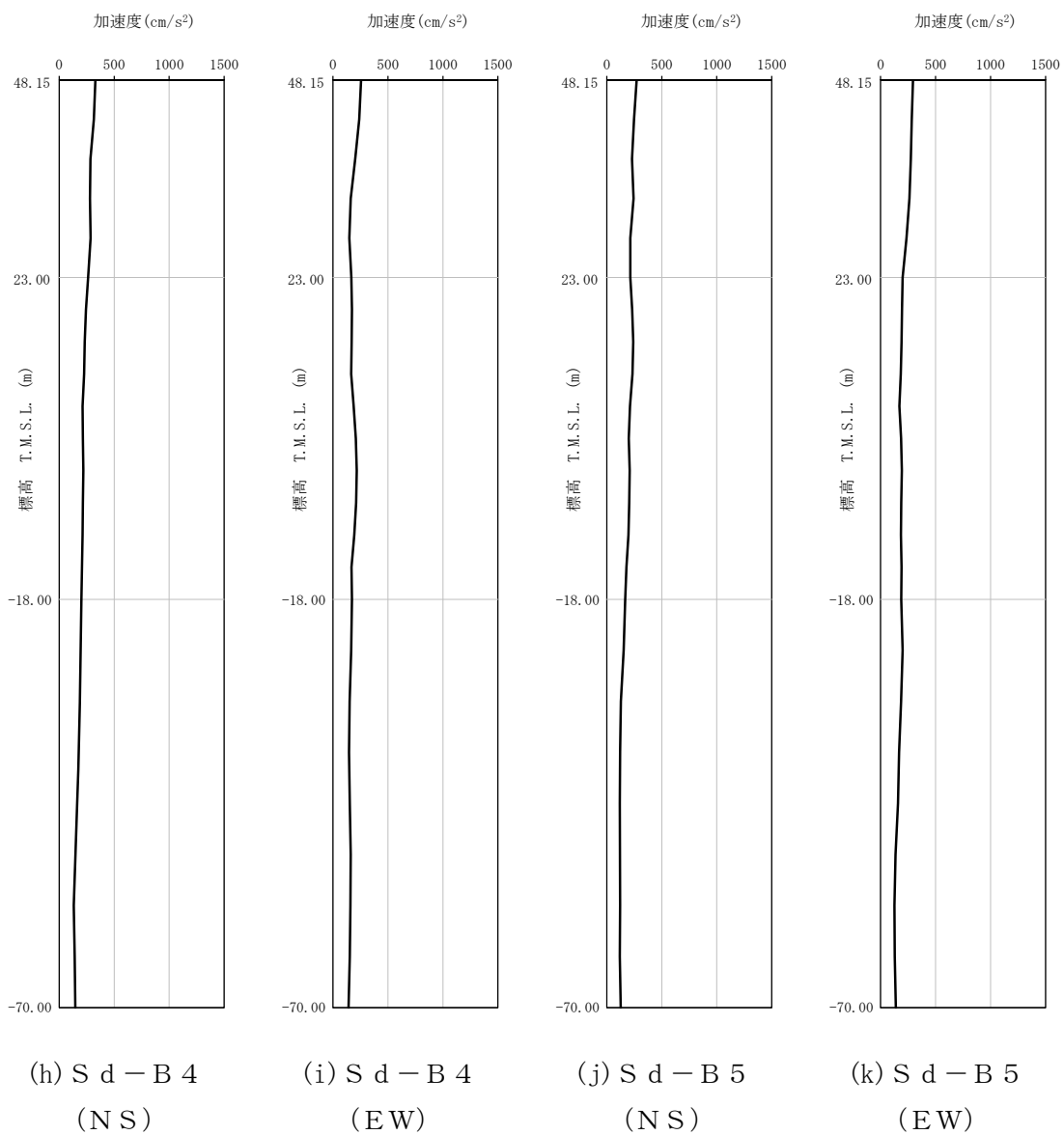
第 4-4 図 最大加速度分布 (S d ) (3/8)
