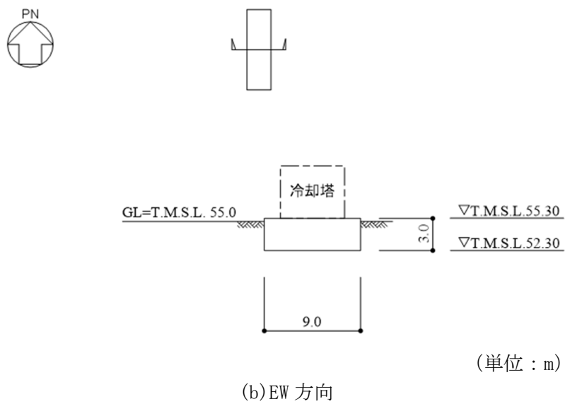
第 2.2-2 図 概略断面図
