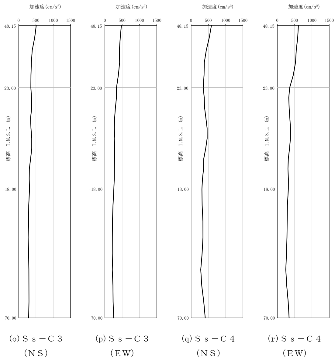
第 4-3 図 最大加速度分布 (S s ) (5/8)
