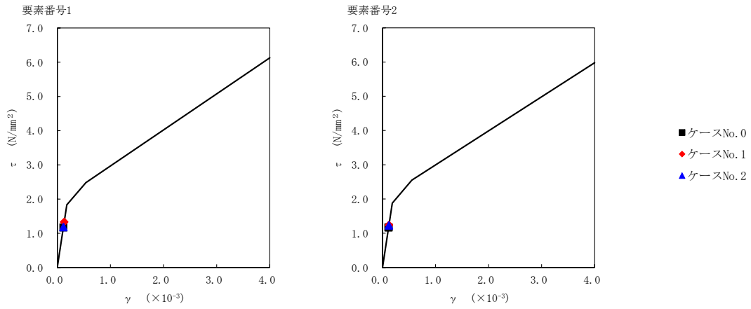
第 5.3-18 図 \tau - \gamma 関係と最大応答値 (S s - A (H) , EW 方向)
