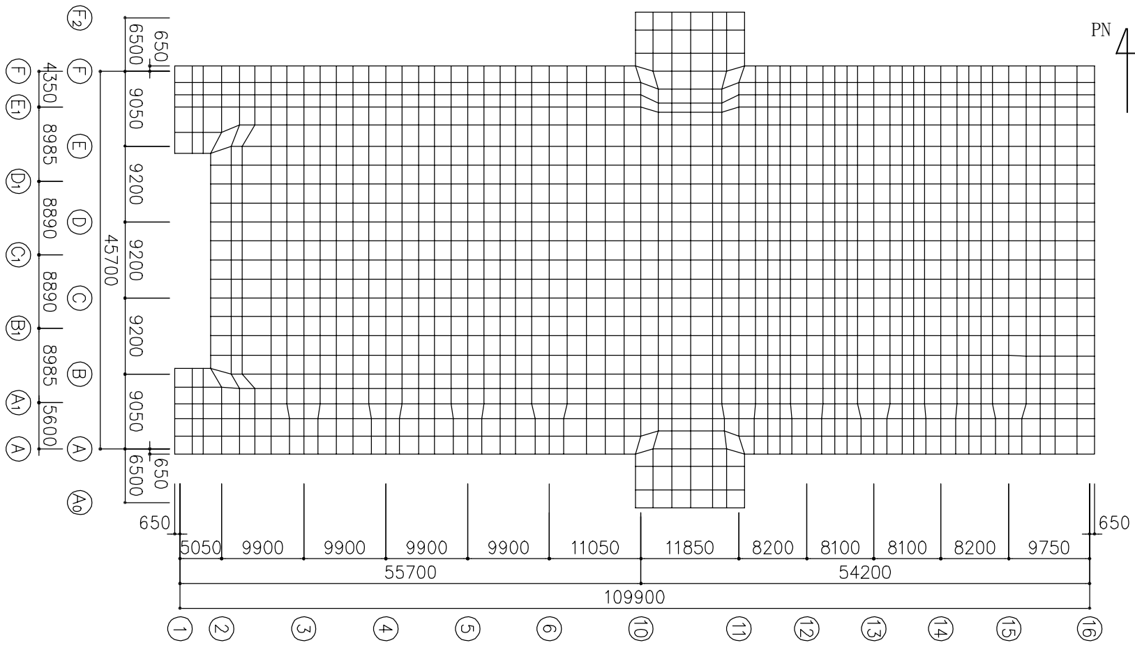
第 4.1-1 図 解析モデル (単位 : mm)
