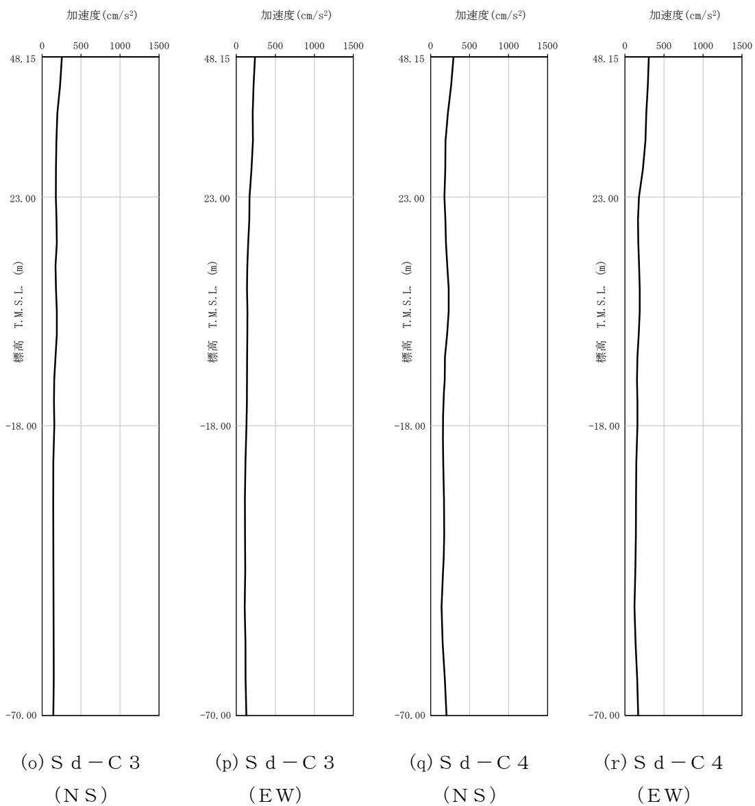
第 4-4 図 最大加速度分布 (S d) (5/8)
