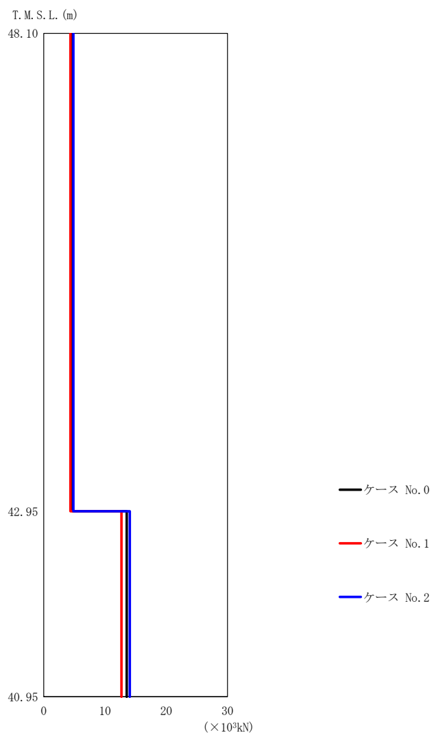
第 5.3-38 図 最大応答軸力（鉛直方向）（1/2）
