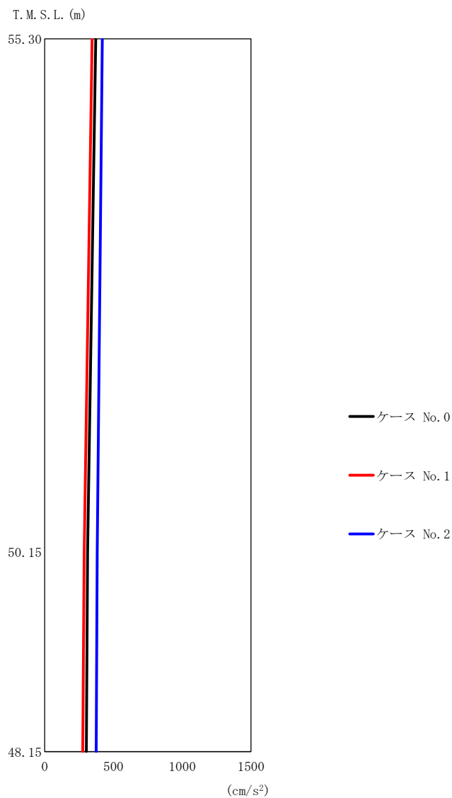
第 5.3-32 図 最大応答加速度 (NS 方向) (2/5)
