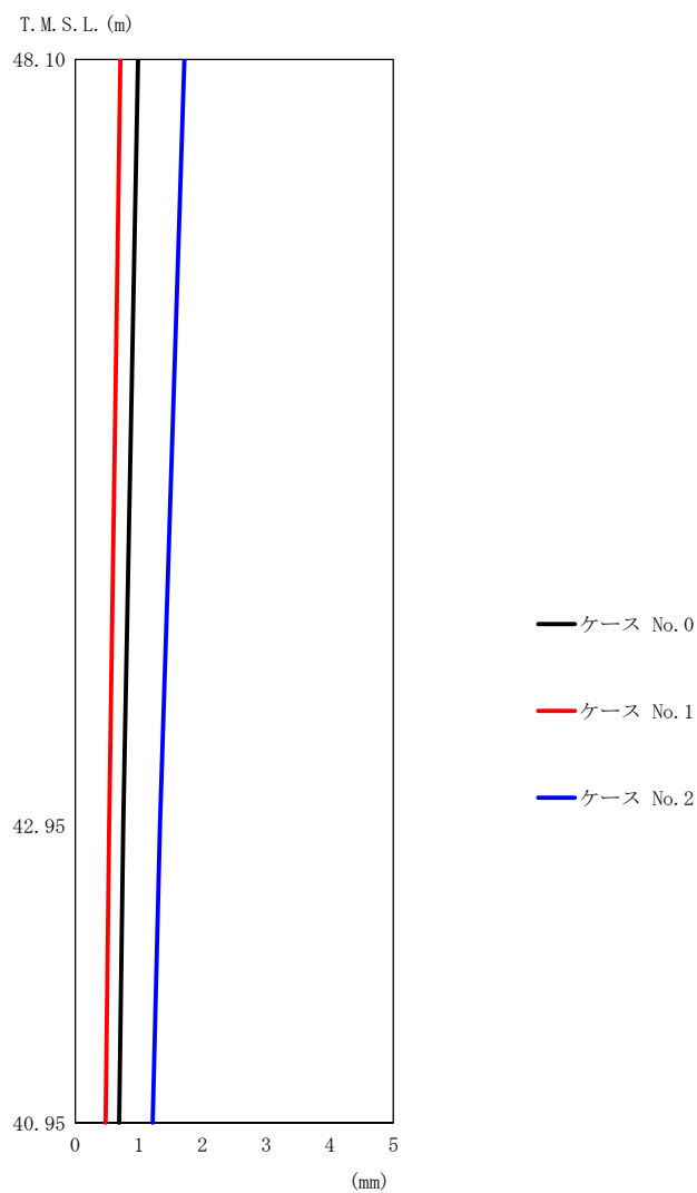
(d) S d - C 4 (EW)
