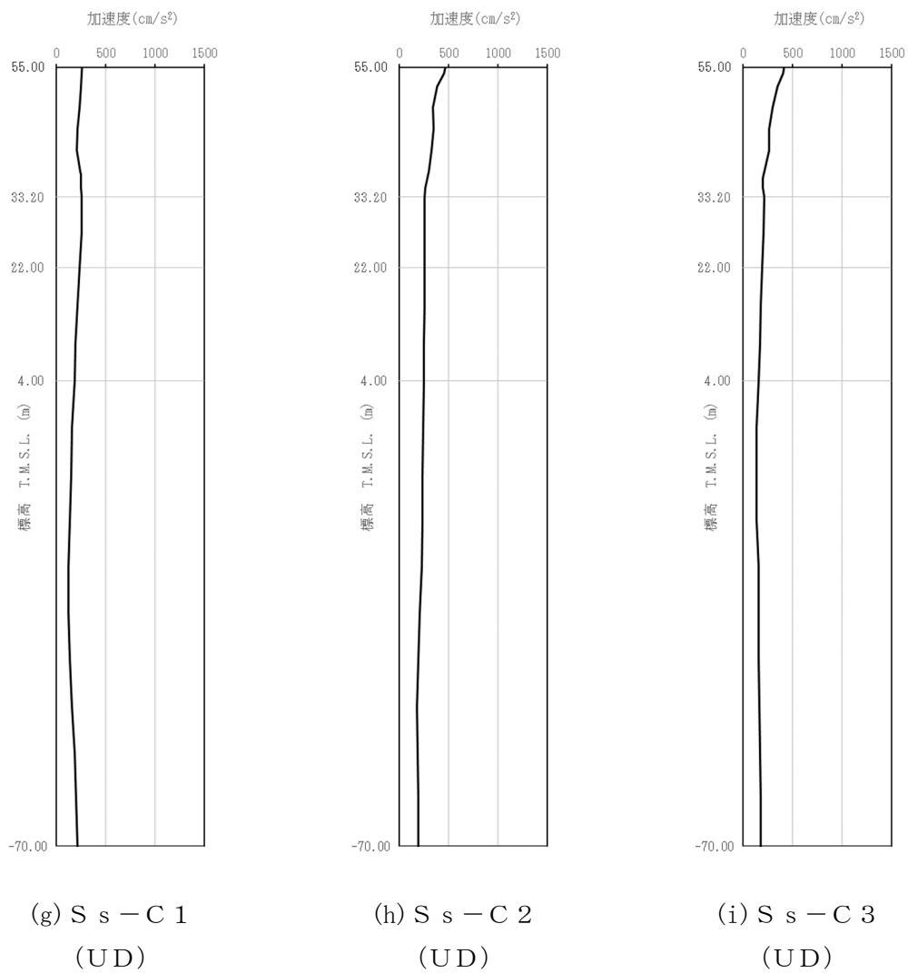
第 4-2 図 最大加速度分布 ( S_s ) (8/8)
