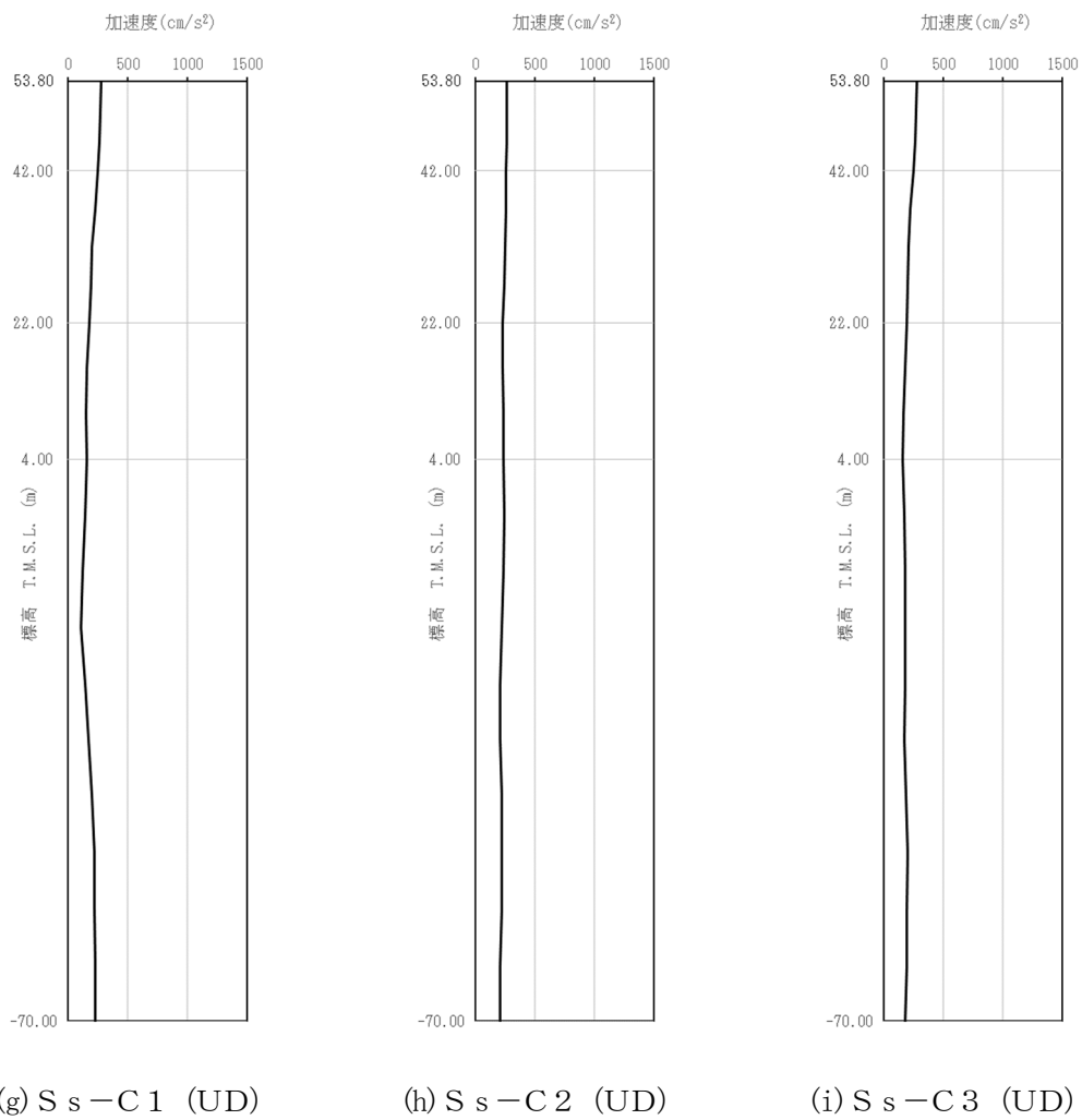
第 4-3 図 最大加速度分布 ( S_s ) (8/8)
