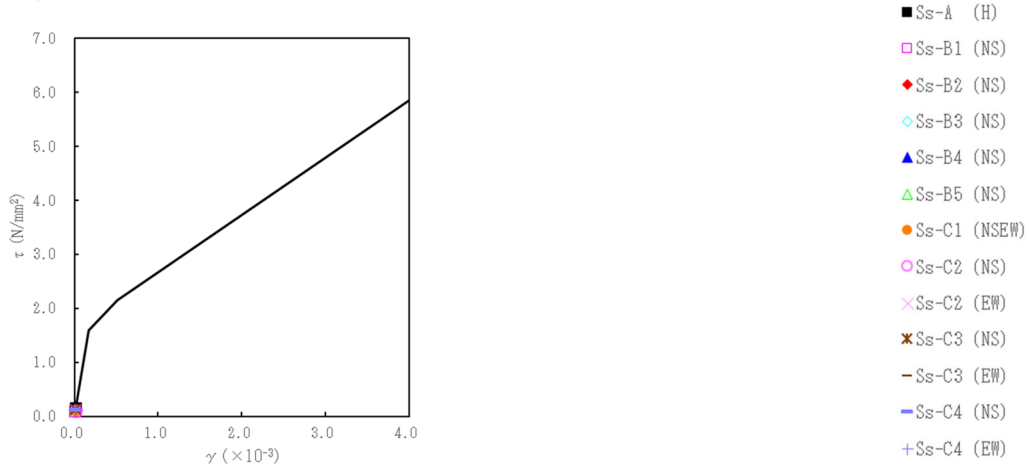
第 5.2-12 図 \tau - \gamma 関係と最大応答値 (基準地震動 S_s , ケース No. 0, NS 方向)
