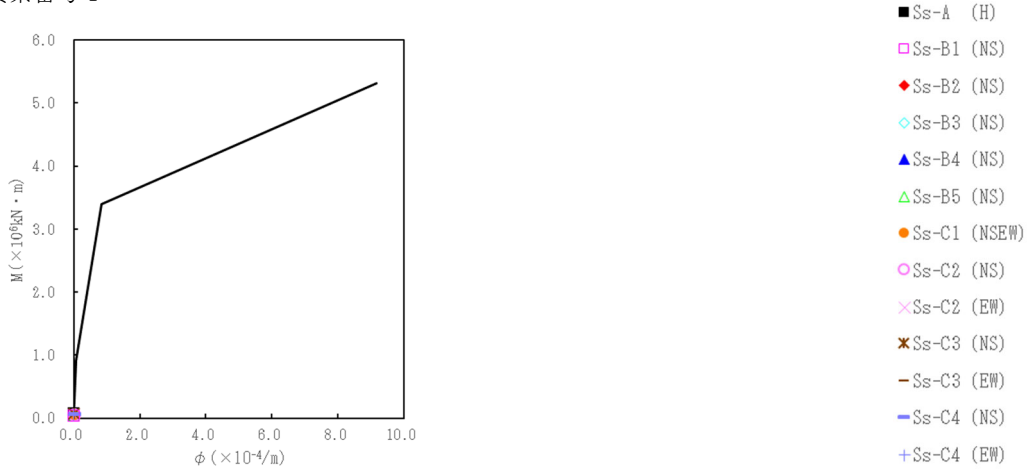
第 5.2-13 図 M - \phi 関係と最大応答値 (基準地震動 S_s , ケース No. 0, NS 方向)
