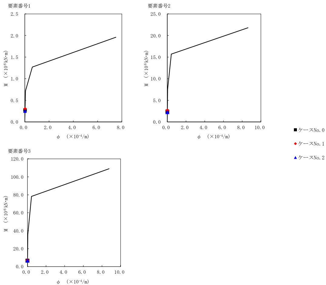
第 5.3-13 図 M-φ 関係と最大応答値 (S s -A (H), NS 方向)
