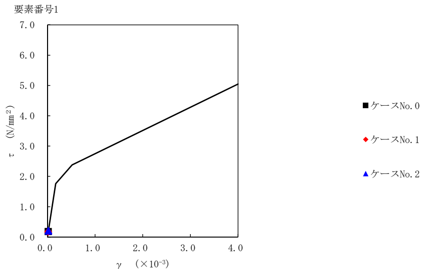
第 5.3-57 図 τ-γ 関係と最大応答値 (S d - C 4 (EW) , EW 方向)
