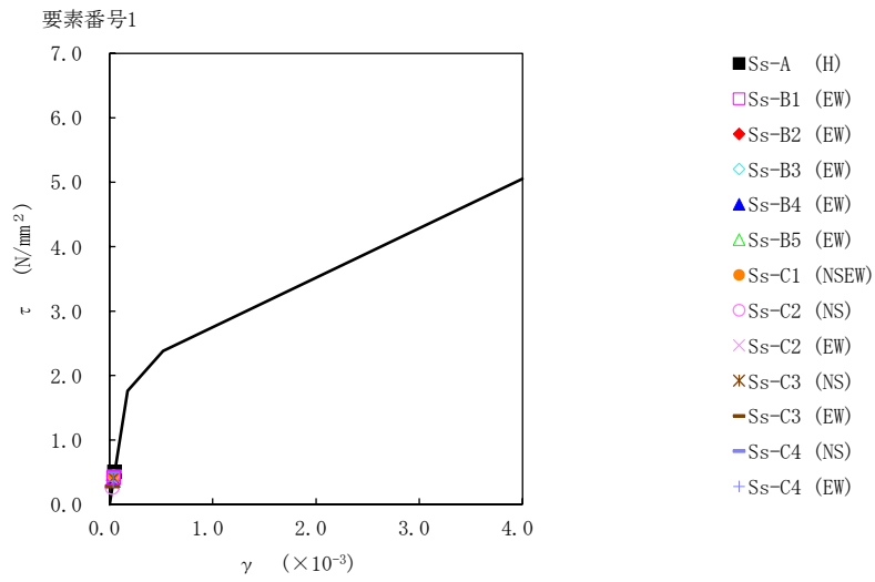
第5.2-14図 τ-γ 関係と最大応答値 (基準地震動 S s , ケース No.0, EW 方向)
