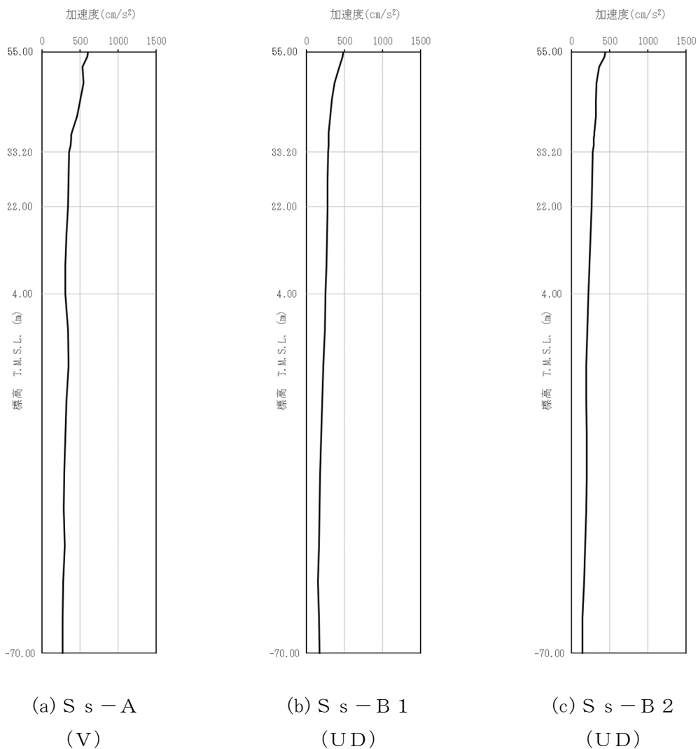
第 4-2 図 最大加速度分布 (S s) (6/8)
