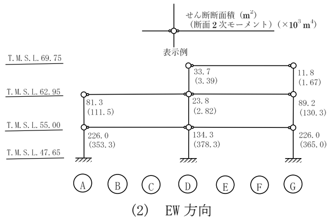
第 4.1-1 図 せん断力分配解析モデル
