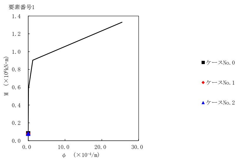
第 5.3-56 図 M-φ 関係と最大応答値 (S d - C 4 (NS) , EW 方向)
