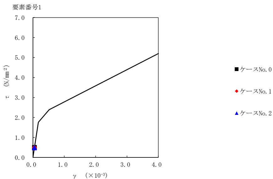
第 5.3-20 図 \tau - \gamma 関係と最大応答値 (S s - A (H) , EW 方向)
