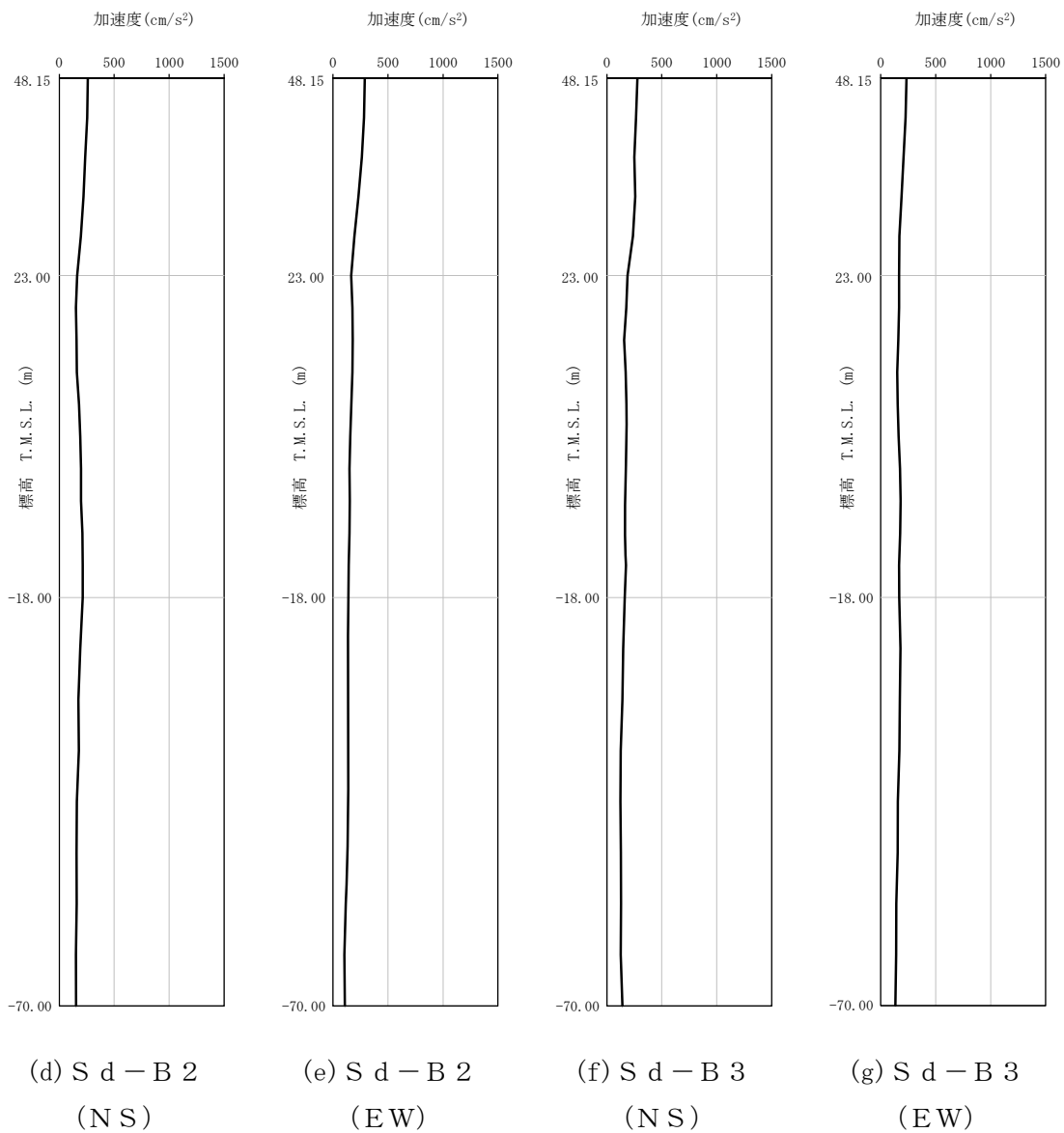
第 4-4 図 最大加速度分布 (S d ) (2/8)
