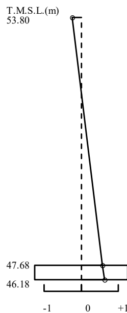
第 5.1-2 図 刺激関数図 (EW 方向)
