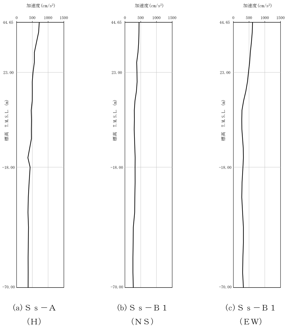
第4-2図 最大加速度分布 (Ss) (1/8)
