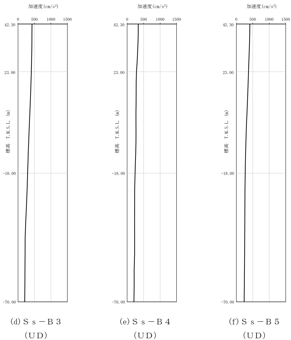
第 4-2 図 最大加速度分布 (S s ) (7/8)
