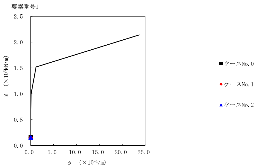
第 5.3-21 図 M- \phi 関係と最大応答値 (S s - A (H) , EW 方向)
