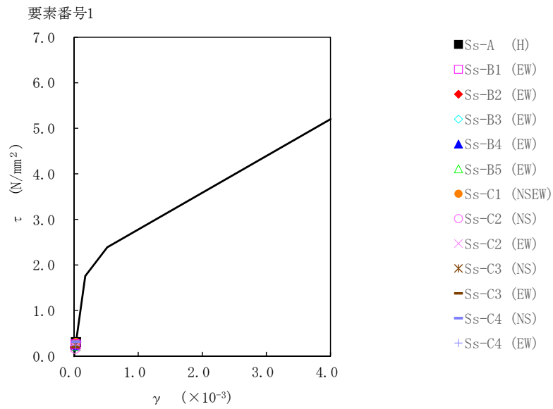
第 5.2-14 図 \tau - \gamma 関係と最大応答値 (基準地震動 S s , ケース No.0, EW 方向)
