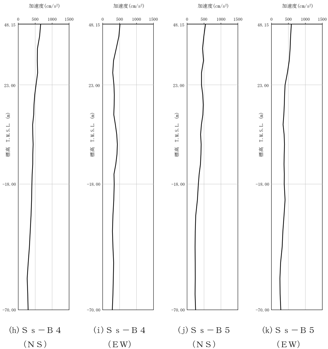
第 4-3 図 最大加速度分布 (S s ) (3/8)
