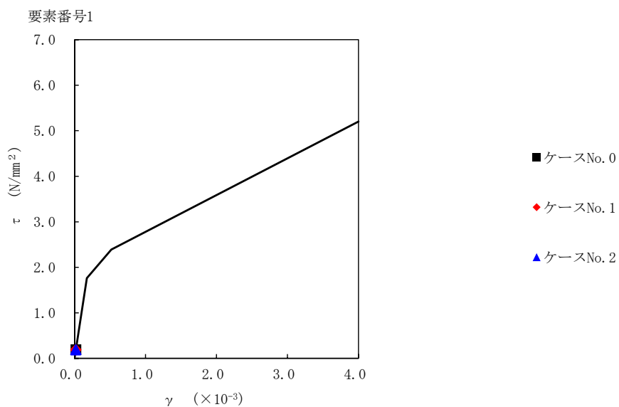
第 5.3-39 図 τ-γ 関係と最大応答値 (S d-A (H), NS 方向)
