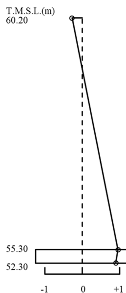
第 5.1-1 図 刺激関数図 (NS 方向)
