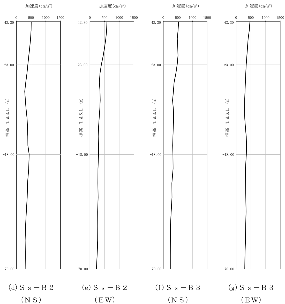
第 4-2 図 最大加速度分布 (S s ) (2/8)
