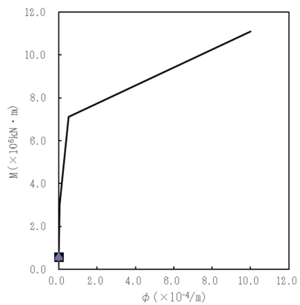
第 5.3-50 図 M- \phi 関係と最大応答値 (S d - C 1 (N S E W) , EW 方向)
