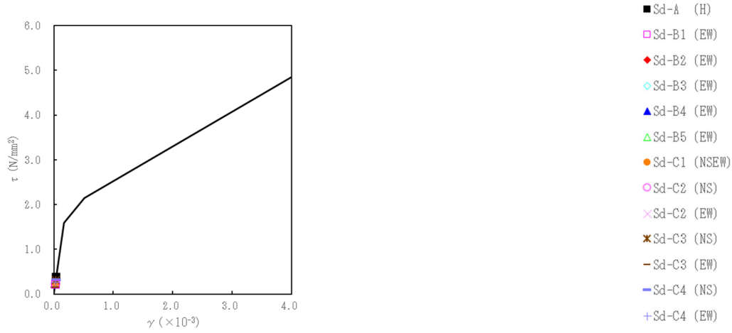
第5.2-29図 τ-γ関係と最大応答値 (弾性設計用地震動S d , ケースNo.0, EW方向)
