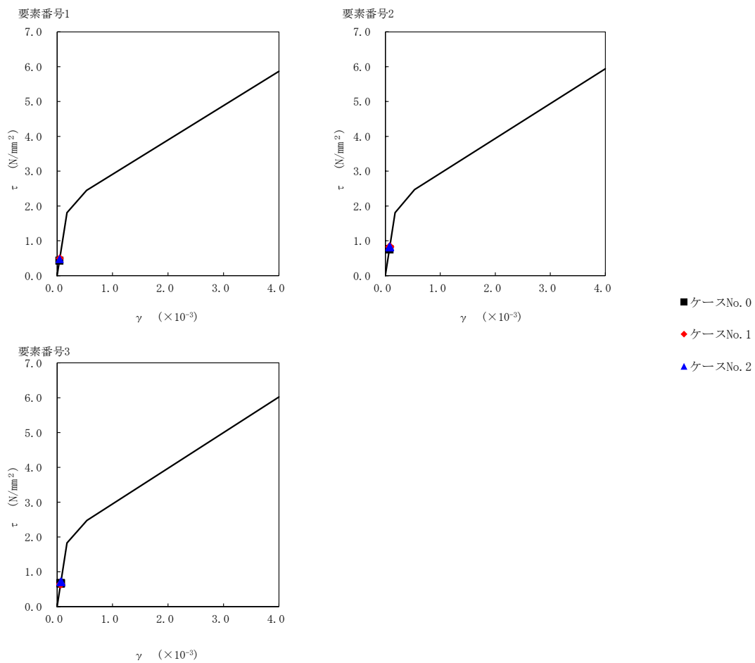
第5.3-20図 \tau - \gamma 関係と最大応答値 (S s -B3 (EW), EW方向)
