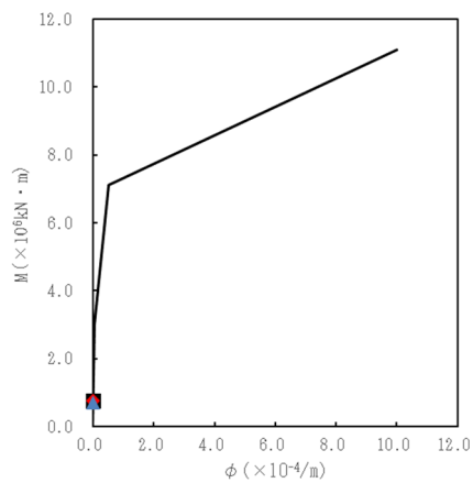
第 5.3-52 図 M- \phi 関係と最大応答値 (S d - C 4 (NS), EW 方向)
