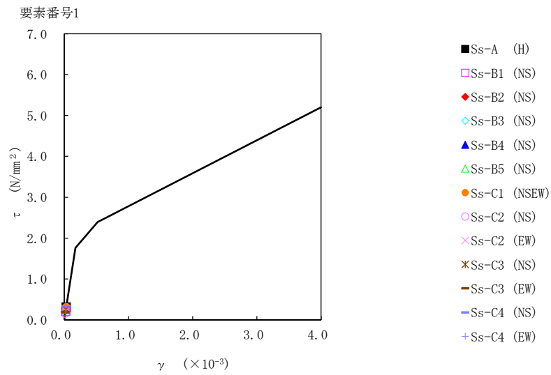
第 5.2-12 図 τ-γ 関係と最大応答値 (基準地震動 S s , ケース No. 0, NS 方向)
