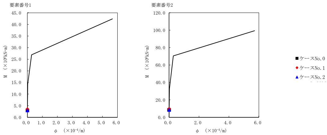
第 5.3-19 図 M - \phi 関係と最大応答値 (S s - A (H) , EW 方向)
