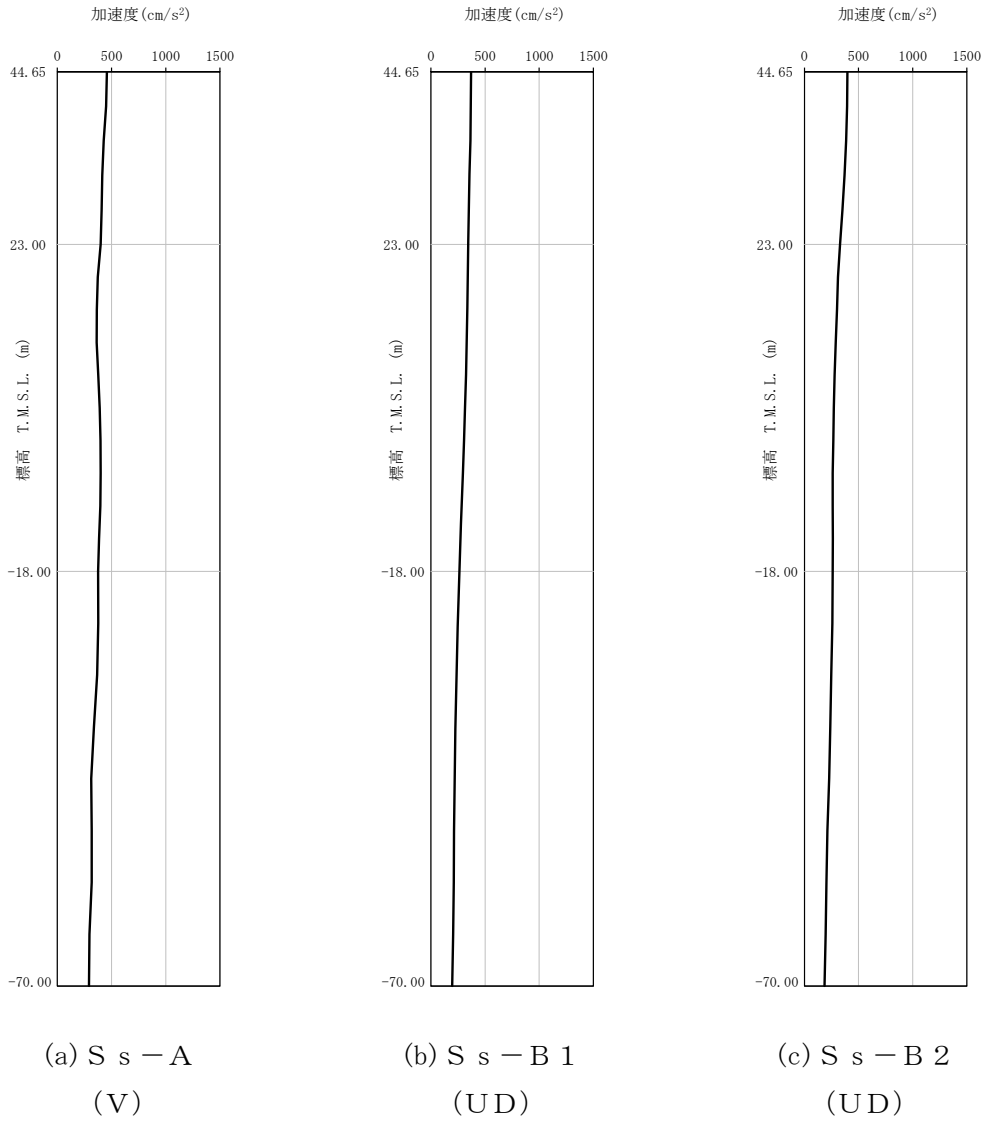
第4-2図 最大加速度分布 (S s ) (6/8)
