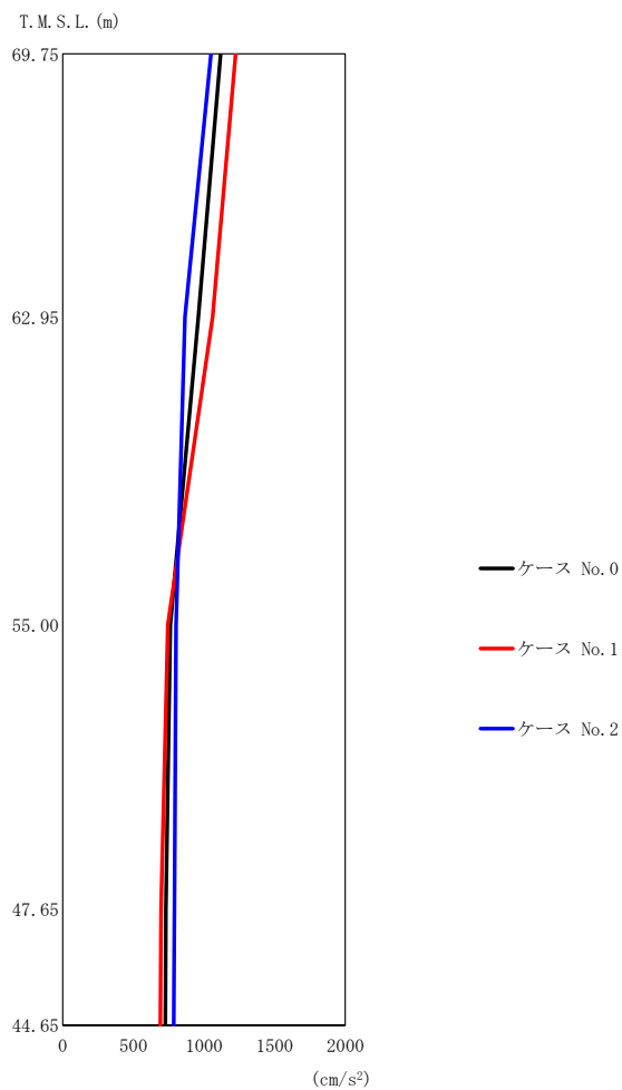
第 5.3-5 図 最大応答加速度 (EW 方向) (1/3)
