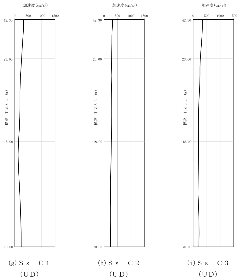
第 4-2 図 最大加速度分布 ( S_s ) (8/8)
