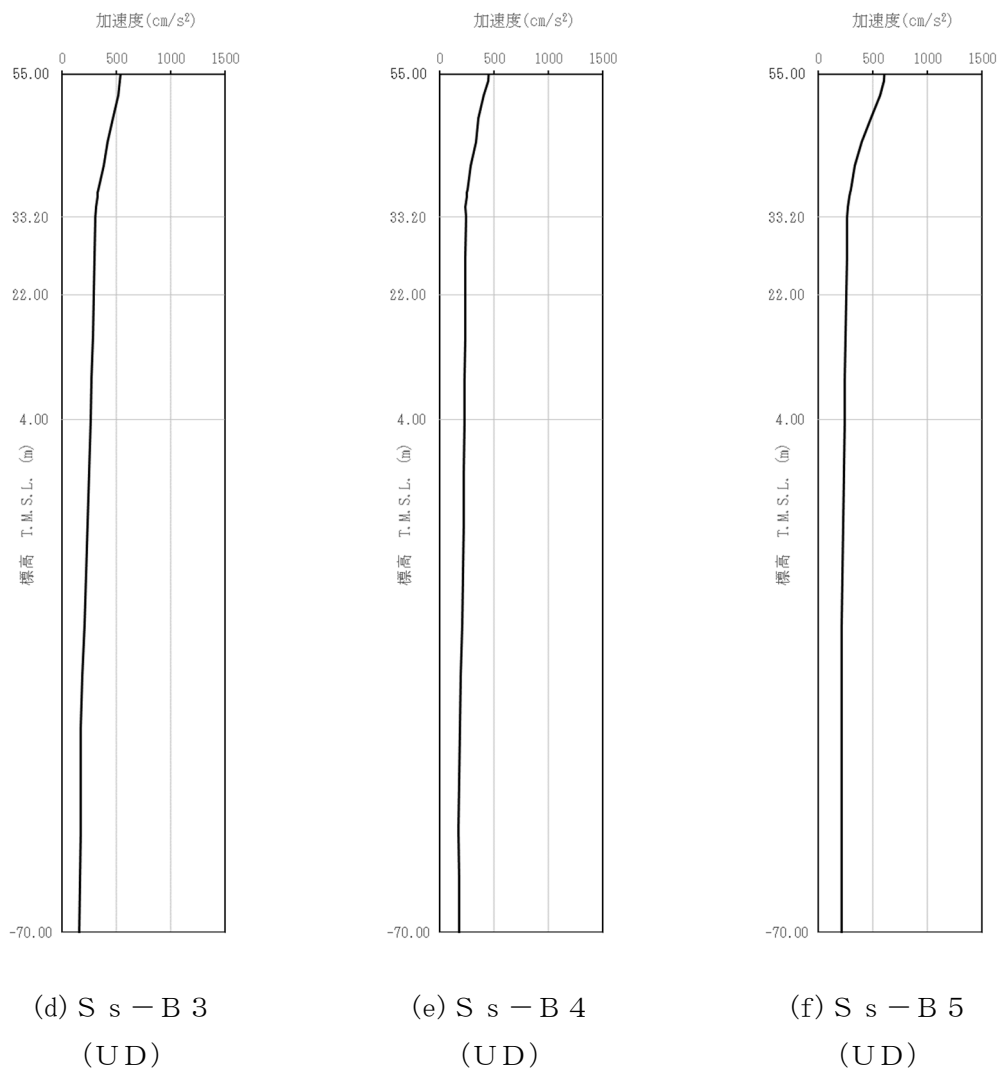
第4-2図 最大加速度分布 ( S_s ) (7/8)
