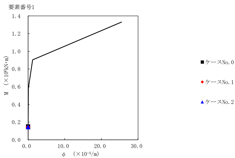
第 5.3-29 図 M-φ 関係と最大応答値 (S s -C4 (NS), EW 方向)
