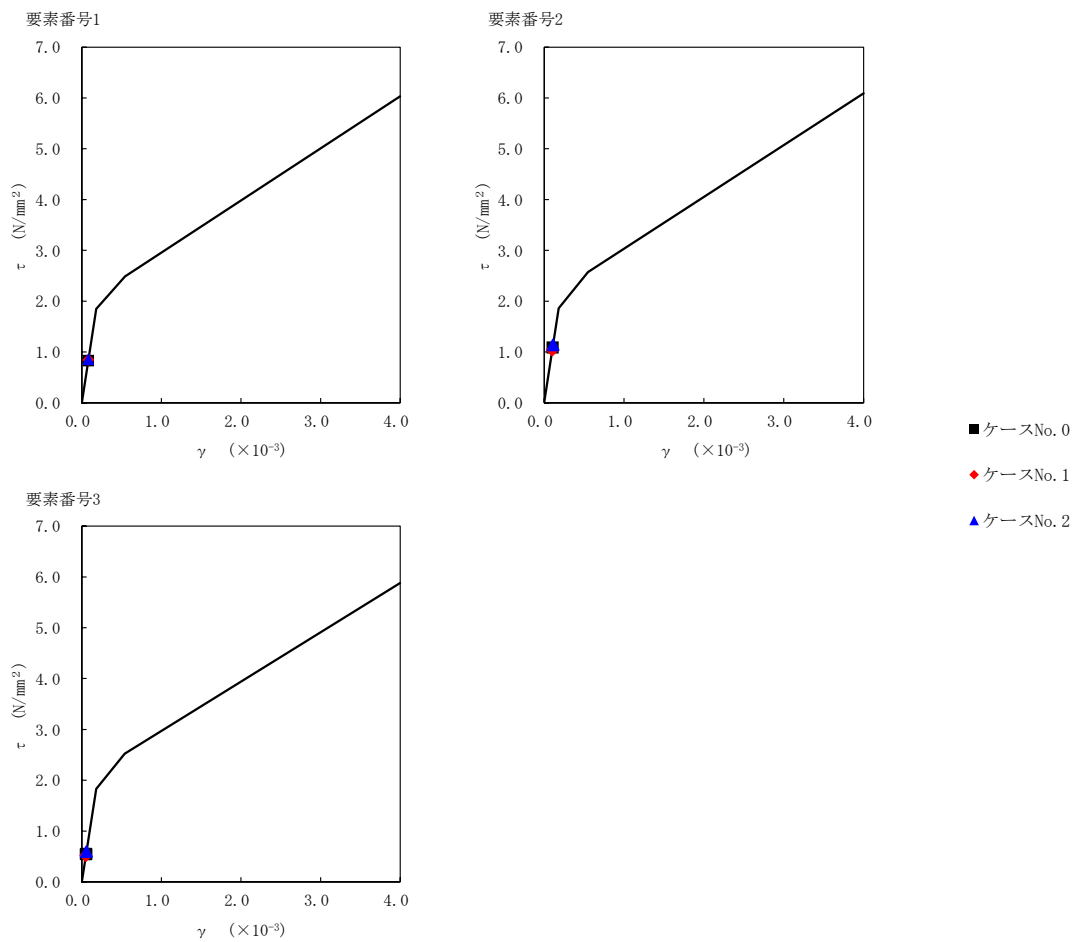
第 5.3-14 図 τ-γ 関係と最大応答値 (S s -B3 (NS), NS 方向)
