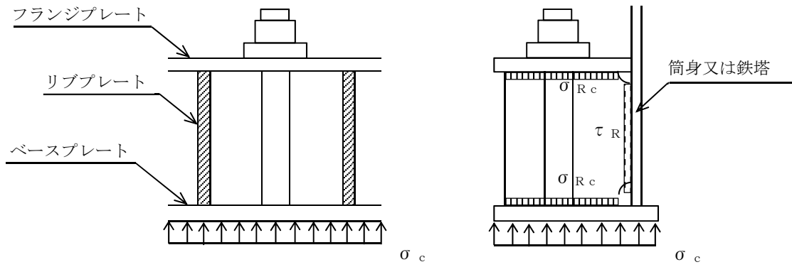
第 3.2-4 図 リブプレート応力算定説明図
