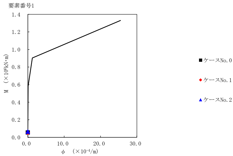
第 5.3-58 図 M-φ 関係と最大応答値 (S d - C 4 (EW) , EW 方向)
