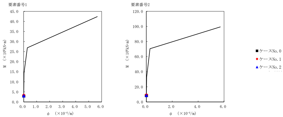
第 5.3-13 図 M- \phi 関係と最大応答値 (S s - A (H) , NS 方向)
