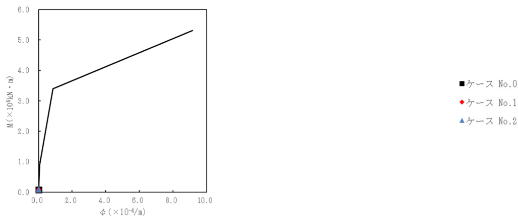
第 5.3-13 図 M-φ 関係と最大応答値 (S s - A (H) , NS 方向)
