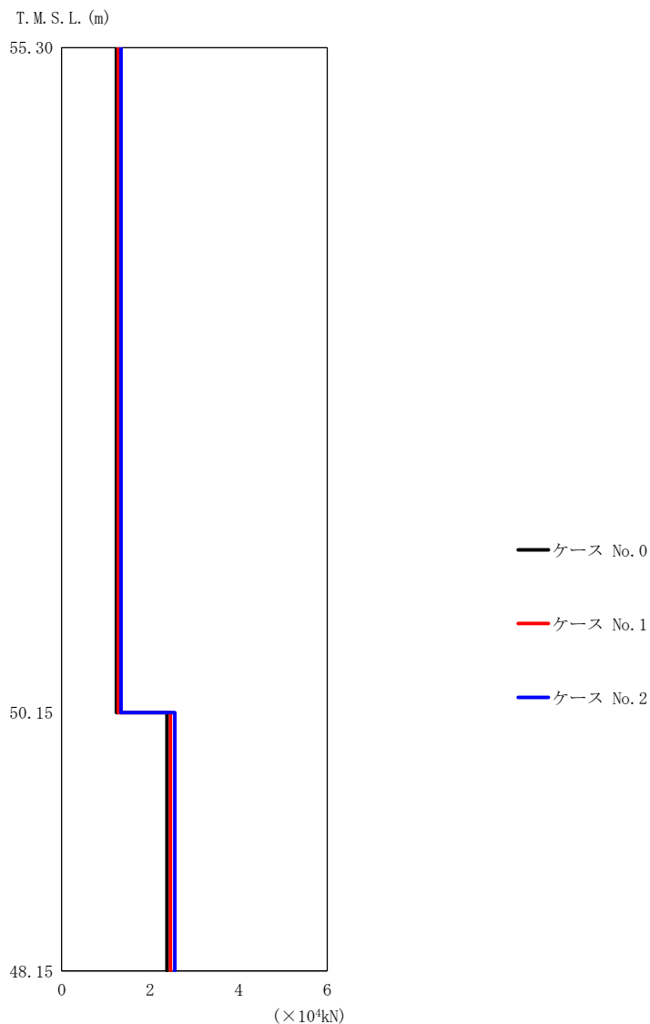
第 5.3-38 図 最大応答せん断力 (EW 方向) (1/5)
