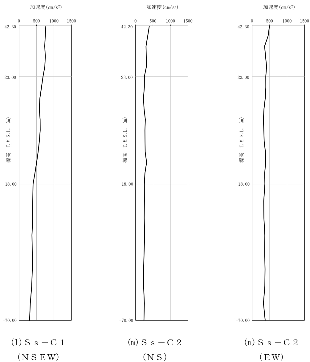
第 4-2 図 最大加速度分布 (S s) (4/8)
