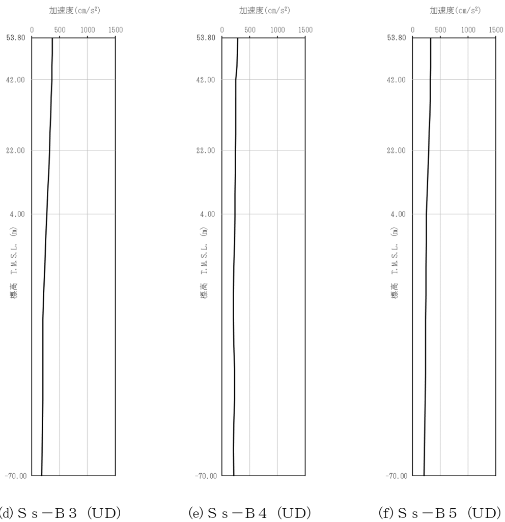
第 4-3 図 最大加速度分布 (S s ) (7/8)
