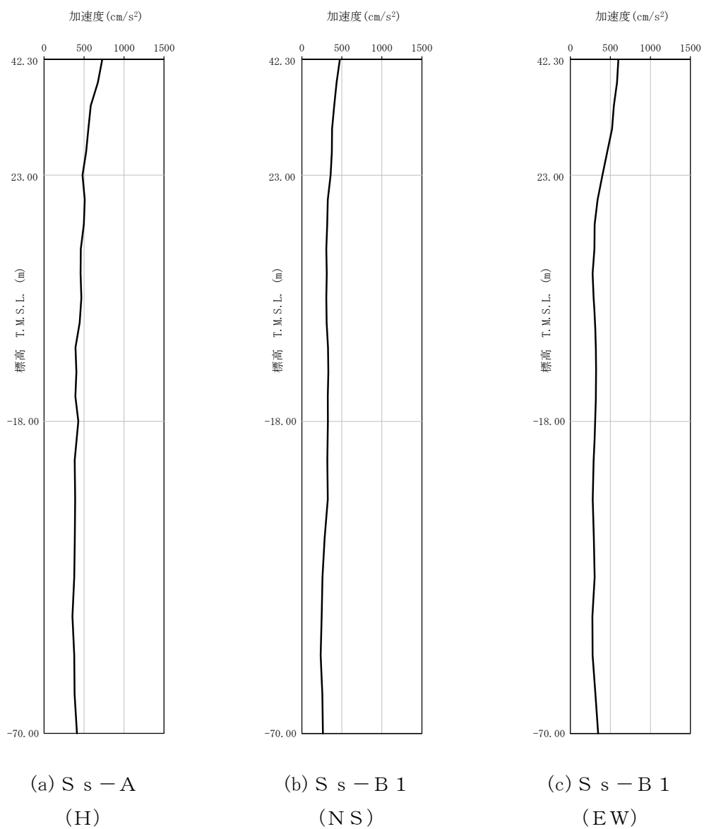
第 4-2 図 最大加速度分布 (S s ) (1/8)
