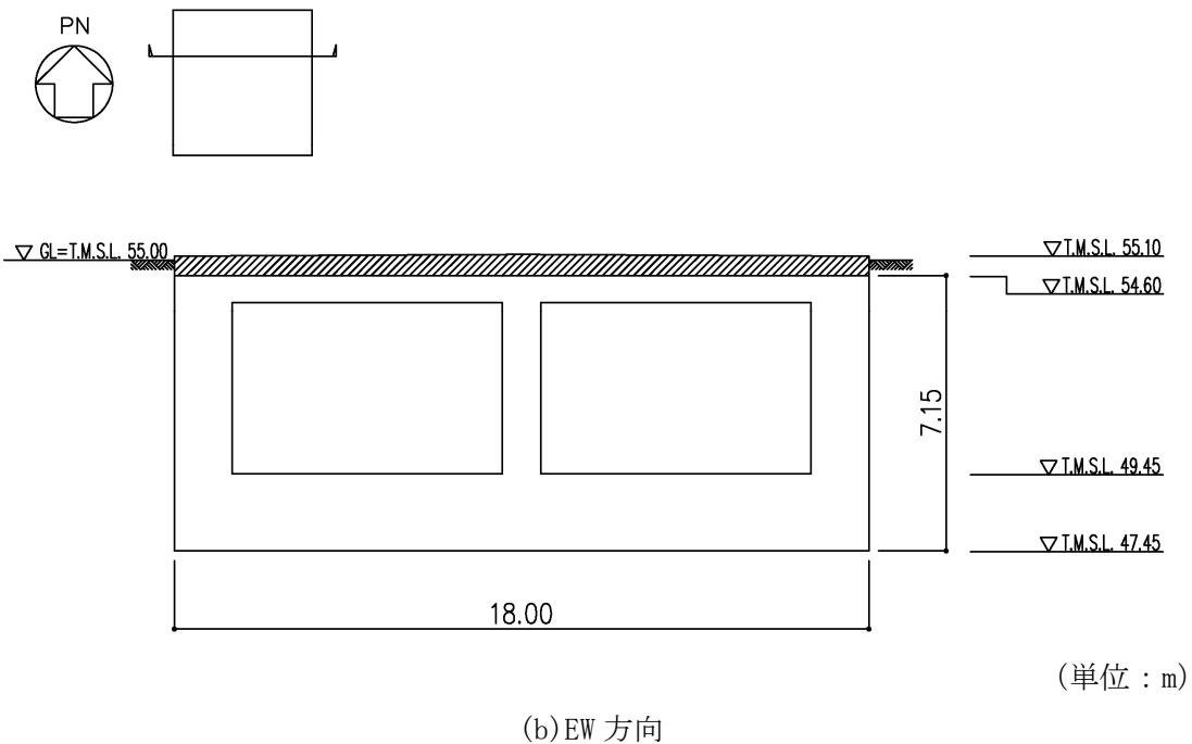
第 2.2-3 図 概略断面図
