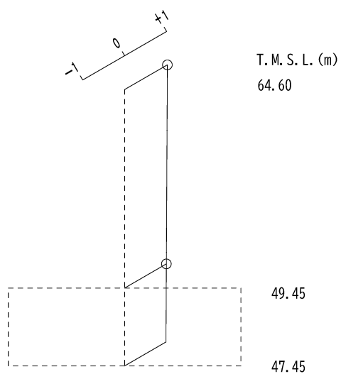
第 5.1-3 図 刺激関数図 (鉛直方向)
