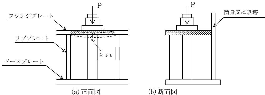
第3.2-3図 フランジプレート応力算定説明図
