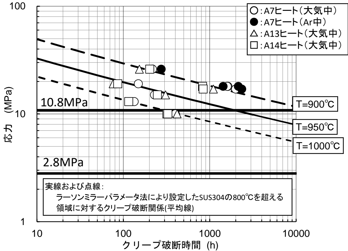
第 4.3.3.1. 16 図 SUS304のクリープ破断時間と応力の関係 (900°Cから 1,000°C)
