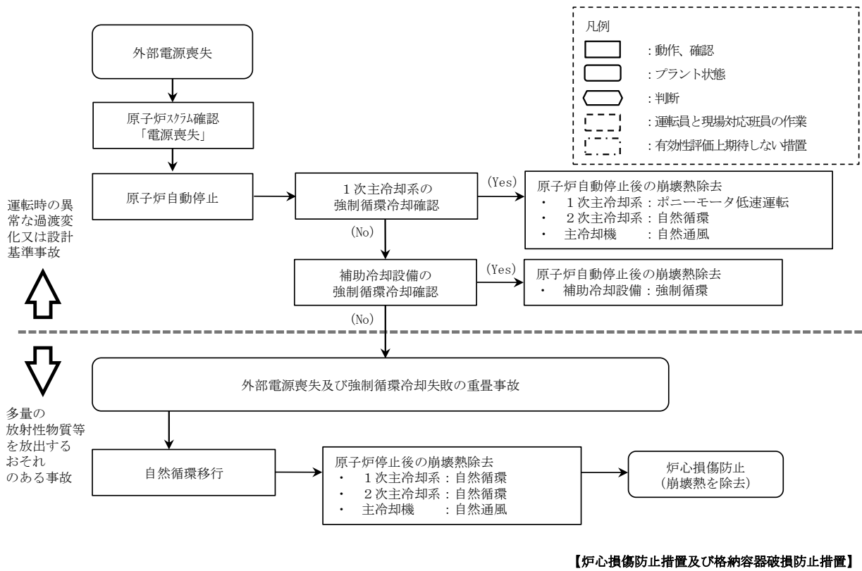
第 4. 3. 3. 12. 1 図 炉心損傷防止措置及び格納容器破損防止措置の対応手順の概要
