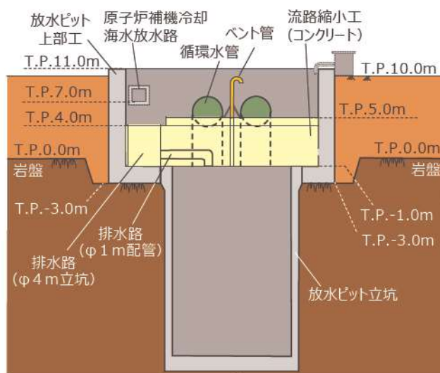
【B-B矢視】
