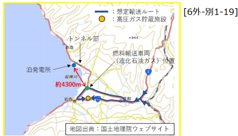
第2.2.2.3-2図 高圧ガス輸送車両火災想定位置と発電用原子炉施設との位置関係
