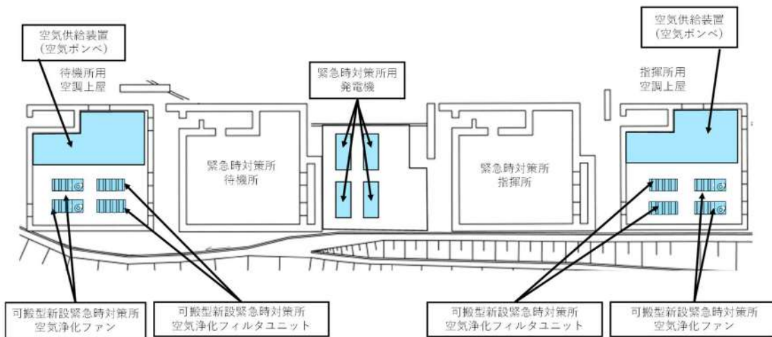
第1.18.5図 可搬型新設緊急時対策所空気浄化ファン，可搬型新設緊急時対策 所空気浄化フィルタユニット，空気供給装置（空気ポンペ）設置場所
