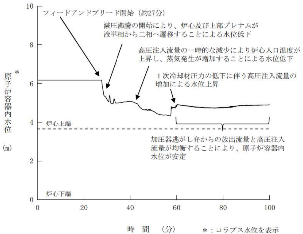
第 7.1.1.10 図 原子炉容器内水位の推移
