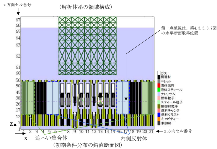
第 4.3.3.3.8 図 SIMMER-IVにおける初期物質分布
