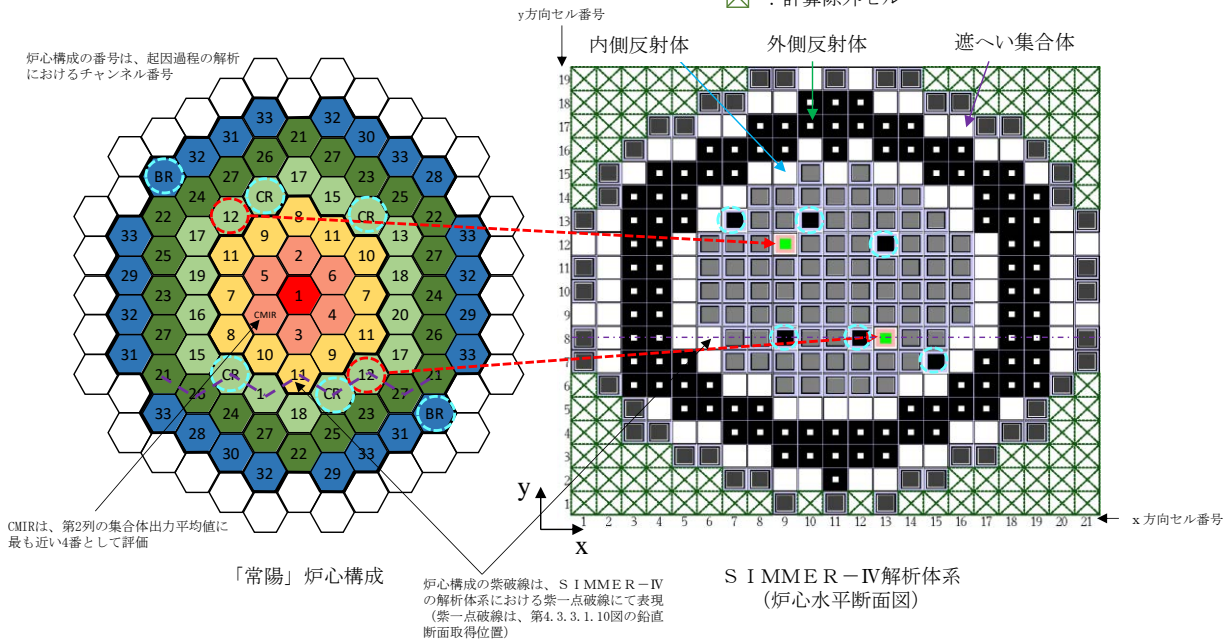
第4.3.3.1.9図 SIMMER-IVにおける解析体系 (遷移過程の解析)
