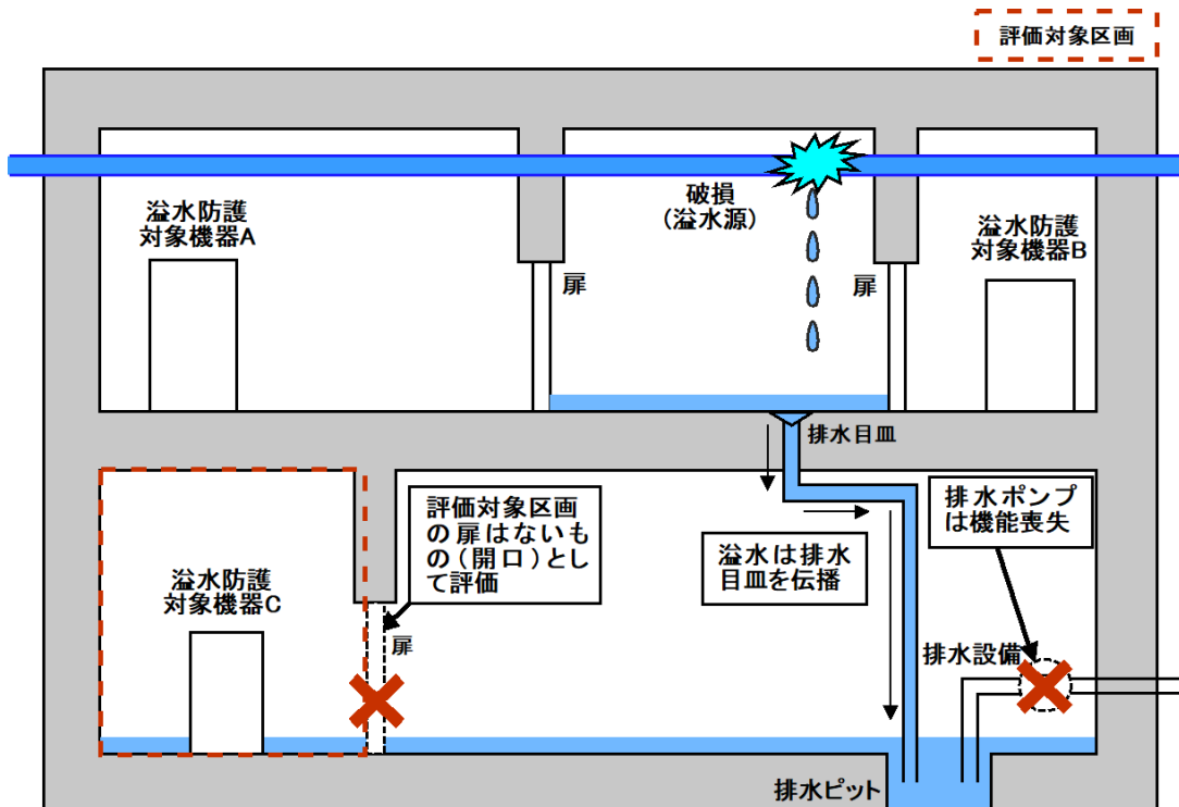
第1図 溢水経路の設定イメージ (3/4)
