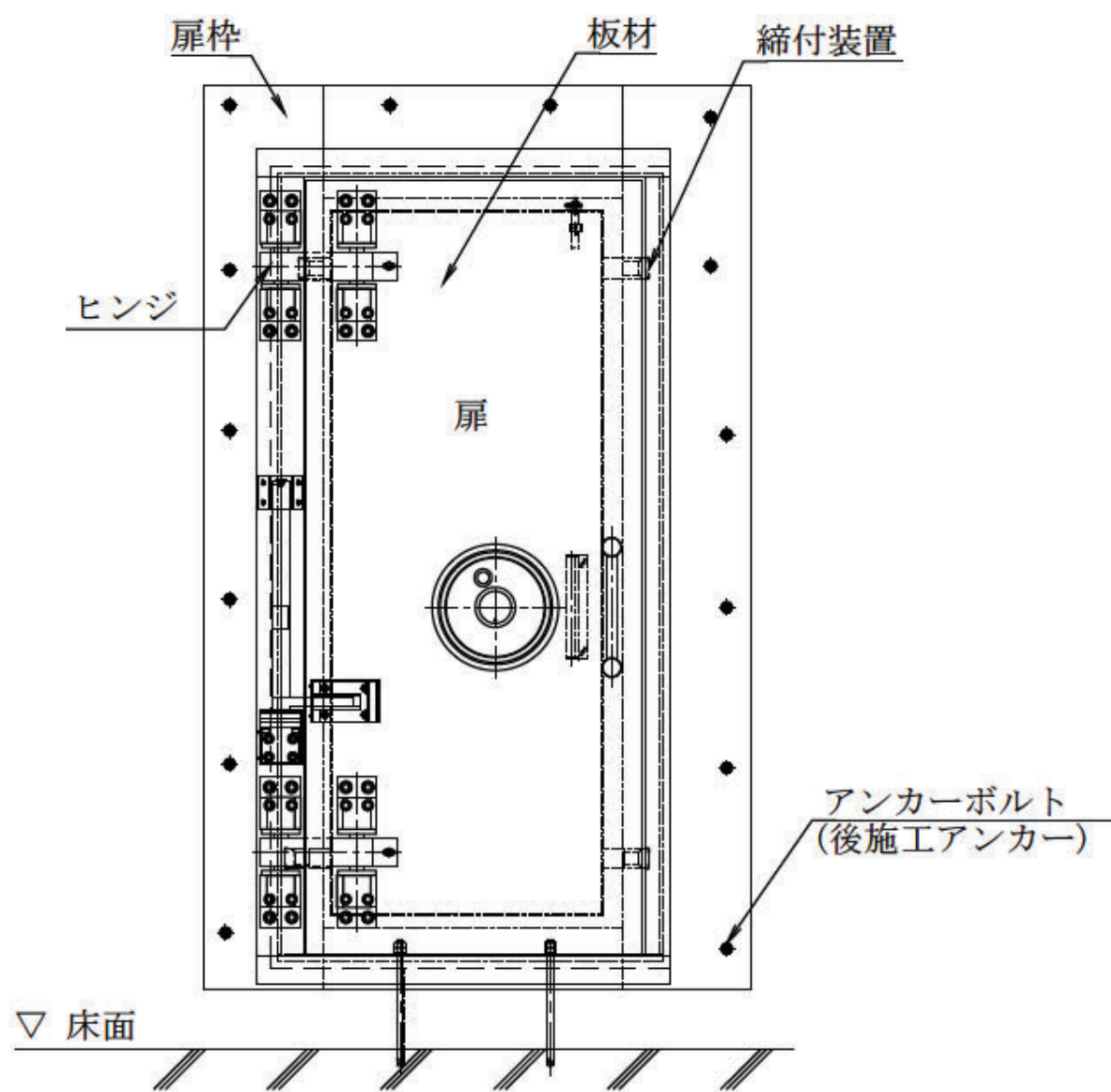
第4-2図 水密扉の概要図
