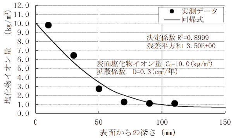
図1(7/9) 取水構造物海中帯 (SP-ci-2u-1) の回帰分析結果 (上：中性化考慮あり[○データを棄却]、下：中性化考慮なし)
