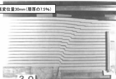
図-8 豊浦標準砂地盤における剪断層の発達過程 (Dv: 底盤の鉛直変位量) (基底の逆断層傾斜角: 75°, 地盤の層厚: 400mm)
