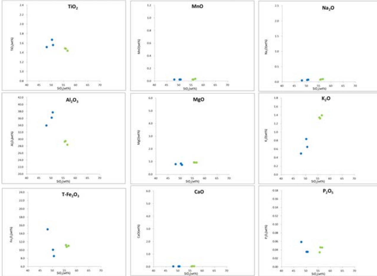
ハーカ一図
