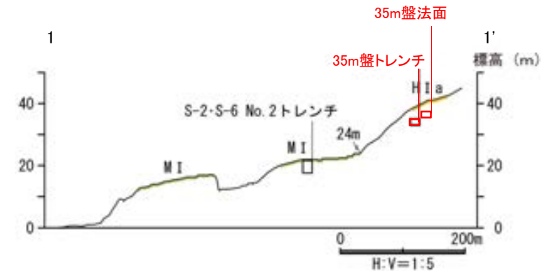
地形断面図
