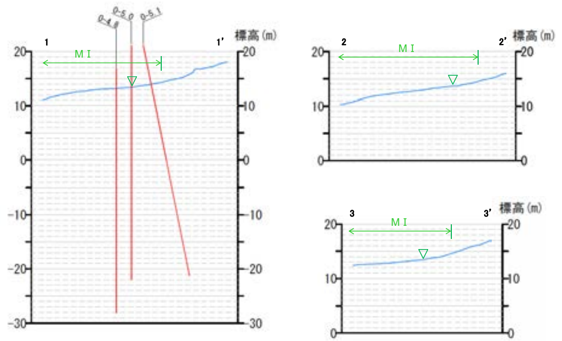
旧地形 S-2・S-6延長位置(地表) ボーリング孔
