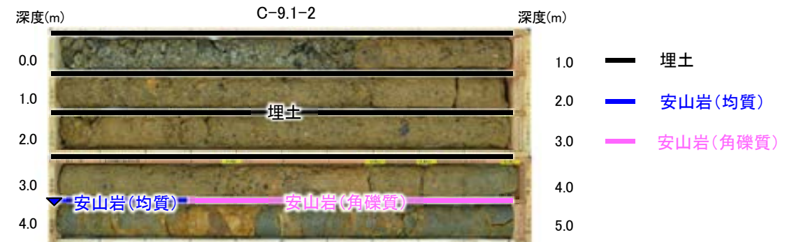
コア写真(深度0~5m) ▼ 埋土と安山岩(均質)の境界 (EL19.36m)
