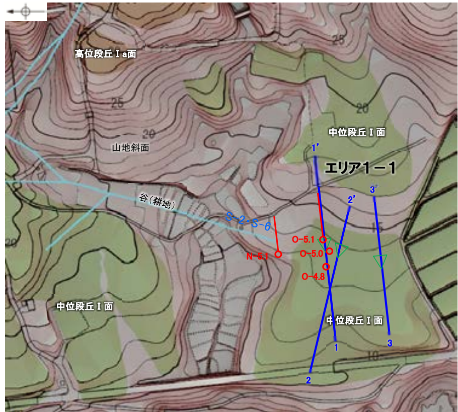
位置図(エリア1-1) 断層(地表に投影) 断面線 S-2・S-6延長位置(地表) 鉛直ボーリング 斜めボーリング
