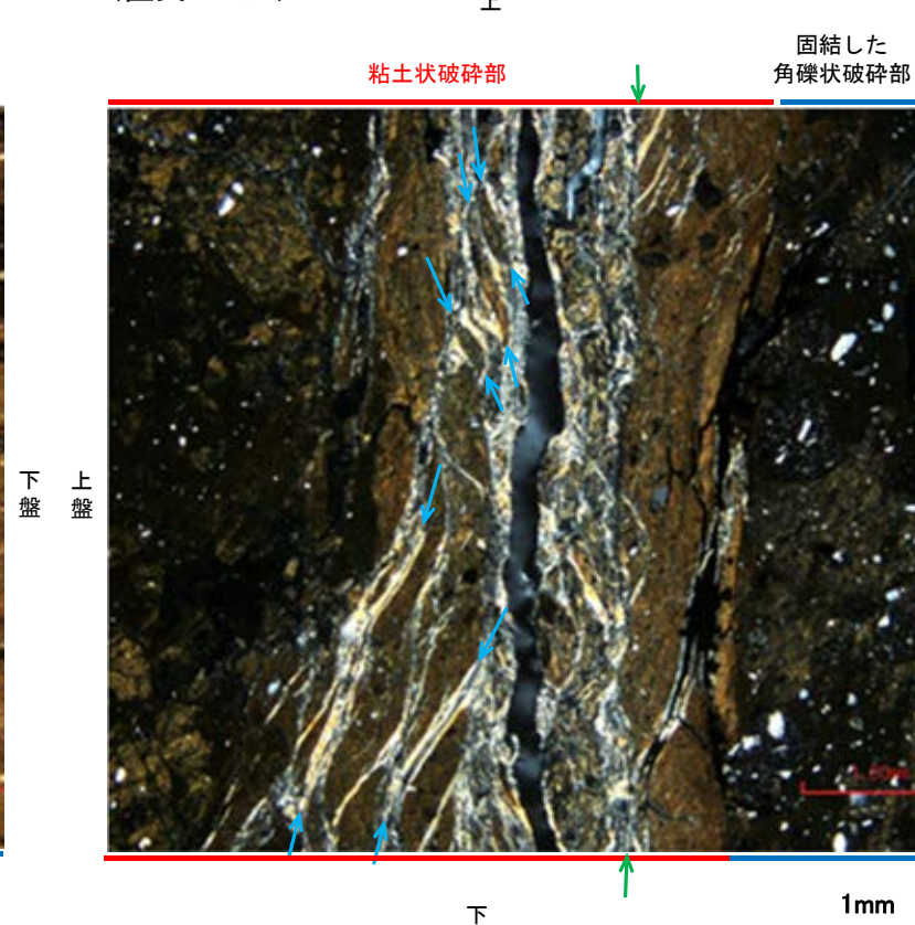
(直交ニコル)
