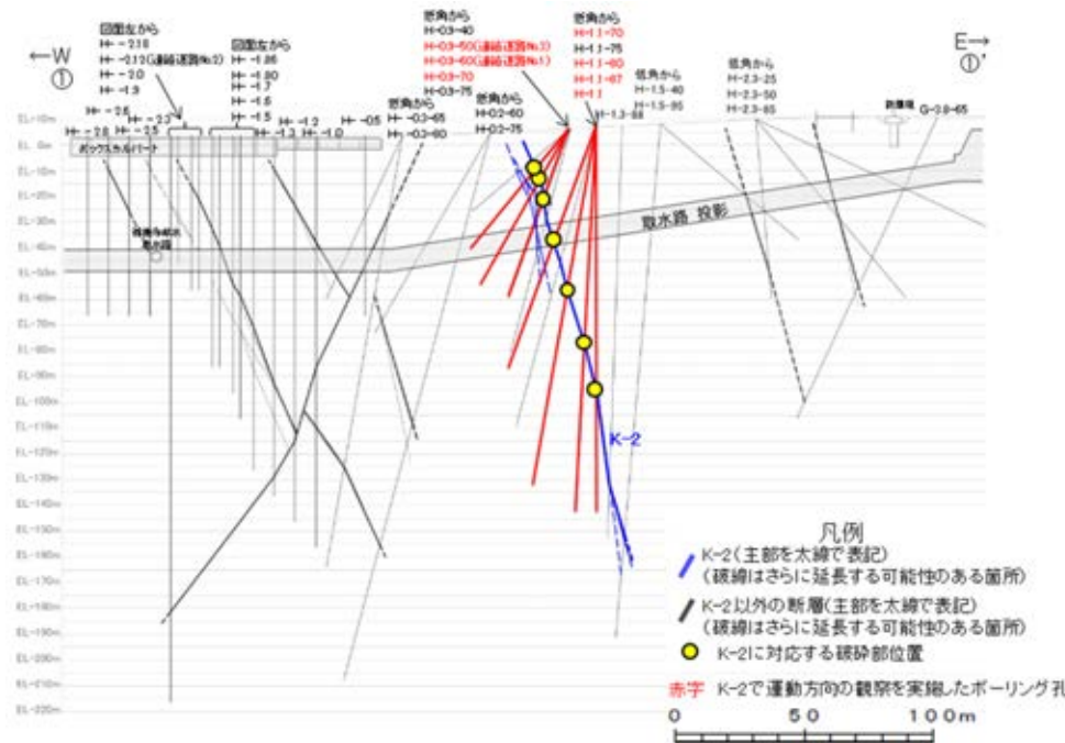
①-①'断面図
