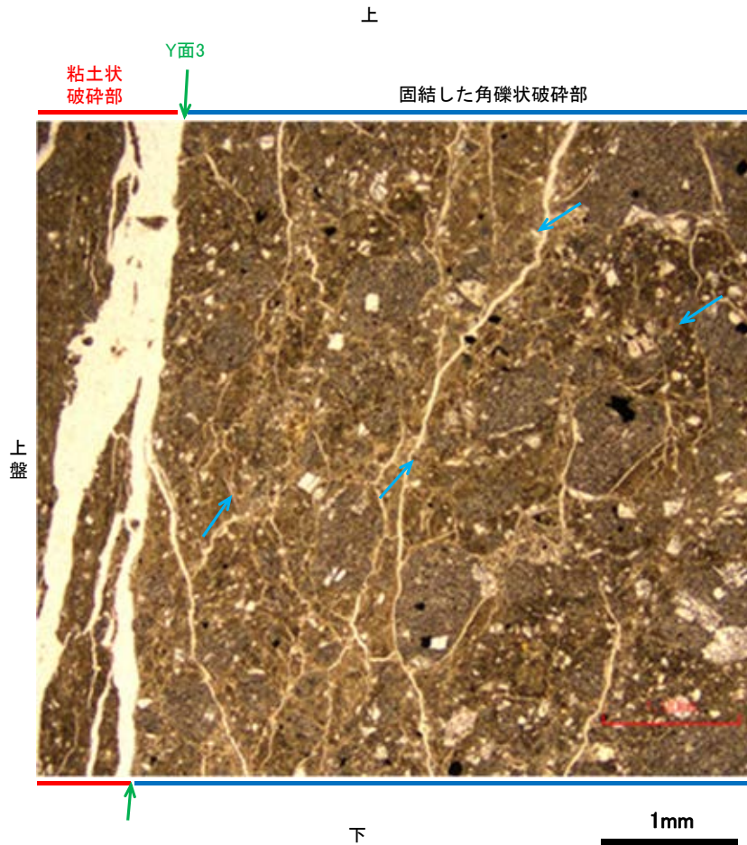
(単ニコル)
