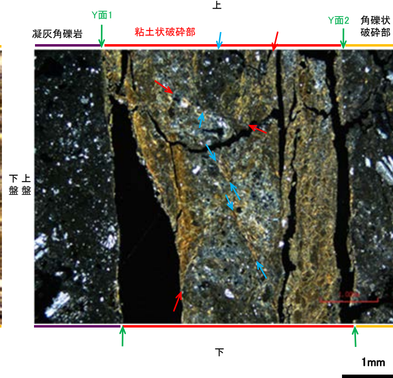
(直交ニコル)
