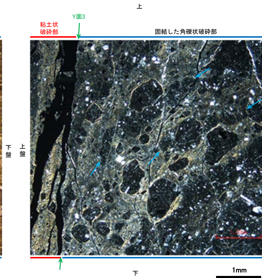
(直交ニコル)
